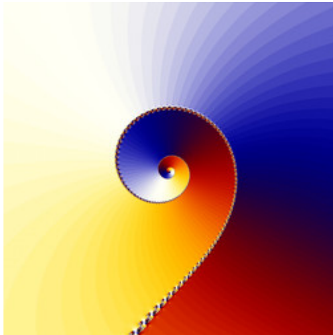
mt-newton-error-03b.jpg
