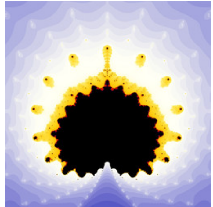
mt-modulate-mset-02.jpg
