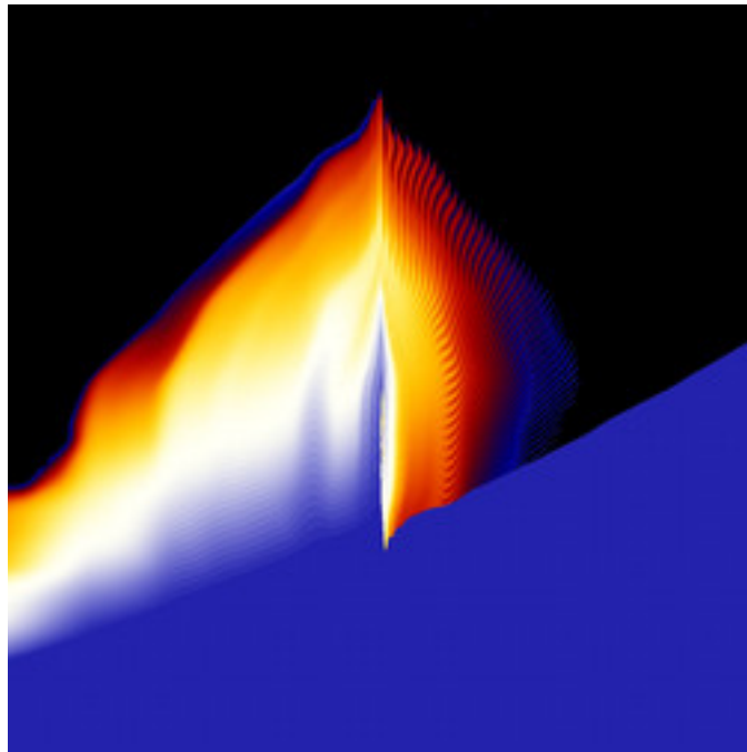
lkm3-FourierPopCorn-15B.jpg
