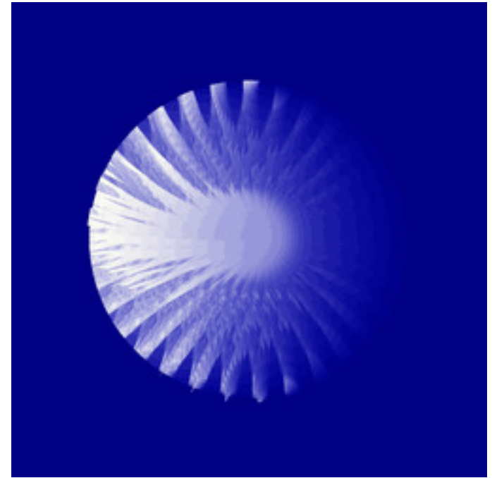
reb-PseudoZeePi-01.jpg
