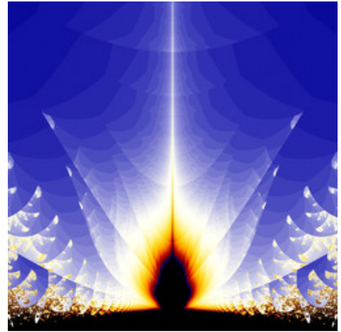
mt-barnsleyishMest-01.jpg
