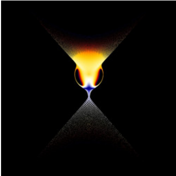
mt-zeepop-mset-04.jpg
