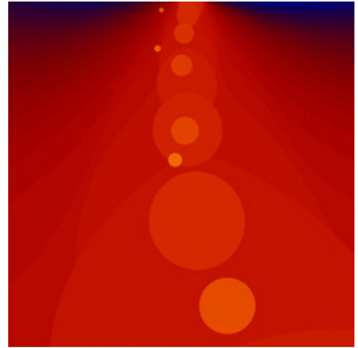
dmj-PhoenixDoubleNova-16.jpg
