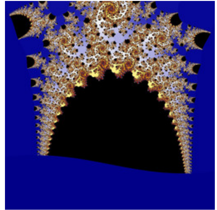
reb-GopalsamyExp-01.jpg
