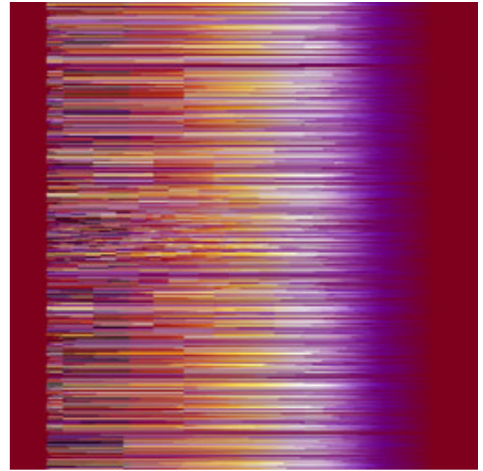
mt-GeneralizedCelticJulia-61.jpg
