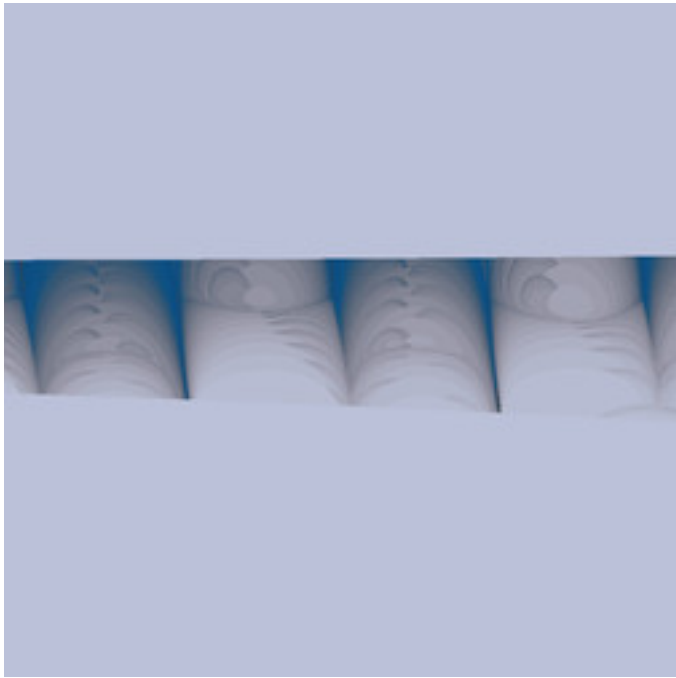
asz-andrextrandom-1-06.jpg
