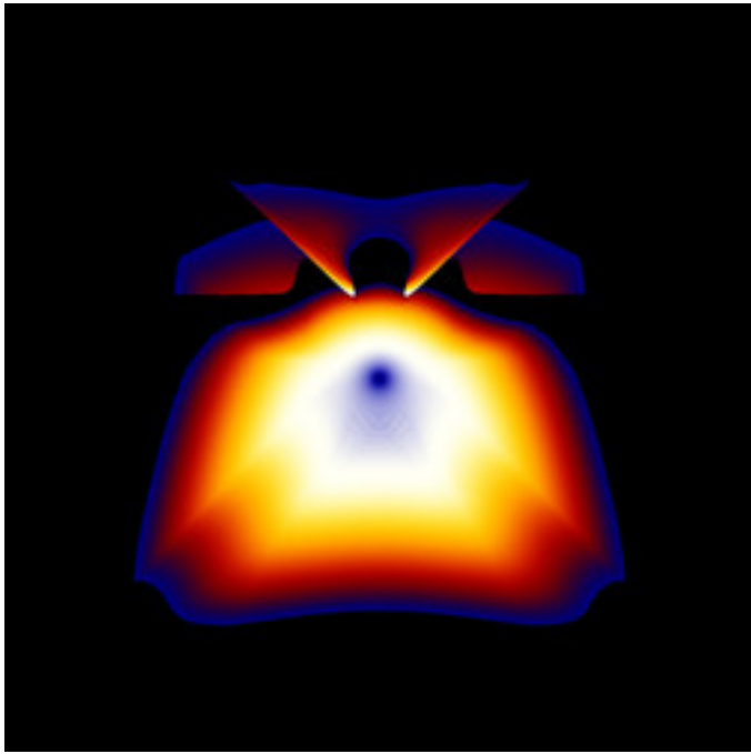
mt-zeepop-mset-01.jpg
