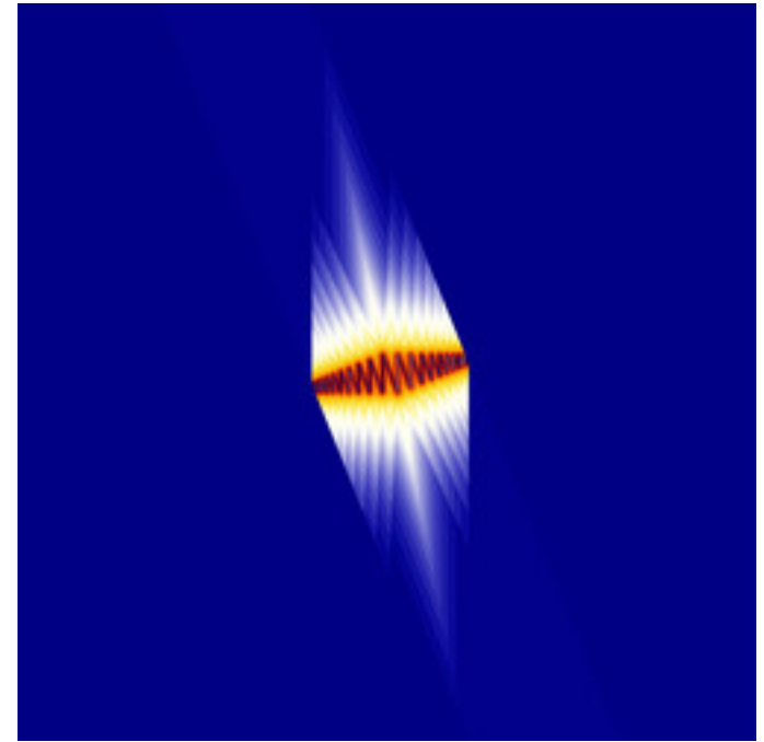
reb-FunBarnsley1Julia-02.jpg
