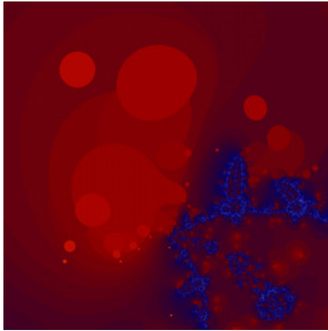
dmj-PhoenixDoubleNova-23.jpg
