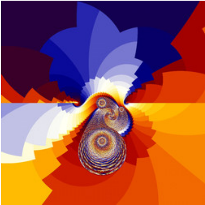
reb-JuliaTentMap-13D.jpg
