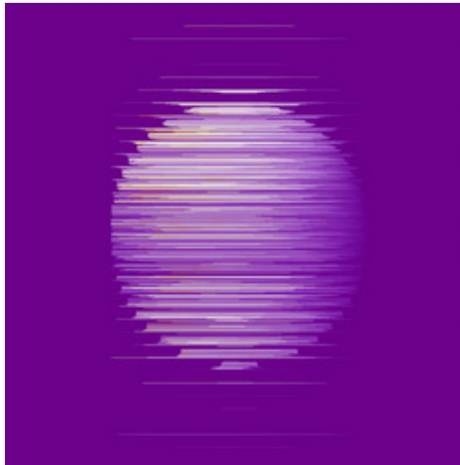
mt-GeneralizedCelticJulia-65.jpg
