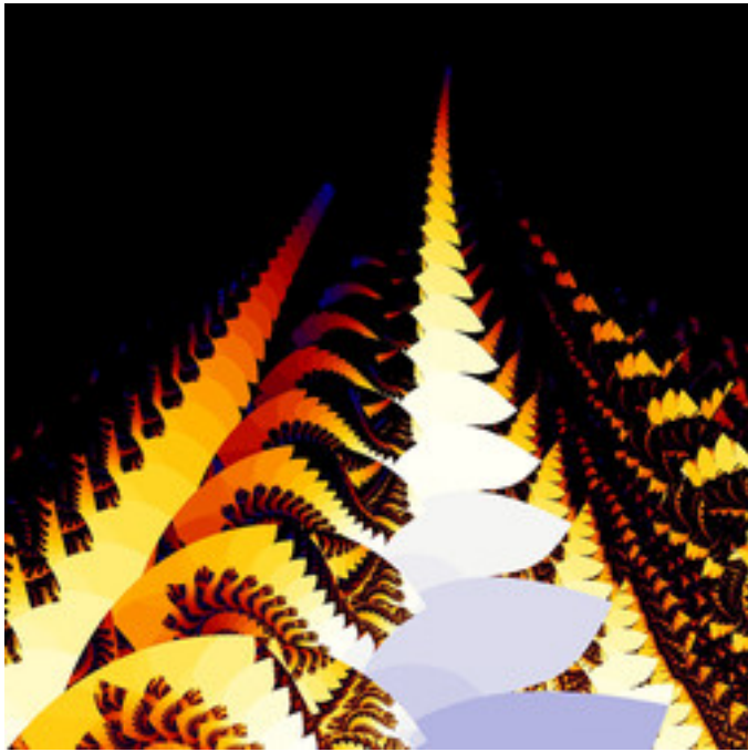
mt-barnsleyishMest-03.jpg
