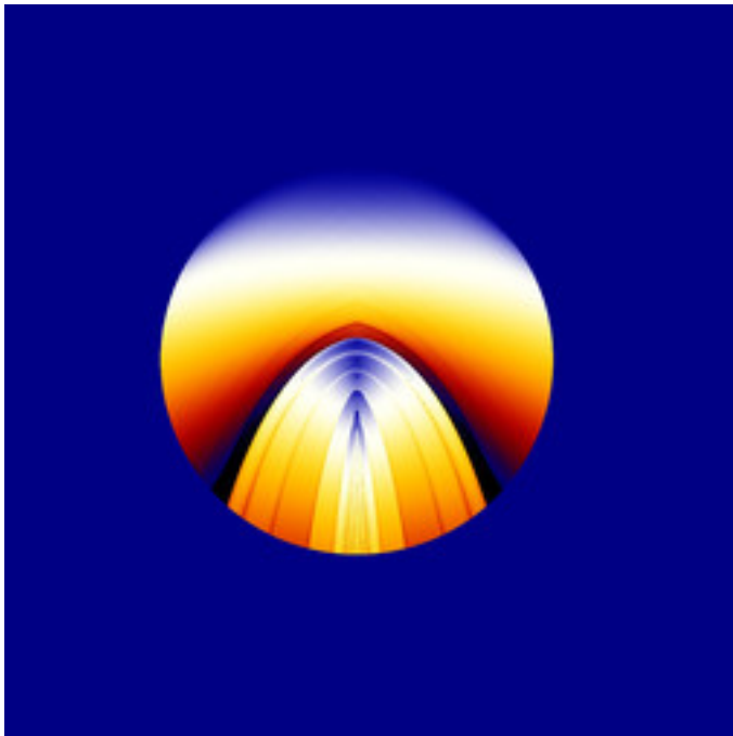
mt-zeepop-julia-10.jpg
