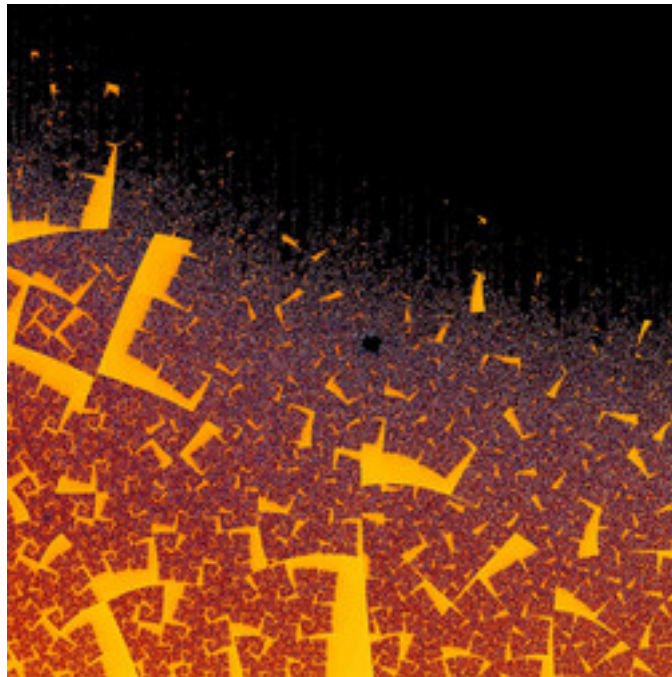
mt-rudys-cubic-mandelbrot-22.jpg
