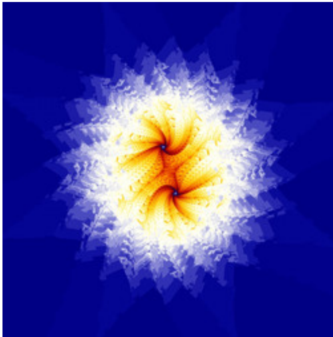
reb-JuliaTentMap-25.jpg
