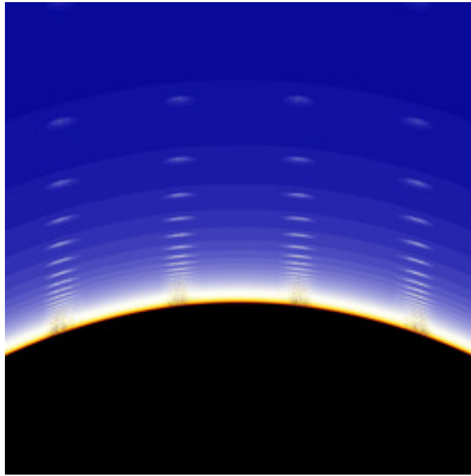
mt-ring-mset-02.jpg
