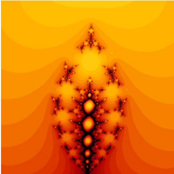
lkm3-AlternativeFunctions-10.jpg
