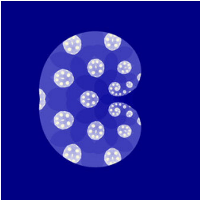
reb-ZeePi-02.jpg
