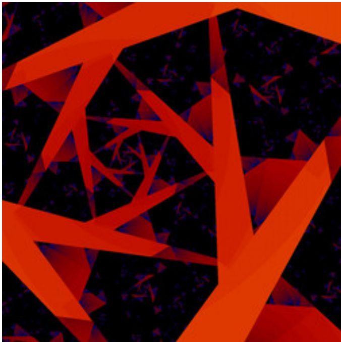
lkm-GeneralTentMandelbrot-09.jpg
