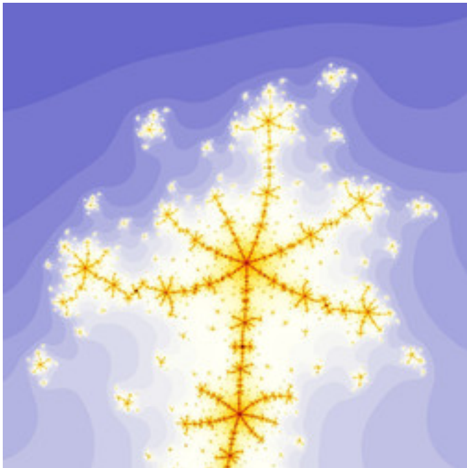
mt-990807aMset-10.jpg
