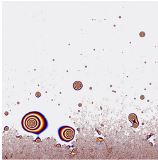
dmj-PhoenixDoubleNova-32.jpg
