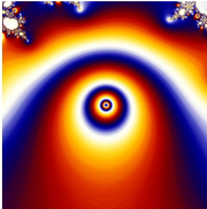
dmj-DoubleNova-02.jpg
