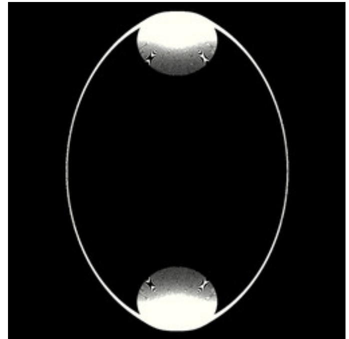
reb-FormulaTracer-09D.jpg
