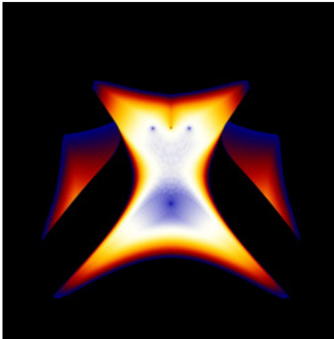
mt-zeepop-mset-44.jpg
