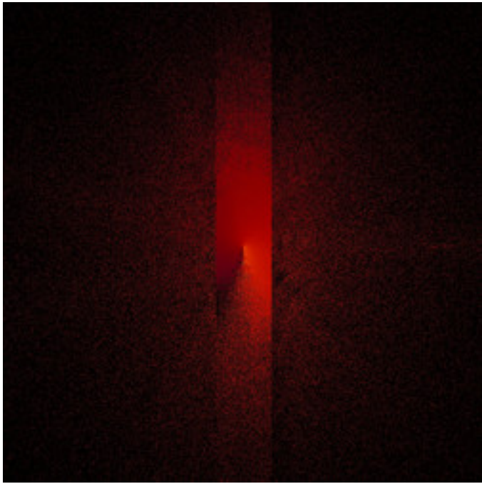
mt-newton-twist-11.jpg
