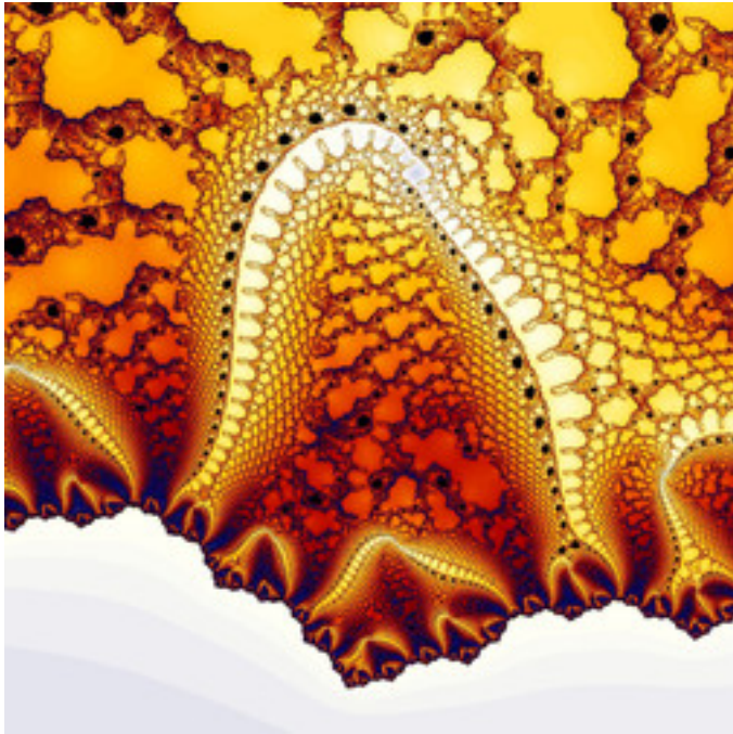
Ikm3-ExtraFoam-06.jpg
