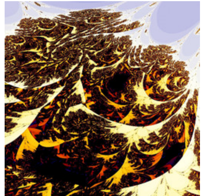
mt-bifunctionalMset-02.jpg
