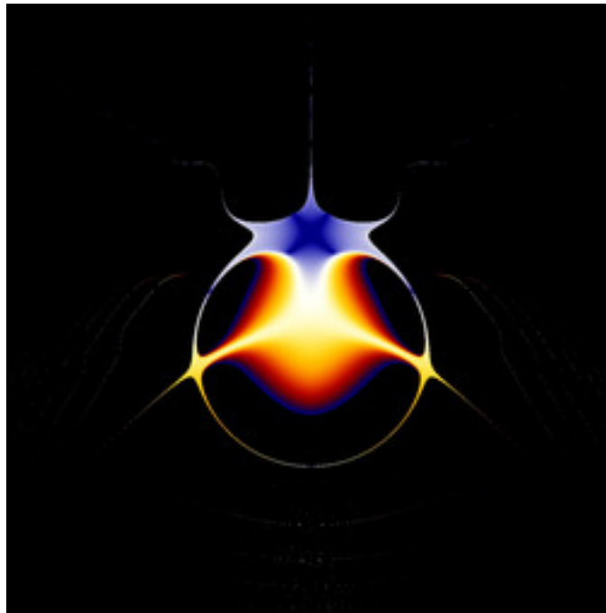
mt-zeepop-mset-15.jpg
