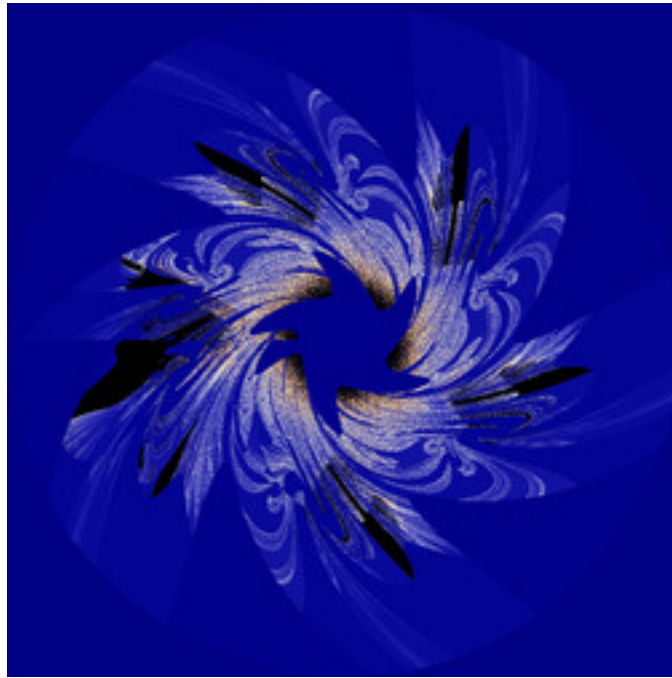
ahm-IndependantPower_04.jpg
