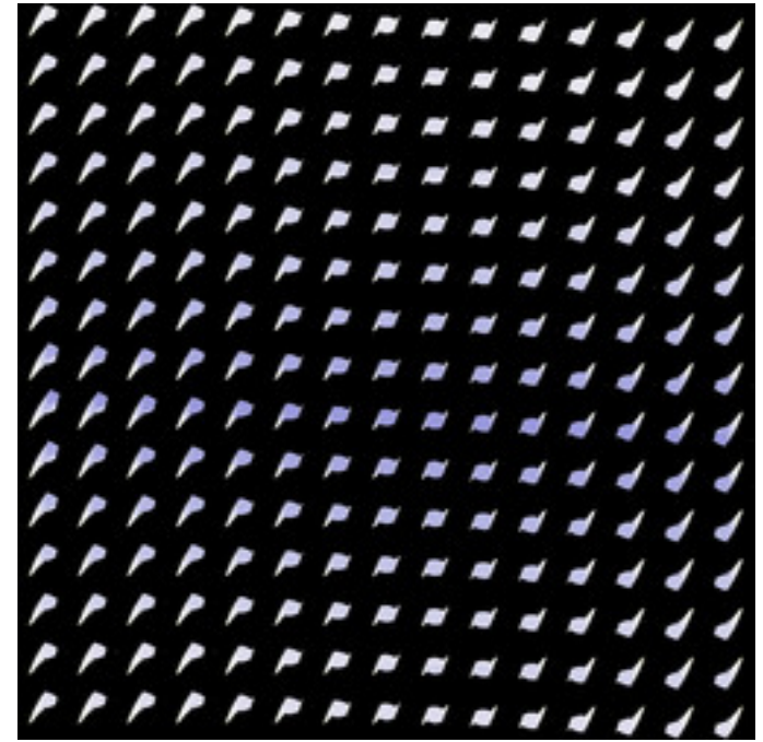
mt-zeepop-julia-29.jpg
