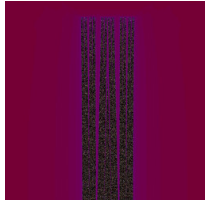
mt-GeneralizedCelticJulia-04.jpg
