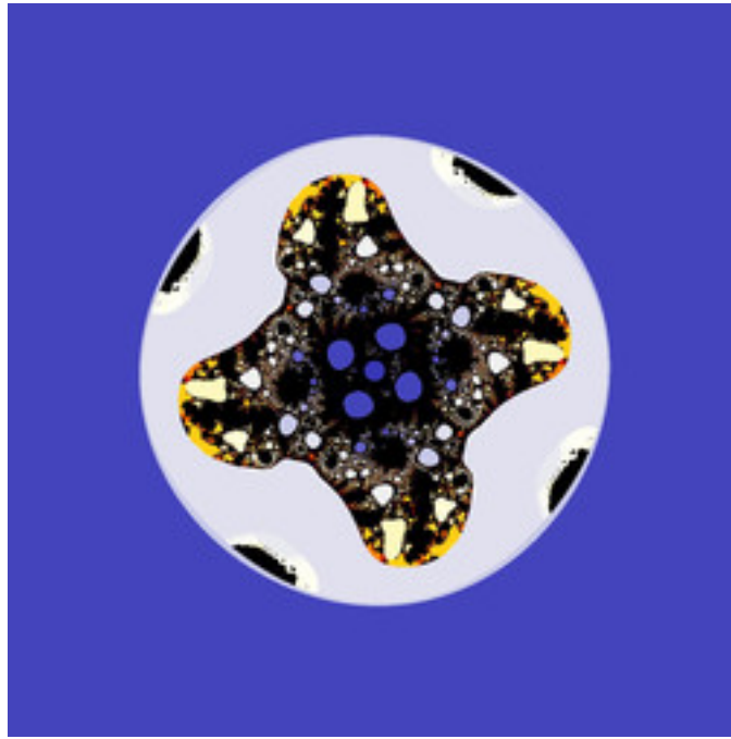
mt-rudys-cubic-mandelbrot-19.jpg
