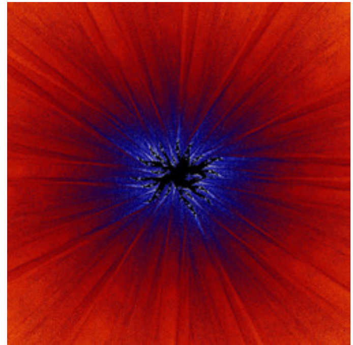
mt-rudys-cubic-julia-06.jpg
