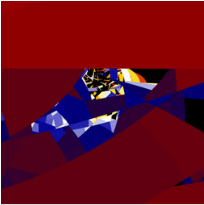
mt-990807bMset-19.jpg
