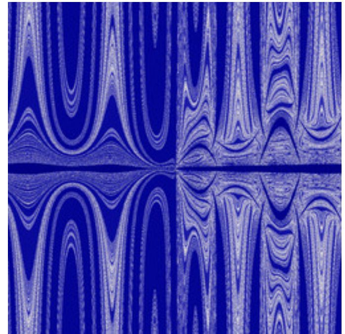
reb-GopalsamyFn-18.jpg
