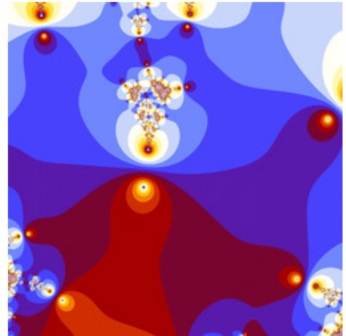
dmj-DoubleNova-13.jpg
