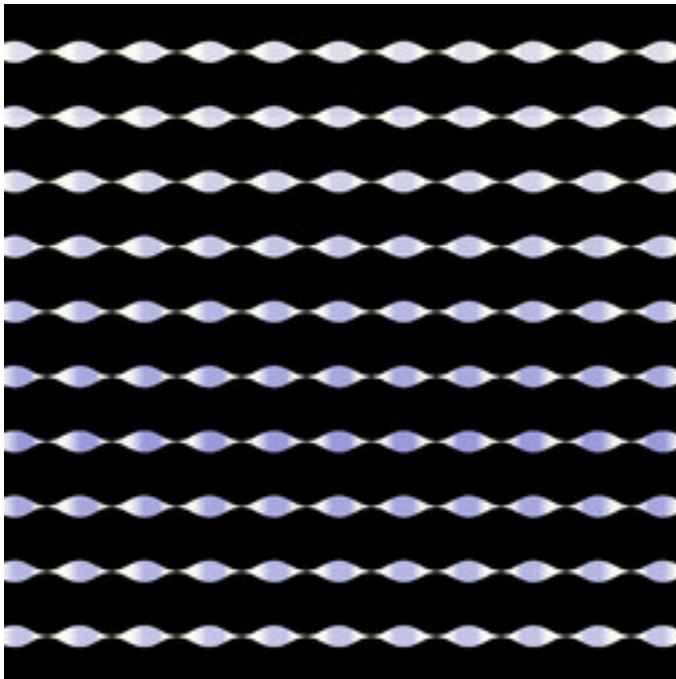
mt-zeepop-julia-28.jpg
