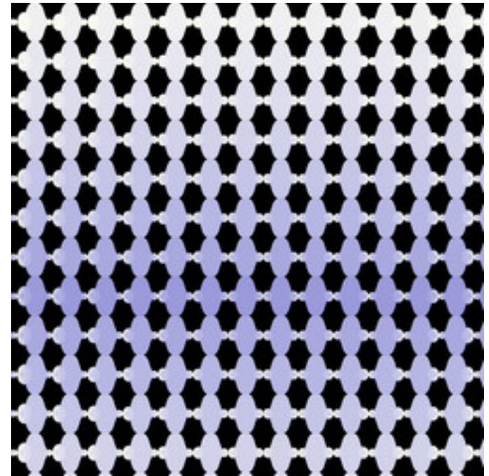
mt-zeepop-julia-26.jpg
