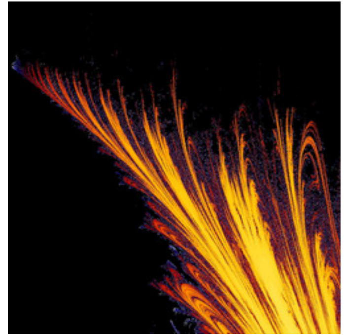
lkm3-RotatedMandelbrot-02.jpg
