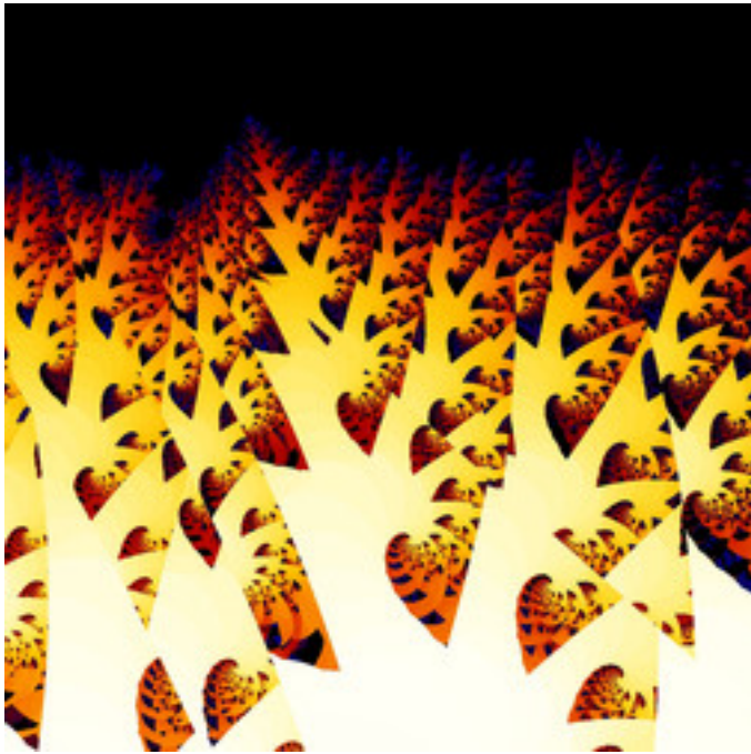
mt-barnsleyishMest-09.jpg
