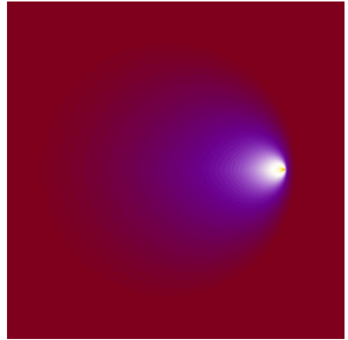
mt-GeneralizedCelticJulia-13.jpg
