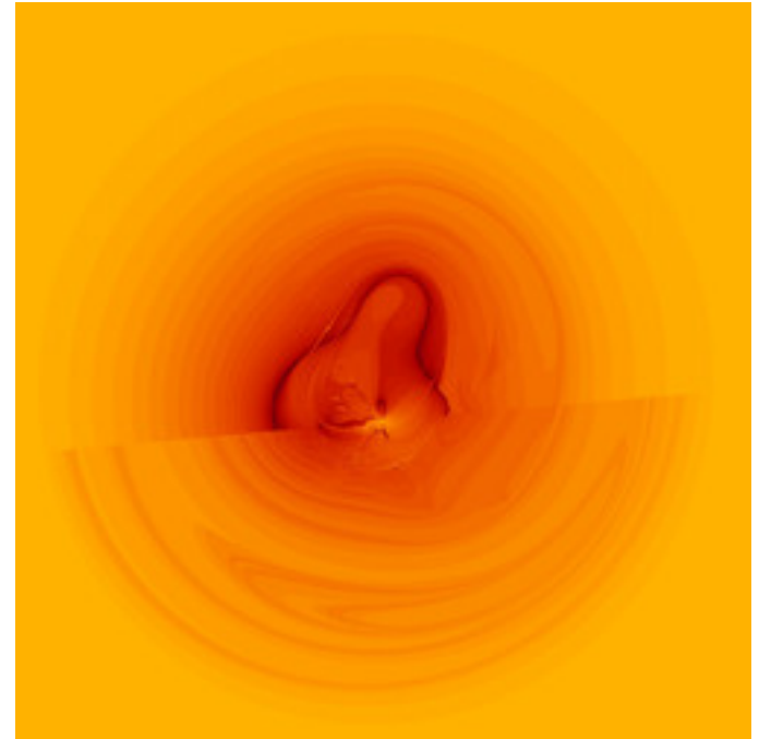
asz-andrexrandom-1-25.jpg
