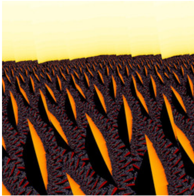
mt-rudys-cubic-mandelbrot-25.jpg
