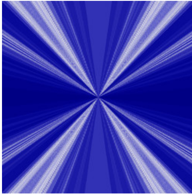
reb-GopalsamyFn-28.jpg
