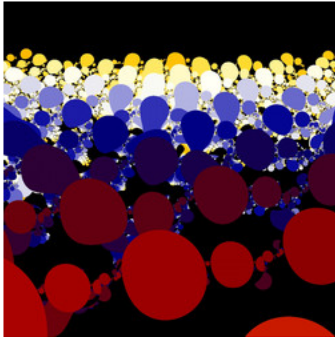
mt-barnsleyishMest-20.jpg
