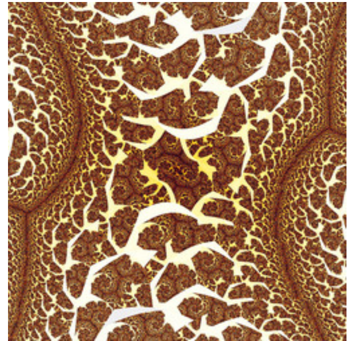
mt-barnsleyishJulia-13.jpg
