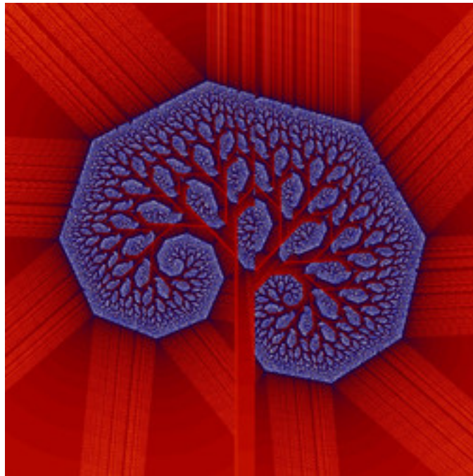
reb-IFSEscape1-06B.jpg
