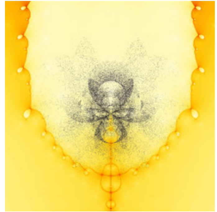
mt-newton-error-04a.jpg
