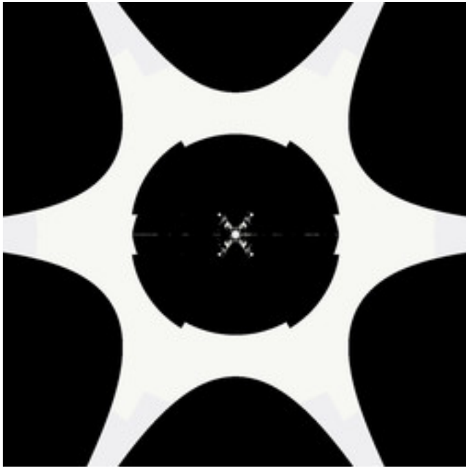
mt-rudys-cubic-mandelbrot-32.jpg
