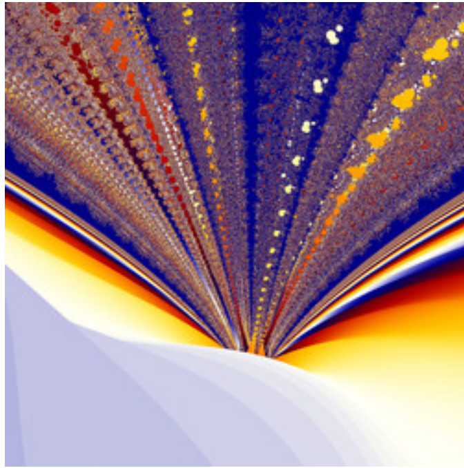
dmj-PhoenixDoubleNova-05.jpg
