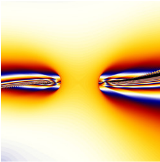
mt-BofNewton1-02.jpg
