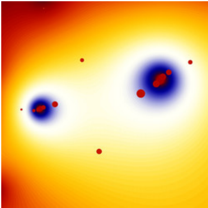
dmj-PhoenixDoubleNova-21.jpg
