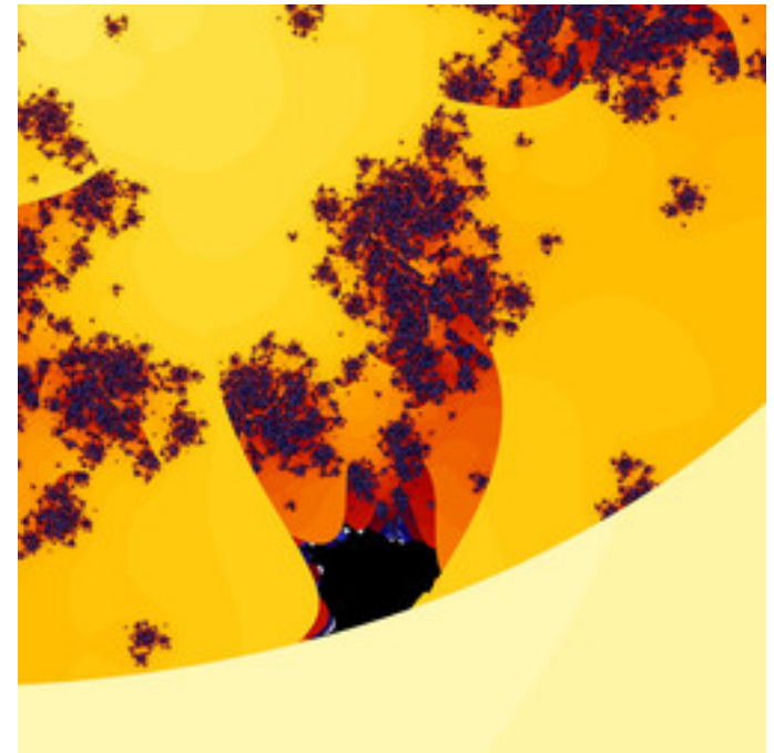
mt-990807aMset-18.jpg
