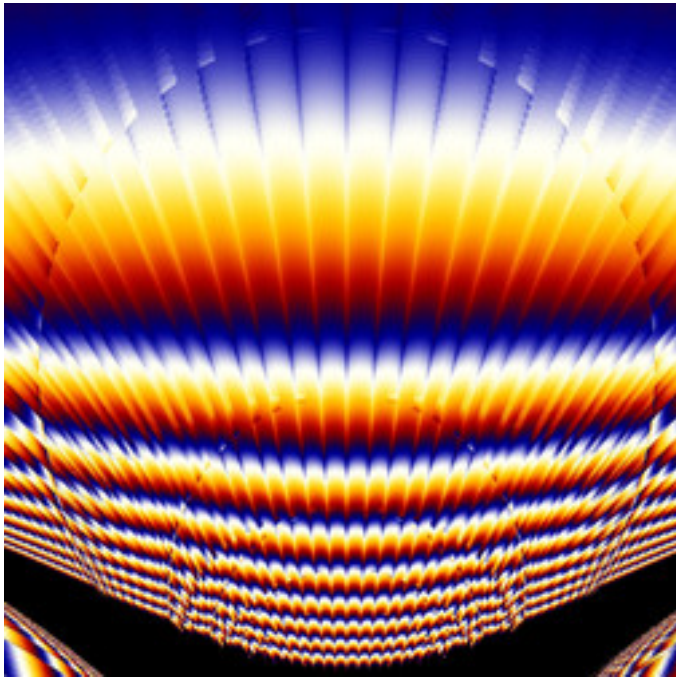
mt-newton-9904a-07.jpg
