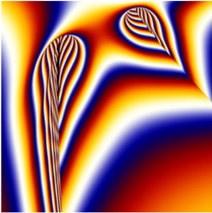
mt-newton-9904a-01.jpg
