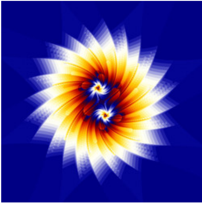
reb-JuliaTentMap-23.jpg
