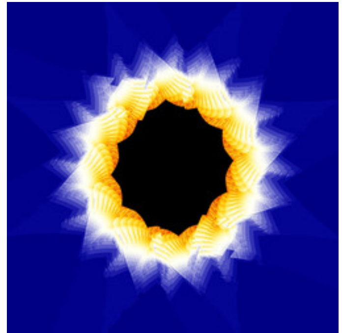
reb-JuliaTentMap-30.jpg
