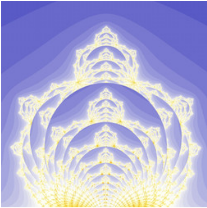
dmj-OrbitBoost-06.jpg
