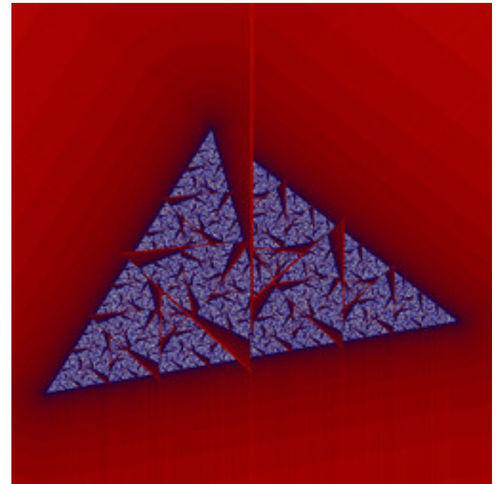
reb-IFSEscape1-10.jpg
