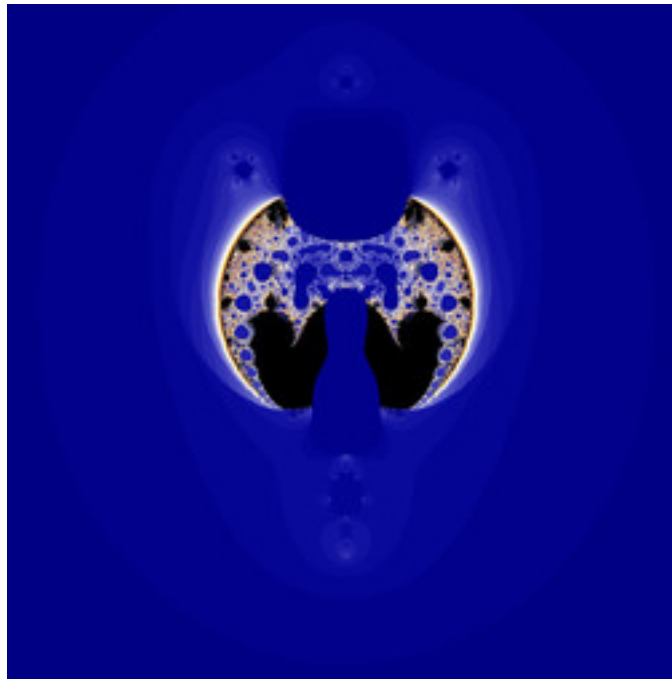
reb-Ikenagafn-01.jpg
