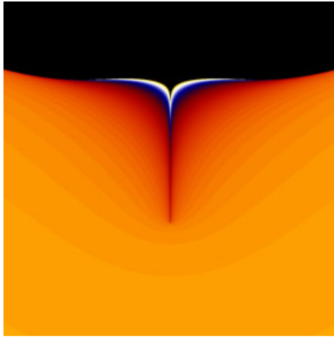
mt-990807bMset-06.jpg
