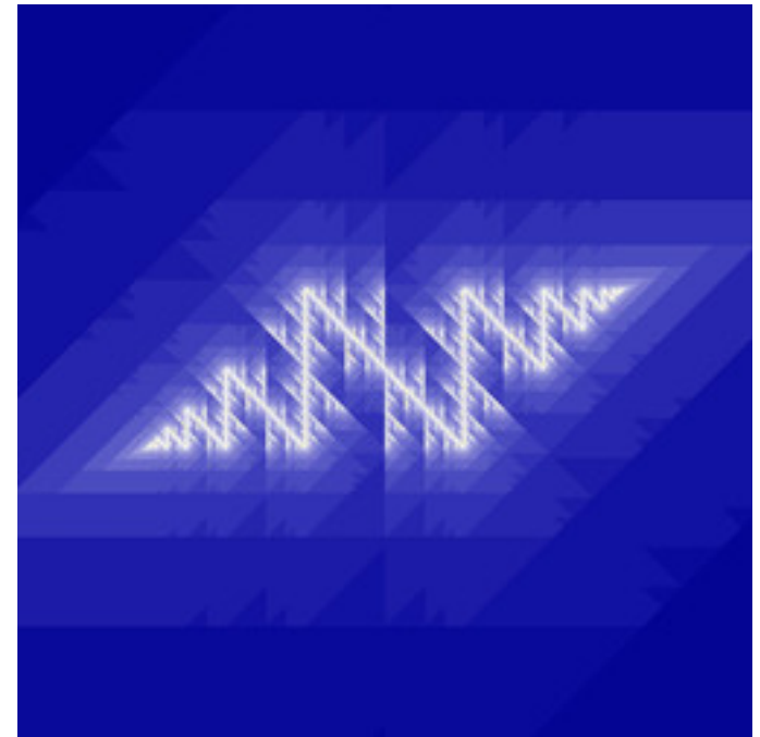
reb-FunBarnsley1Julia-01A.jpg
