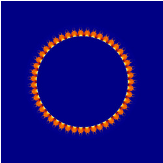
mt-pseudo-magnet-julia-01.jpg
