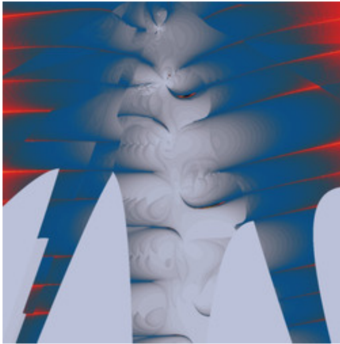
asz-andrextrandom-1-05.jpg
