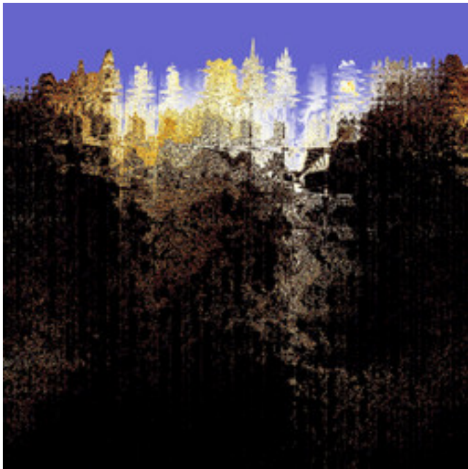
lkm3-FourierPopCorn-06A.jpg
