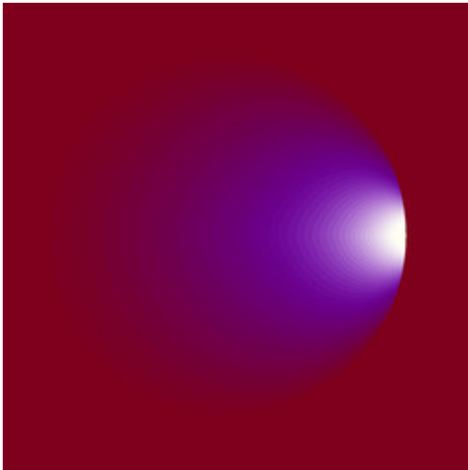
mt-GeneralizedCelticJulia-12.jpg
