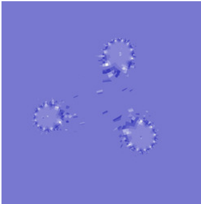
mt-rudys-cubic-julia-01.jpg
