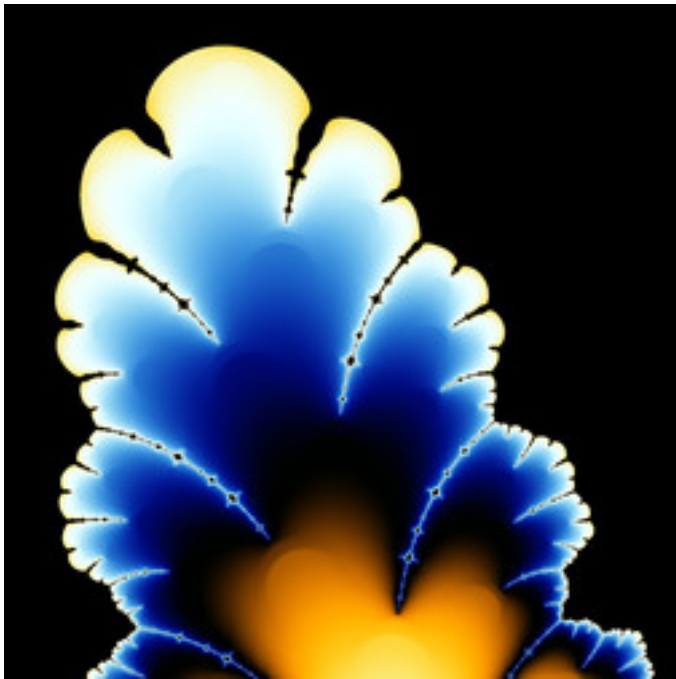
standard-FastMandel-07.jpg
