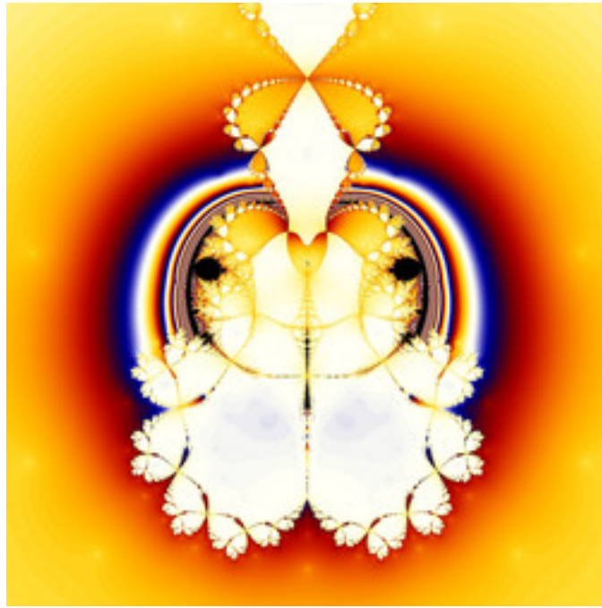
mt-newton-error-12.jpg
