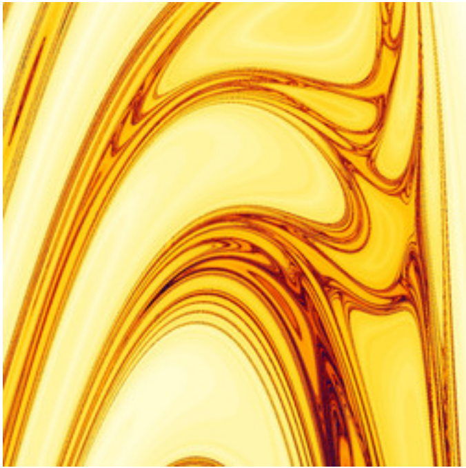
mt-990625bMset-03.jpg
