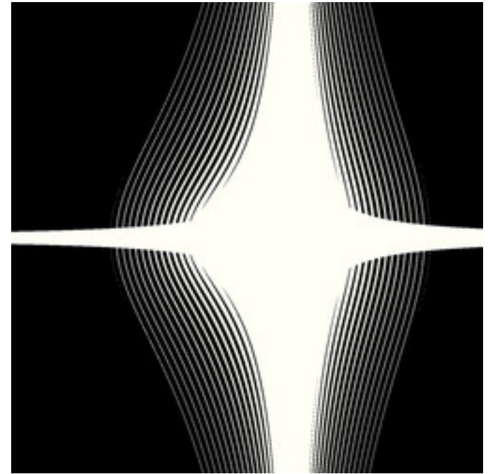
reb-FormulaTracer-15B.jpg
