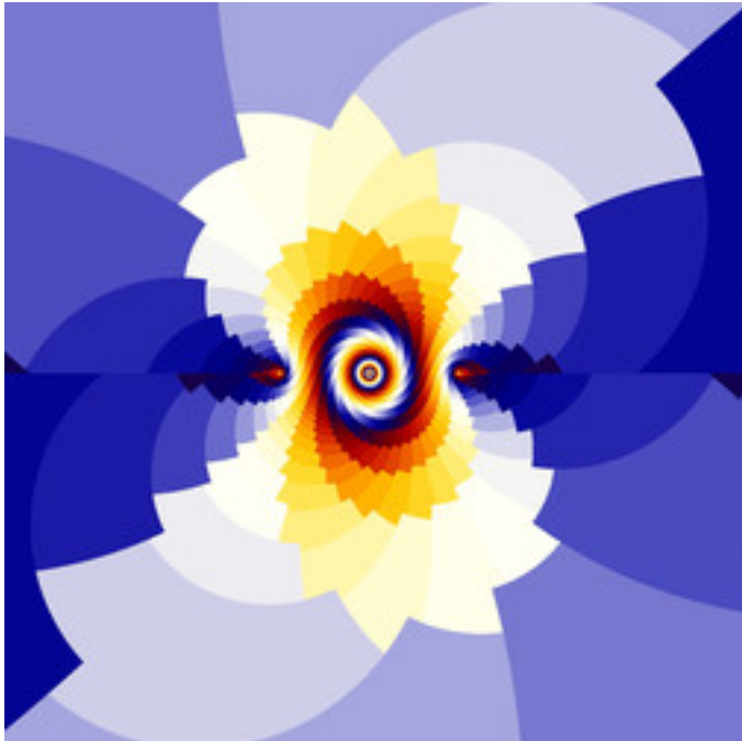
reb-JuliaTentMap-19.jpg
