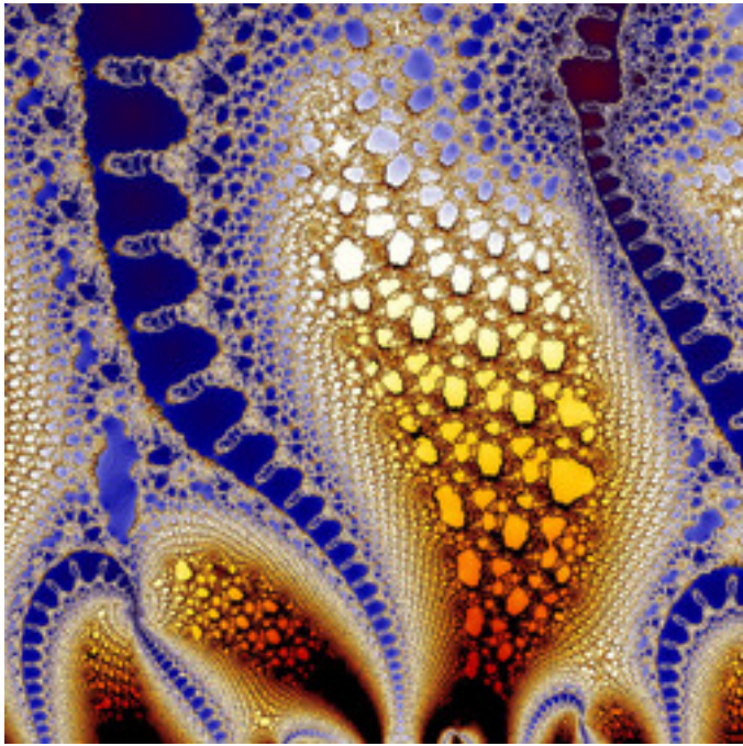
lkm3-ExtraFoam-03.jpg
