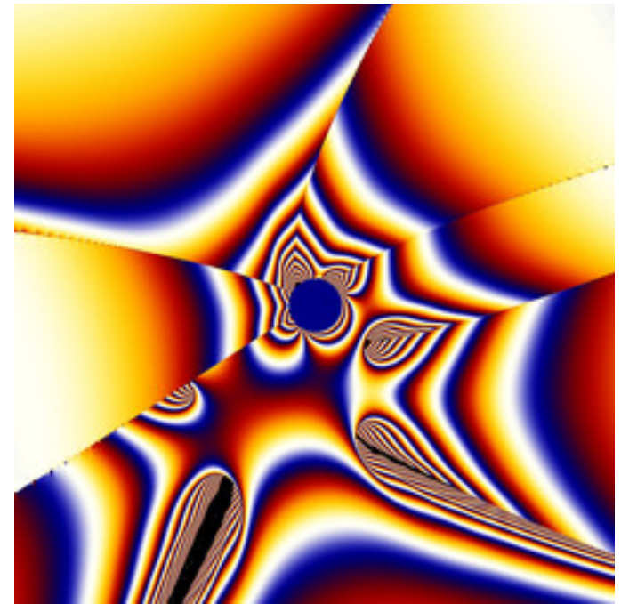
mt-newton-9904a-02.jpg
