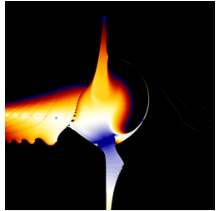
mt-zeepop-mset-23.jpg
