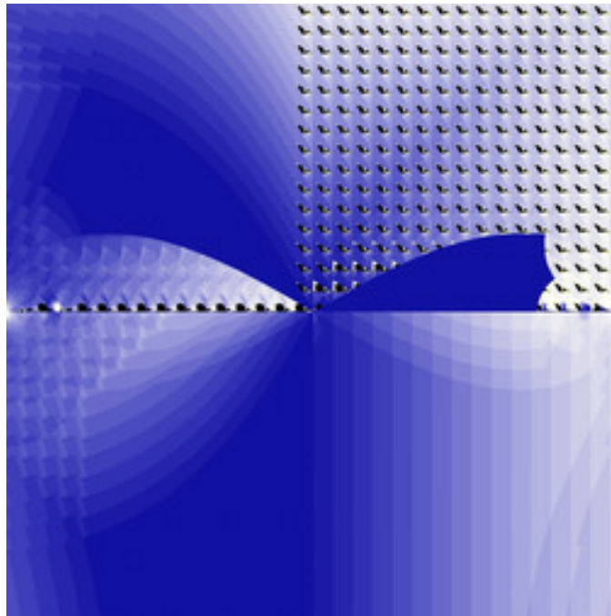
mt-zeepop-julia-21.jpg
