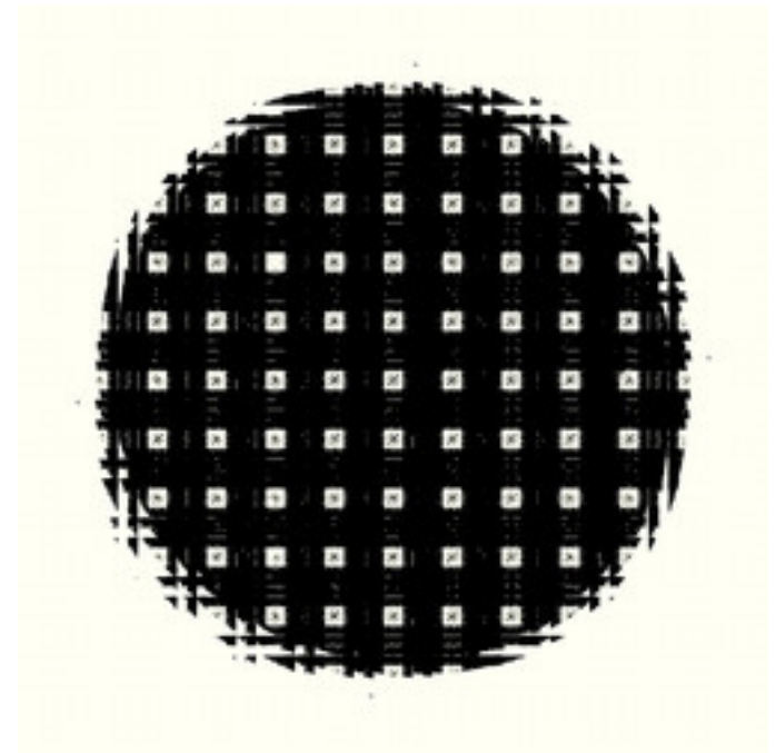
lkm3-FourierPopCorn-09.jpg
