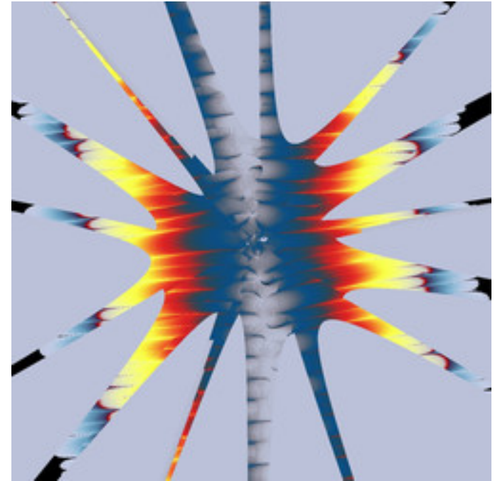
asz-andrextandom-1-07.jpg
