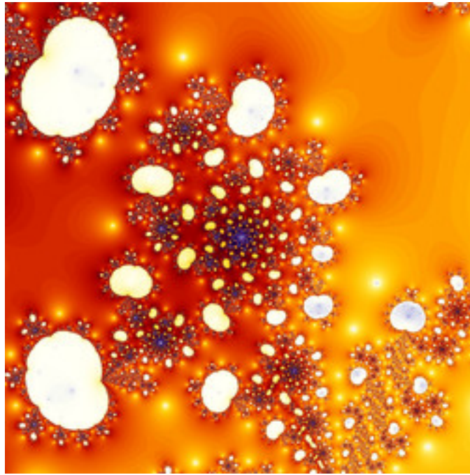
dmj-DoubleNova-05.jpg
