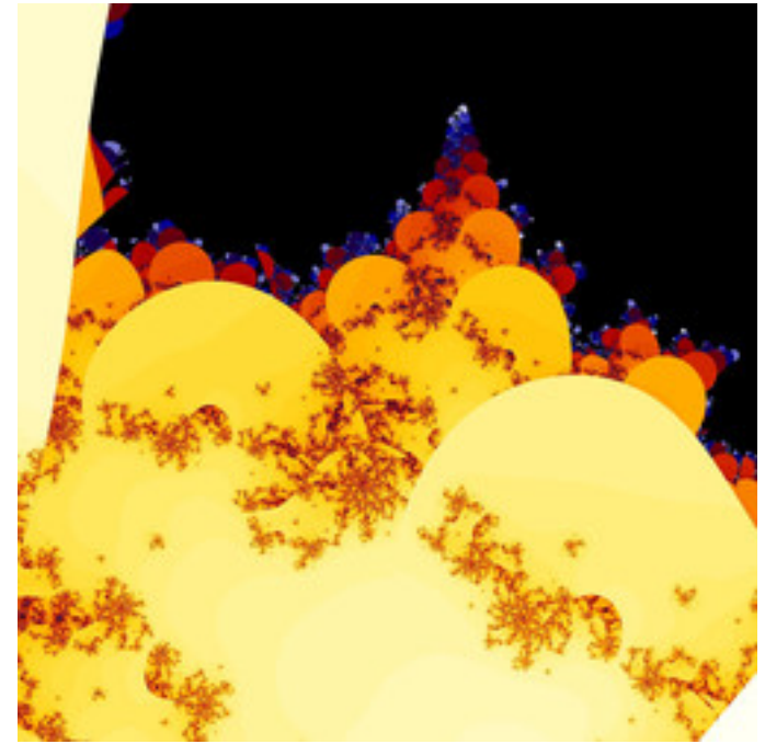
mt-990807aMset-21.jpg
