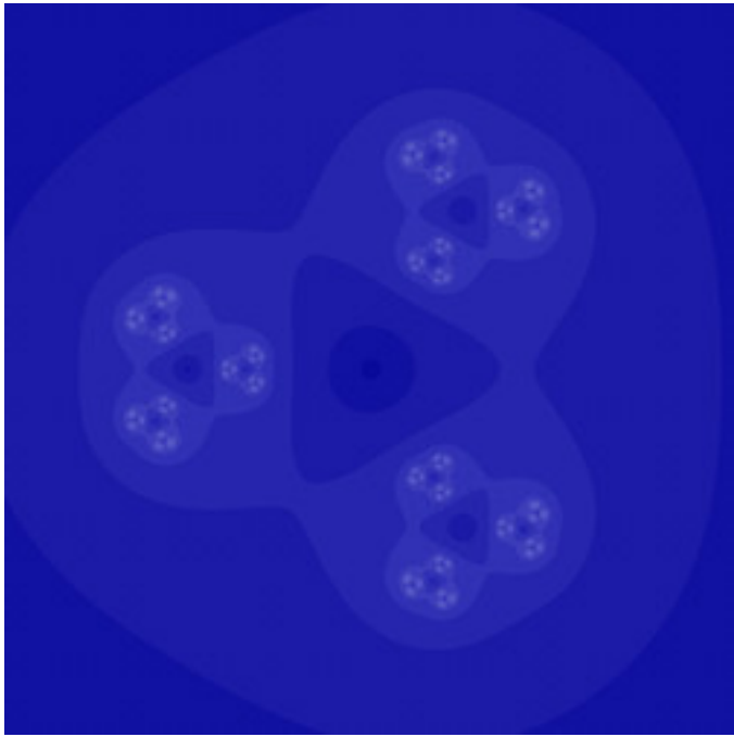
dmj-DoubleJulia-01.jpg
