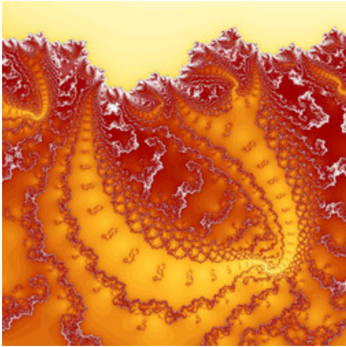
Ikm3-ExtraFoam-09.jpg
