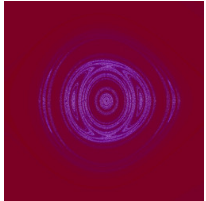
mt-GeneralizedCelticJulia-10.jpg
