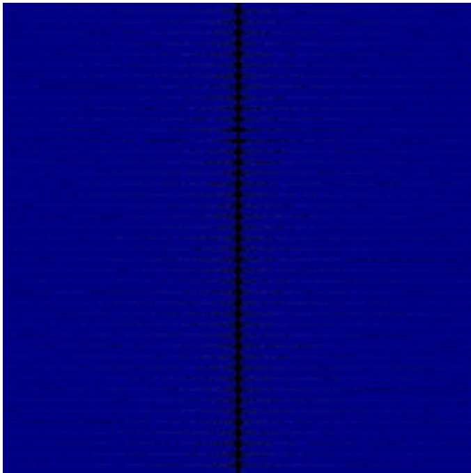
reb-GopalsamyFn-04.jpg
