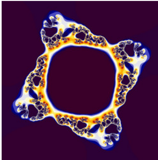
mt-rudys-cubic-mandelbrot-16.jpg
