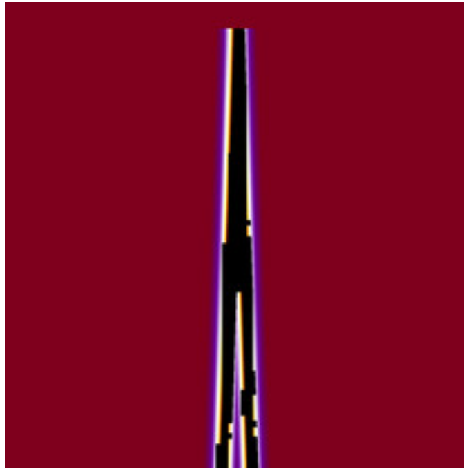
mt-GeneralizedCelticJulia-14.jpg
