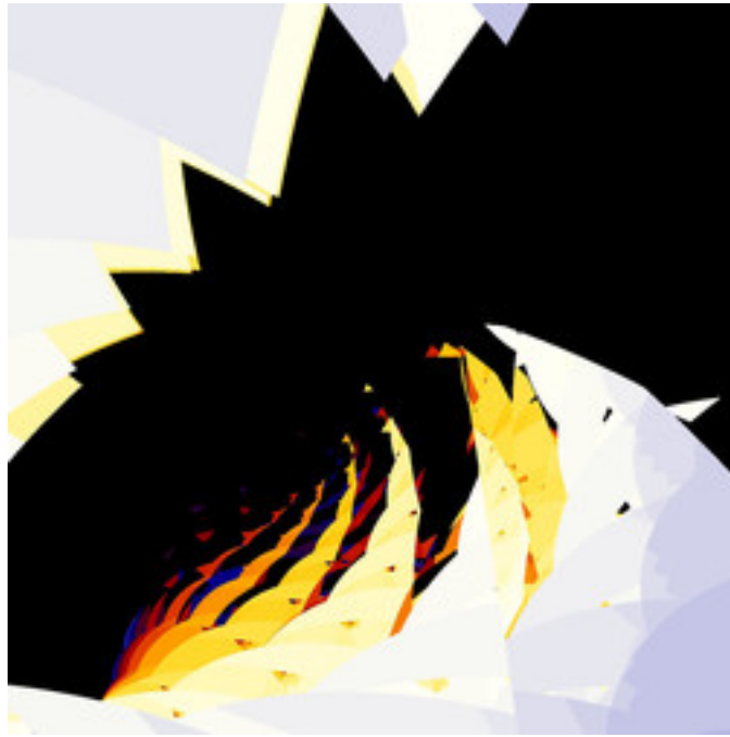
mt-990807bMset-18.jpg
