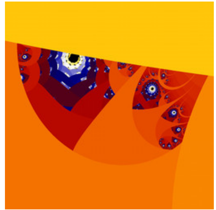
lkm-GapMandelbrot-08.jpg
