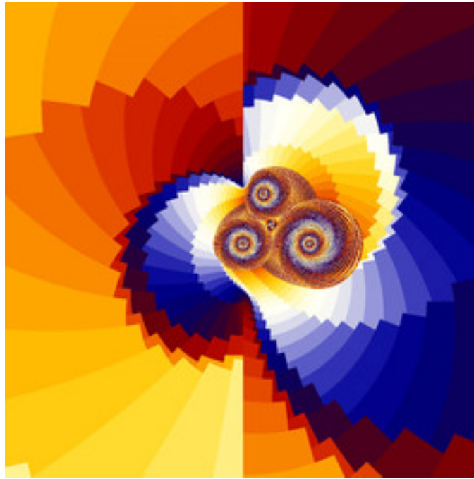
reb-JuliaTentMap-12.jpg
