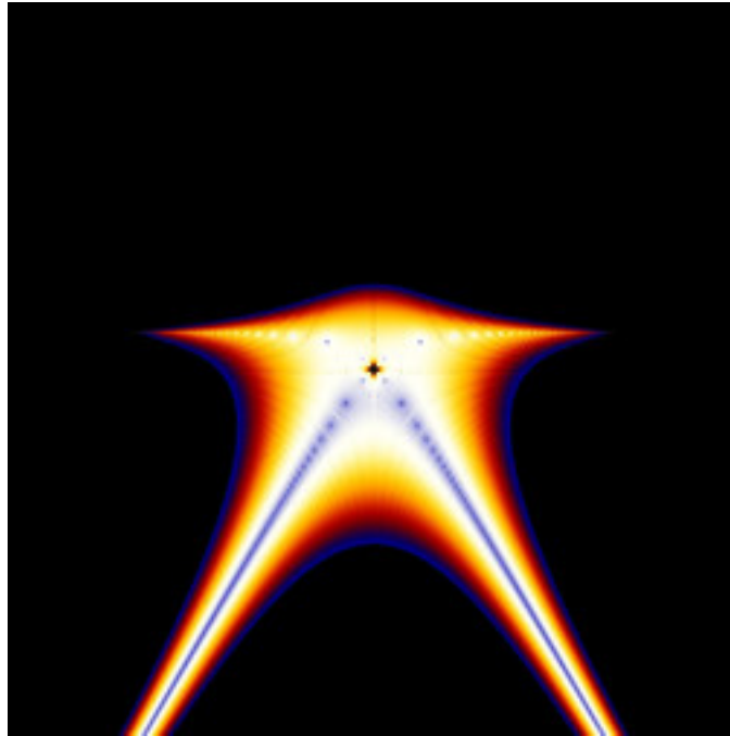
mt-zeepop-mset-50.jpg
