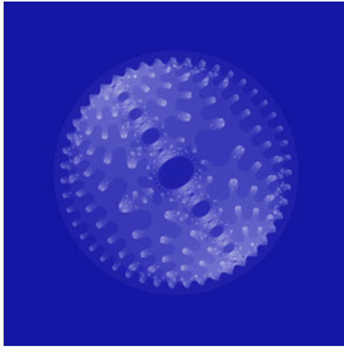
mt-pseudo-magnet-julia-03.jpg
