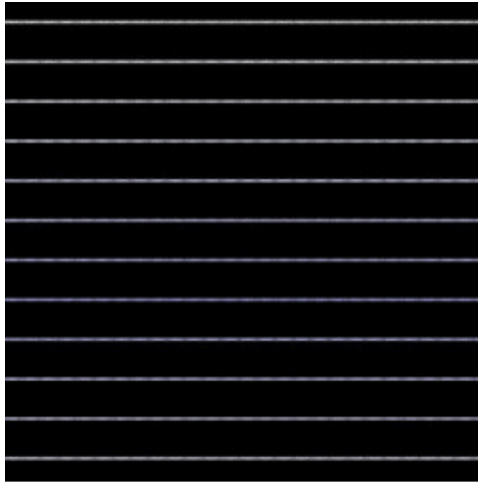
mt-zeepop-julia-24.jpg
