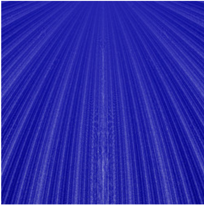
lkm3-UnitVectorTweakMandelbrot-01.jpg
