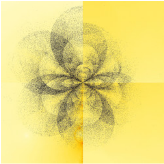
mt-newton-error-22a.jpg
