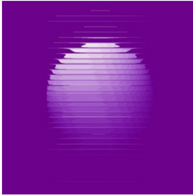
mt-GeneralizedCelticJulia-62.jpg
