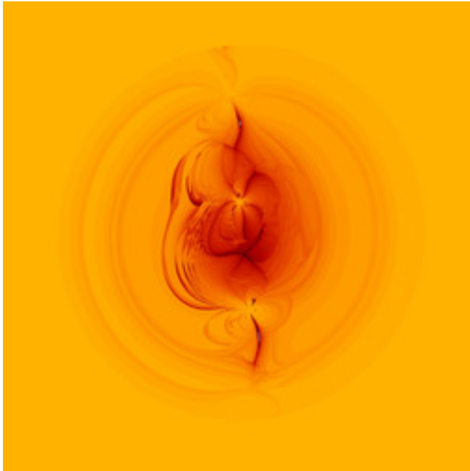
asz-andrexrandom-1-27.jpg
