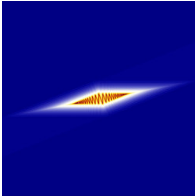
reb-FunBarnsley1Julia-03.jpg
