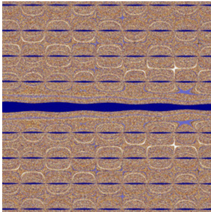
reb-GopalsamyFn-19.jpg
