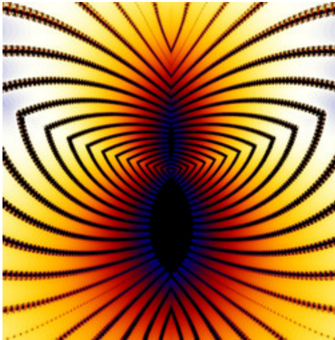
lkm-EmbossedNewton-01.jpg
