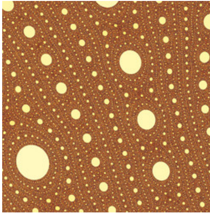
lkm-MitchsMandelbrot-08.jpg
