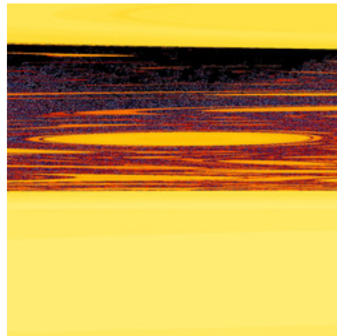
mt-990625bMset-10.jpg
