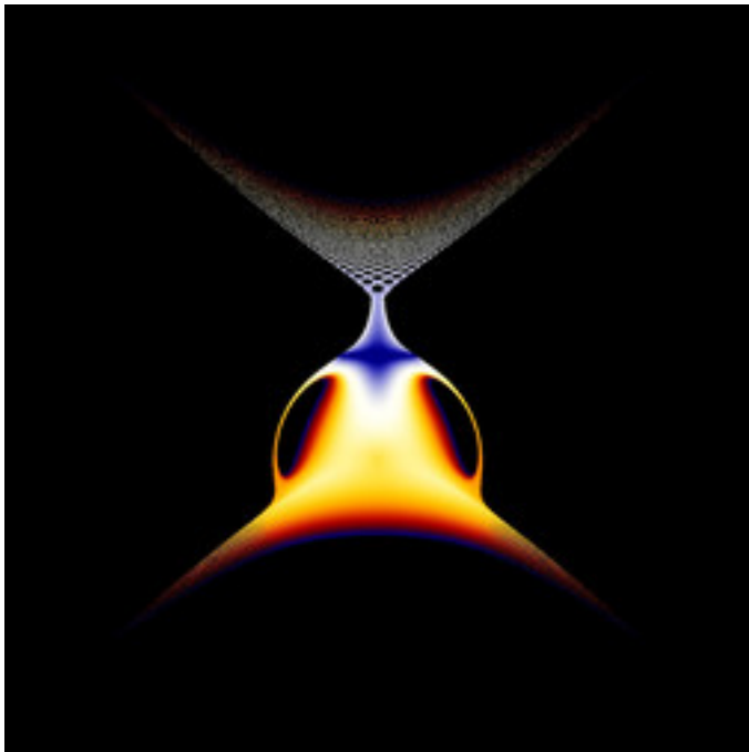
mt-zeepop-mset-34.jpg
