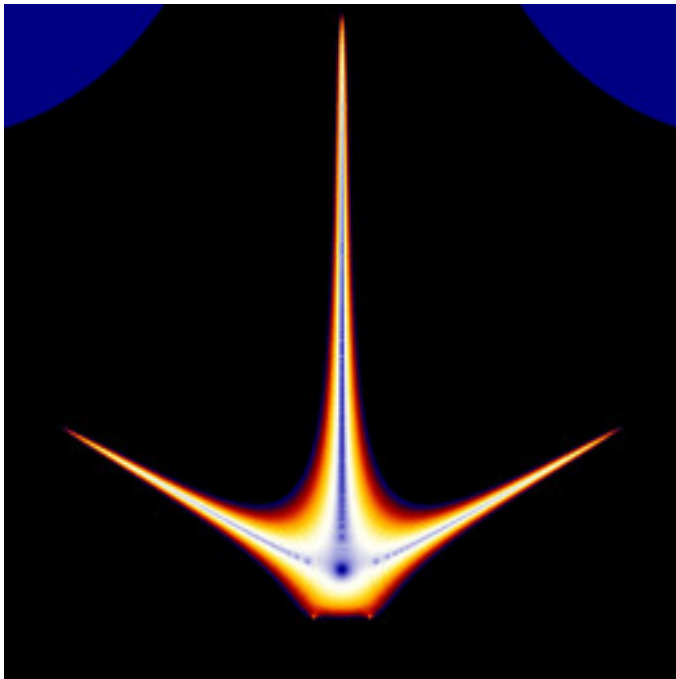
mt-zeepop-mset-16.jpg
