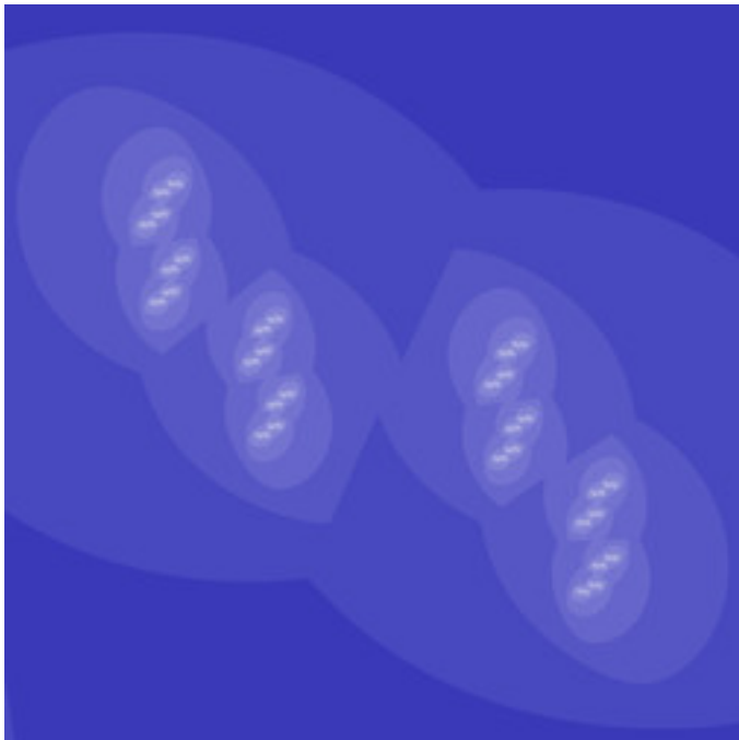
mt-barnsleyishJulia-03.jpg
