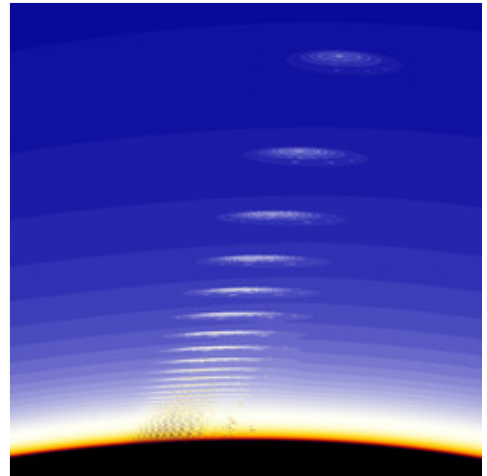
mt-ring-mset-04.jpg
