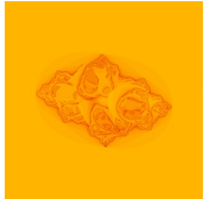
reb-JuliaCrossOrbitLambda-01.jpg
