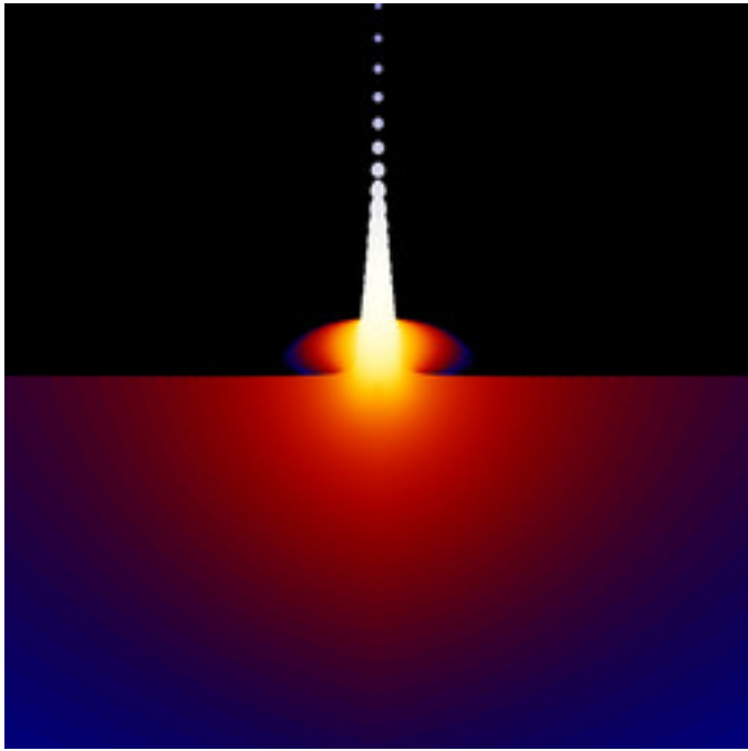
mt-zeepop-mset-25.jpg
