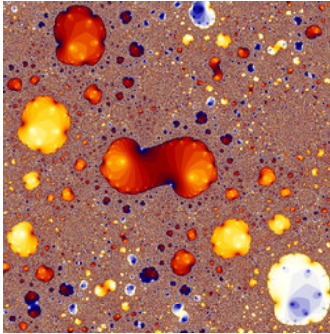
dmj-DoubleNova-11.jpg
