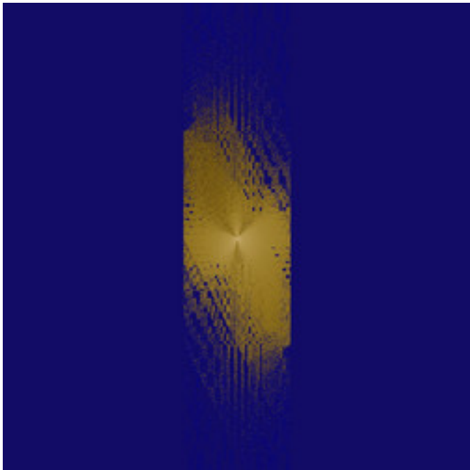
mt-newton-error-julia-02.jpg
