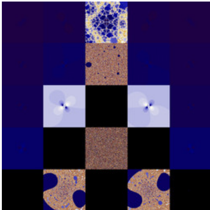
dmj-ManyNova-09.jpg
