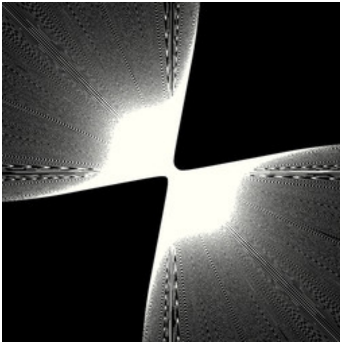
reb-FormulaTracer-05D.jpg
