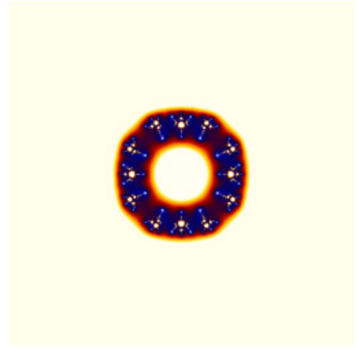
mt-rudys-cubic-mandelbrot-06.jpg
