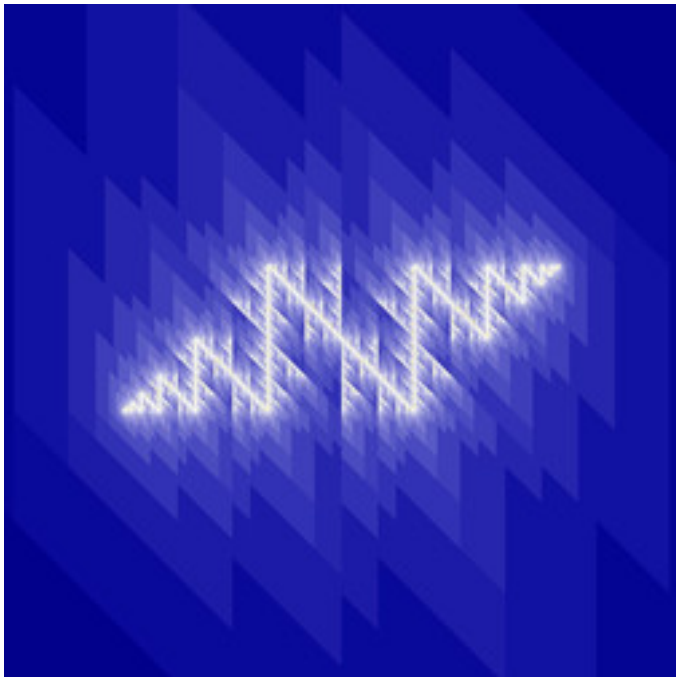
reb-FunBarnsley1Julia-01C.jpg
