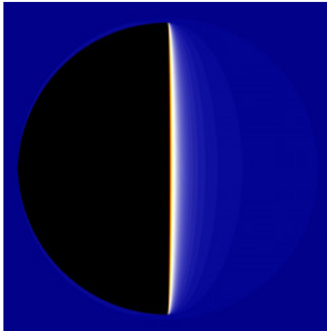
mt-bifunctionalMset-09.jpg
