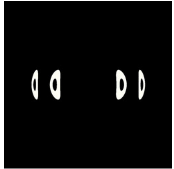
reb-FormulaTracer-13C.jpg
