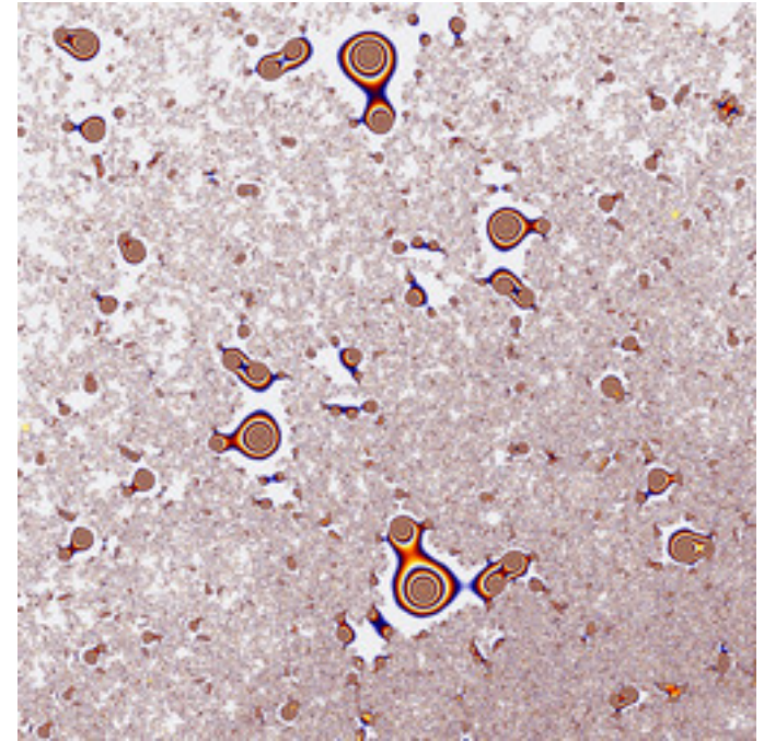
dmj-PhoenixDoubleNova-34.jpg
