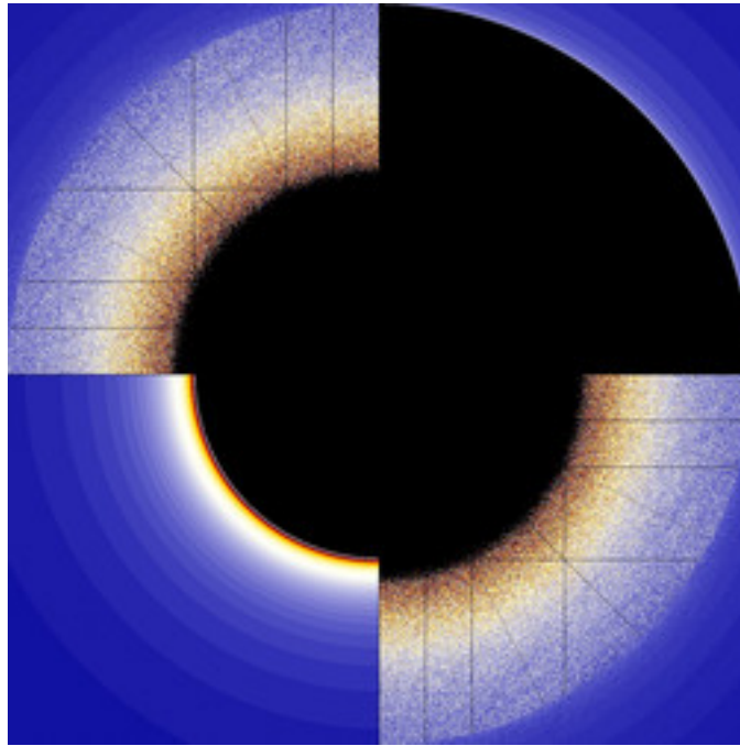
reb-SlopeExpFun_BarnsleyM2-03.jpg
