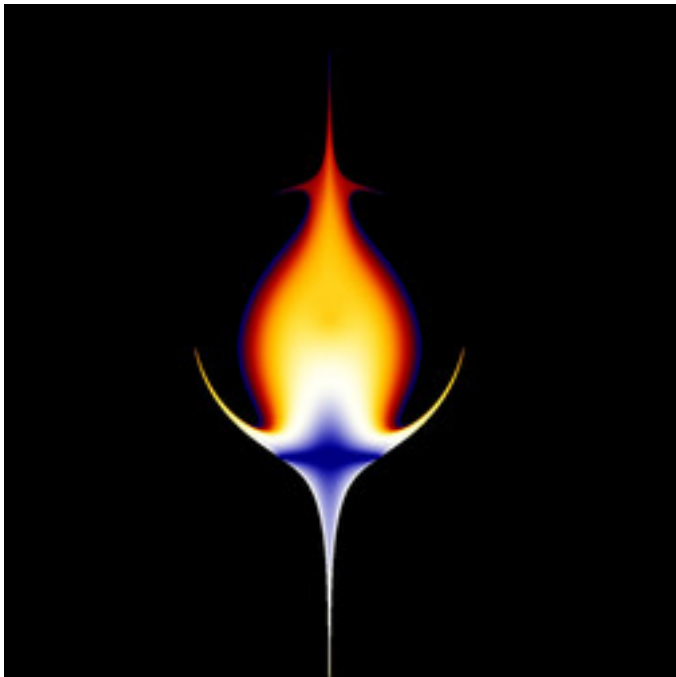
mt-zeepop-mset-22.jpg
