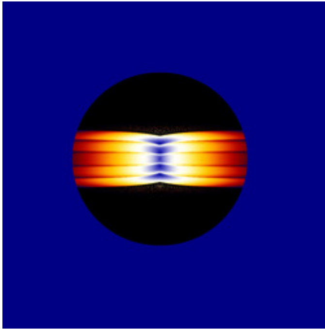
mt-zeepop-julia-06.jpg
