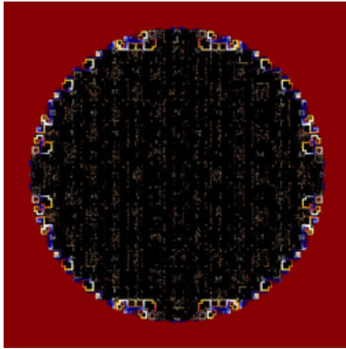
lkm3-FourierPopCorn-04B.jpg
