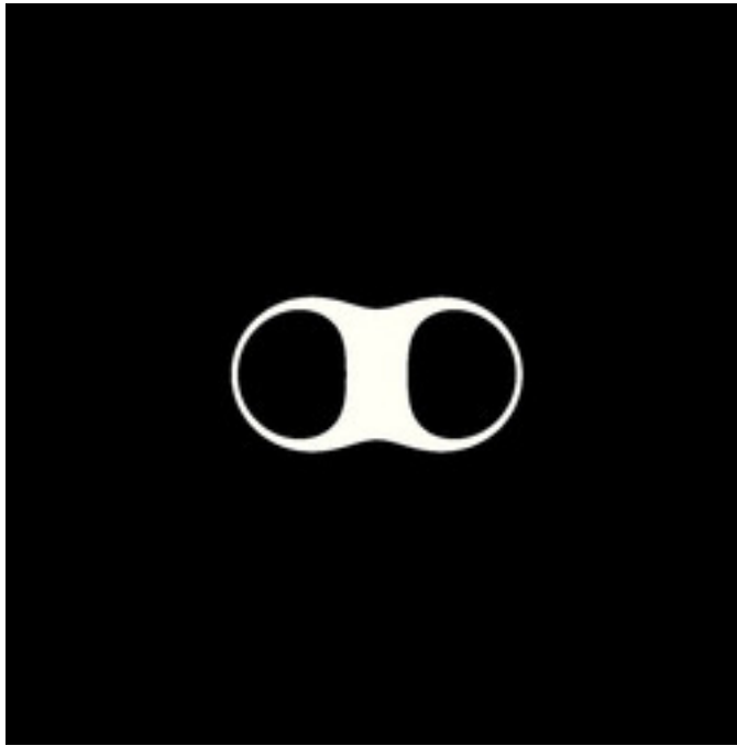
reb-FormulaTracer-16A.jpg
