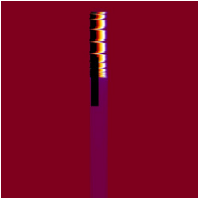
mt-GeneralizedCelticJulia-30.jpg
