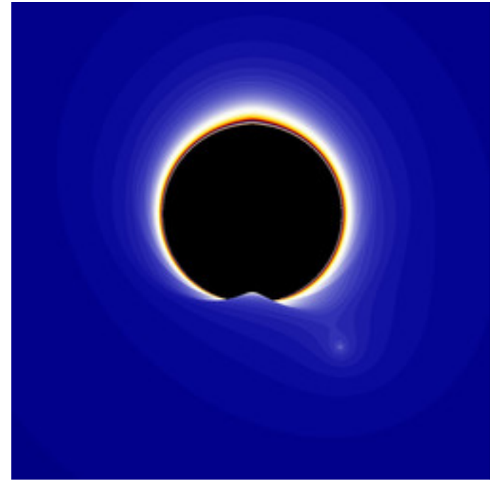
reb-Ikenagafn-03.jpg
