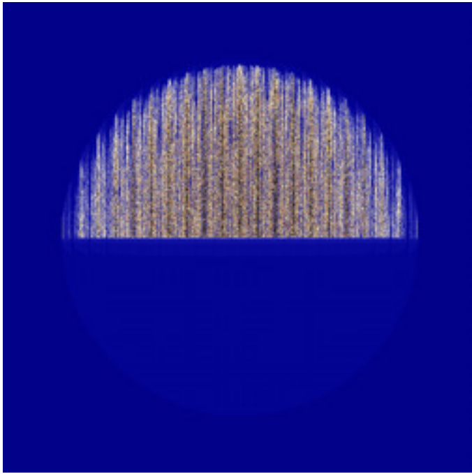
mt-bifunctionalMset-13.jpg
