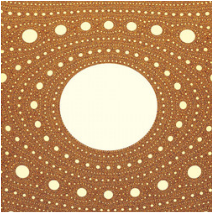
lkm-MitchsMandelbrot-09.jpg
