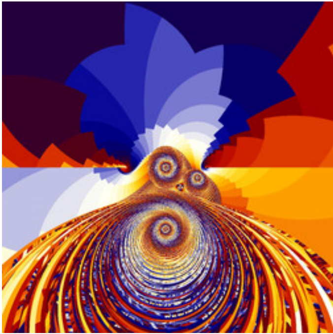
reb-JuliaTentMap-13.jpg
