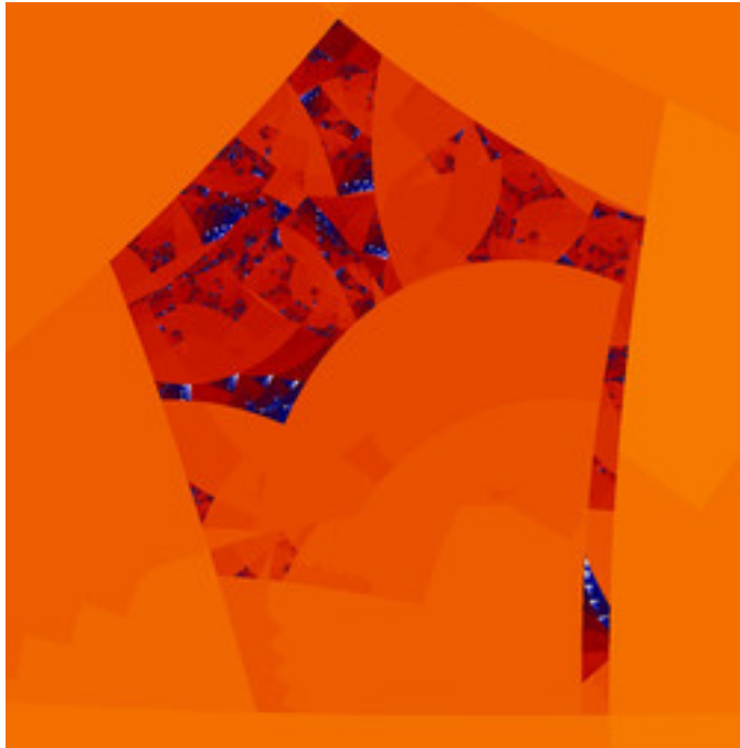
mt-990807bMset-09.jpg
