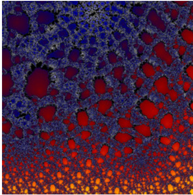
lkm3-ExtraFoam-02.jpg
