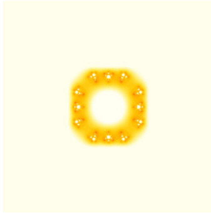
mt-rudys-cubic-mandelbrot-07.jpg
