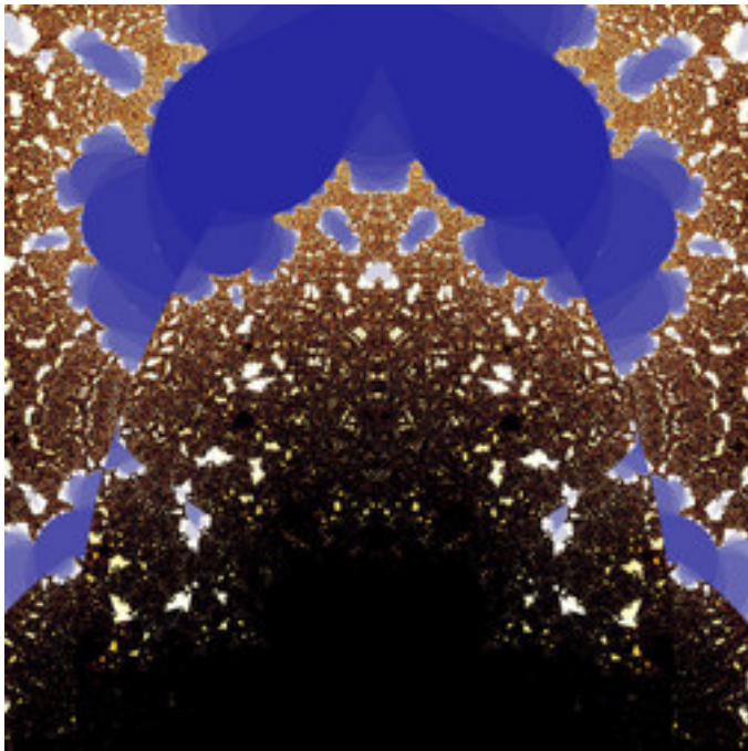
mt-990807aMset-14b.jpg
