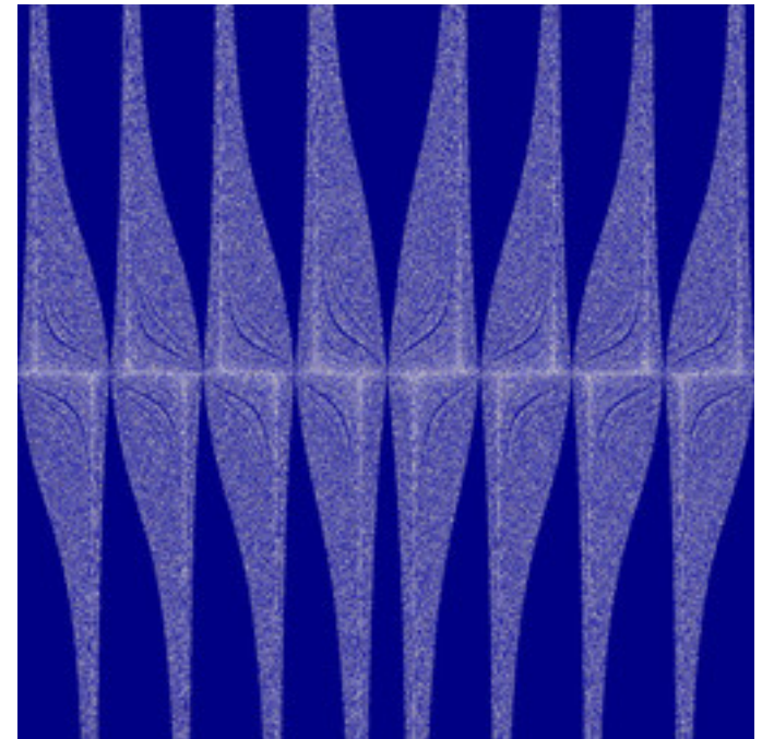
reb-GopalsamyFn-12.jpg
