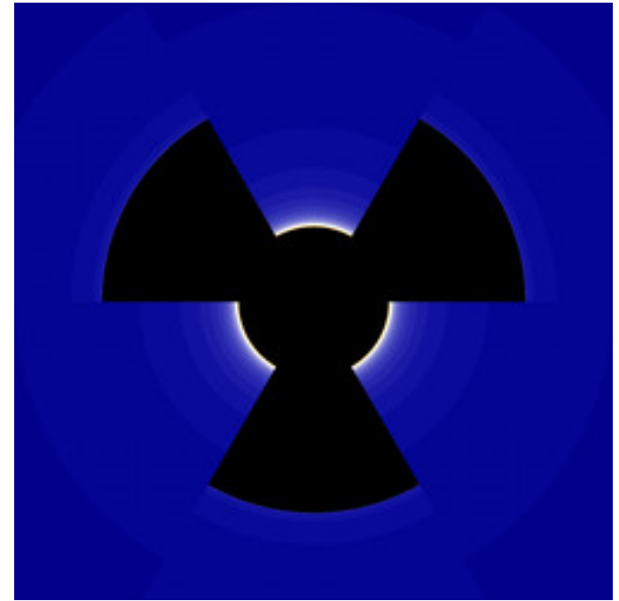
reb-SlopeExpFun_BarnsleyM2-02.jpg
