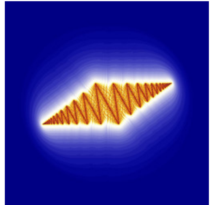
reb-FunBarnsley1Julia-05A.jpg
