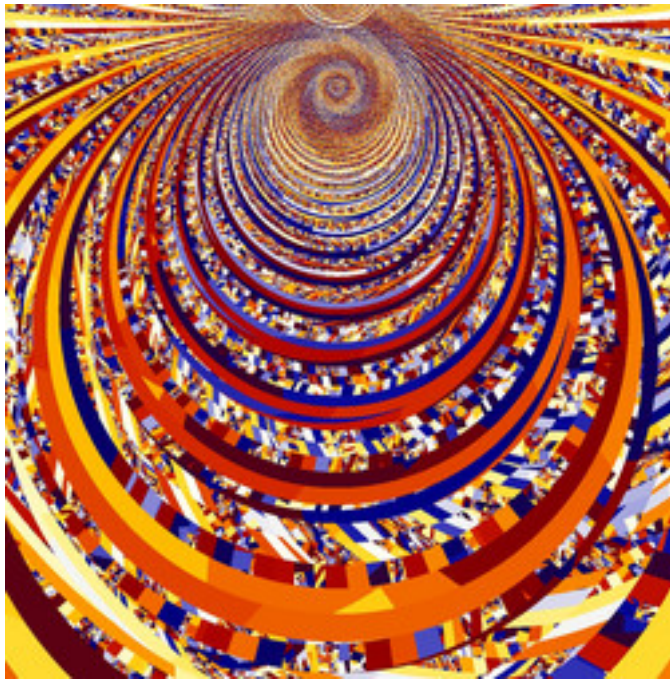
reb-JuliaTentMap-21.jpg
