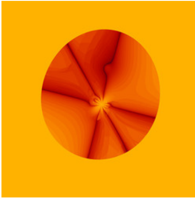
asz-andrexrandom-1-29.jpg
