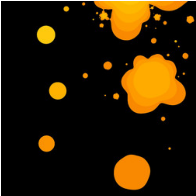
Ikm3-AlternativeFunctions-04.jpg
