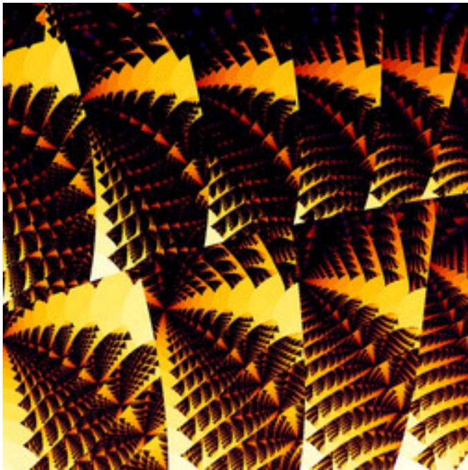
mt-barnsleyishMest-06.jpg
