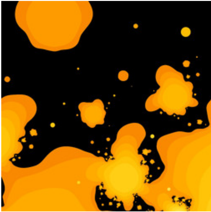
lkm3-AlternativeFunctions-01.jpg
