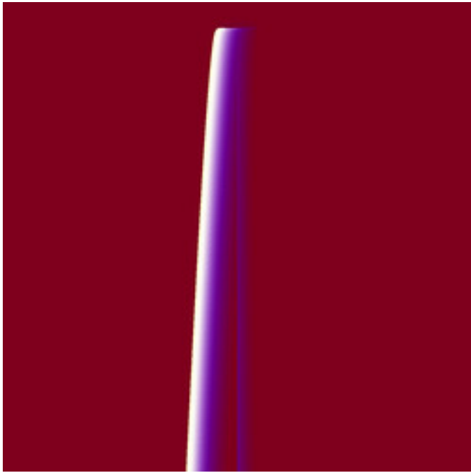
mt-GeneralizedCelticJulia-15.jpg
