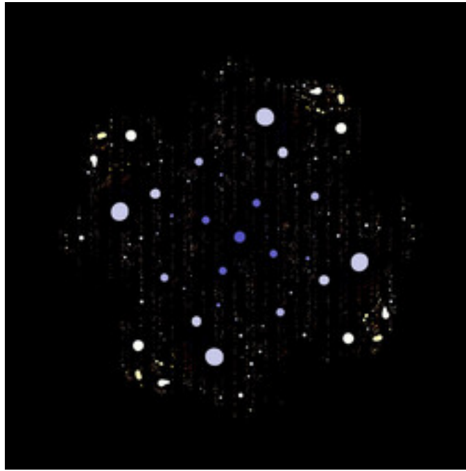
mt-rudys-cubic-mandelbrot-13.jpg
