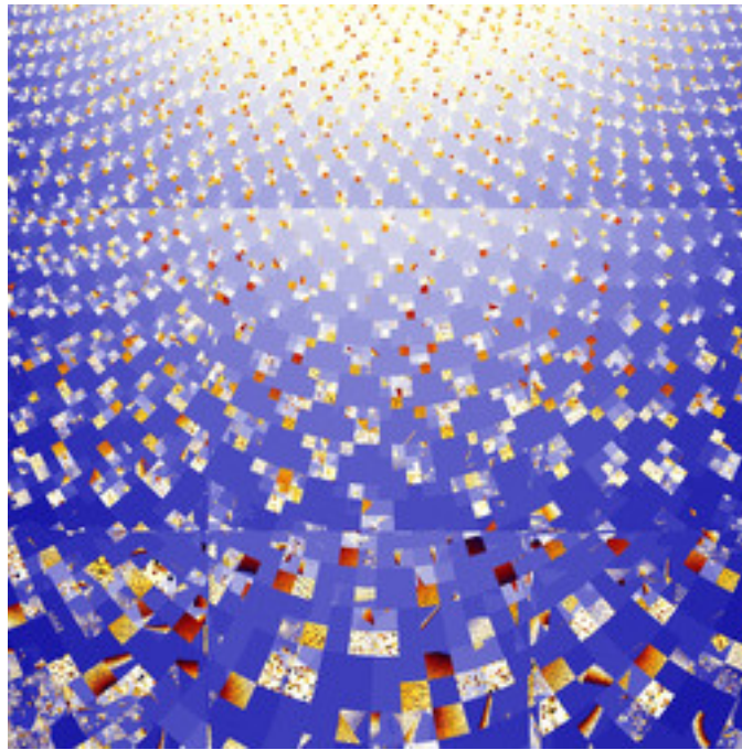
mt-biomorphIMset-07.jpg
