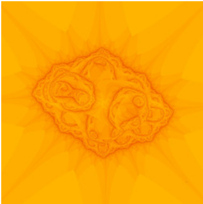
reb-JuliaCrossOrbitLambda-03.jpg
