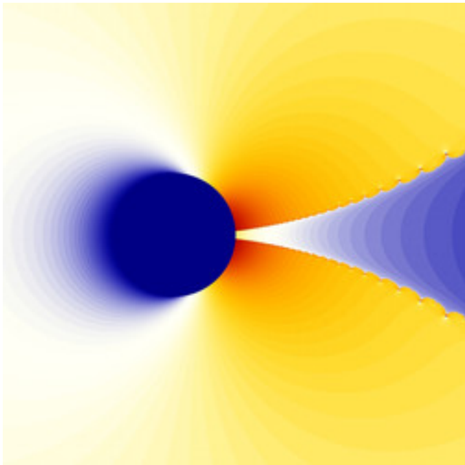
dmj-Magnet1-01.jpg
