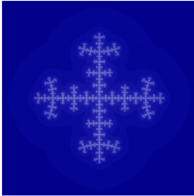
mt-GeneralizedCelticJulia-02.jpg
