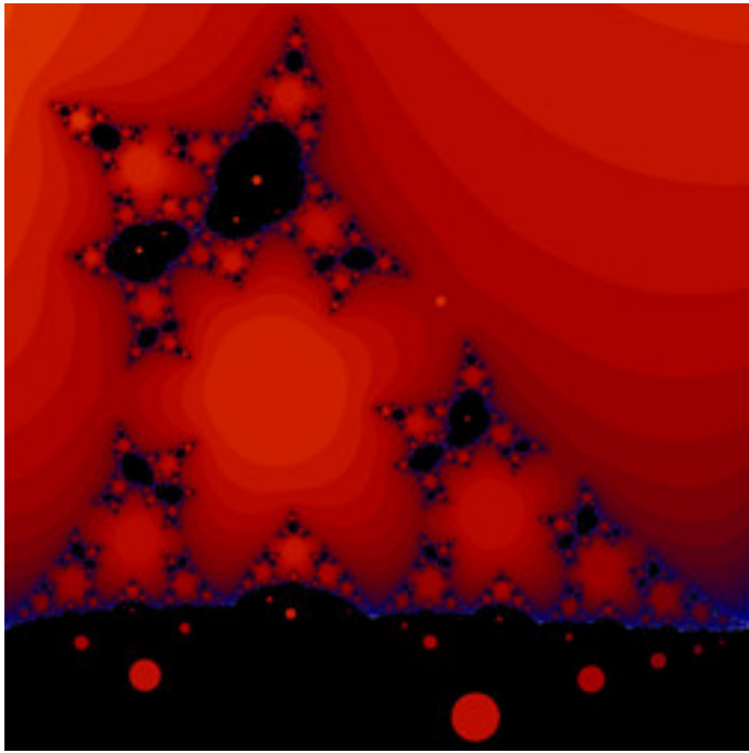
Ikm3-AlternativeFunctions-07.jpg
