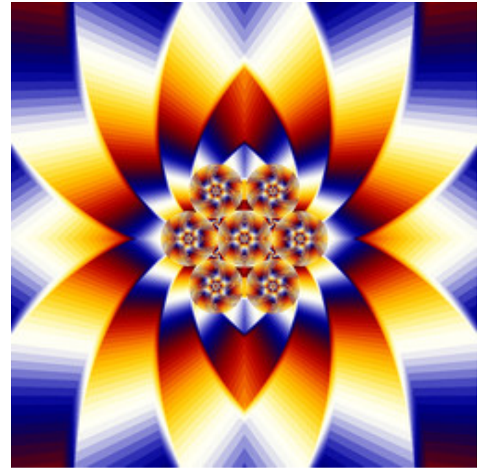
reb-JuliaTentMap-05.jpg
