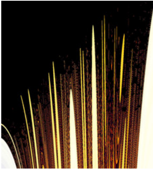
mt-990625bMset-08.jpg
