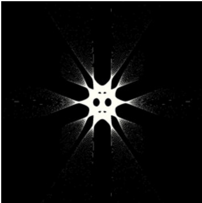
reb-FormulaTracer-04A.jpg
