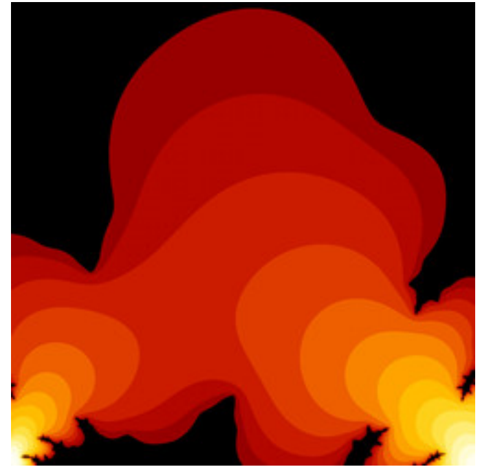
lkm-CompundingTM-03.jpg
