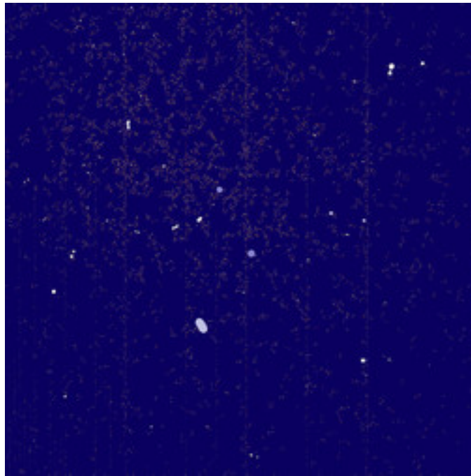
dmj-PhoenixDoubleNova-26.jpg
