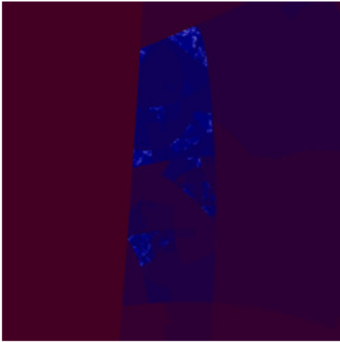
mt-990807bMset-13.jpg
