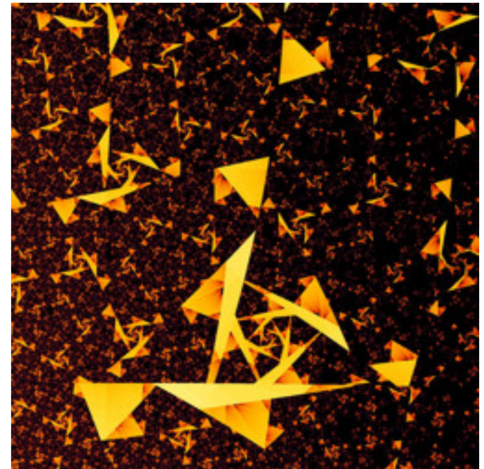
lkm-GeneralTentMandelbrot-08.jpg
