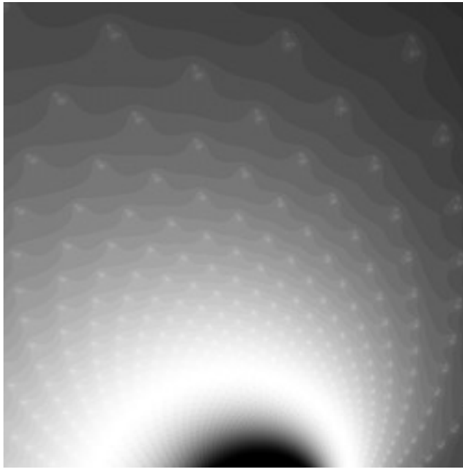
mt-modulate-mset-06.jpg
