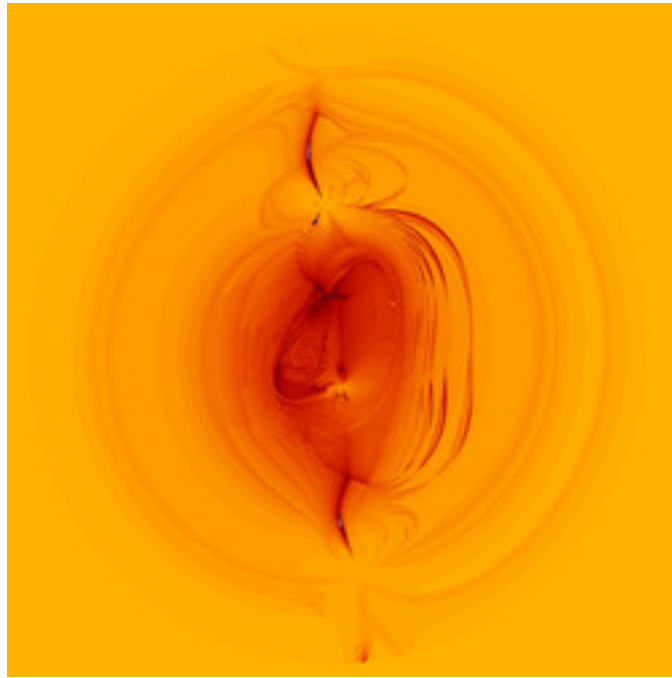
asz-andrextrandom-1-23.jpg
