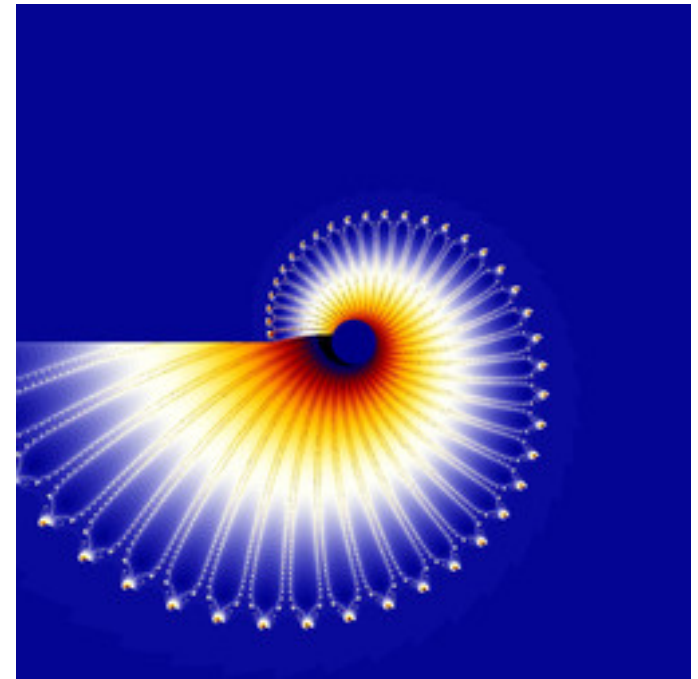
ads-Newton_02.jpg
