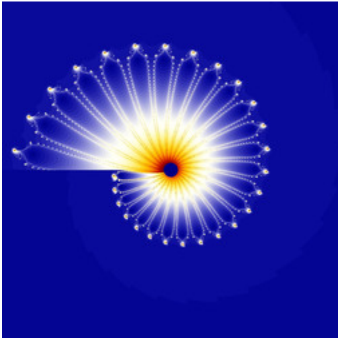
ads-Newton_01.jpg
