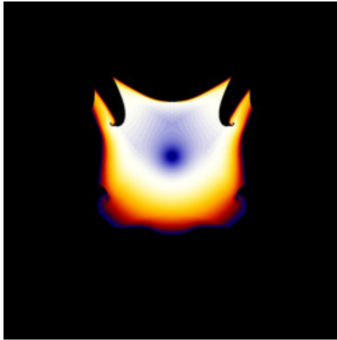
mt-zeepop-mset-30.jpg
