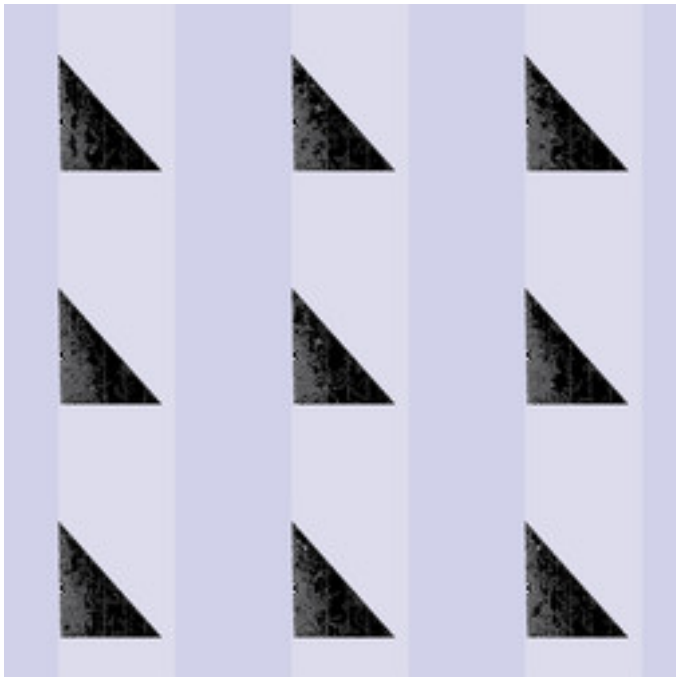
dmj-ManyNova-12.jpg
