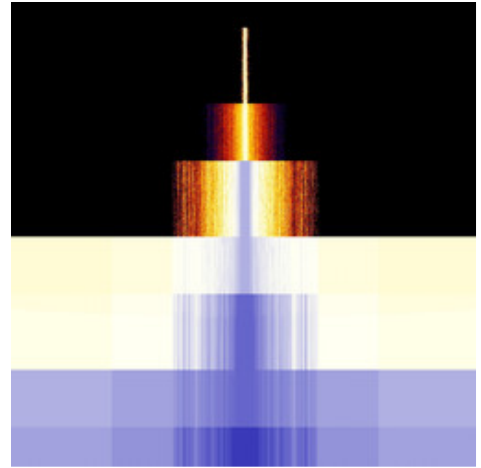
mt-bifunctionalMset-11.jpg
