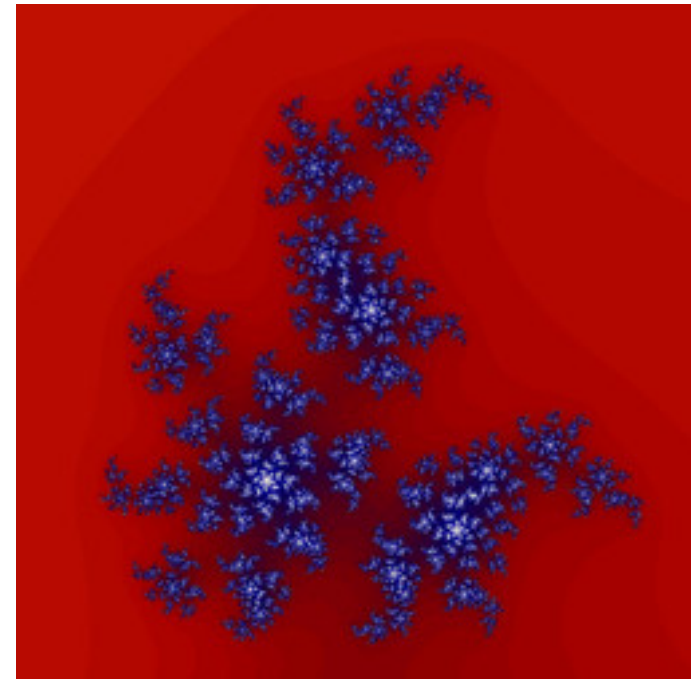
mt-990807bMset-02.jpg
