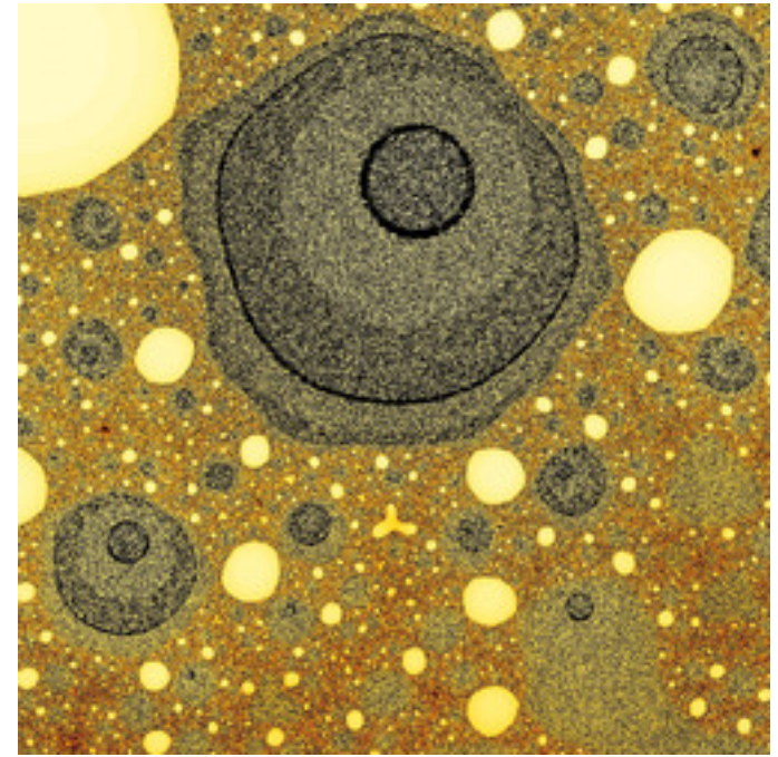
mt-magnetism-model-ii-07.jpg
