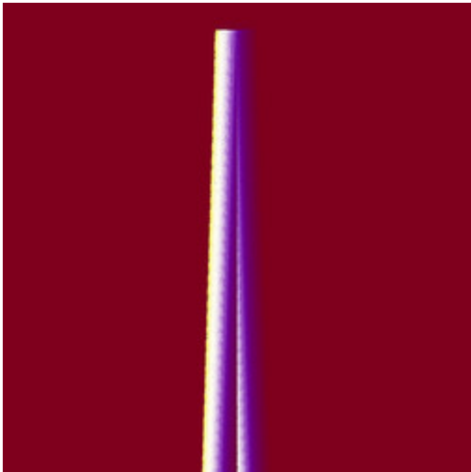
mt-GeneralizedCelticJulia-18.jpg
