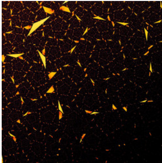
lkm-GeneralTentMandelbrot-08a.jpg
