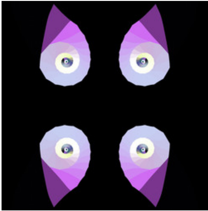
ldm-DM11a-04.jpg
