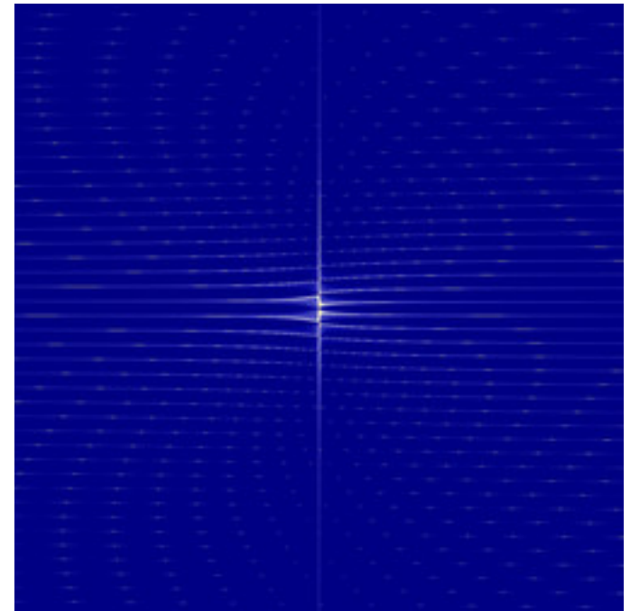
reb-GopalsamyFn-08.jpg
