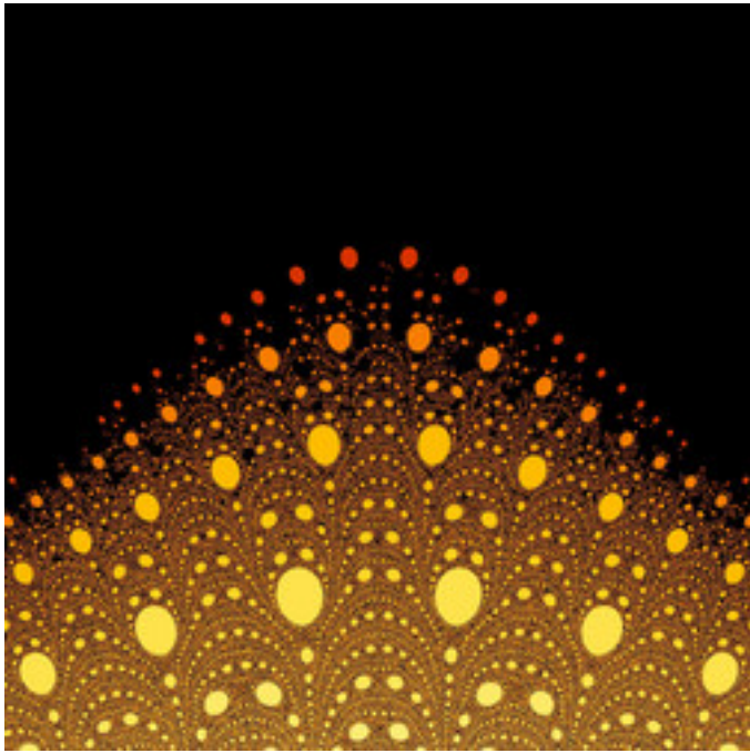
lkm-MitchsMandelbrot-03.jpg
