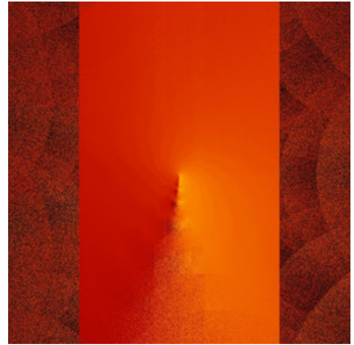
mt-newton-twist-09.jpg
