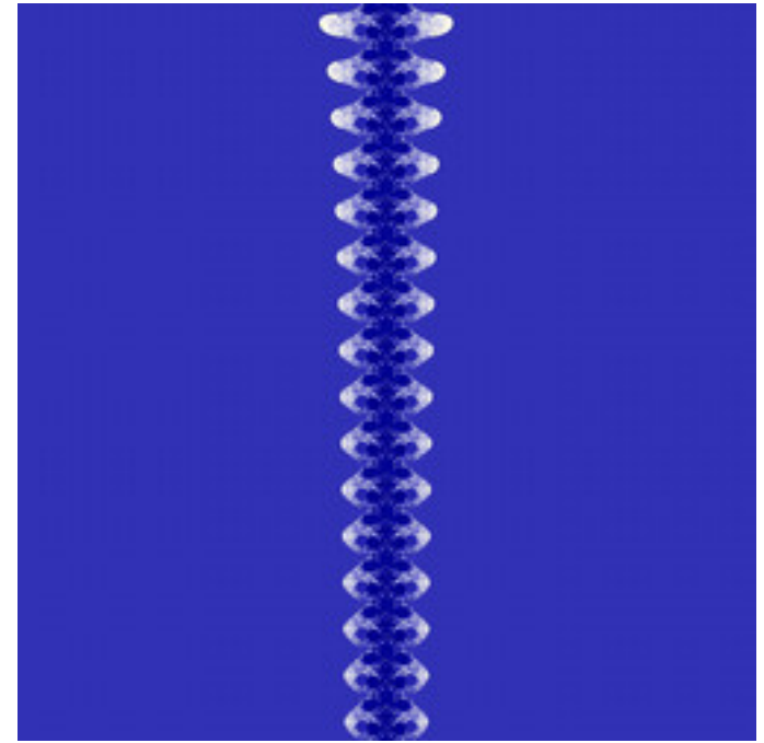
ldm-DM23-11.jpg
