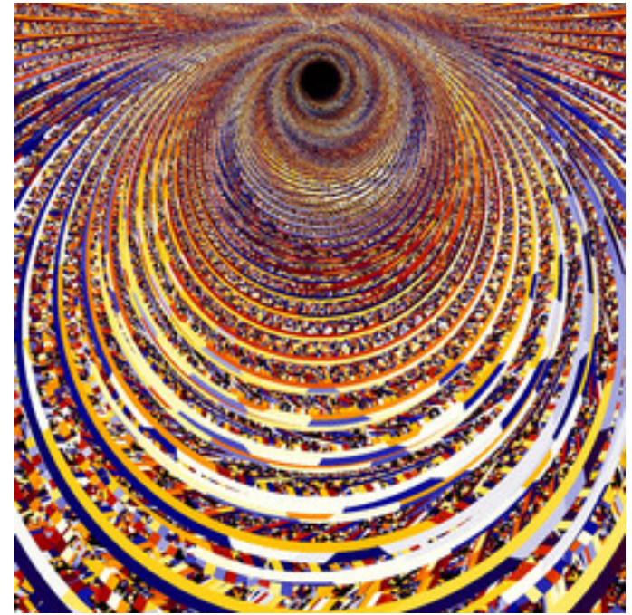
reb-JuliaTentMap-21B.jpg
