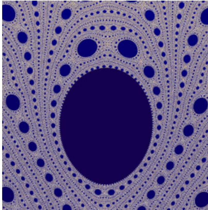
lkm-MitchsMandelbrot-05.jpg
