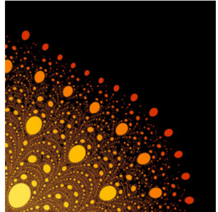
lkm-MitchsMandelbrot-04.jpg
