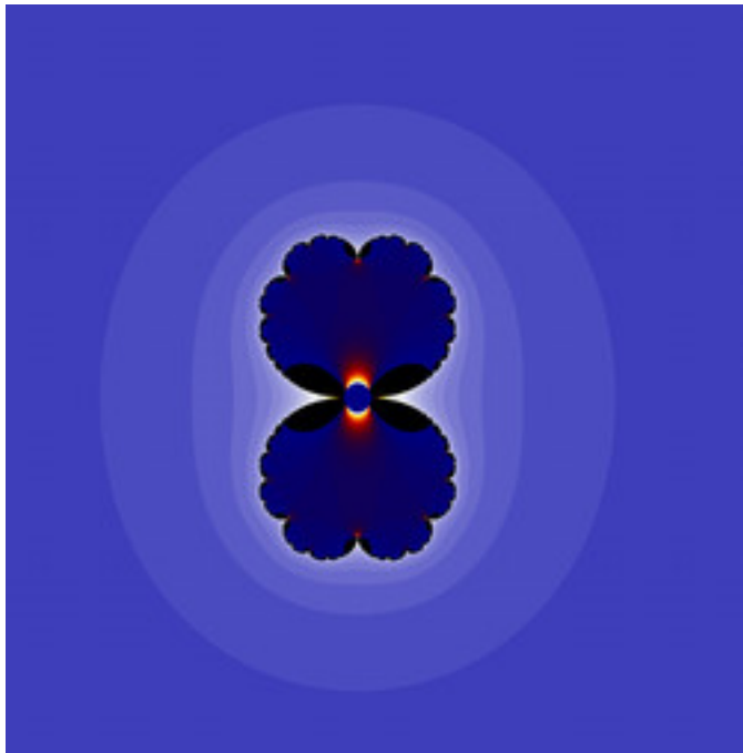
mt-zeepop-mset-56.jpg
