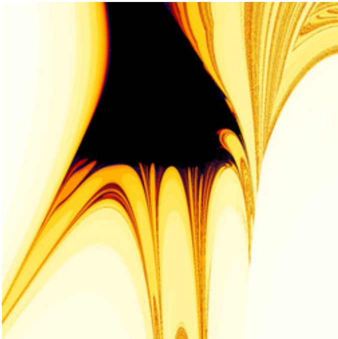
mt-990807aMset-38.jpg
