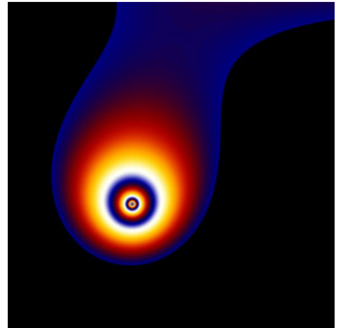
mt-newton-error-03a.jpg
