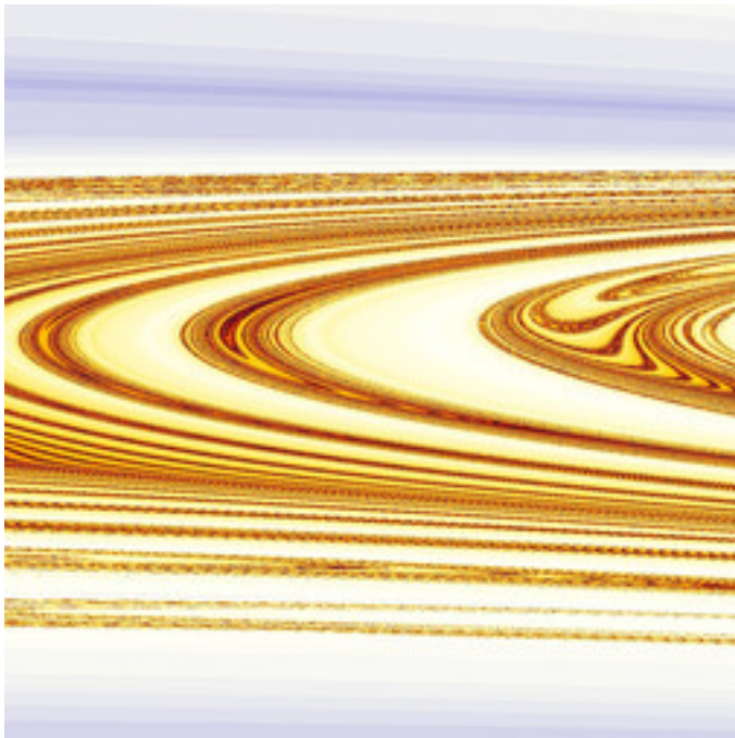
mt-990625bMset-06.jpg
