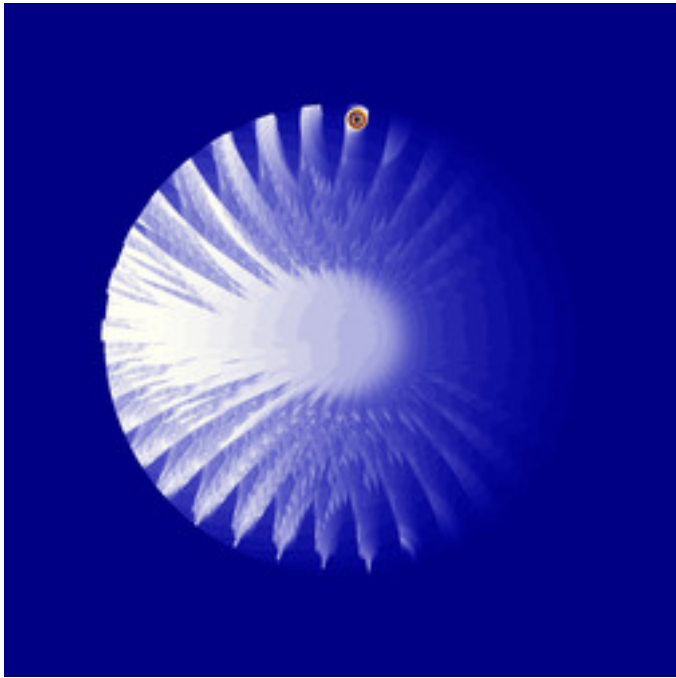
reb-PseudoZeePi-03.jpg
