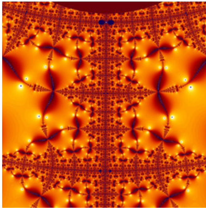
dmj-NovaMandel-03.jpg
