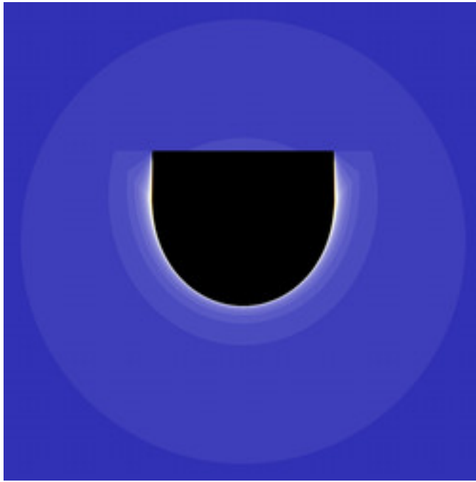
mt-barnsleyishMest-14.jpg
