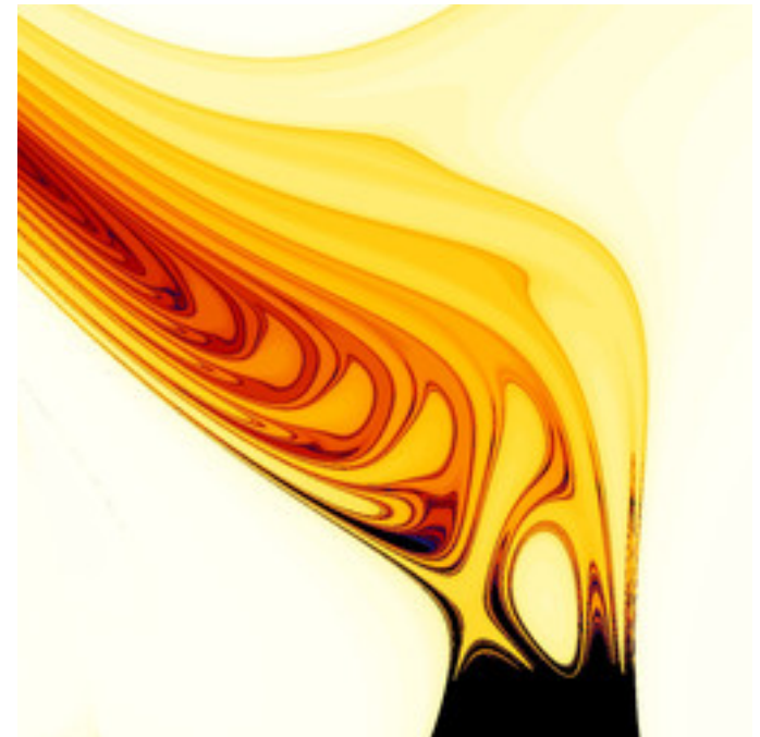
mt-990807aMset-42.jpg
