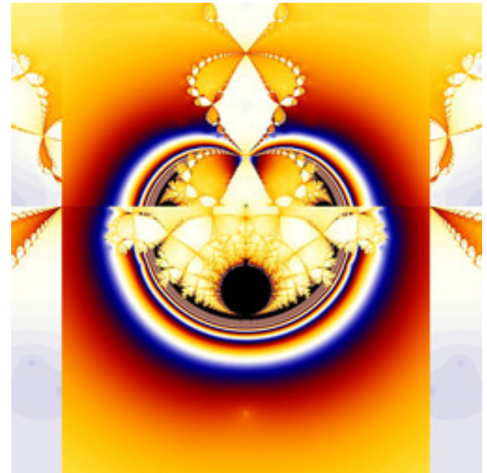
mt-newton-error-23.jpg
