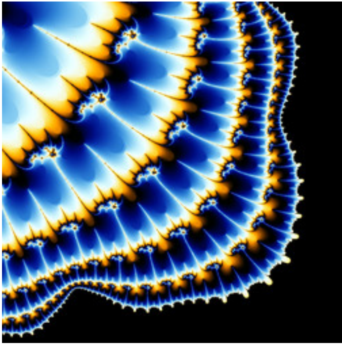
standard-FastMandel-04.jpg
