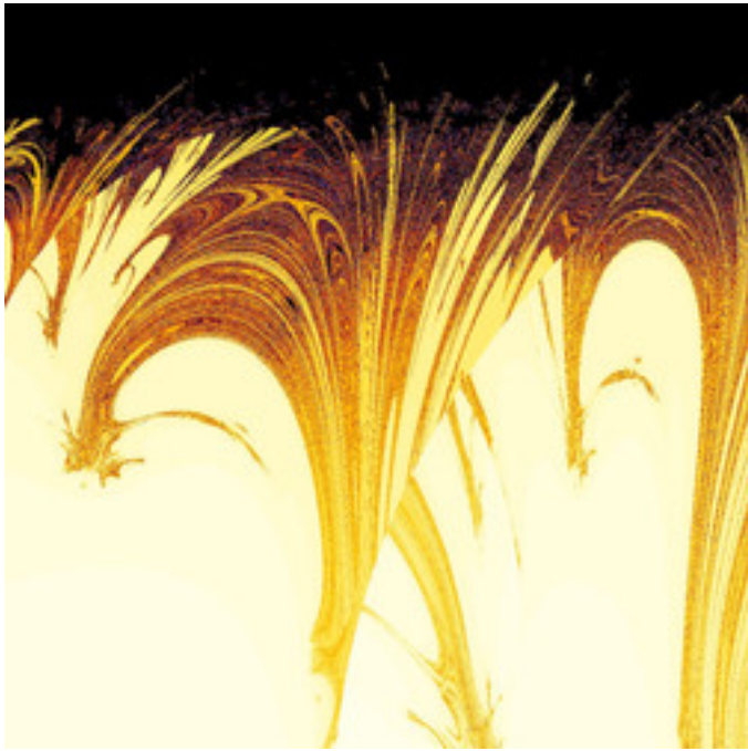
mt-990807aMset-23.jpg
