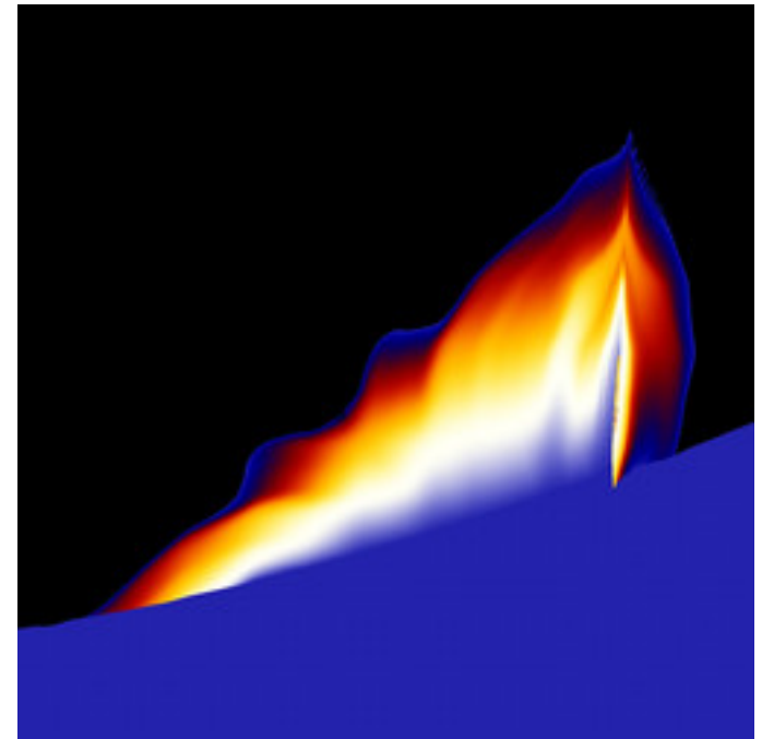
lkm3-FourierPopCorn-15A.jpg
