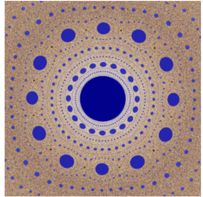
lkm-MitchsMandelbrot-01.jpg
