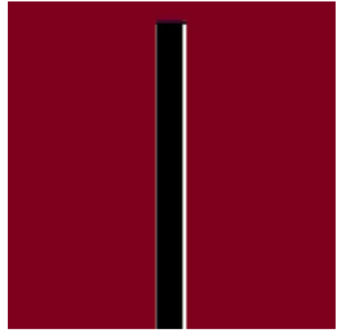
mt-GeneralizedCelticJulia-34.jpg
