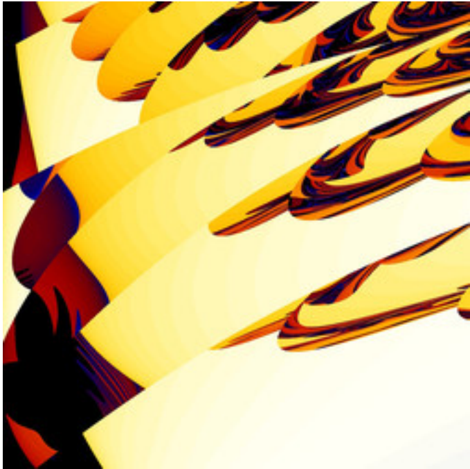
mt-990807aMset-26.jpg
