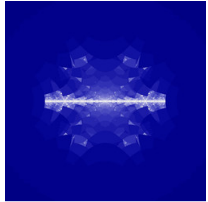
mt-rudys-cubic-mandelbrot-01.jpg
