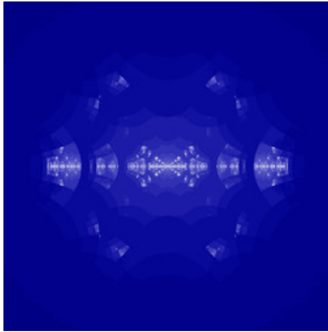
mt-rudys-cubic-mandelbrot-02.jpg
