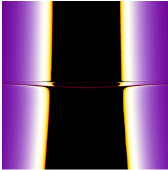
mt-GeneralizedCelticJulia-56.jpg
