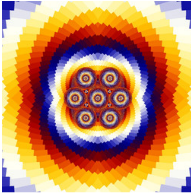
reb-JuliaTentMap-06.jpg
