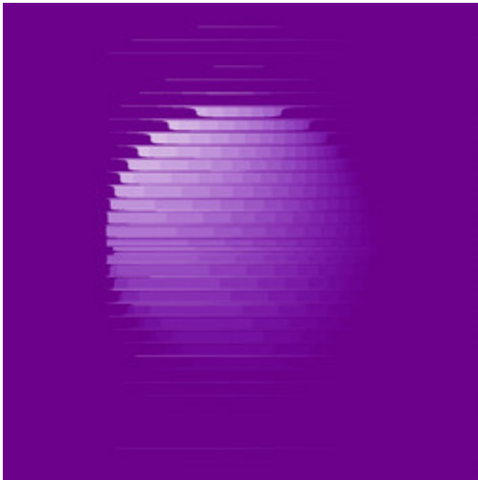
mt-GeneralizedCelticJulia-66.jpg
