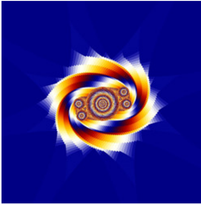
reb-JuliaTentMap-15.jpg
