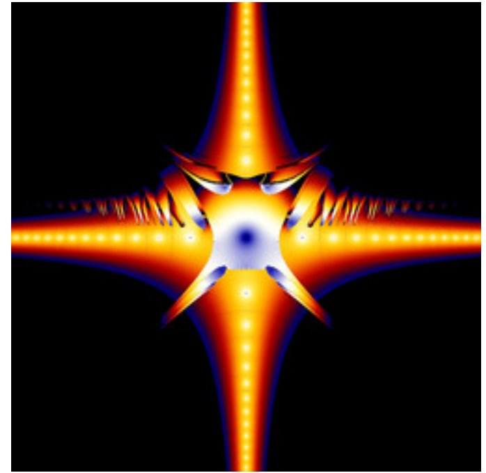
mt-zeepop-mset-11.jpg
