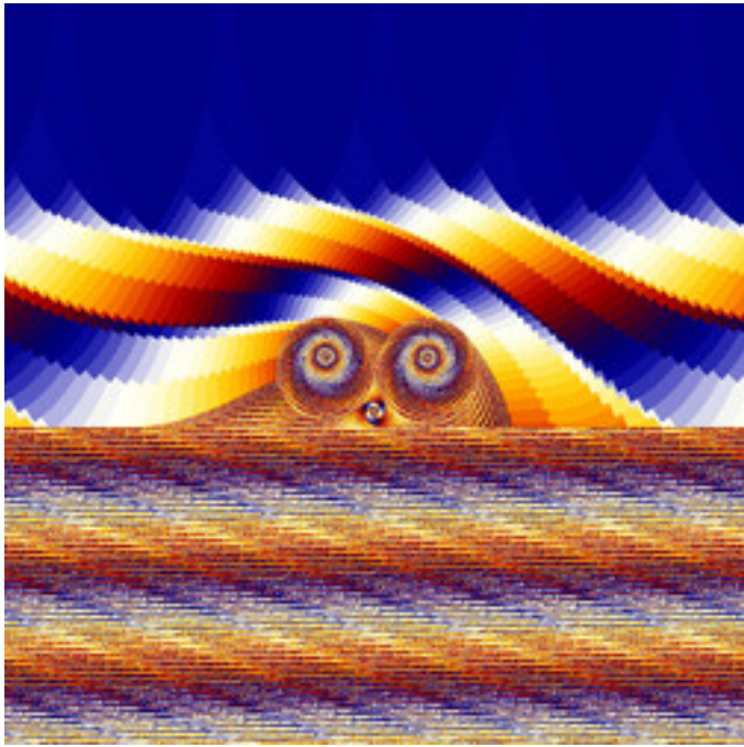
reb-JuliaTentMap-16.jpg
