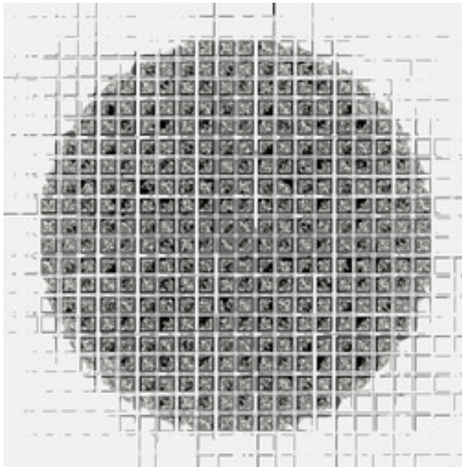
lkm3-FourierPopCorn-10.jpg
