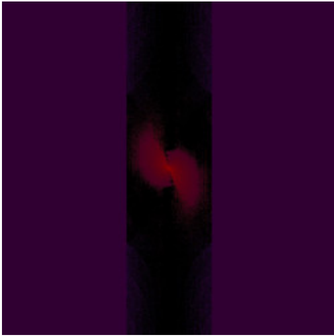
mt-newton-twist-05.jpg
