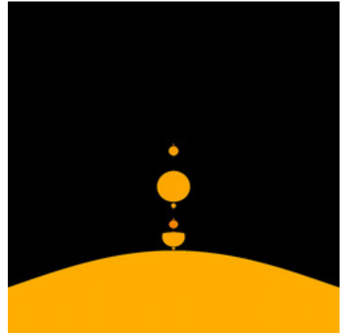
mt-barnsleyishMest-19.jpg
