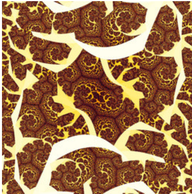
mt-barnsleyishJulia-14.jpg
