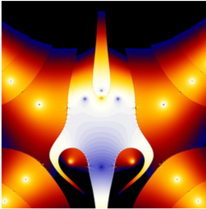
mt-zeepop-mset-24.jpg
