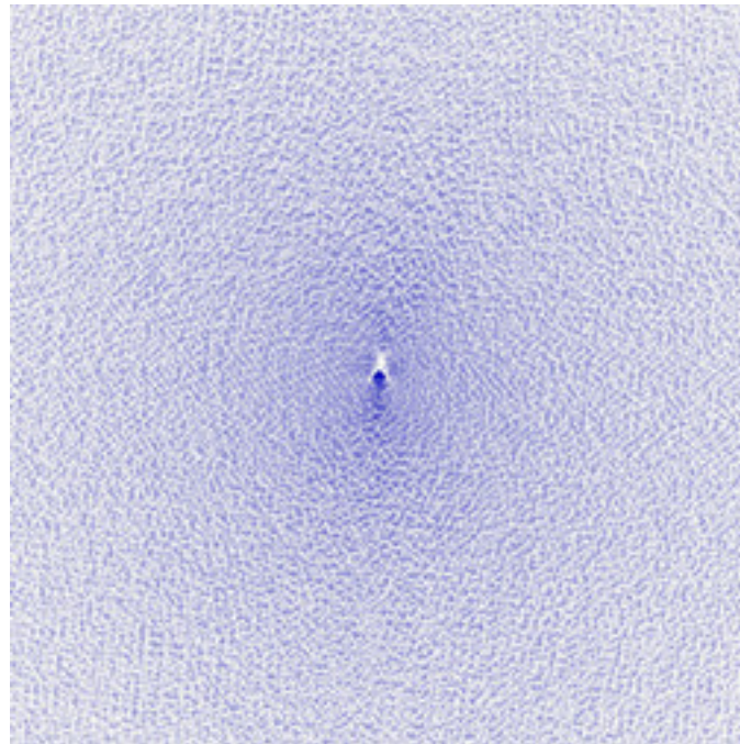
dmj-fBmNovaMandel-01.jpg
