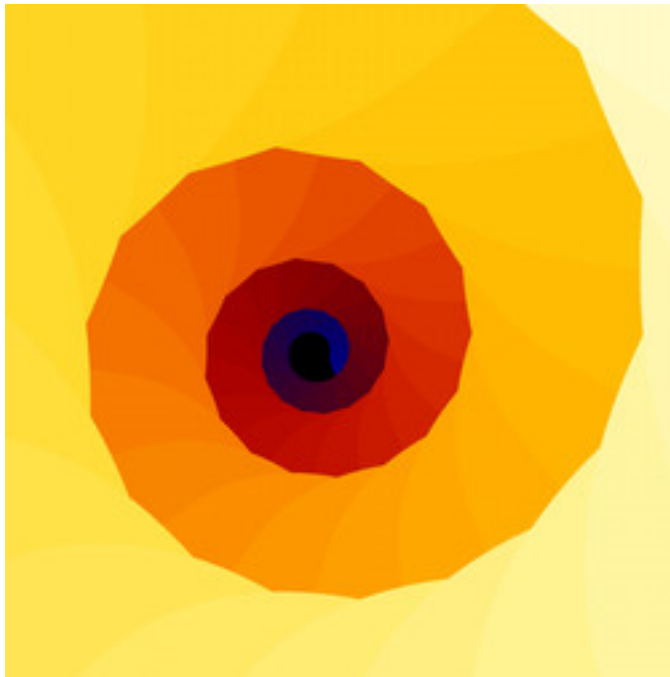
ldm-DM11a-01.jpg
