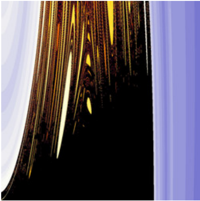
mt-990625bMset-09.jpg
