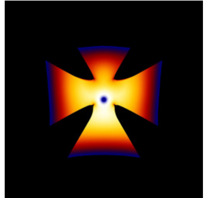
mt-zeepop-mset-02.jpg
