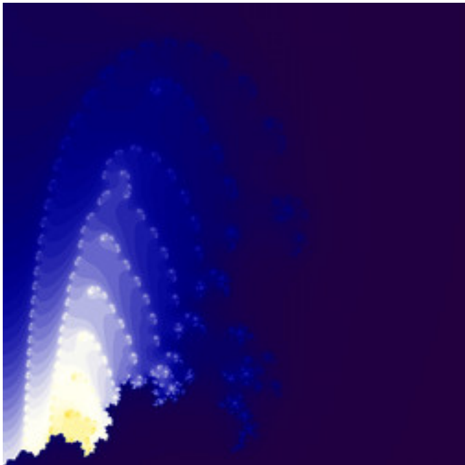
lkm-CompundingTM-02.jpg
