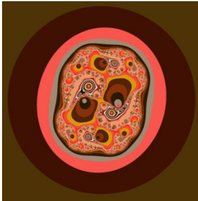
mt-magnetism-model-ii-julia-03.jpg
