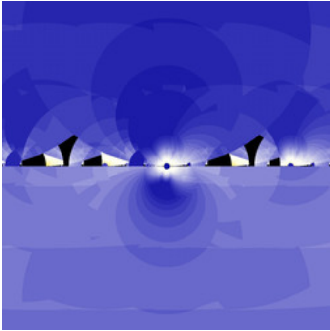
mt-zeepop-julia-19.jpg
