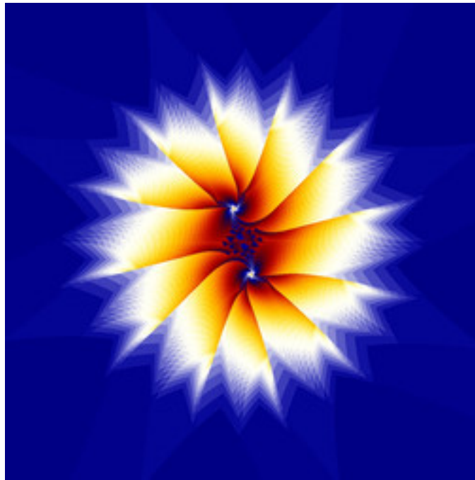
reb-JuliaTentMap-31.jpg
