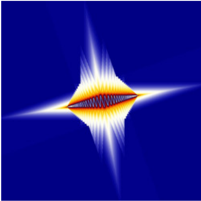
reb-FunBarnsley1Julia-04.jpg
