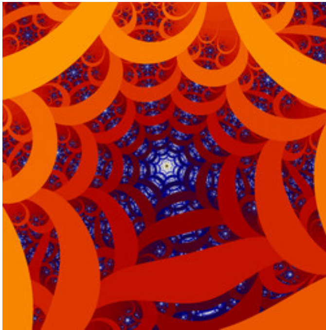
lkm-GapMandelbrot-02.jpg
