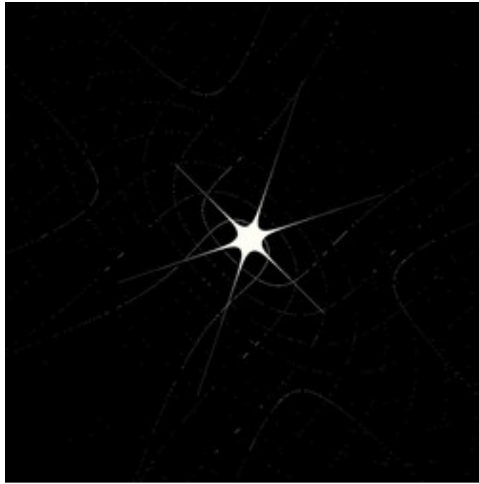
reb-FormulaTracer-06B.jpg
