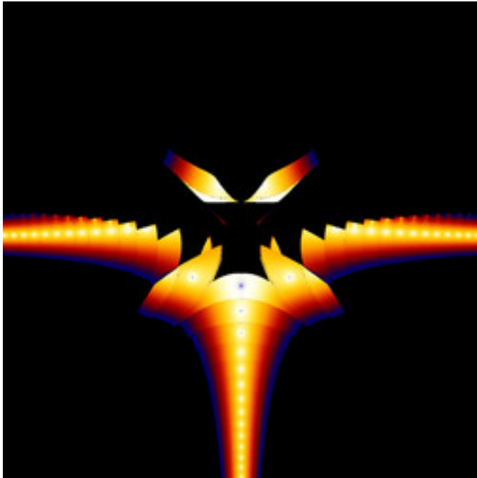
mt-zeepop-mset-10.jpg
