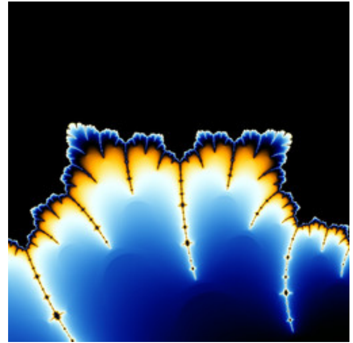
standard-FastMandel-08.jpg
