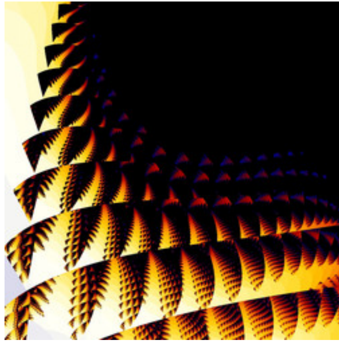
mt-barnsleyishMest-08.jpg
