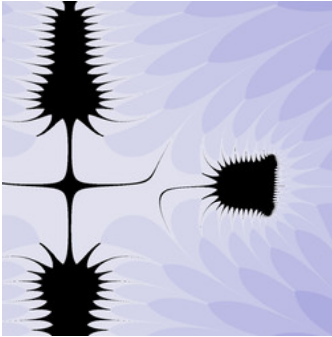
reb-3RDIMManowar01-03.jpg
