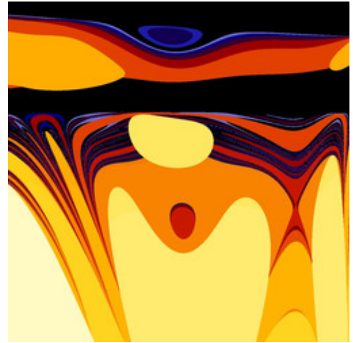
mt-990807aMset-33.jpg
