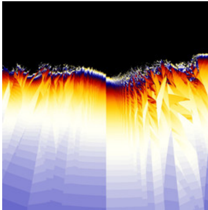
lkm-GeneralTentMandelbrot-NEW1-03.jpg
