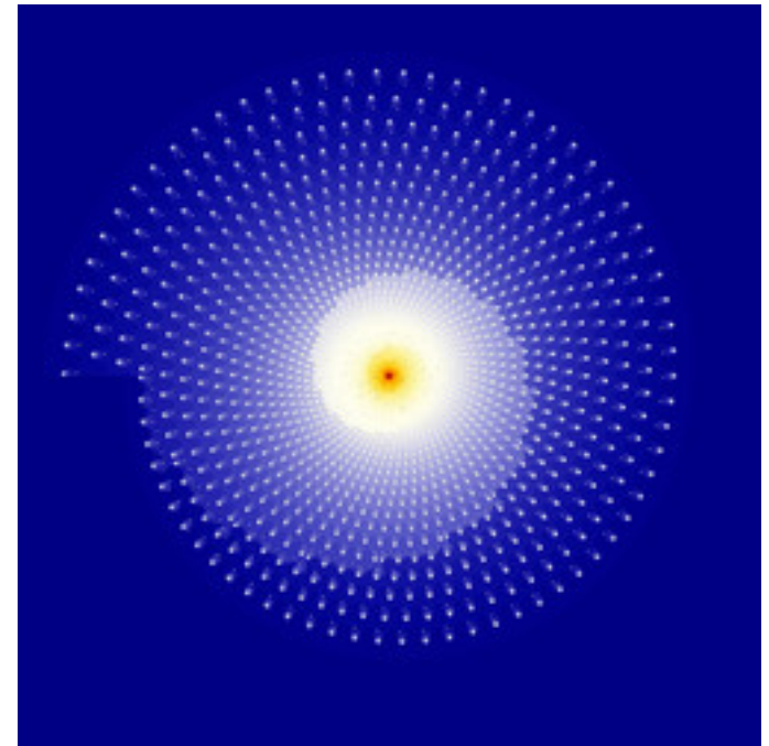
reb-LambdaPower-05.jpg
