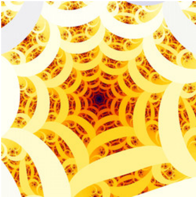
lkm-GapMandelbrot-02A.jpg
