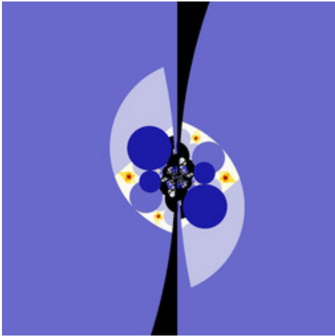
reb-FunBarnsley1Julia-07.jpg
