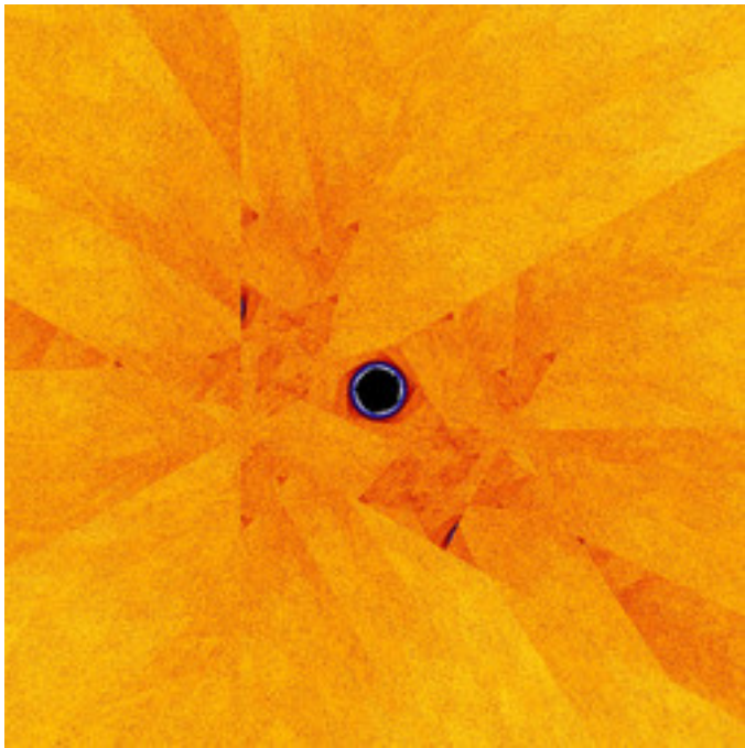
mt-rudys-cubic-julia-02.jpg
