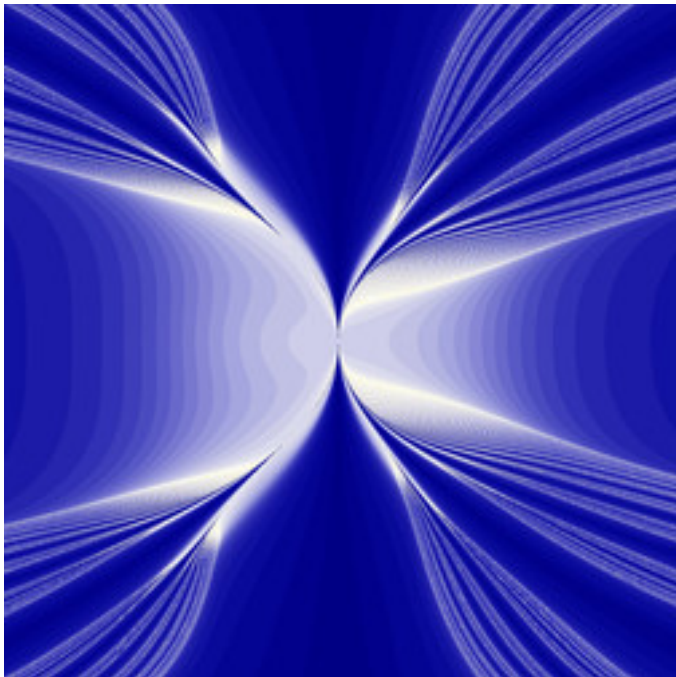
reb-GopalsamyFn-32.jpg
