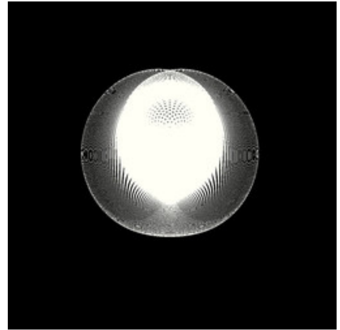
reb-FormulaTracer-02A.jpg
