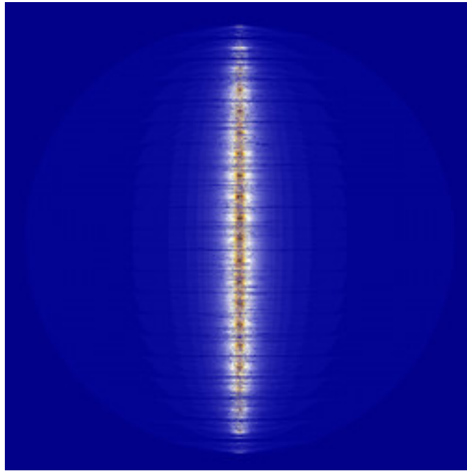
mt-bifunctionalMset-06.jpg
