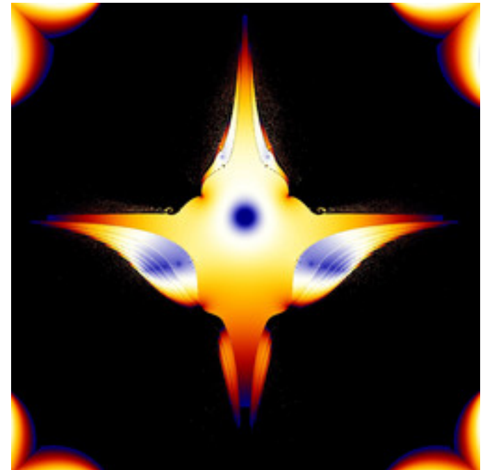
mt-zeepop-mset-26.jpg
