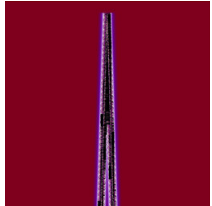
mt-GeneralizedCelticJulia-16.jpg
