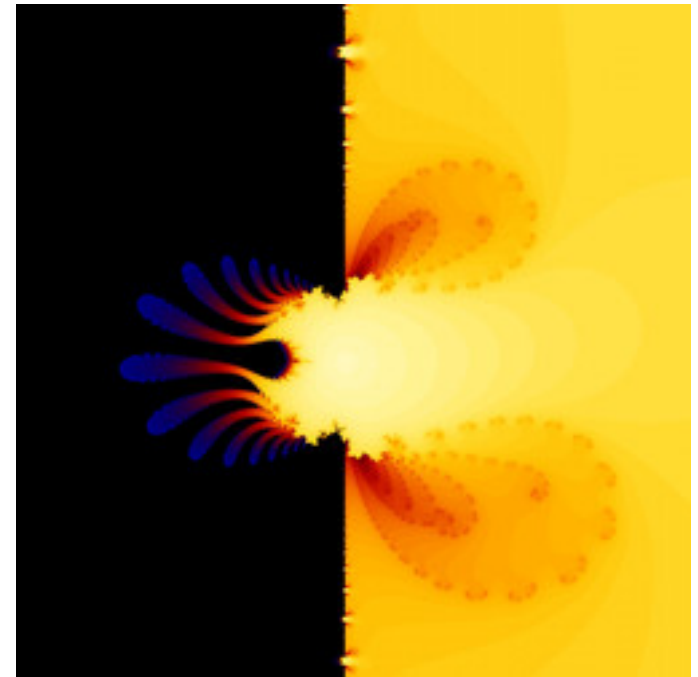
lkm-CompundingTM-06.jpg
