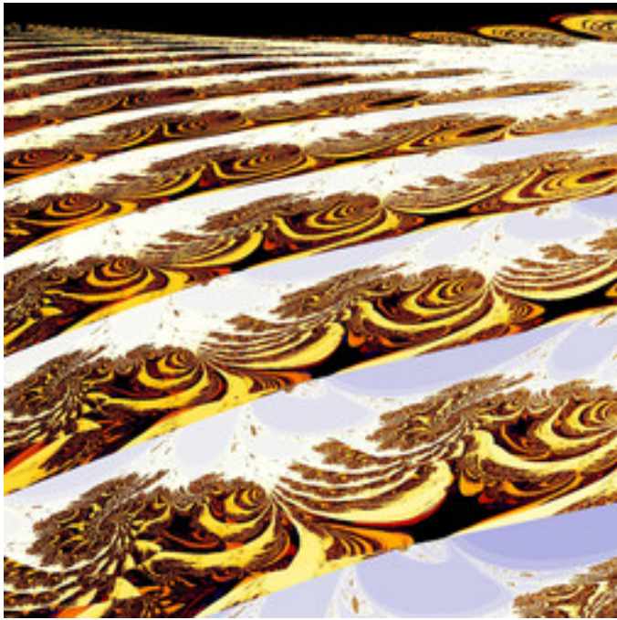
mt-bifunctionalMset-01.jpg
