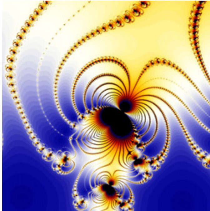
lkm-NewtonMethod-02.jpg
