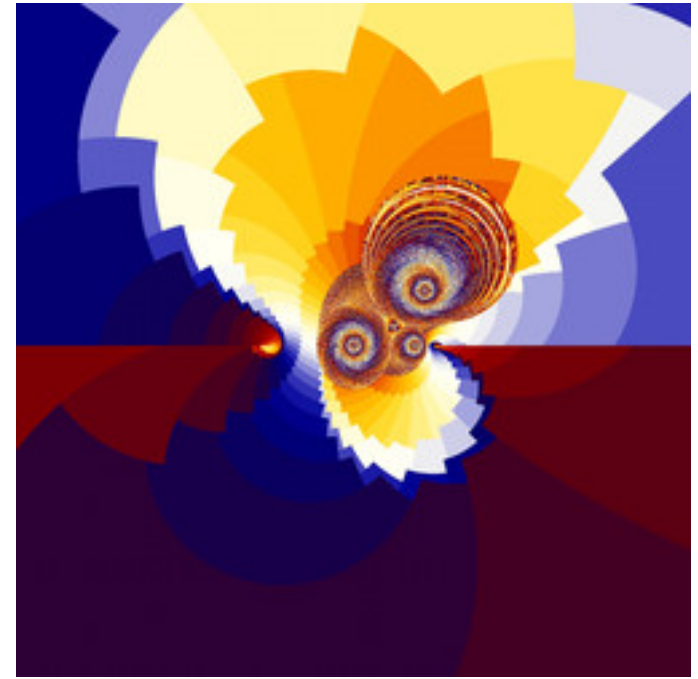
reb-JuliaTentMap-14.jpg
