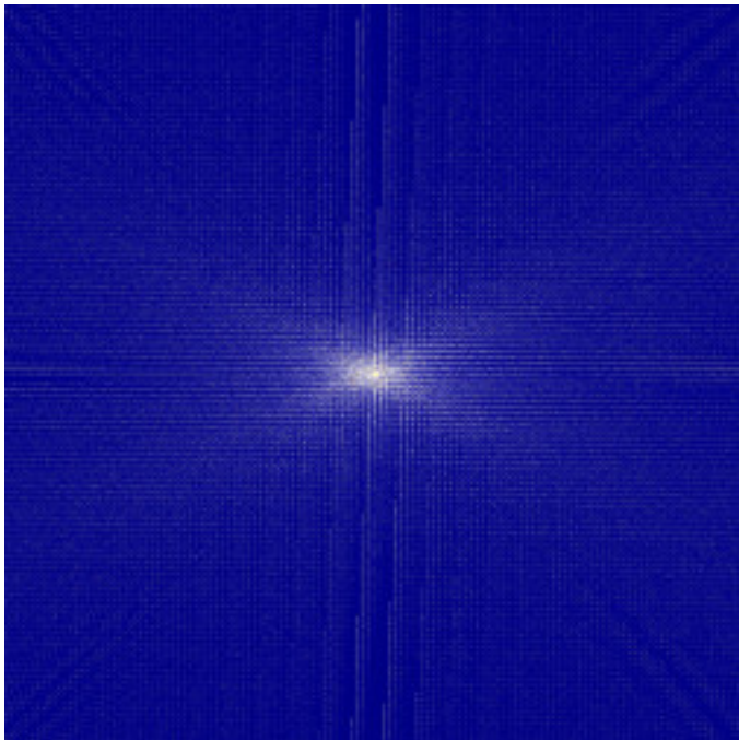
reb-GopalsamyFn-08C.jpg
