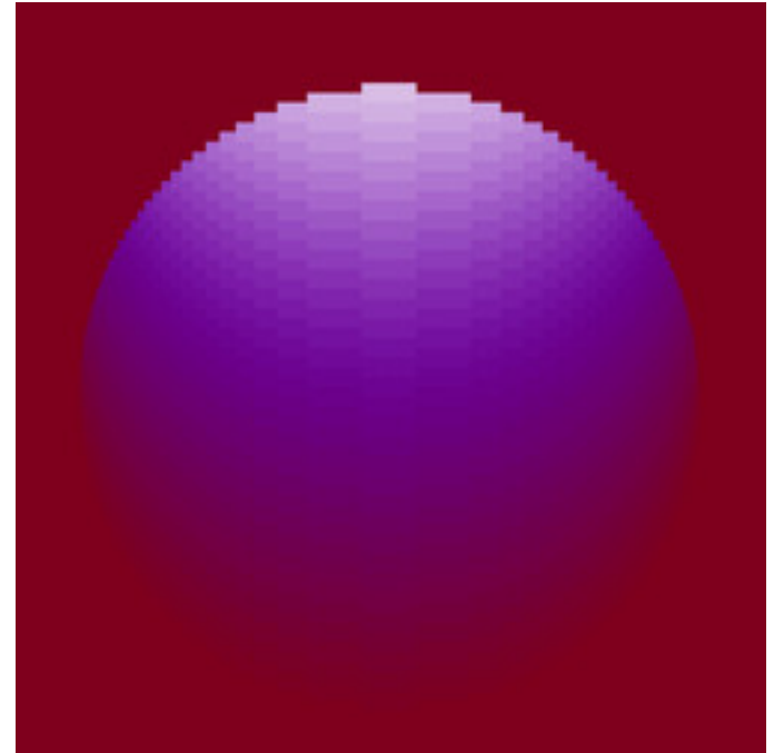
mt-GeneralizedCelticJulia-58.jpg
