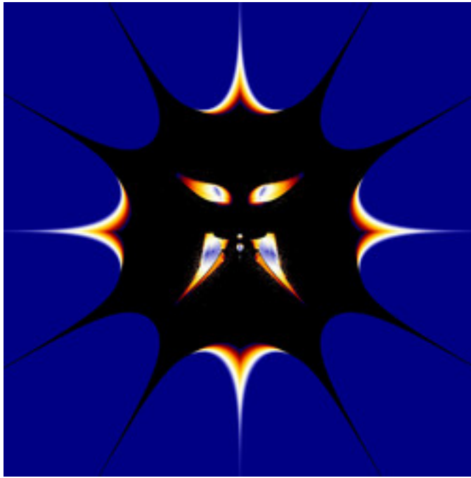
mt-zeepop-mset-47.jpg
