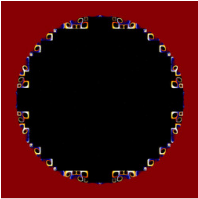
lkm3-FourierPopCorn-04C.jpg
