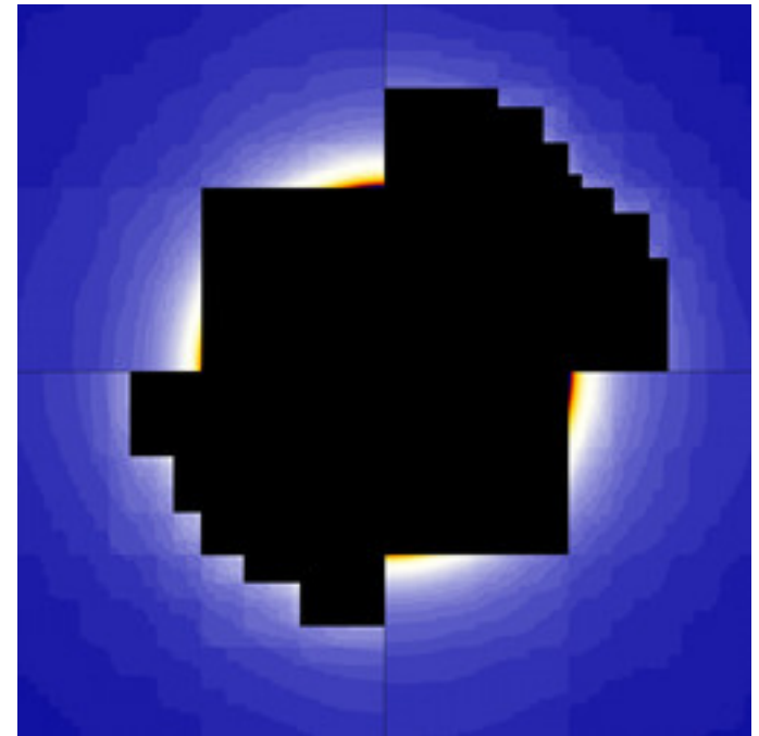
reb-SlopeExpFun_BarnsleyM2-05.jpg
