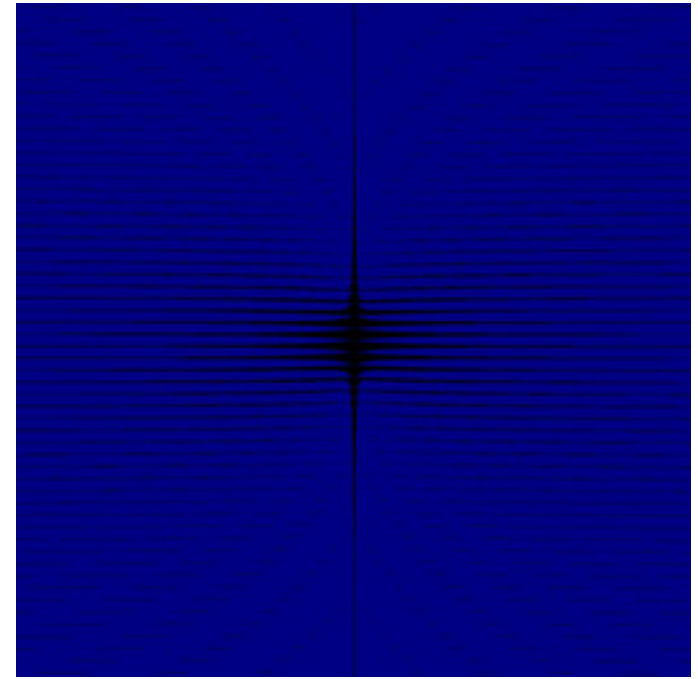
reb-GopalsamyFn-05.jpg
