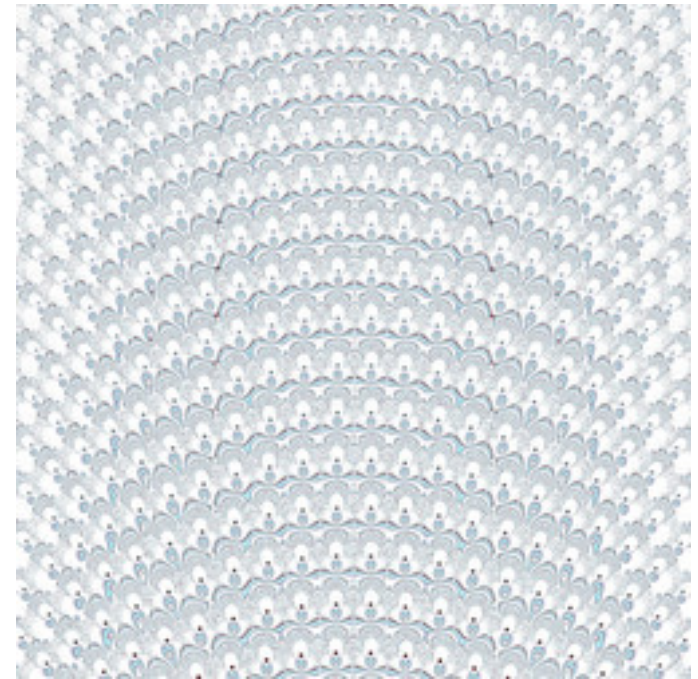
dmj-NovaMandel-11.jpg
