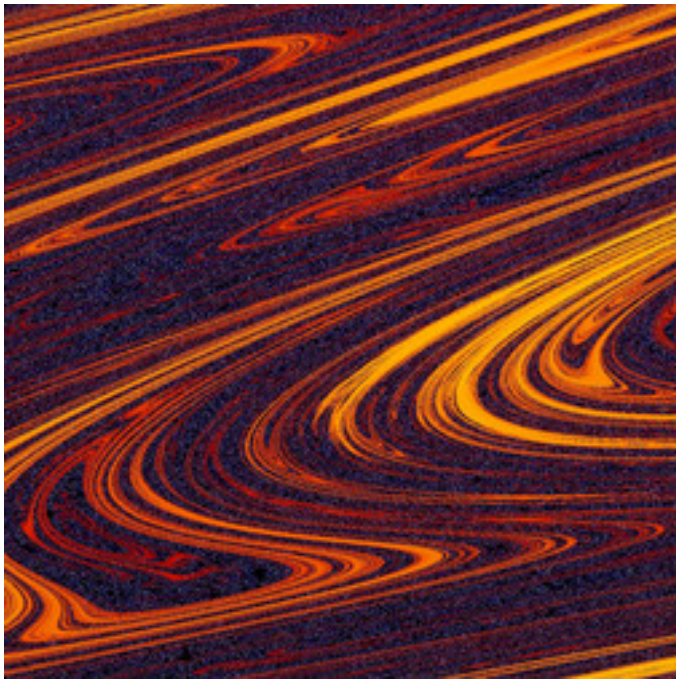
lkm3-RotatedMandelbrot-01.jpg
