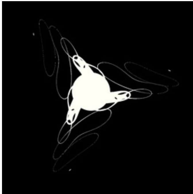
reb-FormulaTracer-03B.jpg
