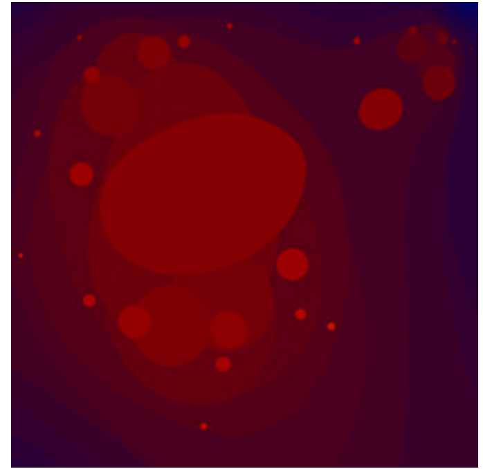
dmj-PhoenixDoubleNova-22.jpg
