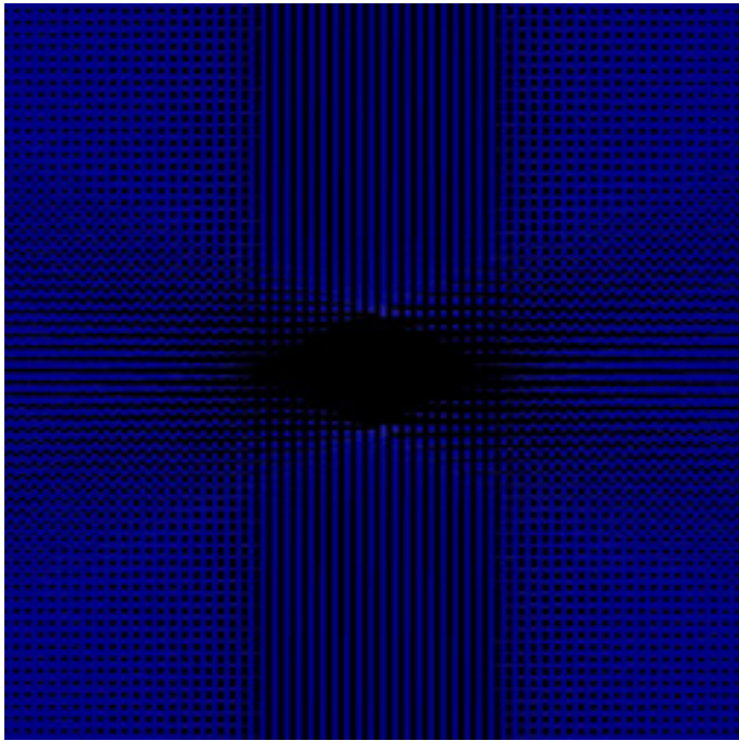
reb-GopalsamyFn-35.jpg
