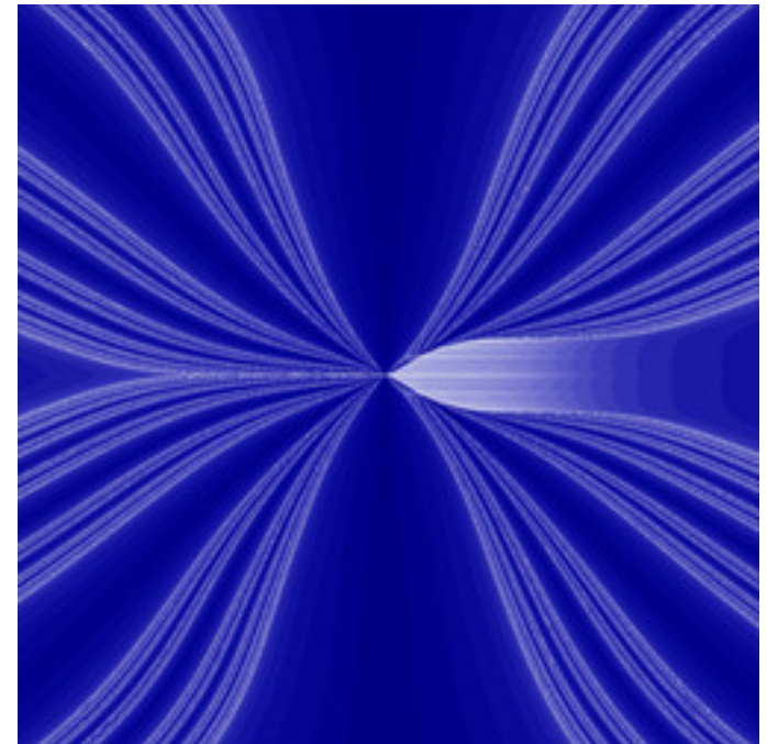
reb-GopalsamyFn-30.jpg
