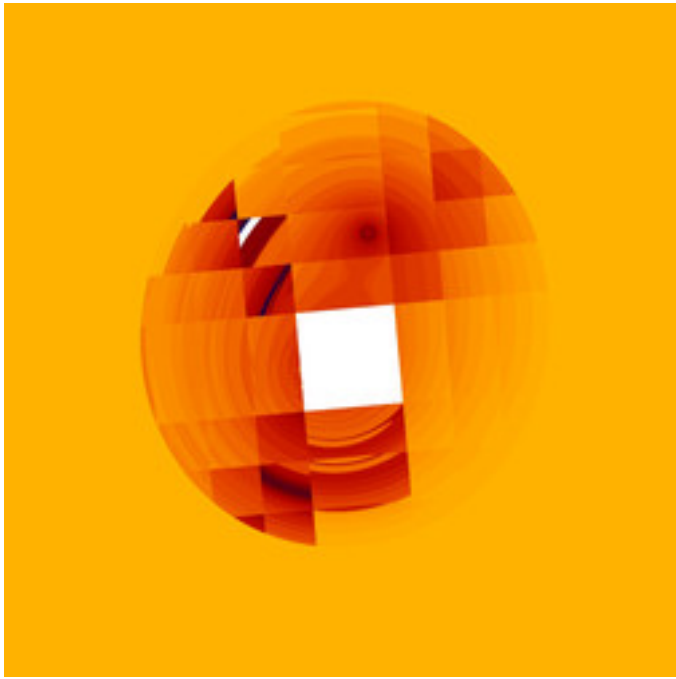
asz-andrexrandom-1-30.jpg
