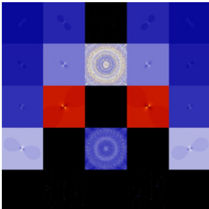
dmj-ManyNova-06.jpg
