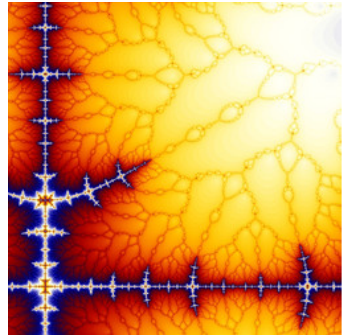
reb-IkenagaRoots-Julia-02.jpg
