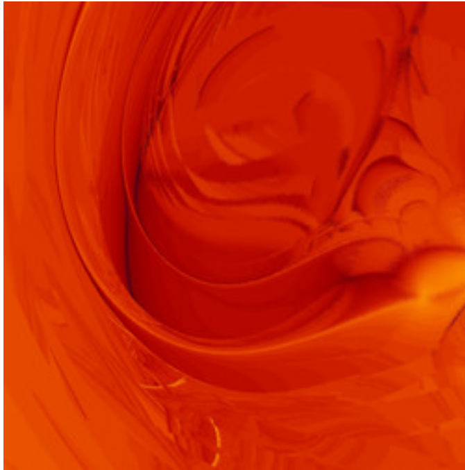
asz-andrexrandom-1-26.jpg
