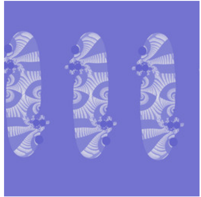
ldm-DM23-101.jpg
