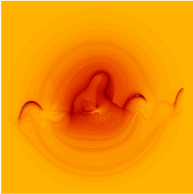
asz-andrextrandom-1-24.jpg
