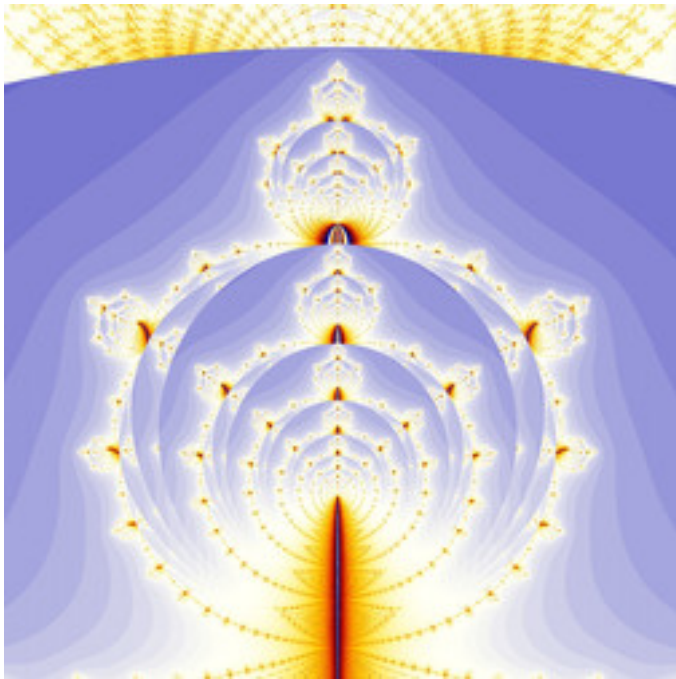
dmj-OrbitBoost-03.jpg
