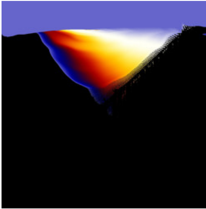
lkm3-FourierPopCorn-13.jpg
