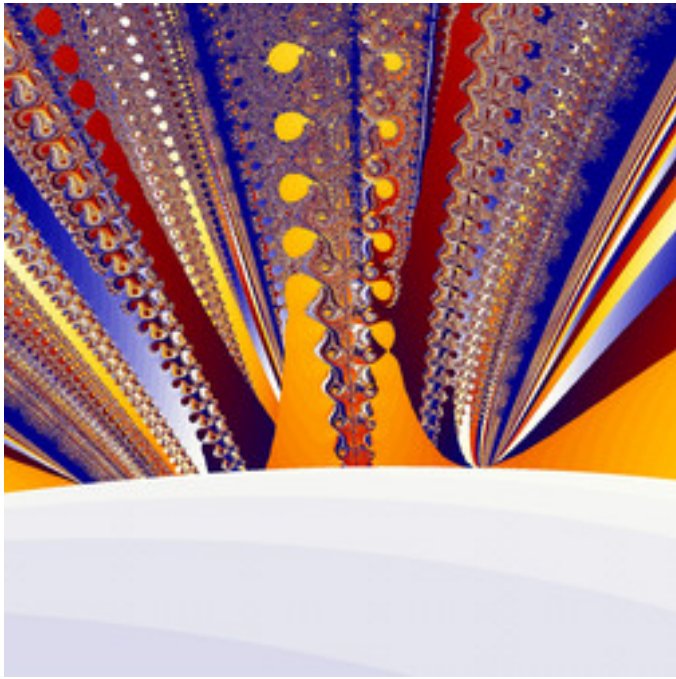
dmj-PhoenixDoubleNova-06.jpg
