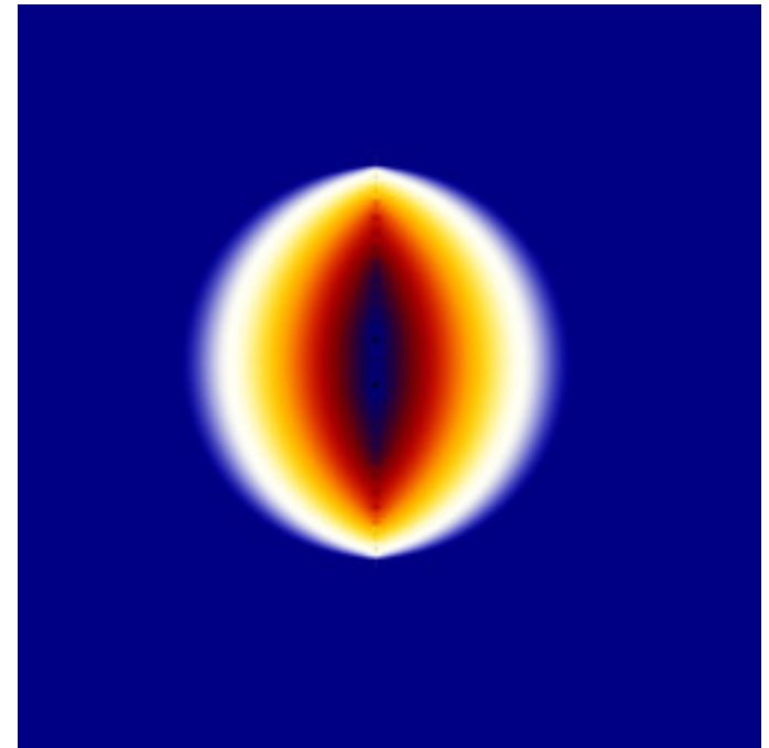
mt-zeepop-julia-08.jpg
