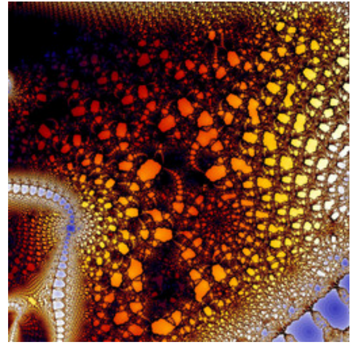
lkm3-ExtraFoam-01.jpg
