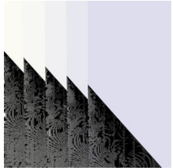
dmj-ManyNova-12B.jpg
