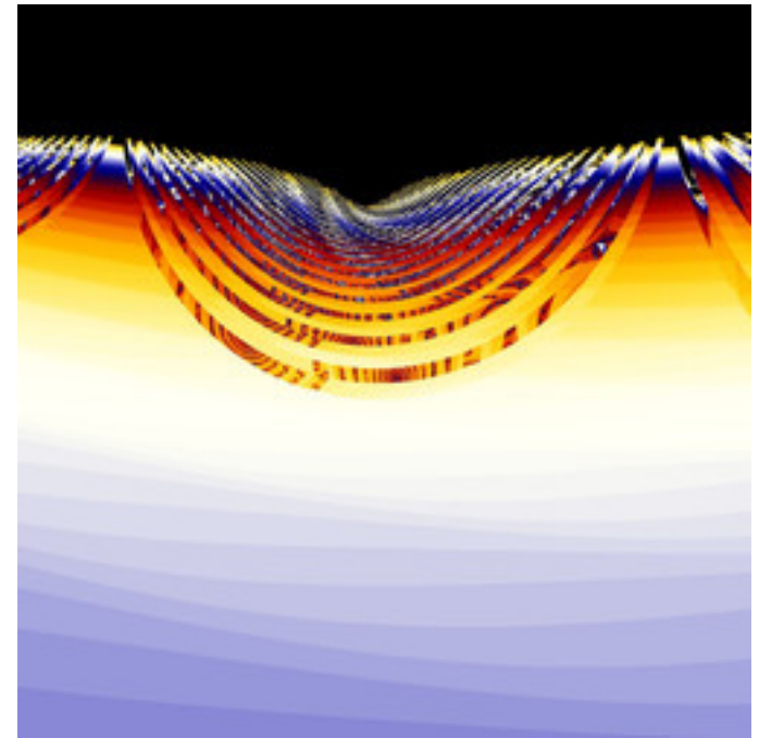
lkm-GeneralTentMandelbrot-NEW1-02.jpg
