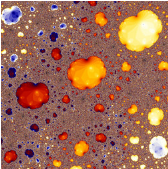
dmj-DoubleNova-09.jpg
