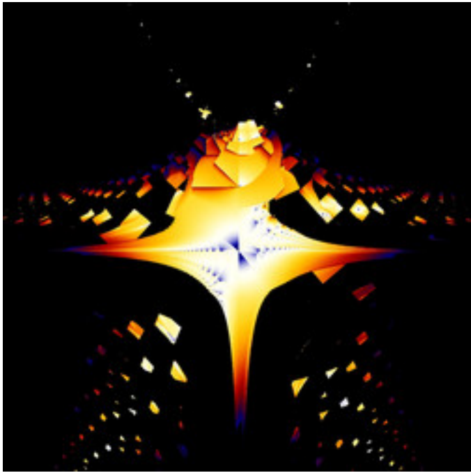
mt-zeepop-mset-37.jpg
