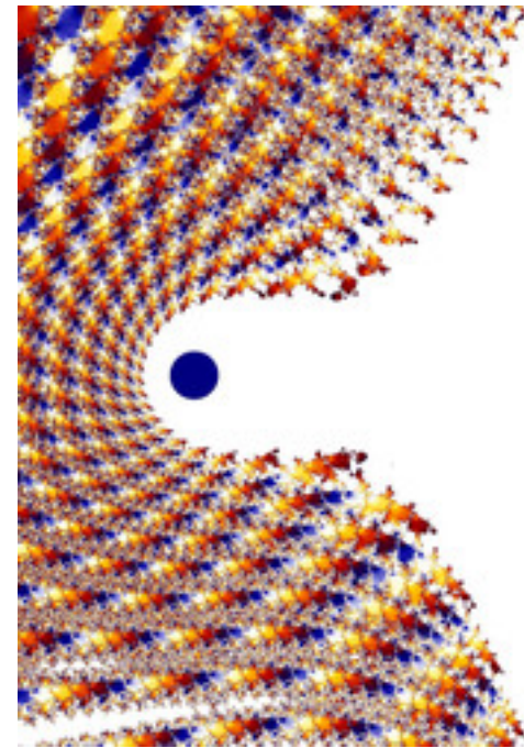
dmj-NovaMandel-02.jpg
