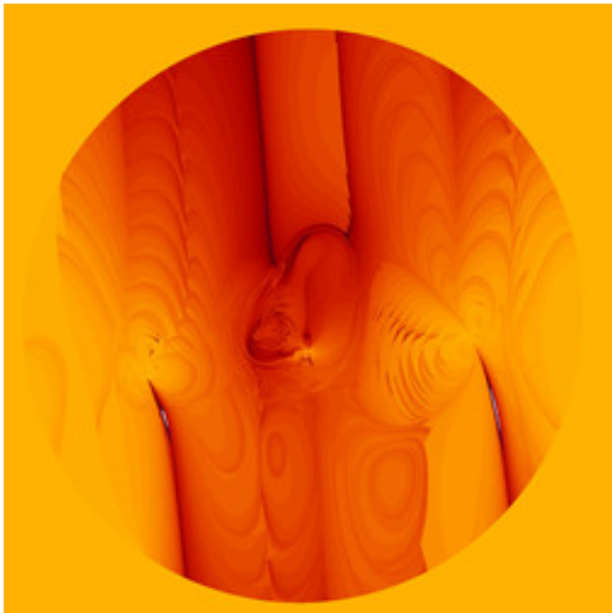
asz-andrextrandom-1-21.jpg
