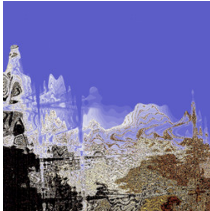
lkm3-FourierPopCorn-05B.jpg
