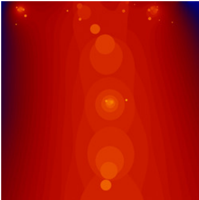
dmj-PhoenixDoubleNova-15.jpg
