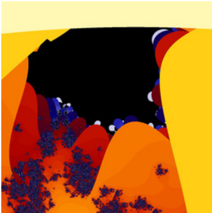
mt-990807aMset-20.jpg
