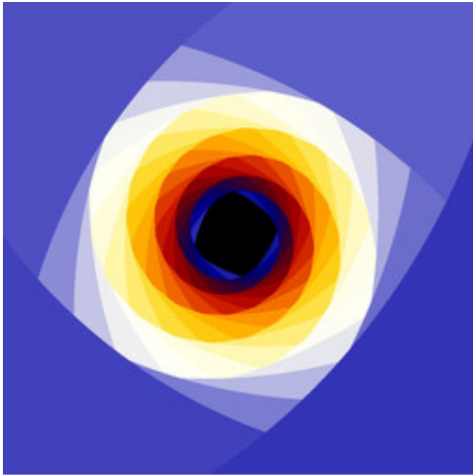
mt-barnsleyishJulia-12.jpg
