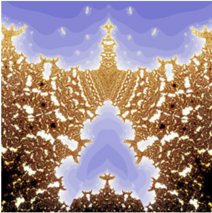
mt-990807aMset-13.jpg
