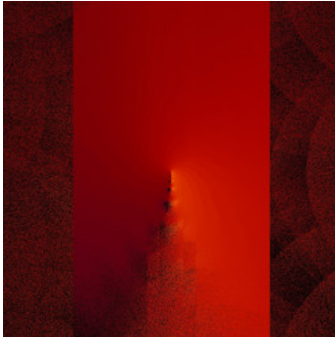
mt-newton-twist-10.jpg
