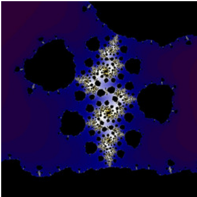
mt-990807aMset-04.jpg
