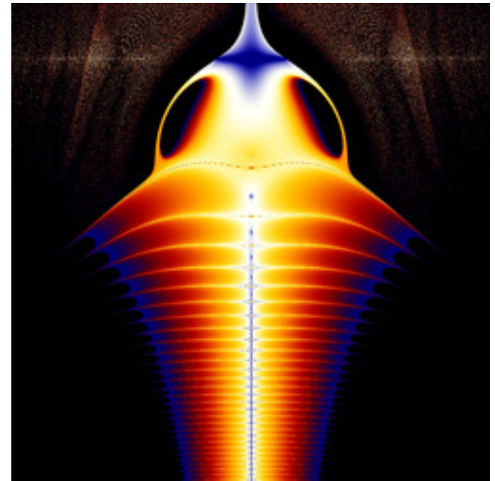
mt-zeepop-mset-14.jpg
