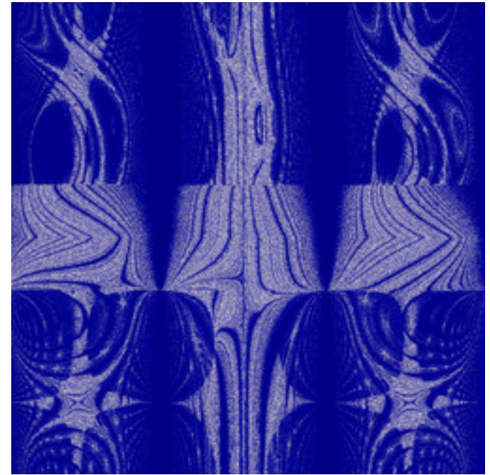
reb-GopalsamyFn-33.jpg
