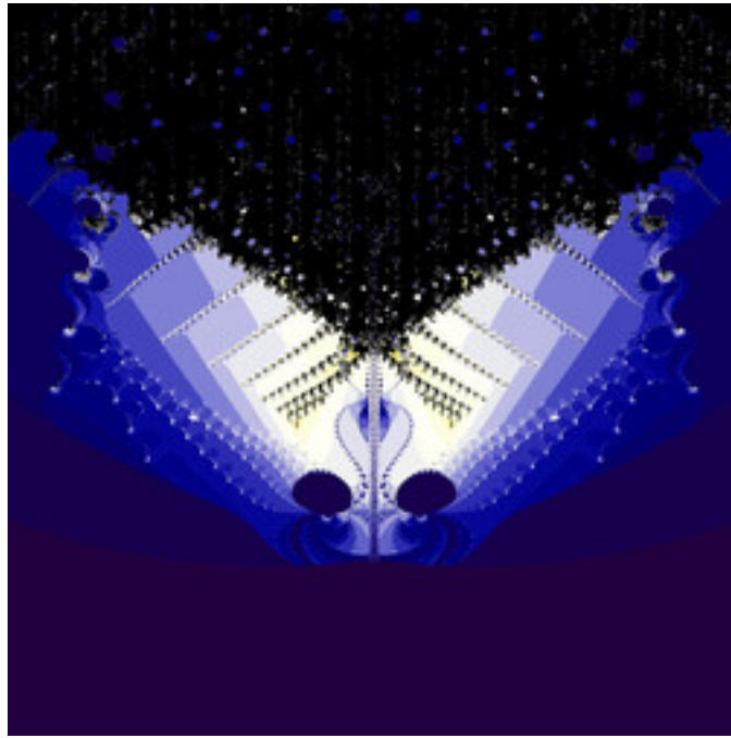
mt-rudys-cubic-mandelbrot-31.jpg
