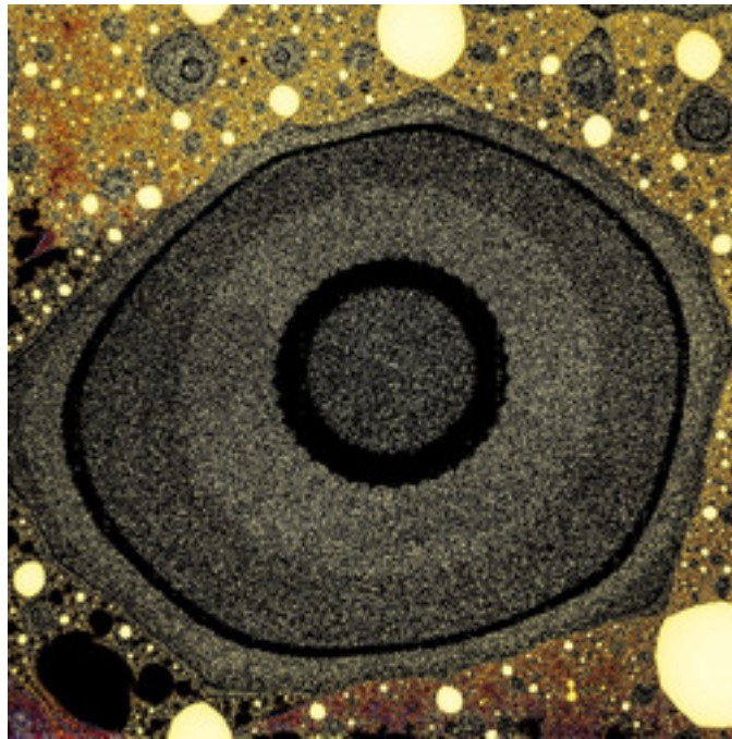
mt-magnetism-model-ii-05.jpg
