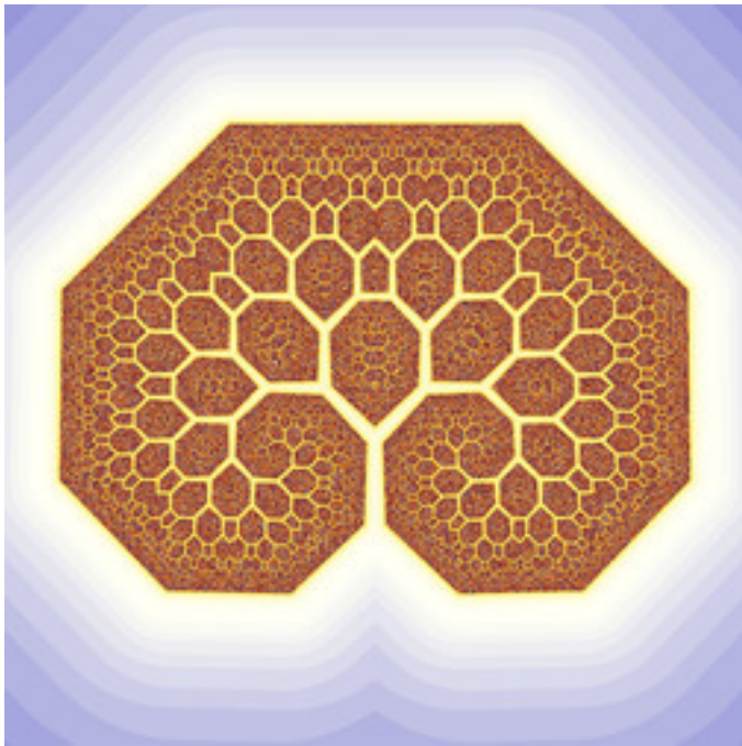
reb-IFSEscape1-02.jpg
