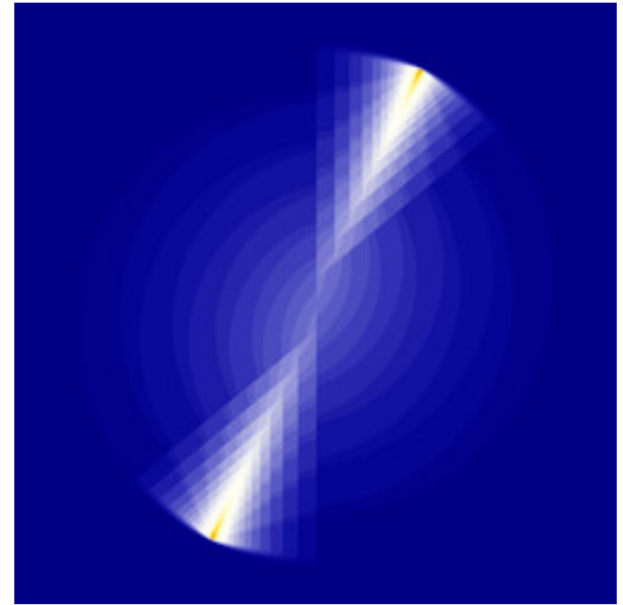
reb-FunBarnsley1Julia-06A.jpg
