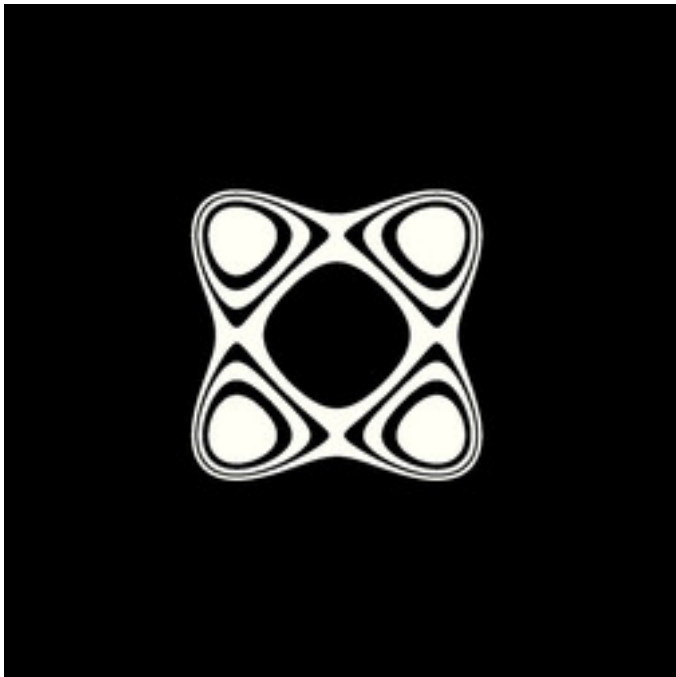
reb-FormulaTracer-01B.jpg
