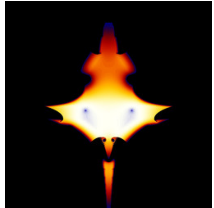
mt-zeepop-mset-43.jpg
