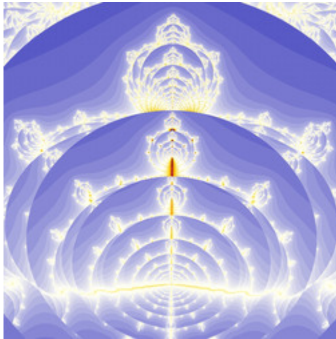
dmj-OrbitBoost-02.jpg
