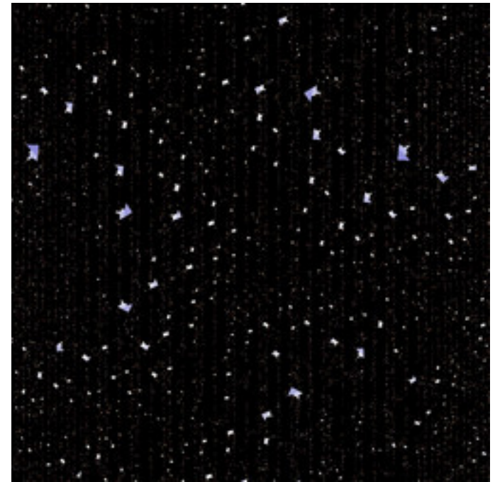
mt-barnsleyishJulia-07.jpg
