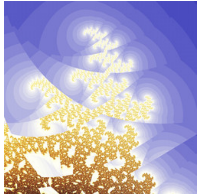
lkm-GeneralTentMandelbrot-02.jpg
