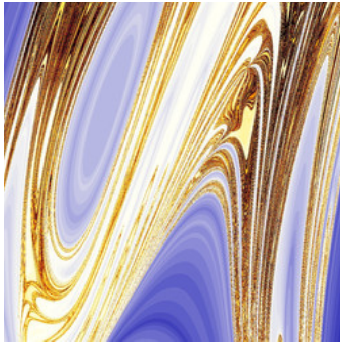
mt-990625bMset-02.jpg
