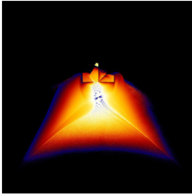
mt-zeepop-mset-06.jpg
