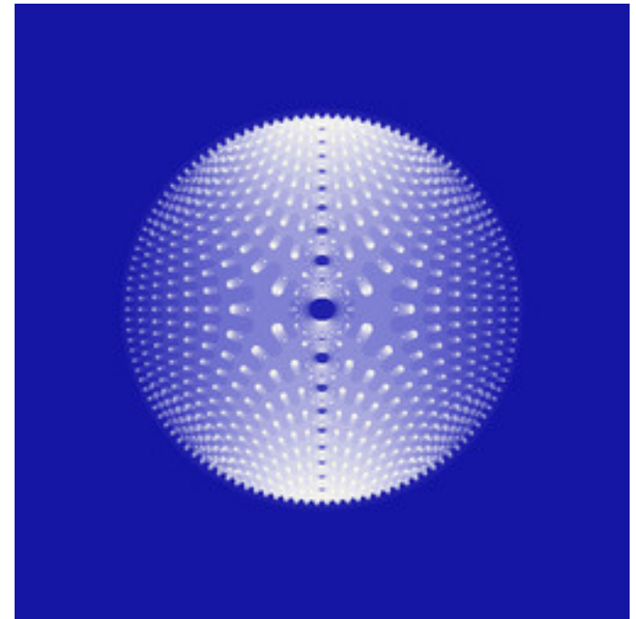
mt-pseudo-magnet-julia-05.jpg
