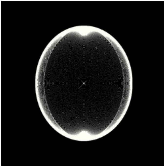
reb-FormulaTracer-09B.jpg
