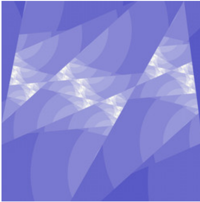
lkm-GeneralTentJulia-02.jpg
