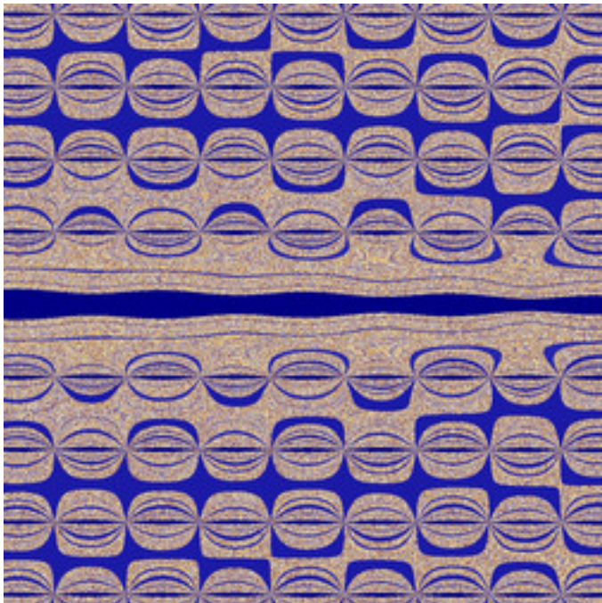
reb-GopalsamyFn-20.jpg
