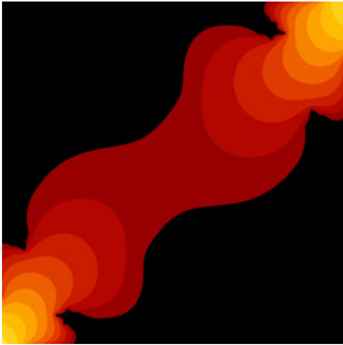
lkm-CompundingTM-05.jpg
