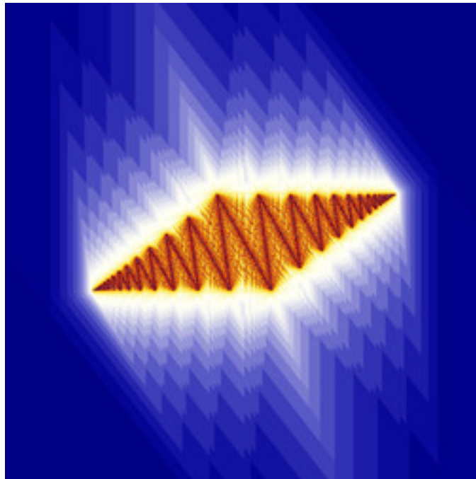
reb-FunBarnsley1Julia-05B.jpg
