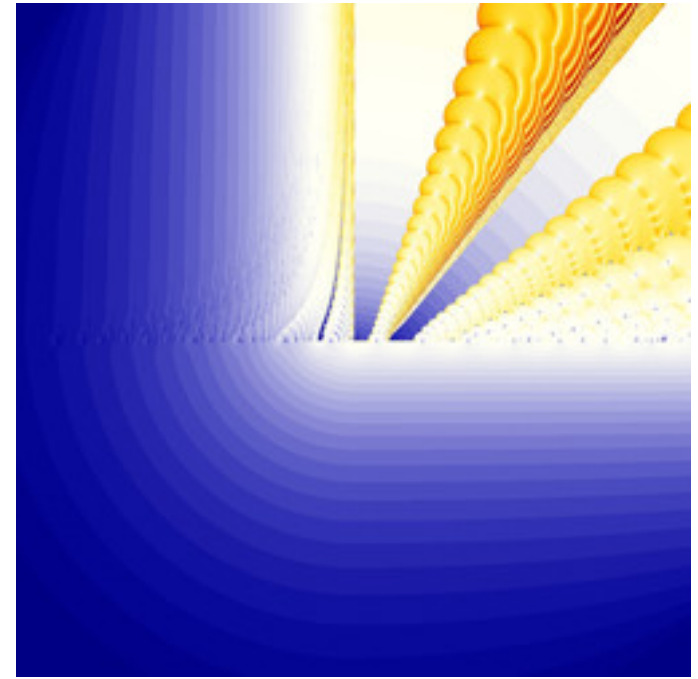
mt-zeepop-julia-11.jpg
