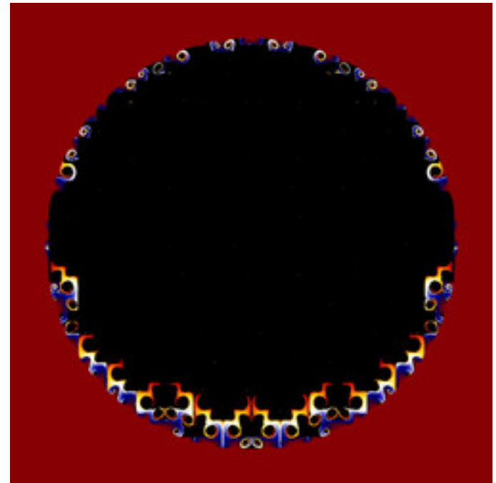
lkm3-FourierPopCorn-04D.jpg
