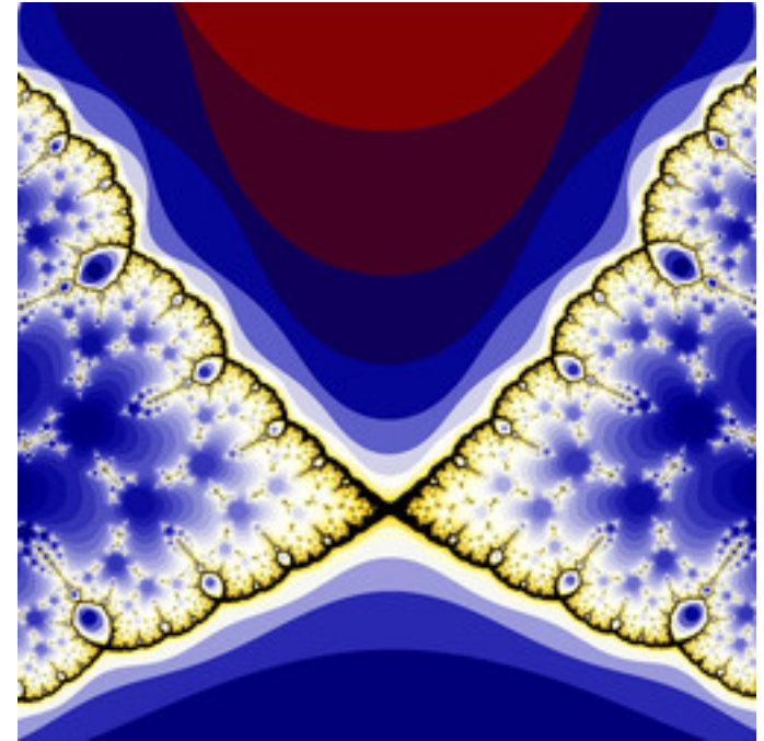
lkm3-AlternativeFunctions-08.jpg
