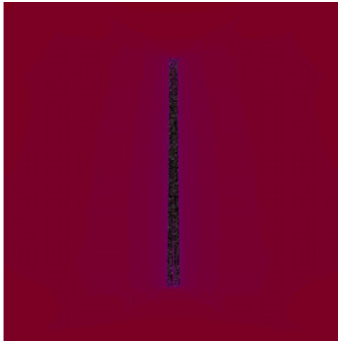
mt-GeneralizedCelticJulia-05.jpg
