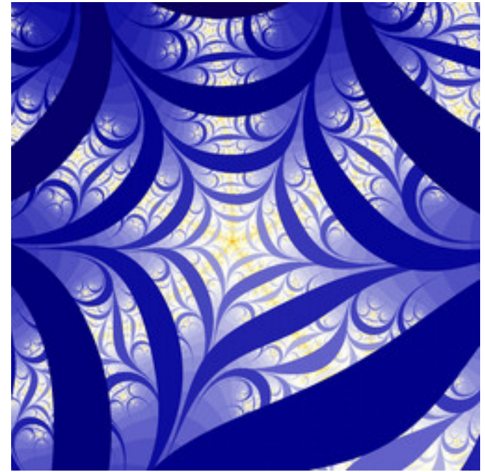
lkm-GapMandelbrot-02B.jpg
