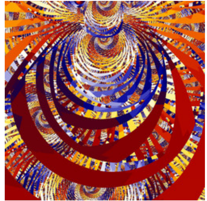
reb-JuliaTentMap-20.jpg
