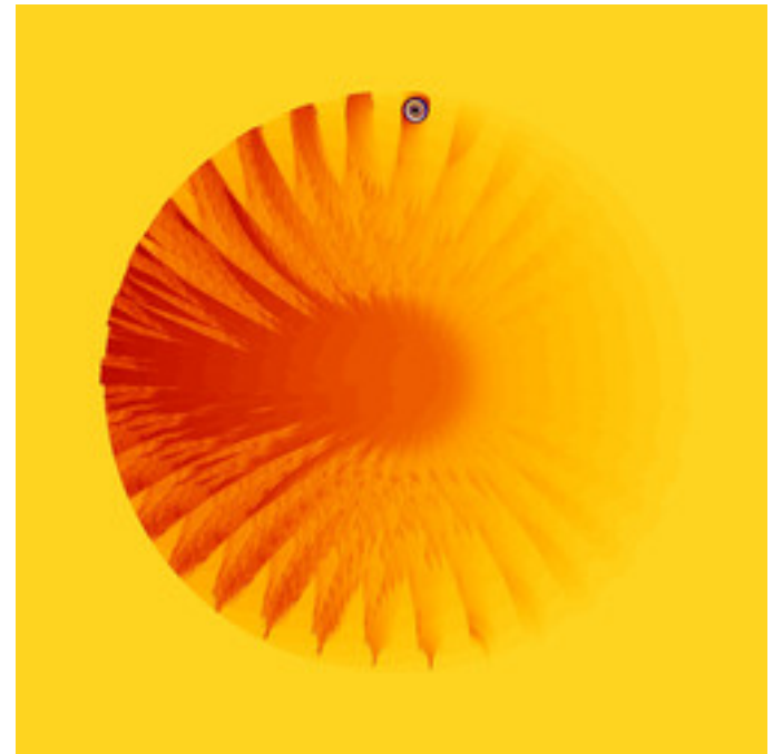
reb-PseudoZeePi-04.jpg
