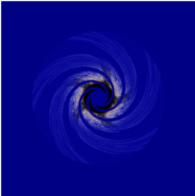
ahm-IndependantPower_08.jpg
