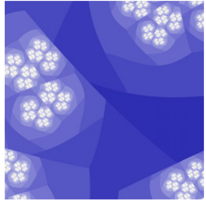
mt-barnsleyishJulia-04.jpg
