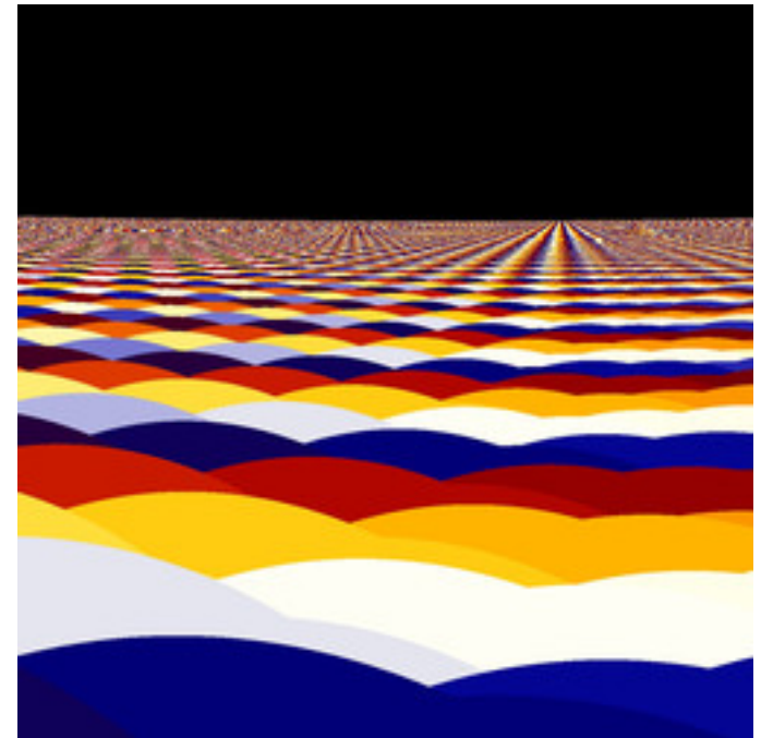
mt-rudys-cubic-mandelbrot-33.jpg
