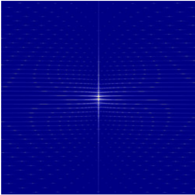
reb-GopalsamyFn-07.jpg
