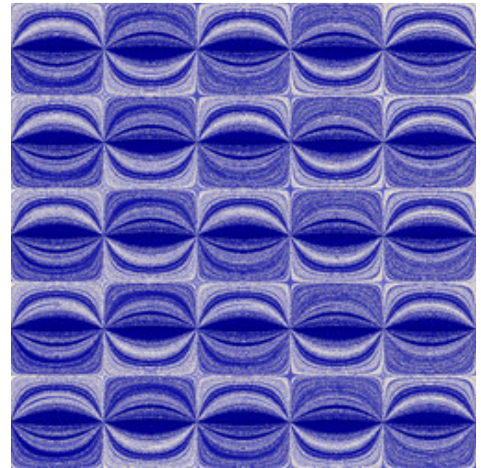
reb-GopalsamyFn-24.jpg
