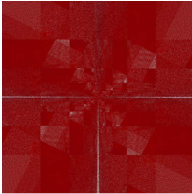
dmj-NovaMandel-103.jpg
