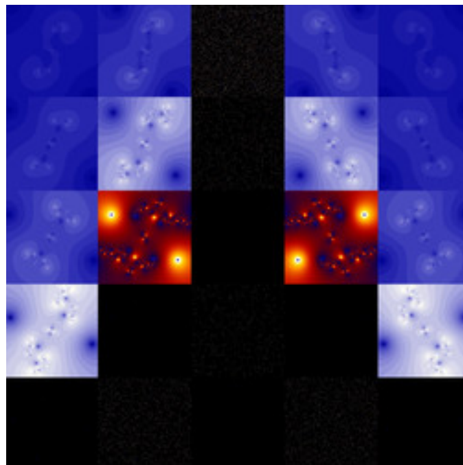
dmj-ManyNova-05.jpg
