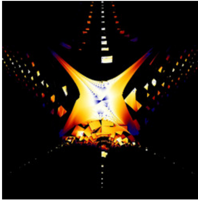
mt-zeepop-mset-18.jpg
