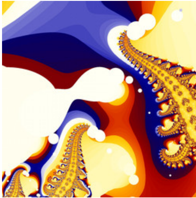
dmj-PhoenixDoubleNova-11.jpg
