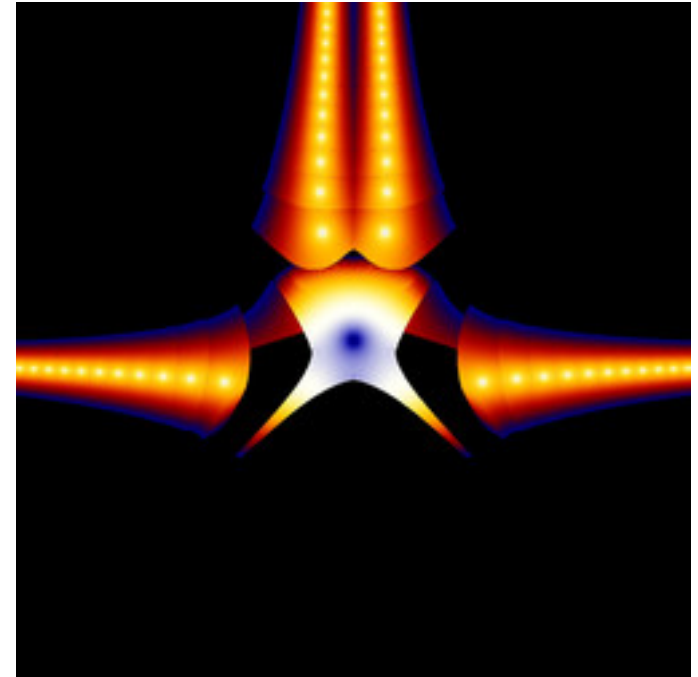
mt-zeepop-mset-08.jpg
