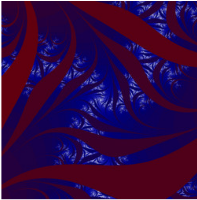
lkm-GapMandelbrot-03.jpg
