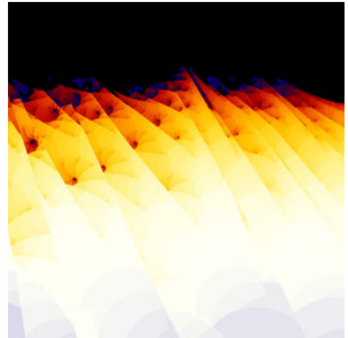
mt-barnsleyishMest-10.jpg
