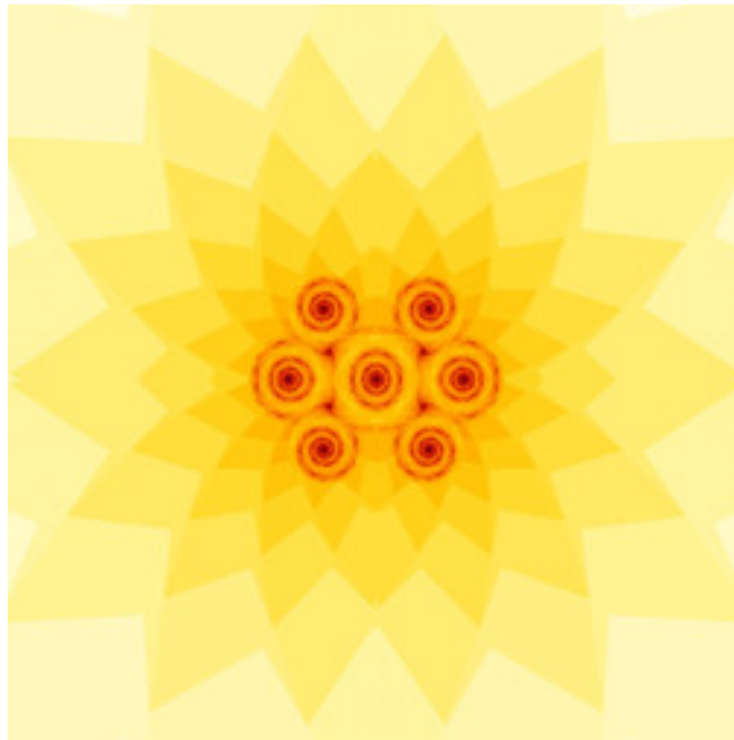
reb-JuliaTentMap-03.jpg
