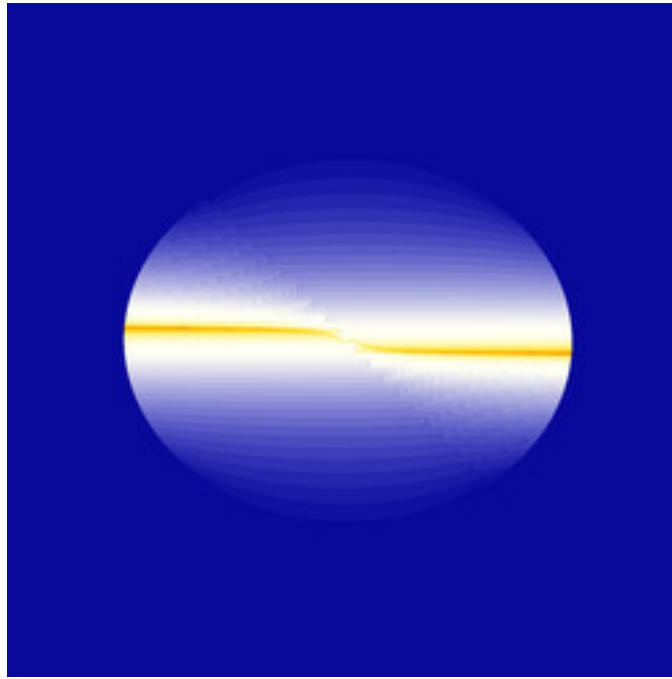
mt-zeepop-julia-18.jpg
