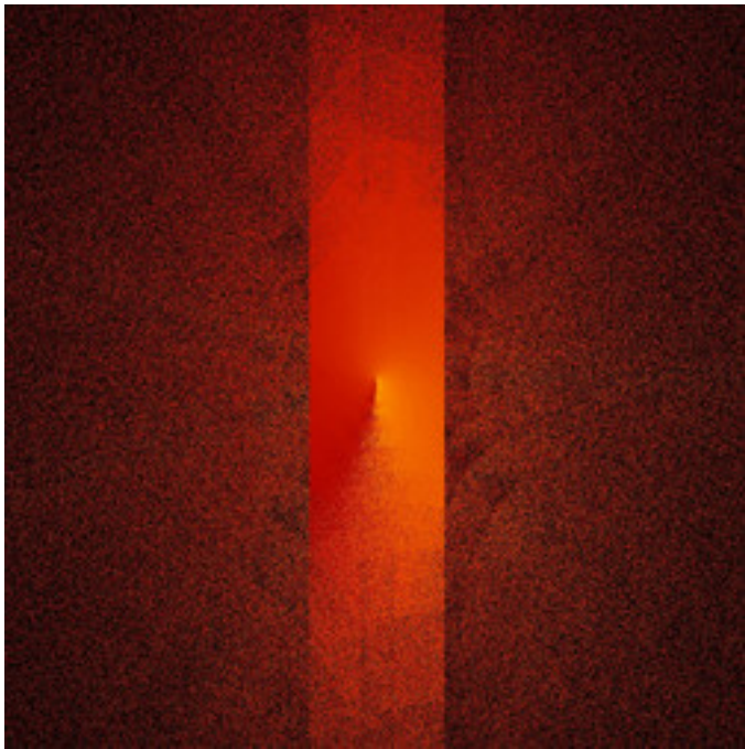
mt-newton-twist-08.jpg
