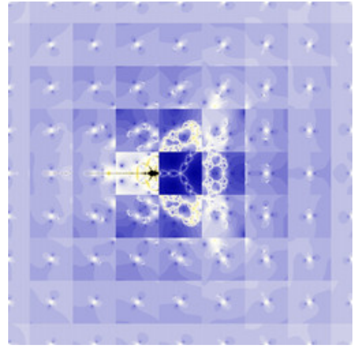
dmj-ManyNova-01.jpg
