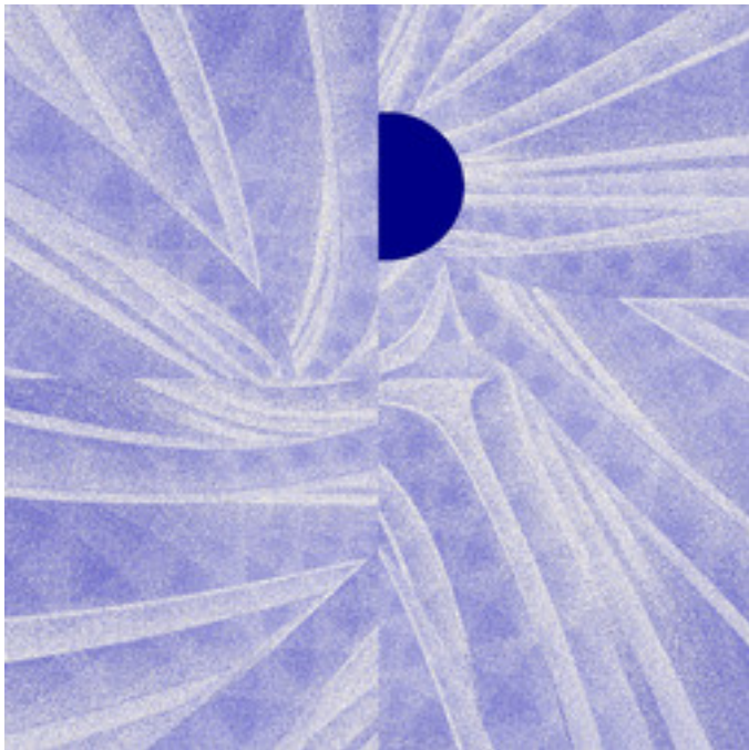
ahm-MonotonicGrowthJulia_05.jpg
