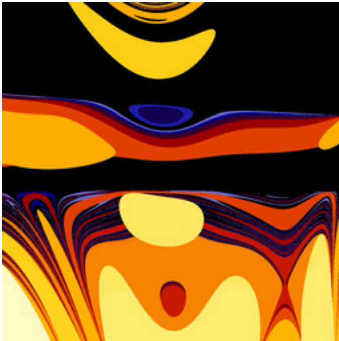
mt-990807aMset-32.jpg
