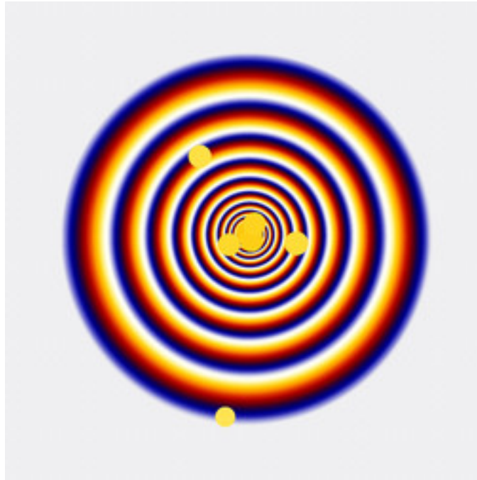
dmj-PhoenixDoubleNova-40.jpg
