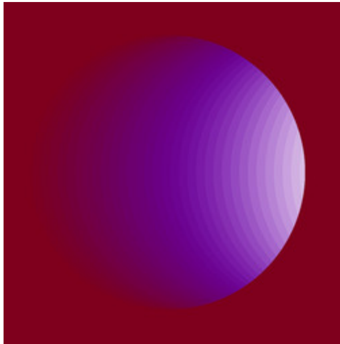
mt-GeneralizedCelticJulia-11.jpg
