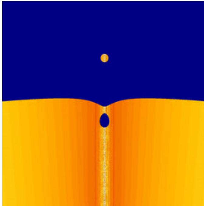
mt-zeepop-julia-15.jpg
