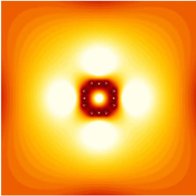
mt-rudys-cubic-mandelbrot-08.jpg
