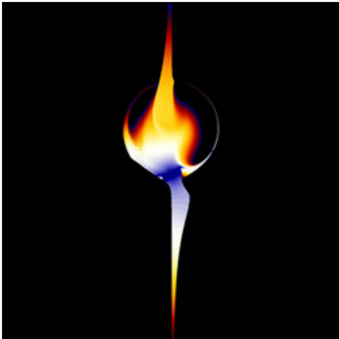
mt-zeepop-mset-40.jpg
