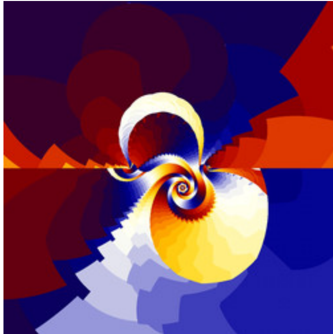
reb-JuliaTentMap-18.jpg
