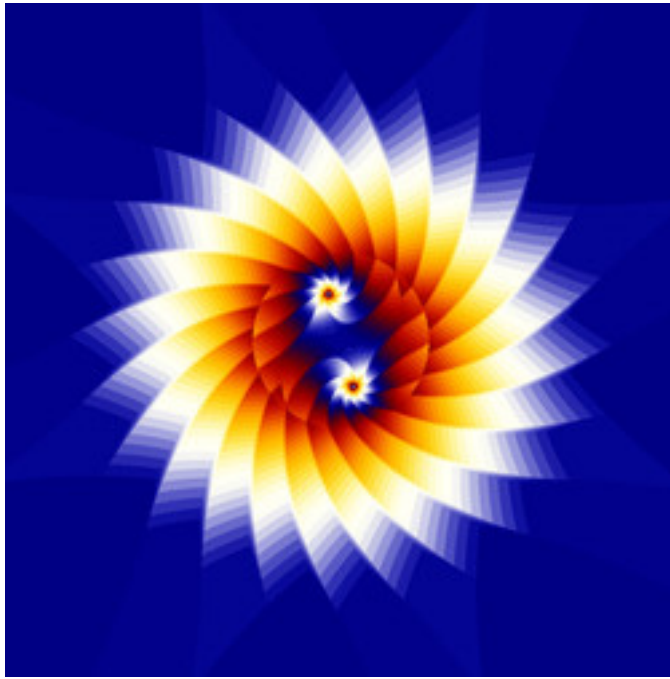
reb-JuliaTentMap-22.jpg
