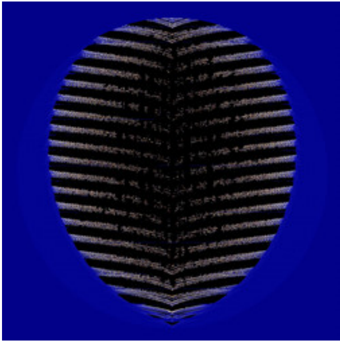
mt-bifunctionalMset-07.jpg
