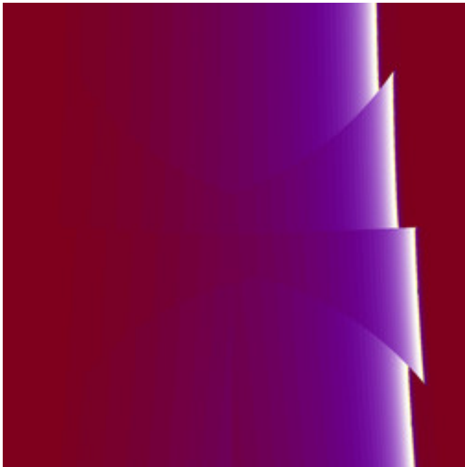
mt-GeneralizedCelticJulia-54.jpg
