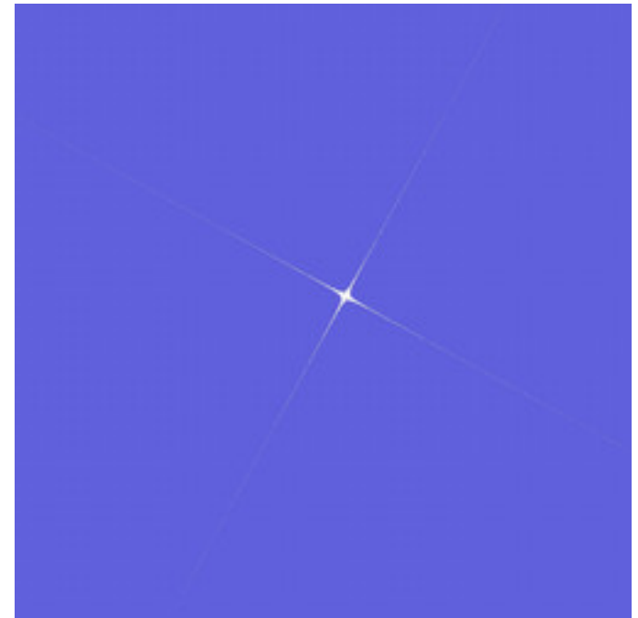
ldm-DM0-01.jpg
