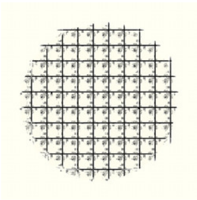
lkm3-FourierPopCorn-08.jpg
