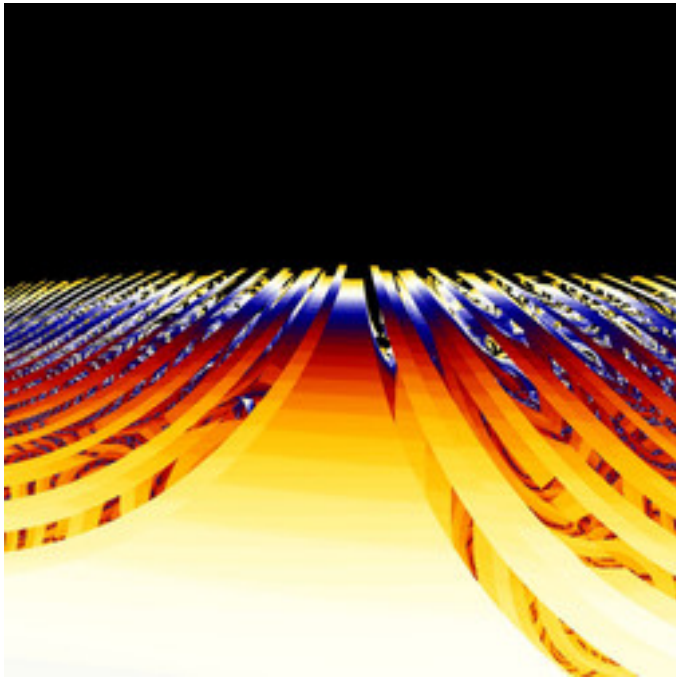
lkm-GeneralTentMandelbrot-NEW1-01.jpg
