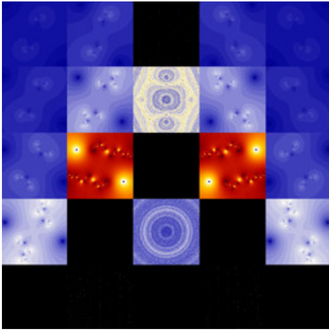
dmj-ManyNova-03.jpg
