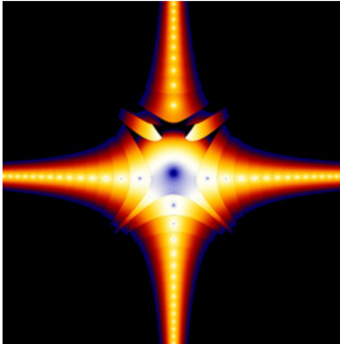
mt-zeepop-mset-09.jpg
