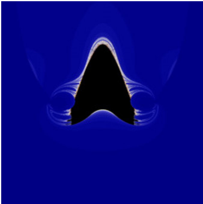
reb-Mask-02.jpg
