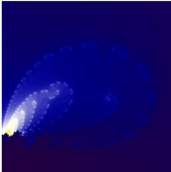
lkm-CompundingTM-01.jpg
