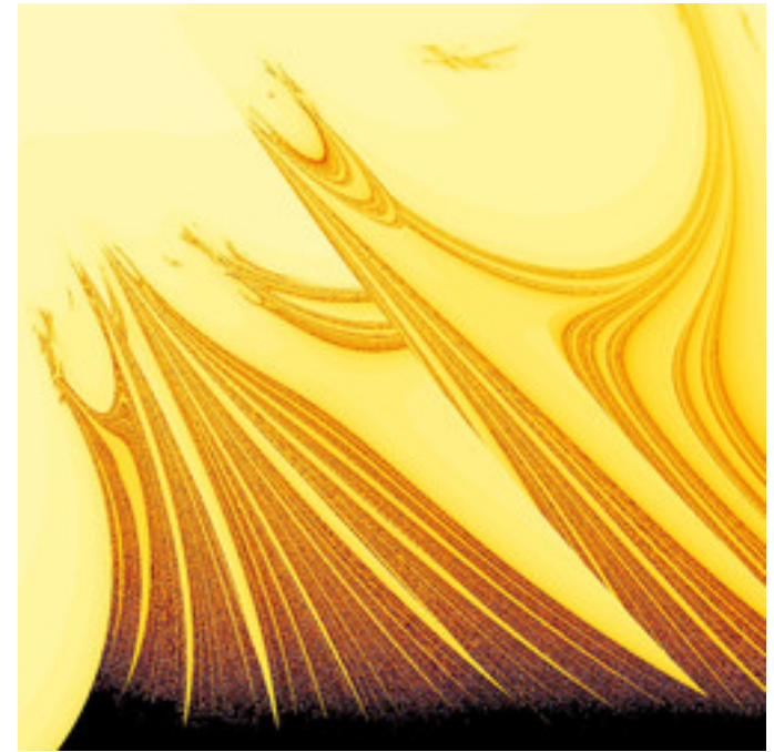
mt-990807aMset-45.jpg
