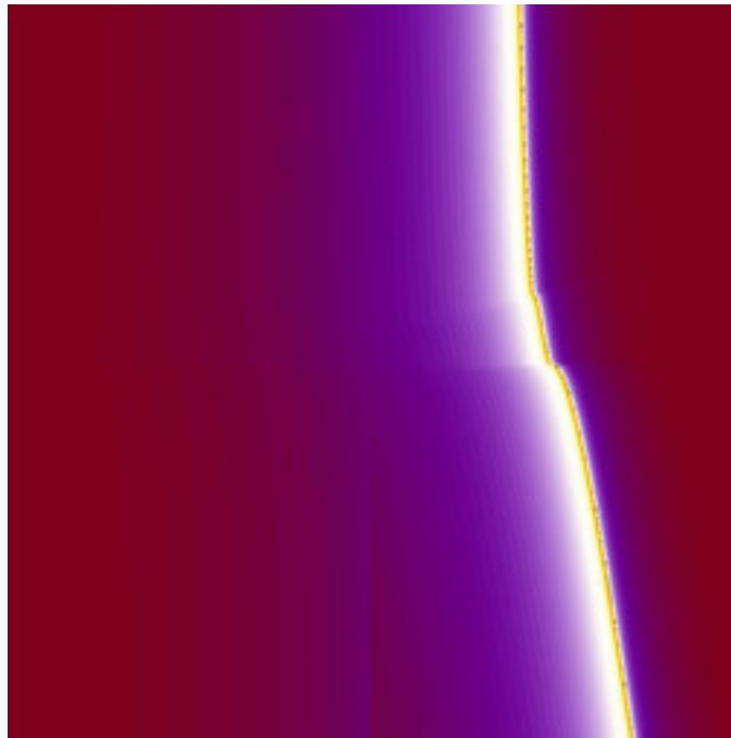
mt-GeneralizedCelticJulia-53.jpg
