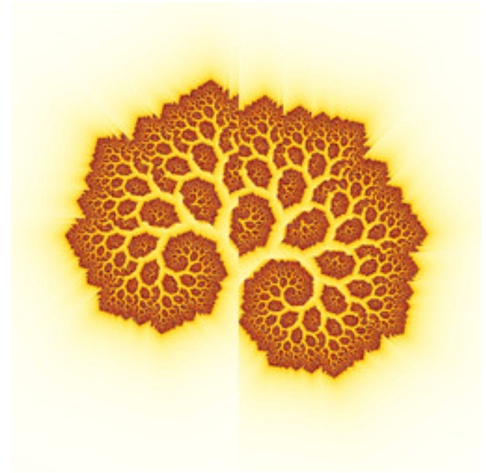
reb-IFSEscape1-03.jpg
