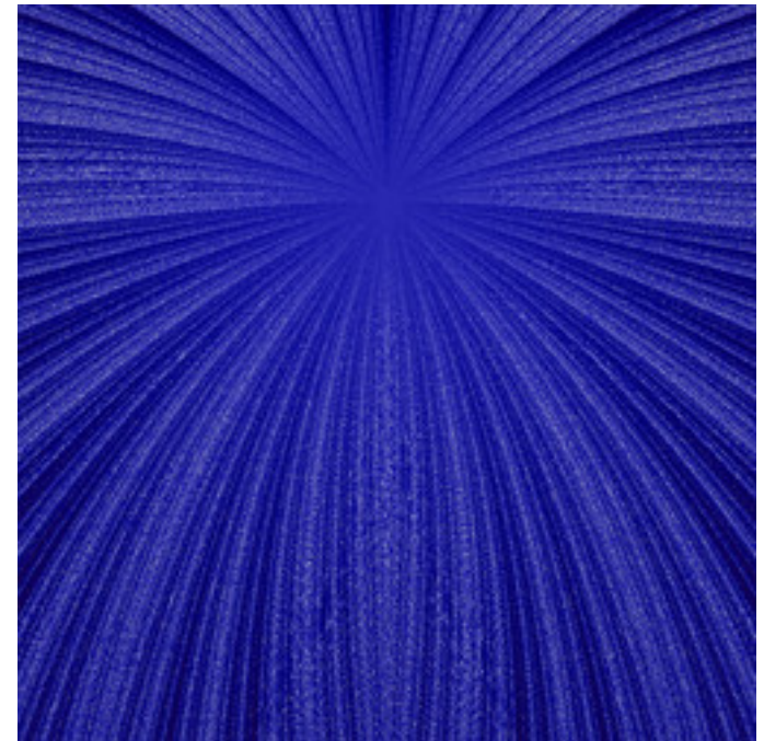
lkm3-UnitVectorTweakMandelbrot-02.jpg
