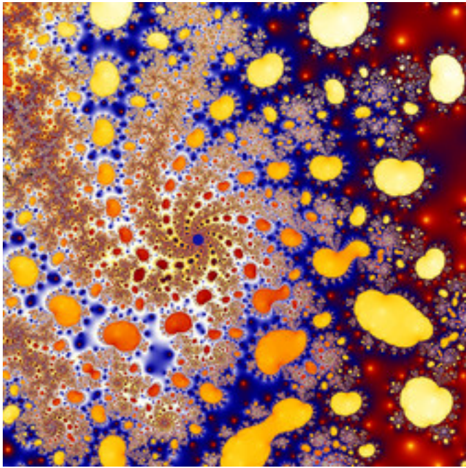
dmj-DoubleNova-06.jpg
