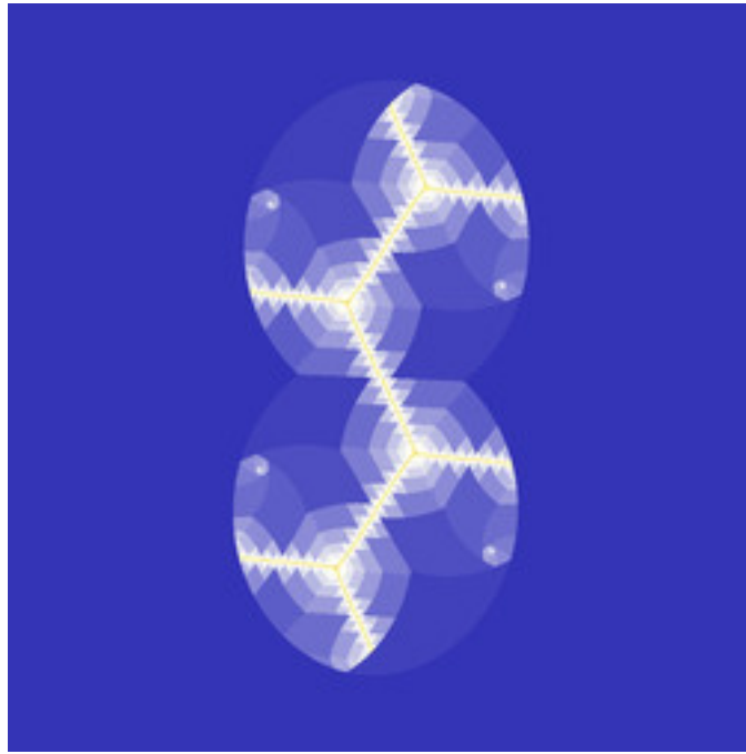
mt-barnsleyishJulia-11.jpg
