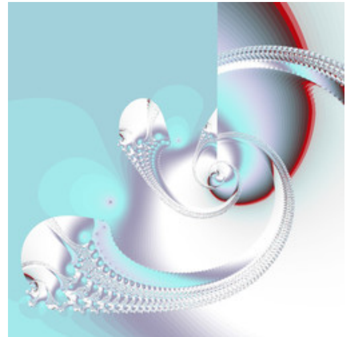
dmj-NovaMandel-05.jpg
