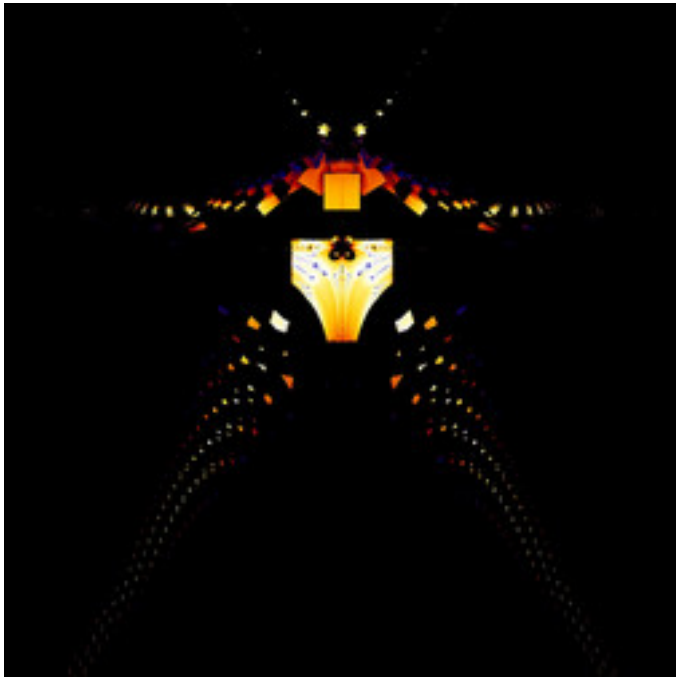
mt-zeepop-mset-48.jpg
