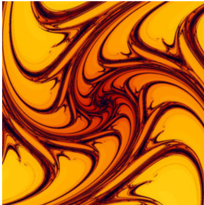
mt-990807aMset-43.jpg
