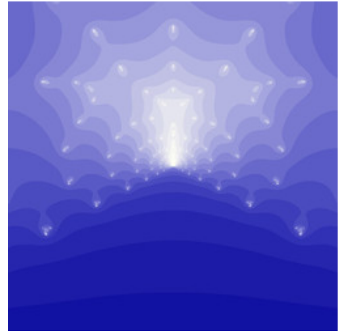
reb-JonHomerSpider-03.jpg
