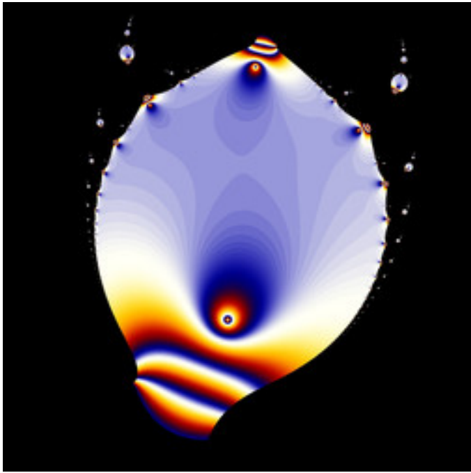
mt-newton-error-17a.jpg
