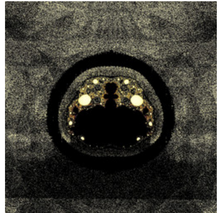
mt-magnetism-model-ii-04.jpg
