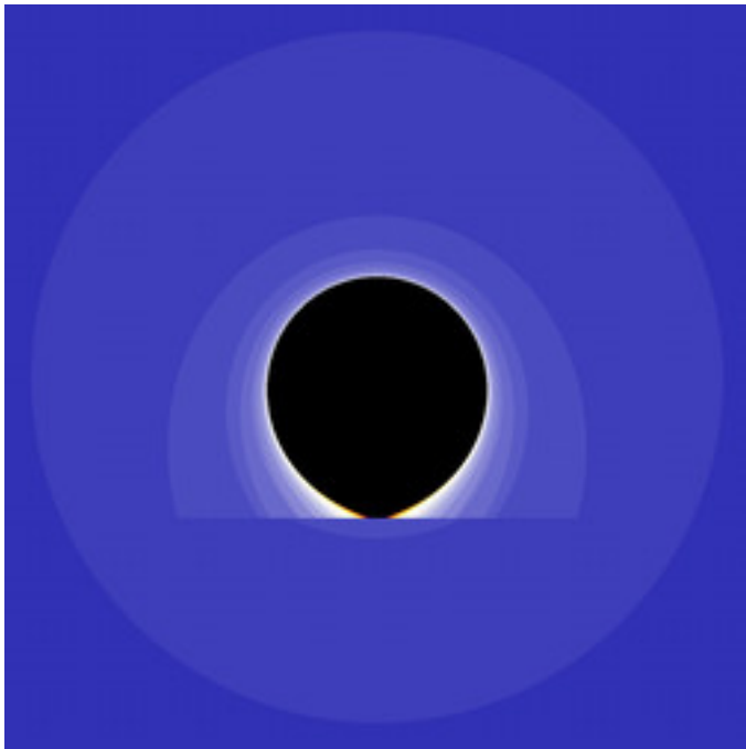
mt-barnsleyishMest-12.jpg
