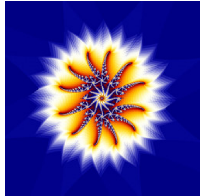
reb-JuliaTentMap-27.jpg
