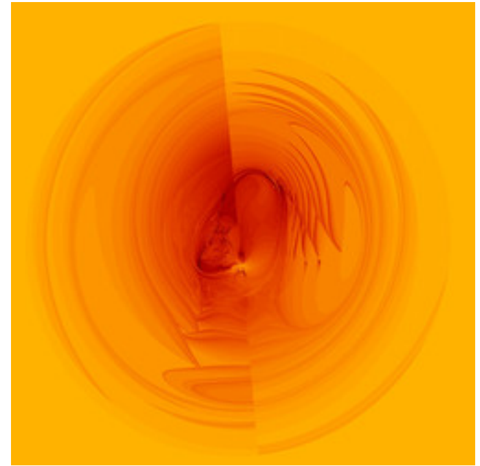
asz-andrextrandom-1-22.jpg
