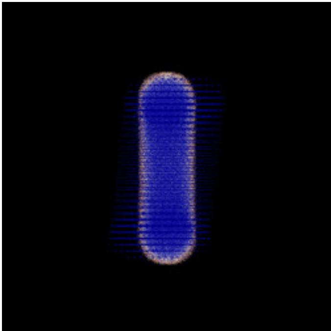
mt-latoocarfian-ii-37.jpg
