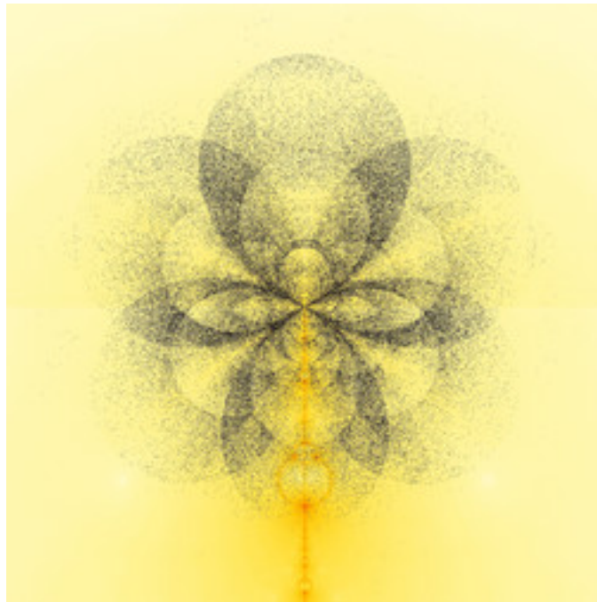
mt-newton-error-23a.jpg
