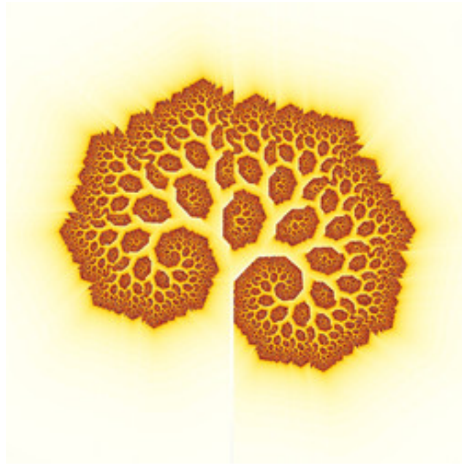
reb-IFSEscape1-04.jpg
