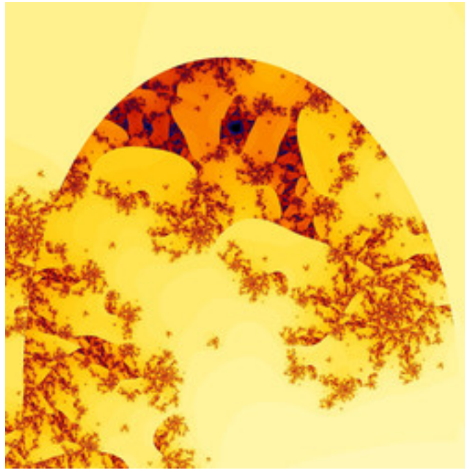
mt-990807aMset-22.jpg
