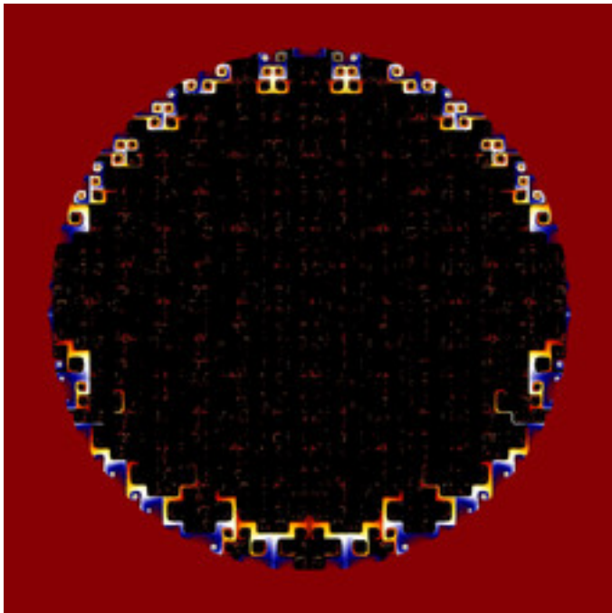
lkm3-FourierPopCorn-04F.jpg
