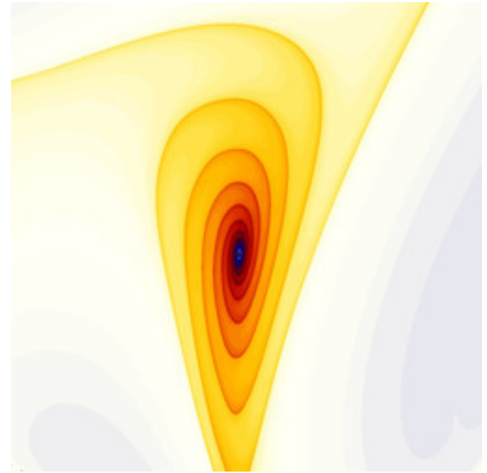
mt-990807aMset-39.jpg
