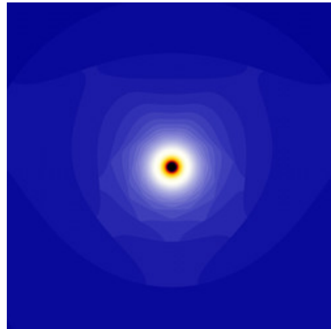
mt-990725a-03.jpg
