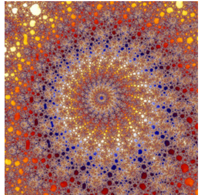
dmj-DoubleNova-07.jpg
