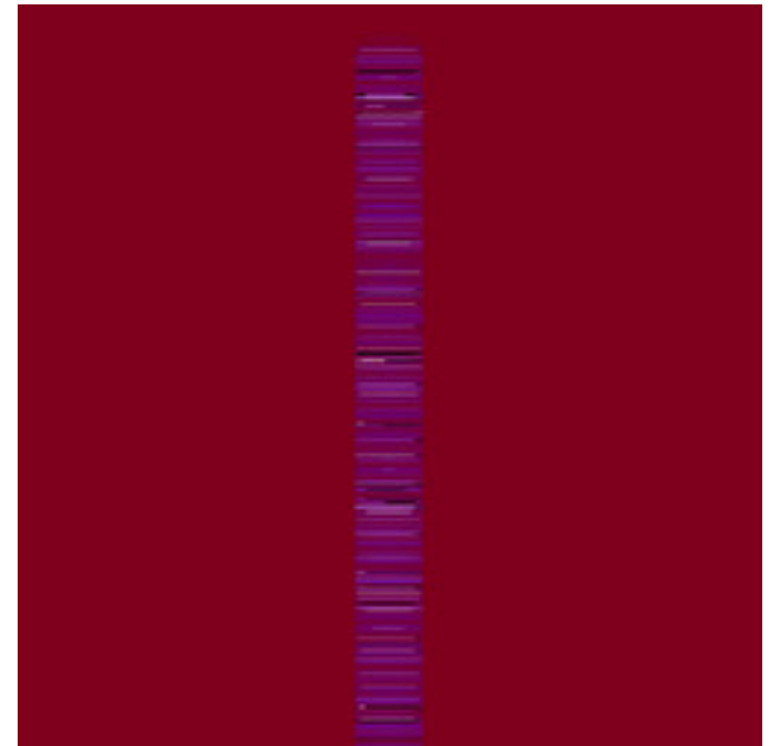
mt-GeneralizedCelticJulia-31.jpg
