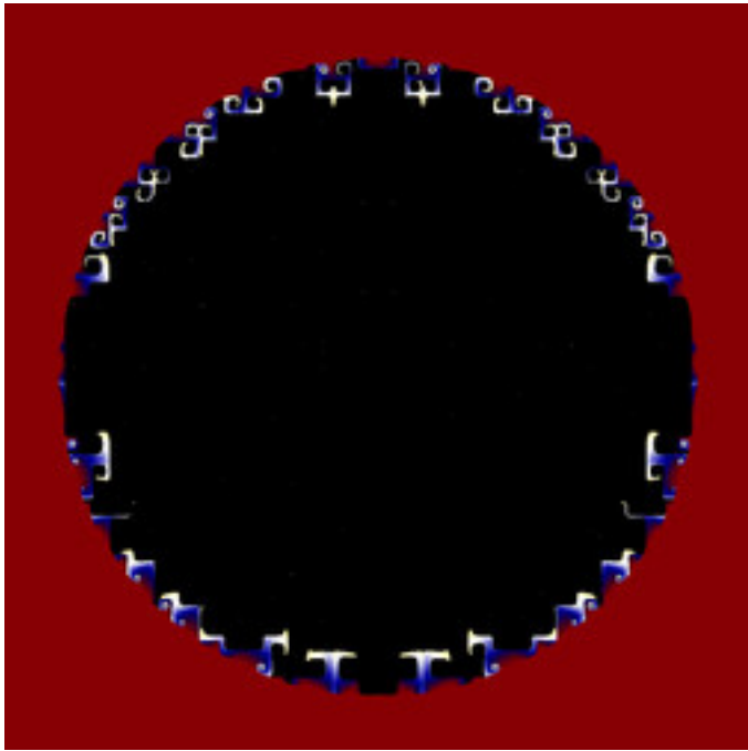
lkm3-FourierPopCorn-04I.jpg
