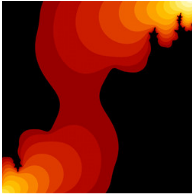
lkm-CompundingTM-04.jpg
