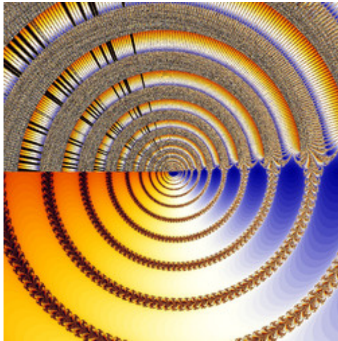
ads-Newton_03.jpg
