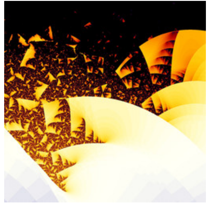
lkm-GeneralTentMandelbrot-05.jpg
