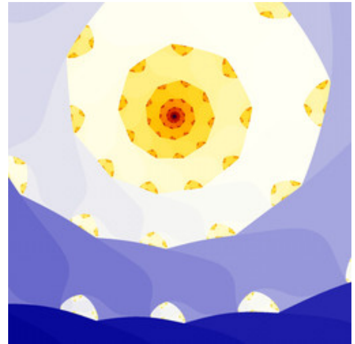
ldm-DM4-02.jpg
