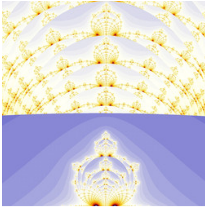
dmj-OrbitBoost-05.jpg
