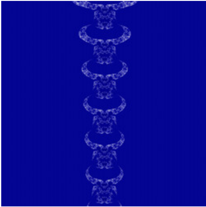
ldm-DM23-07.jpg
