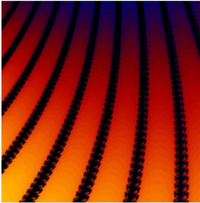
lkm-EmbossedNewton-04.jpg
