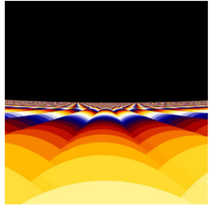
mt-rudys-cubic-mandelbrot-36.jpg
