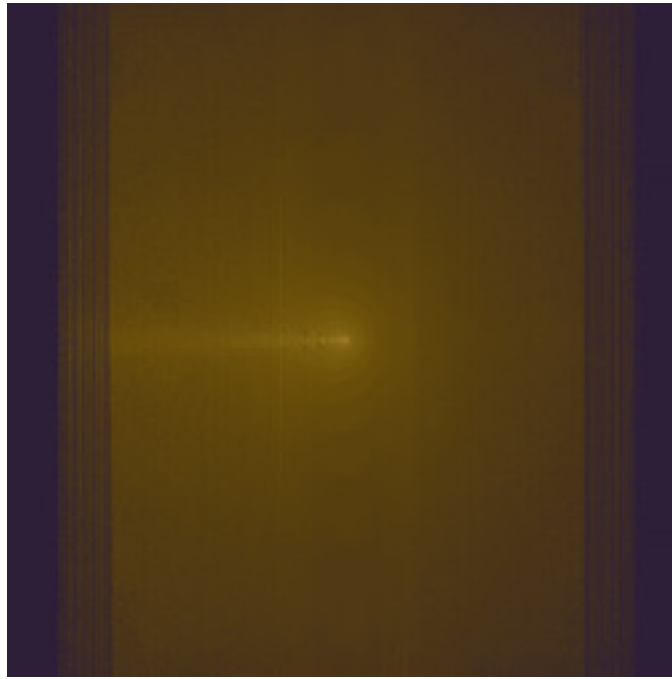
mt-newton-error-julia-04.jpg
