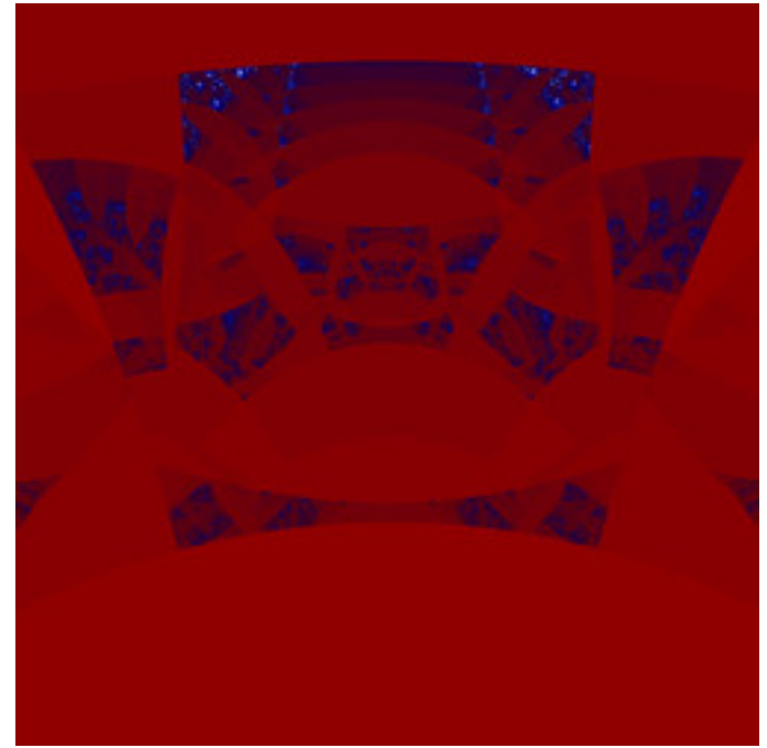
mt-990807bMset-11.jpg
