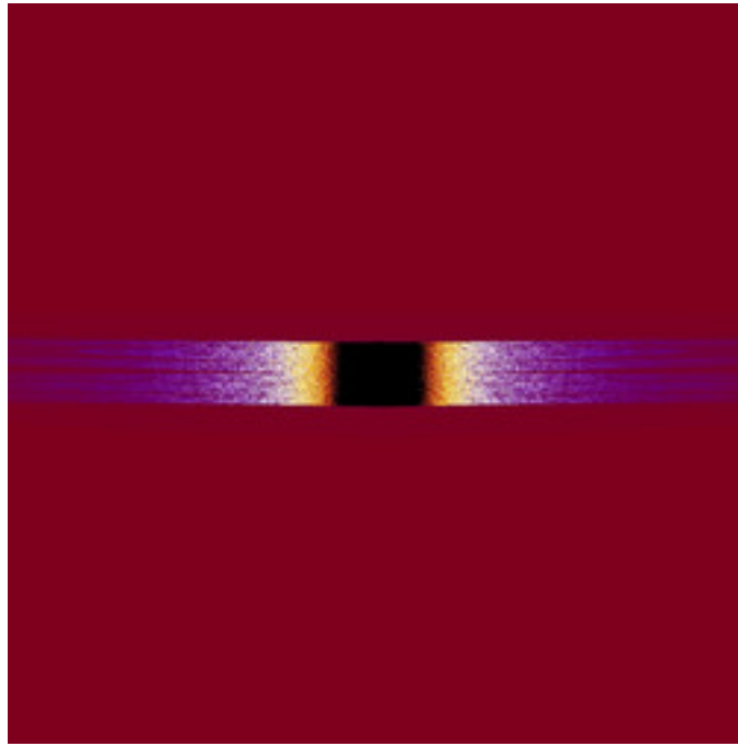
mt-GeneralizedCelticJulia-50.jpg
