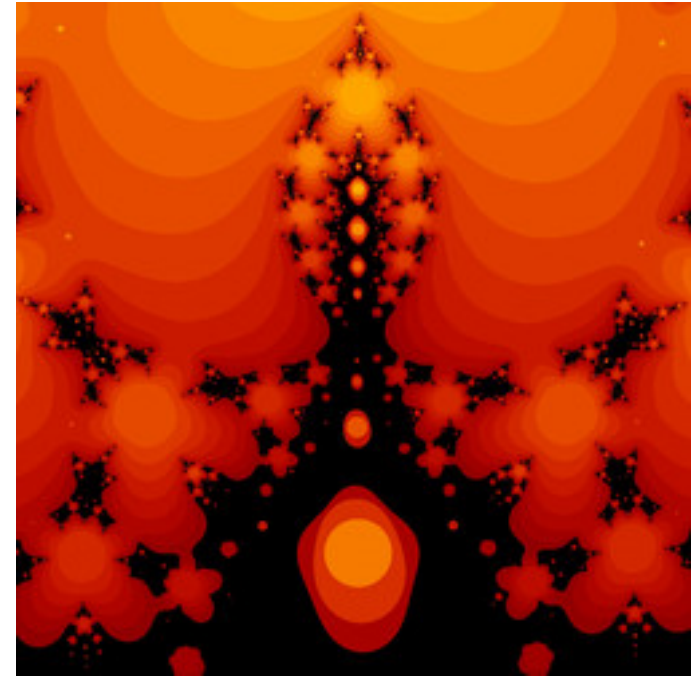
lkm3-AlternativeFunctions-11.jpg
