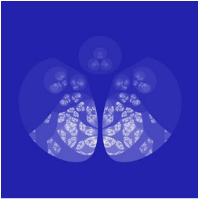
mt-rudys-cubic-mandelbrot-20.jpg
