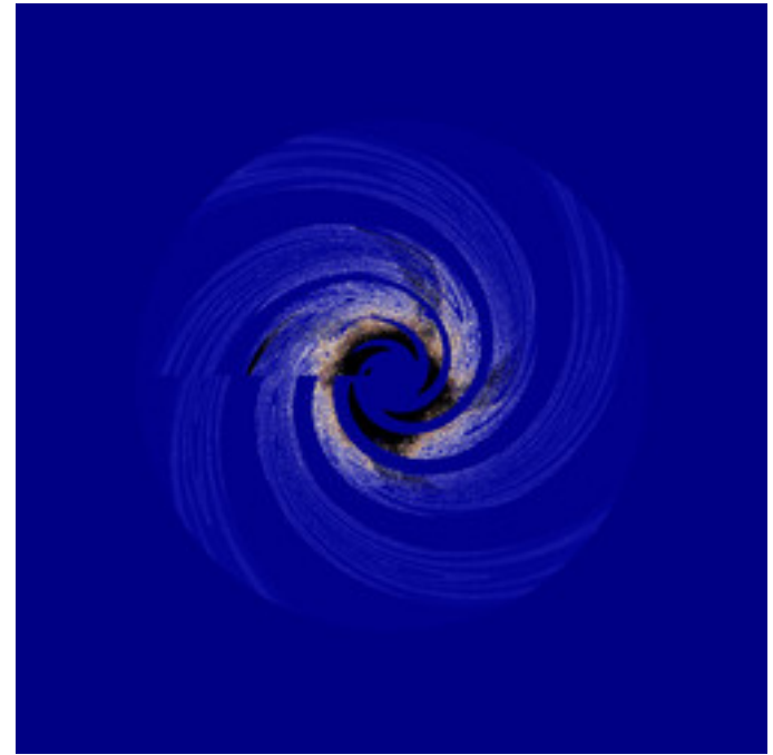
ahm-IndependantPower_09.jpg
