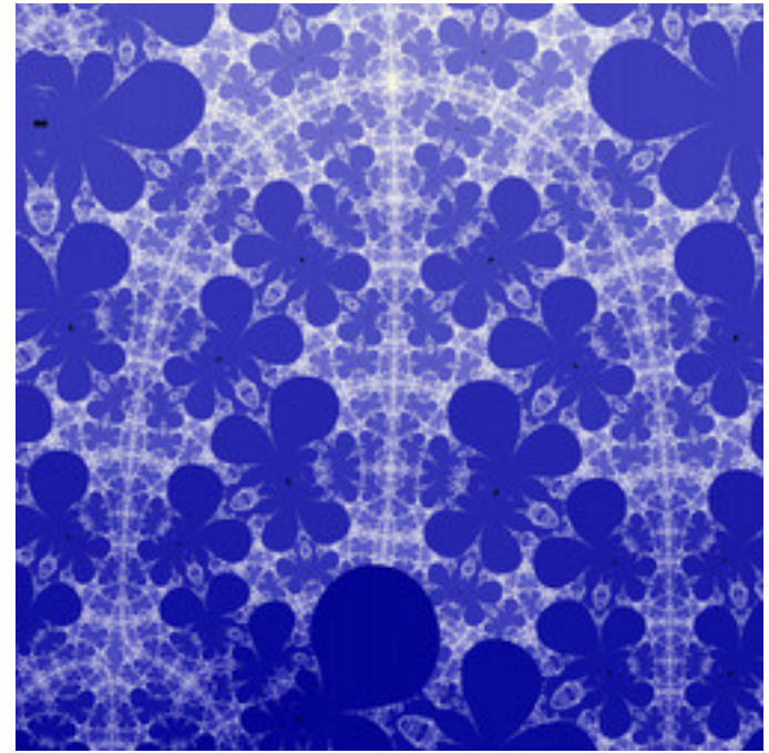
ldm-DM23-05.jpg
