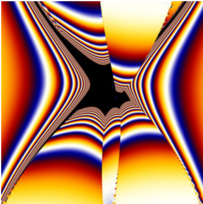
mt-newton-9904a-04.jpg
