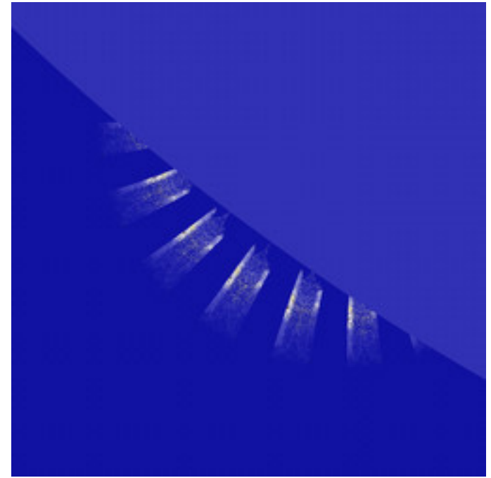
ldm-DM3-01.jpg
