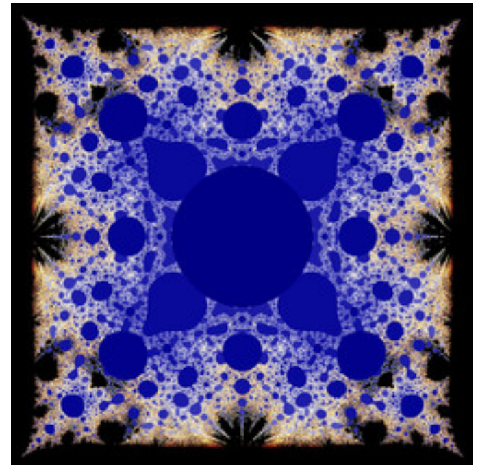
mt-rudys-cubic-mandelbrot-04.jpg
