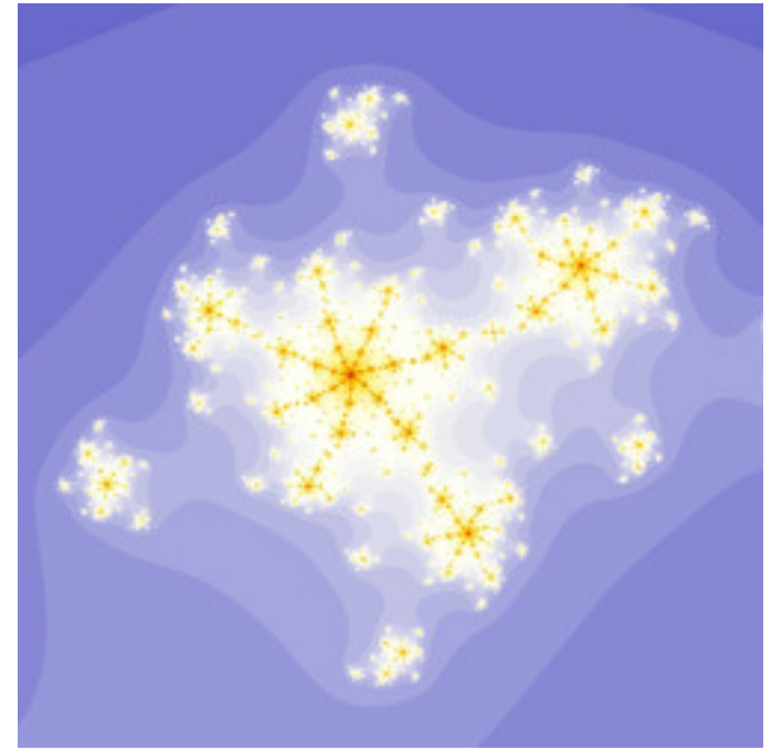
mt-990807aMset-11.jpg
