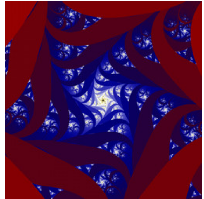
lkm-GapMandelbrot-01.jpg
