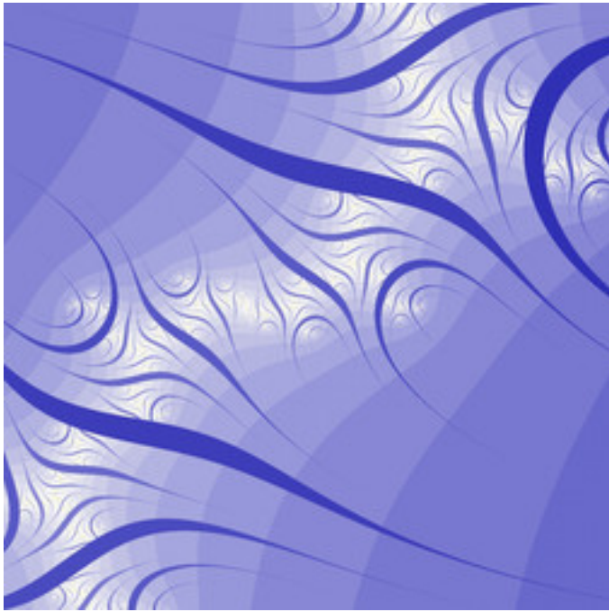
lkm-GapJulia-01.jpg
