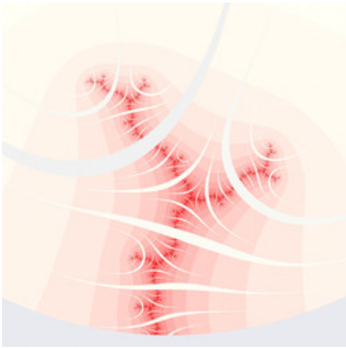
lkm-GapMandelbrot-10.jpg
