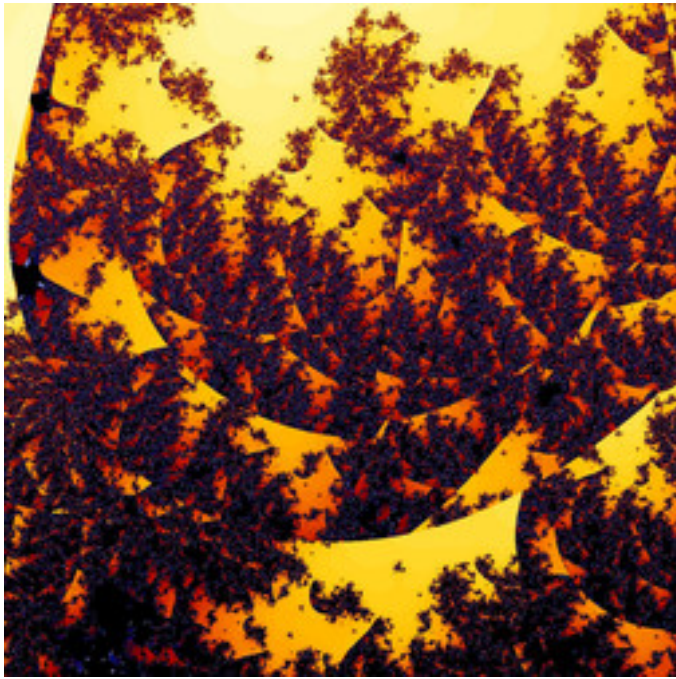
mt-990807aMset-17.jpg
