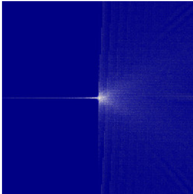
reb-GopalsamyFn-08B.jpg
