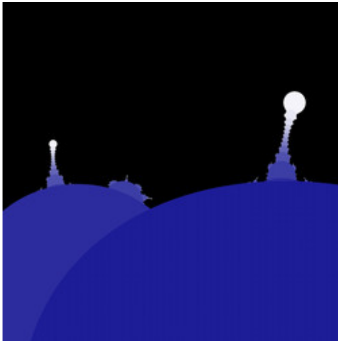
ldm-DM0-02.jpg
