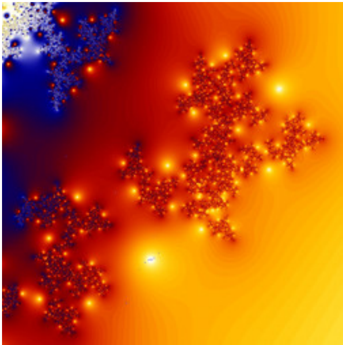
dmj-PhoenixDoubleNova-03.jpg
