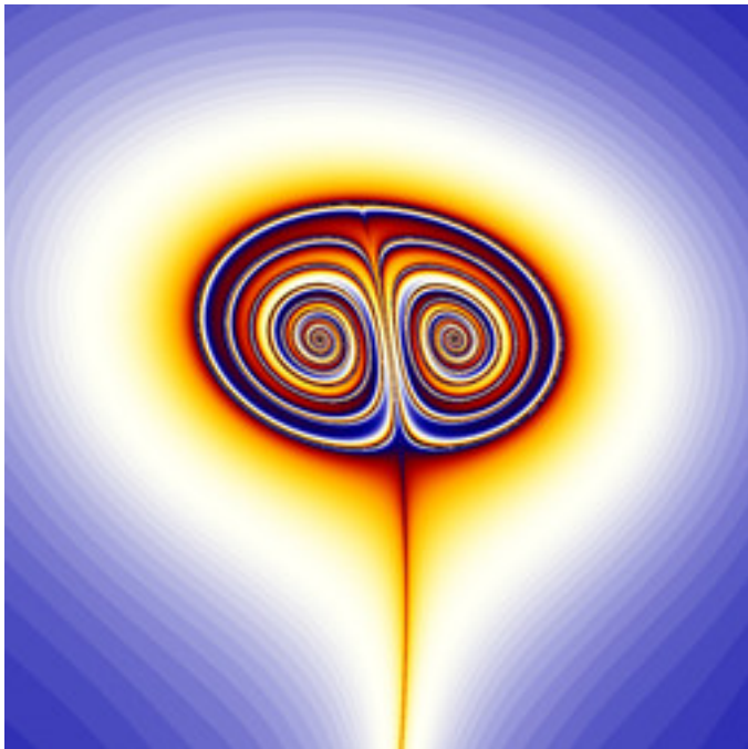
mt-Fractalia1-02.jpg
