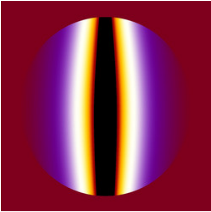
mt-GeneralizedCelticJulia-51.jpg
