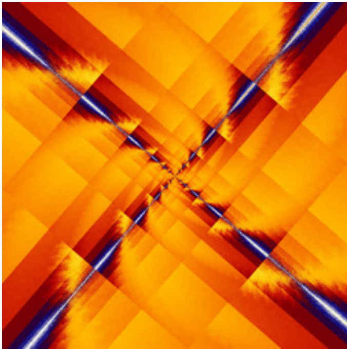
dmj-NovaMandel-101.jpg
