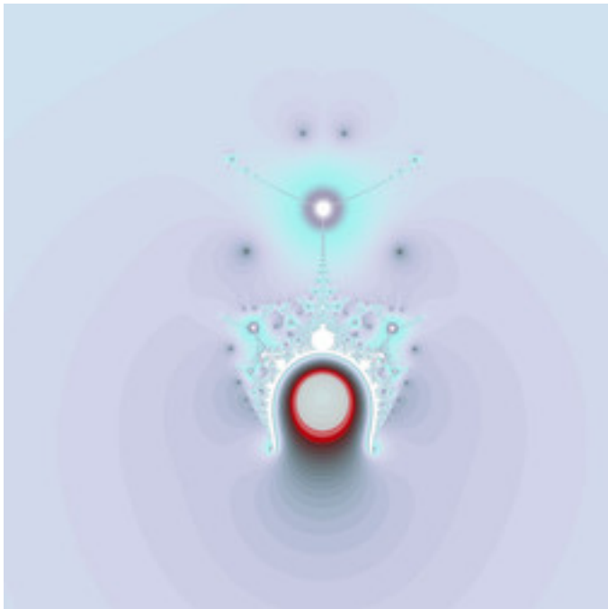
dmj-NovaMandel-07.jpg
