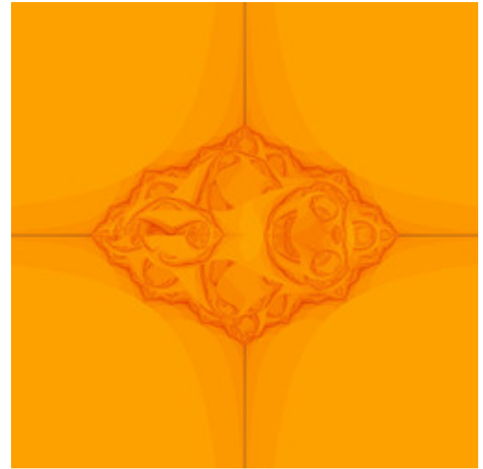
reb-JuliaCrossOrbitLambda-04.jpg
