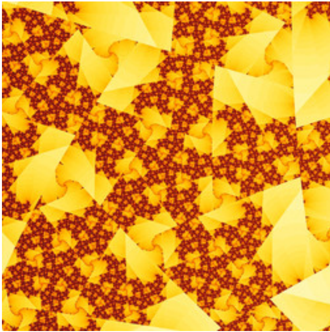
lkm-GeneralTentMandelbrot-07.jpg
