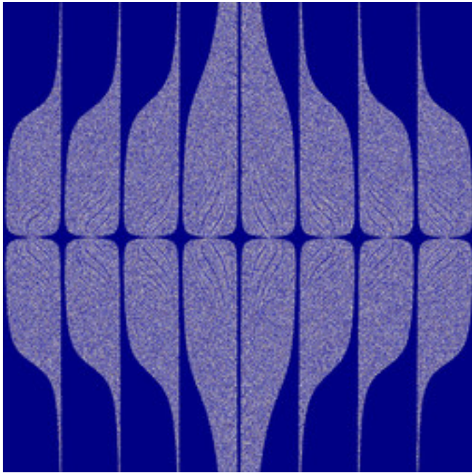
reb-GopalsamyFn-11.jpg
