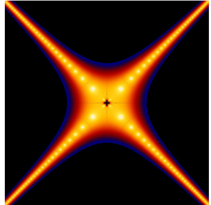
mt-zeepop-mset-49.jpg
