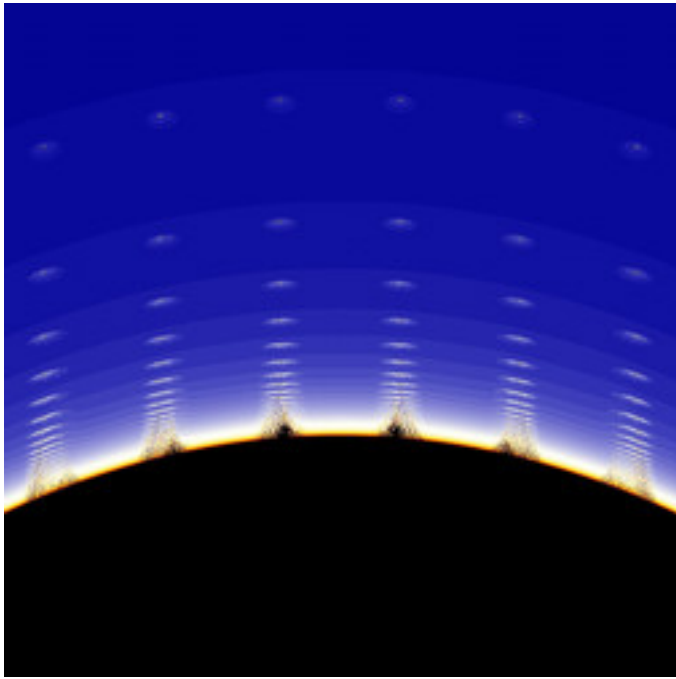
mt-ring-mset-03.jpg
