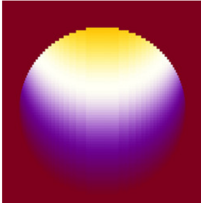
mt-GeneralizedCelticJulia-59.jpg
