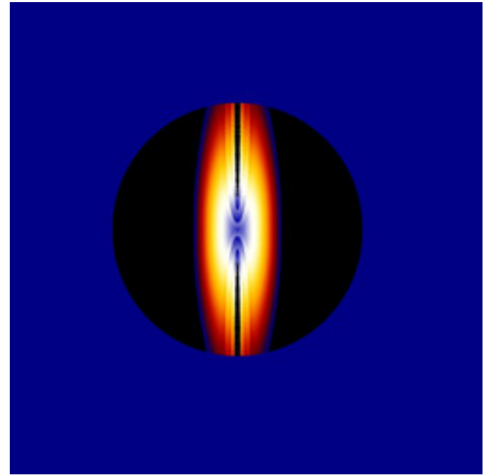
mt-zeepop-julia-05.jpg
