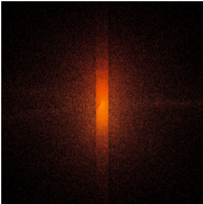
mt-newton-twist-02.jpg
