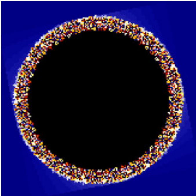
reb-FunBarnsley1Julia-14.jpg
