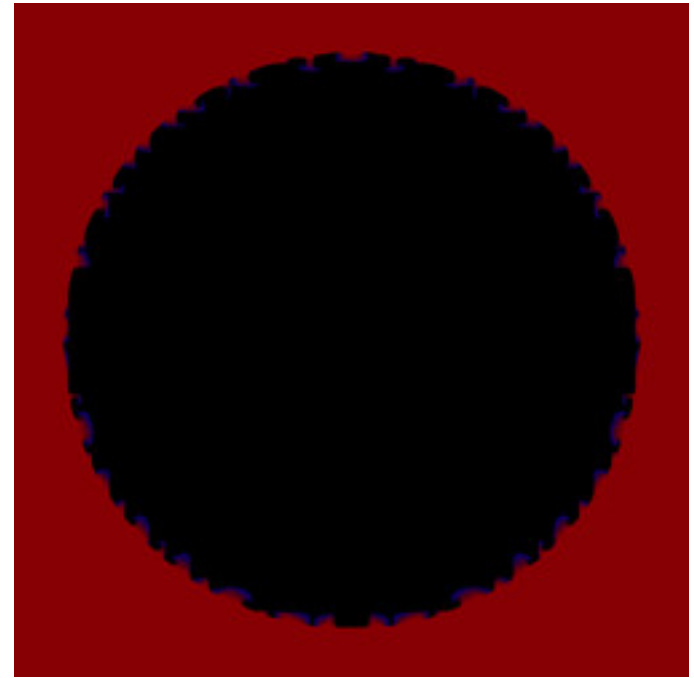
lkm3-FourierPopCorn-04G.jpg
