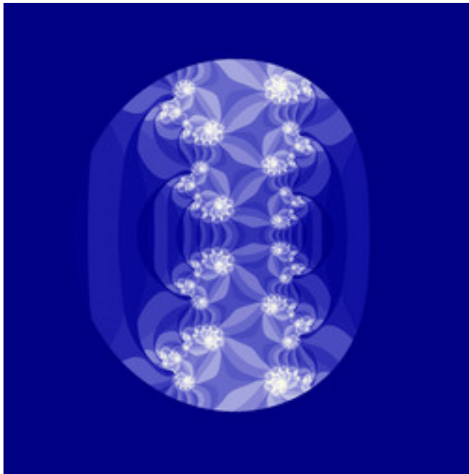
reb-ZeePi-01.jpg
