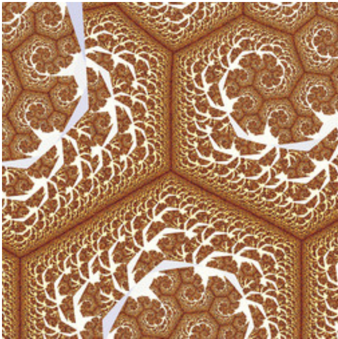
mt-barnsleyishJulia-09.jpg
