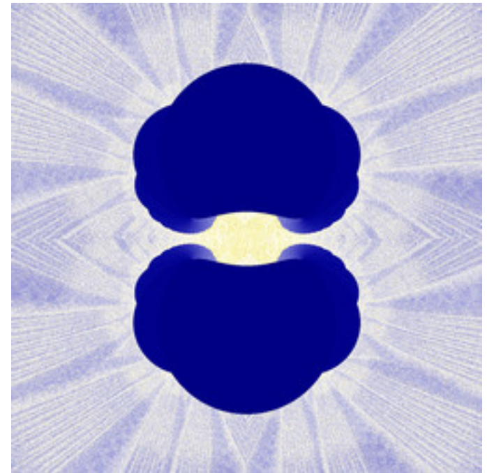
ahm-MonotonicGrowthJulia_03.jpg
