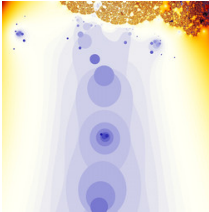
dmj-PhoenixDoubleNova-02.jpg
