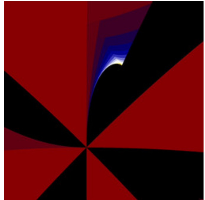
mt-990807bMset-20.jpg
