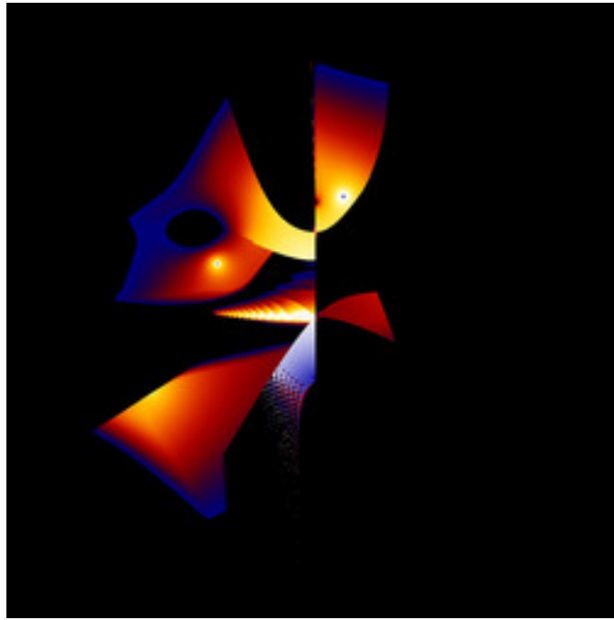
mt-zeepop-mset-42.jpg
