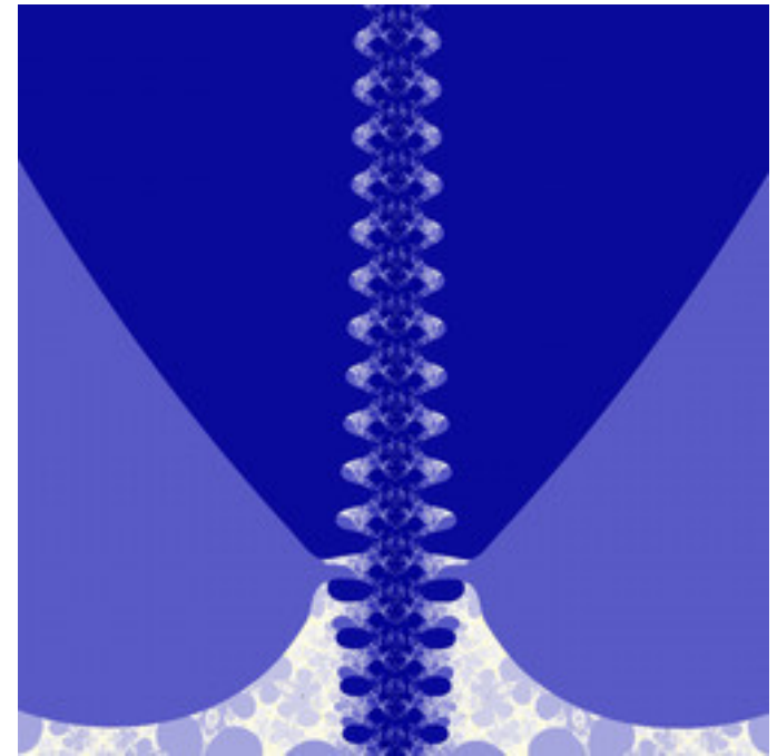
ldm-DM23-08.jpg
