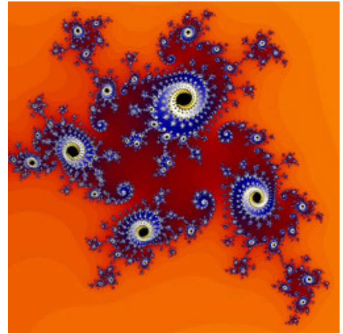
mt-990807bMset-05.jpg
