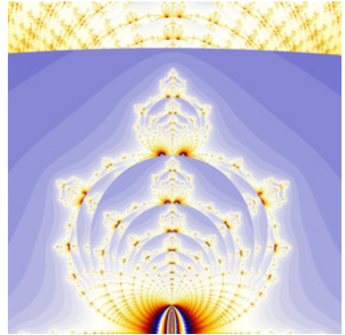
dmj-OrbitBoost-04.jpg
