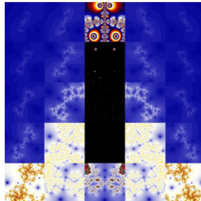
dmj-ManyNova-04.jpg
