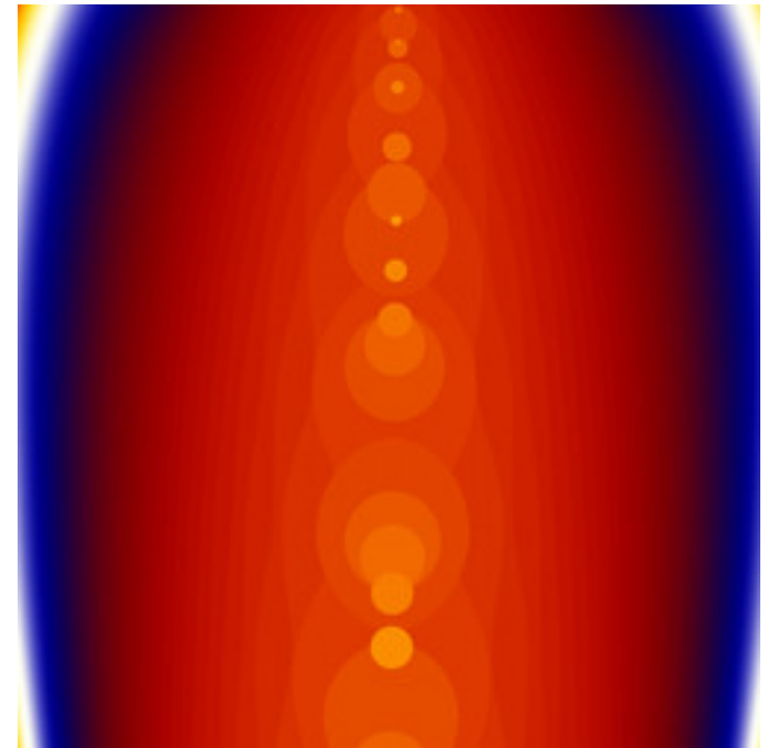
dmj-PhoenixDoubleNova-13.jpg
