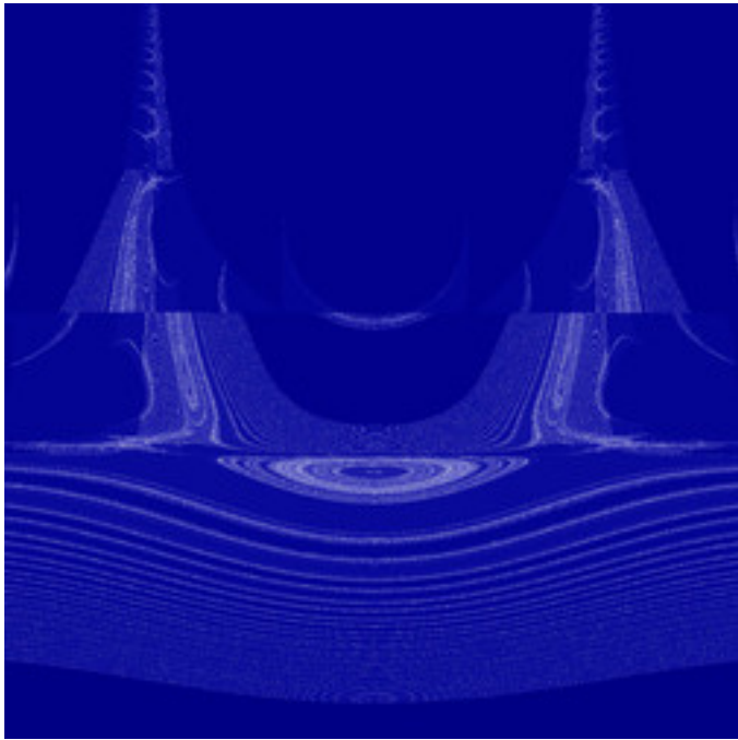
reb-GopalsamyFn-01.jpg
