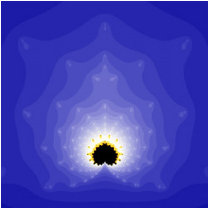
mt-modulate-mset-01.jpg
