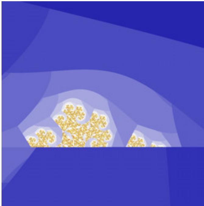
mt-barnsleyishJulia-02.jpg
