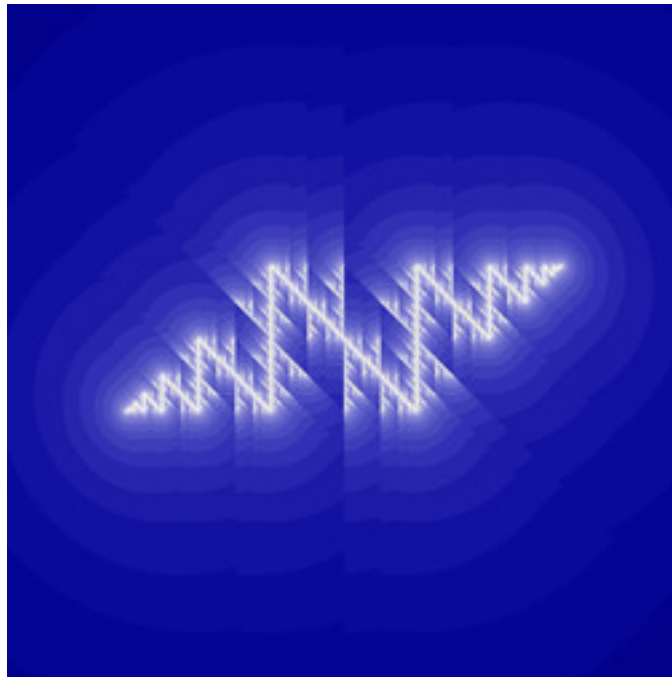
reb-FunBarnsley1Julia-01B.jpg
