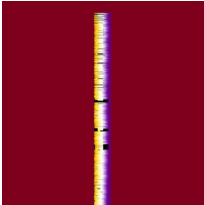
mt-GeneralizedCelticJulia-32.jpg
