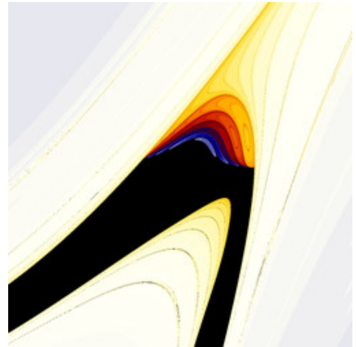
mt-990807aMset-36.jpg
