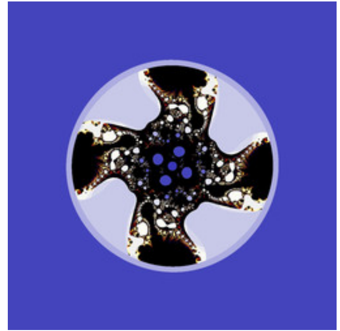
mt-rudys-cubic-mandelbrot-18.jpg
