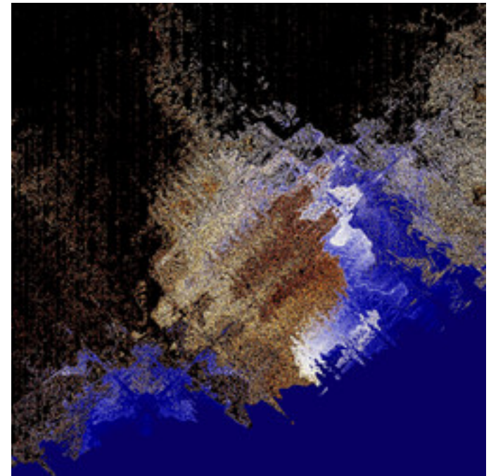
lkm3-FourierPopCorn-05A.jpg
