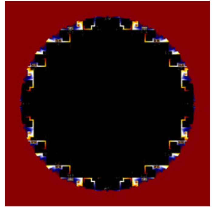
lkm3-FourierPopCorn-04A.jpg
