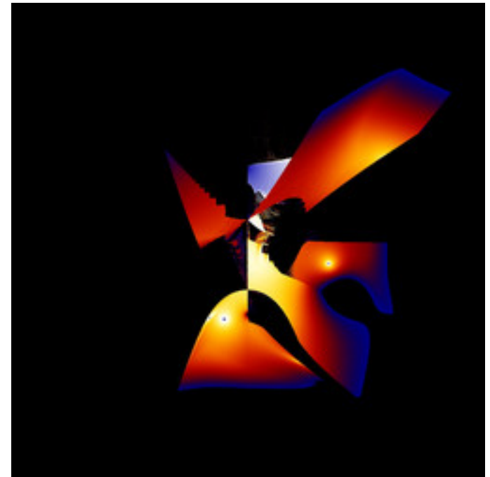
mt-zeepop-mset-32.jpg
