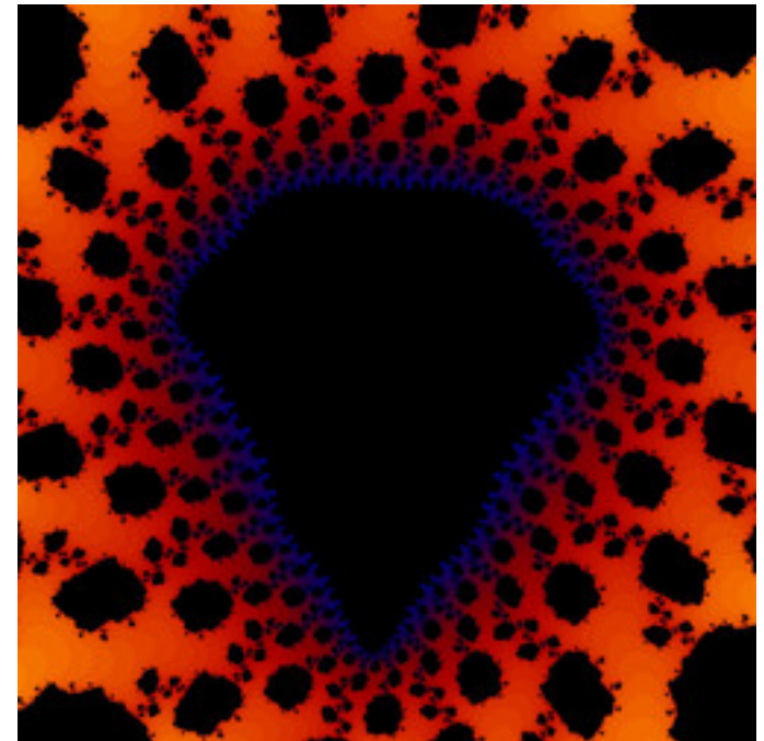
mt-990807aMset-02.jpg
