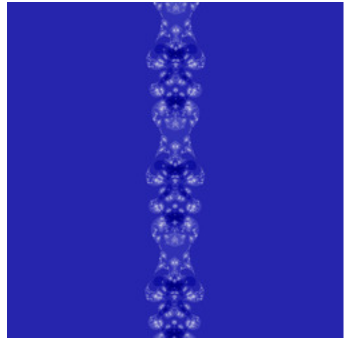
ldm-DM23-13a.jpg
