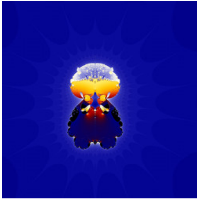
mt-zeepop-mset-53.jpg
