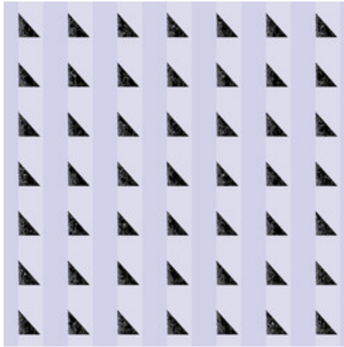
dmj-ManyNova-13.jpg
