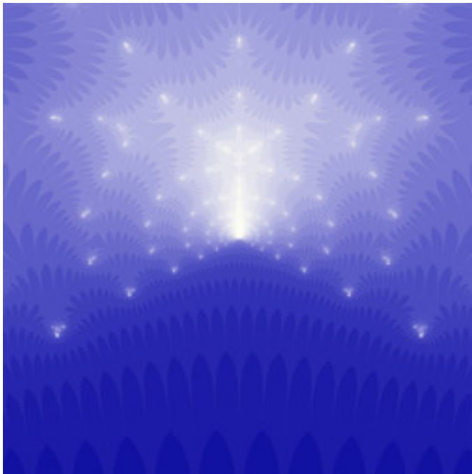
reb-JonHomerSpider-02.jpg
