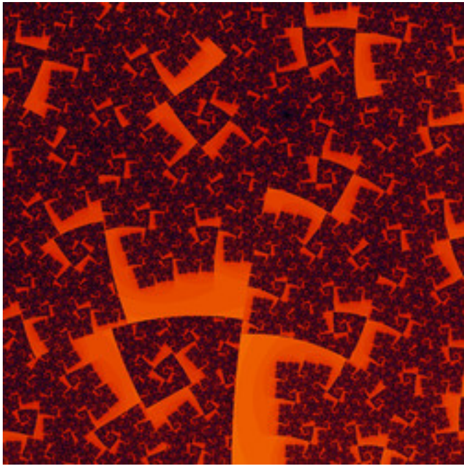
mt-rudys-cubic-mandelbrot-26.jpg
