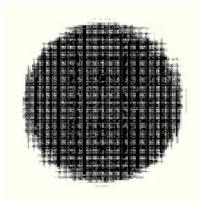
lkm3-FourierPopCorn-07.jpg
