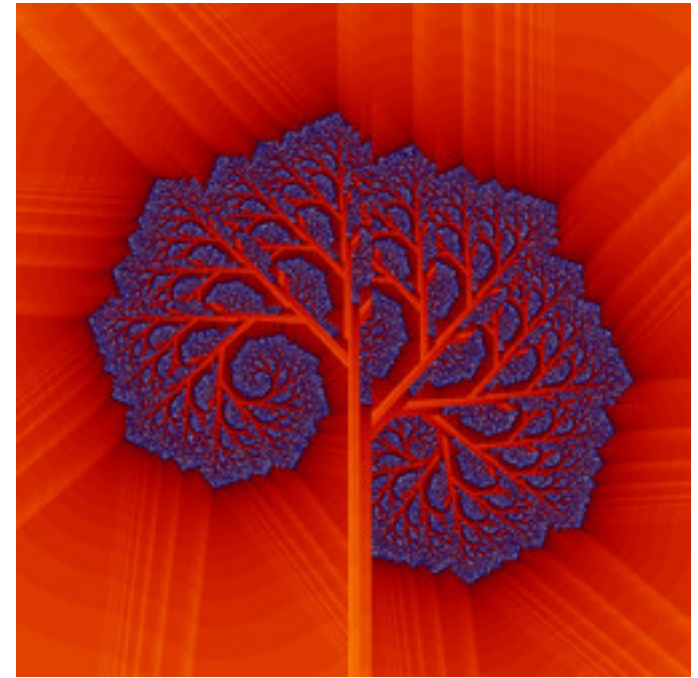
reb-IFSEscape1-07B.jpg
