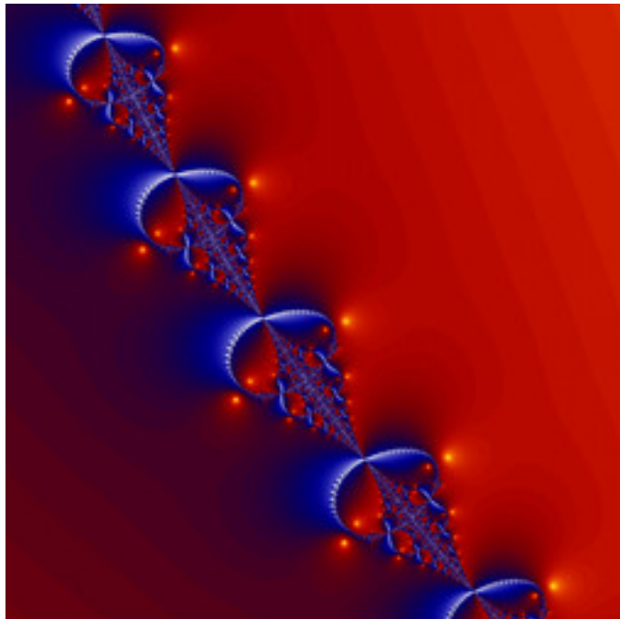
dmj-NovaMandel-01.jpg
