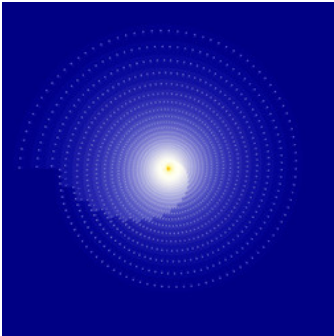
reb-LambdaPower-01.jpg
