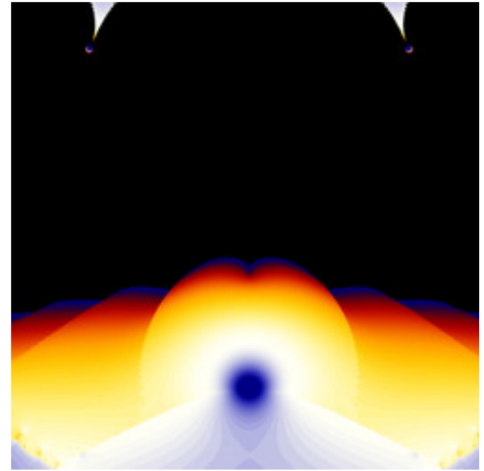
mt-zeepop-mset-52.jpg
