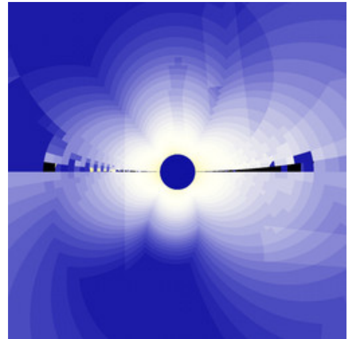
mt-zeepop-julia-20.jpg
