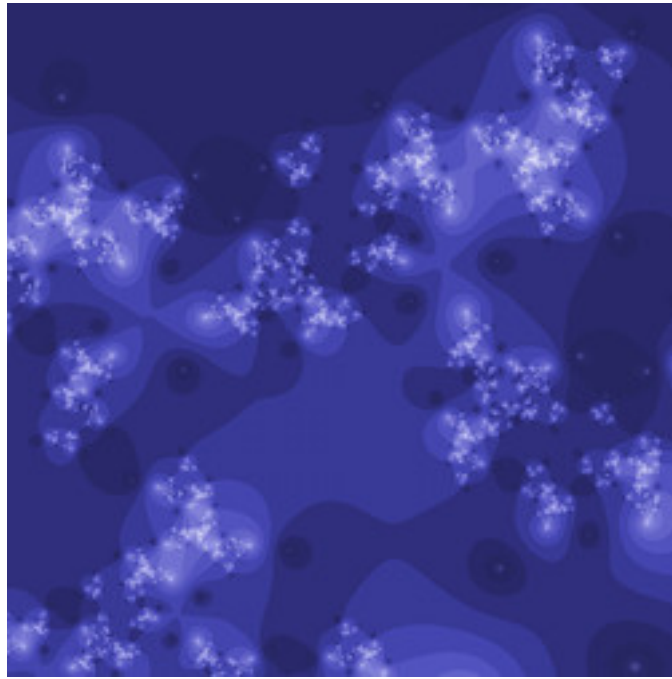
dmj-DoubleHalleyNova-03.jpg
