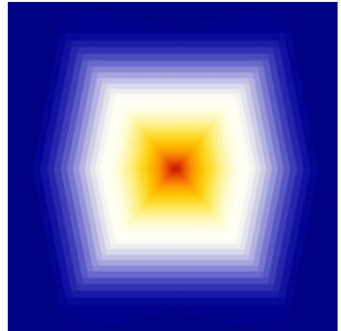
reb-FunBarnsley1Julia-13A.jpg
