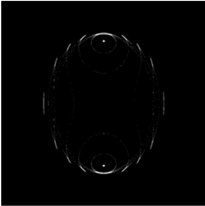
reb-FormulaTracer-09C.jpg
