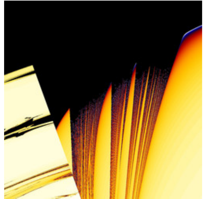
mt-990807aMset-24.jpg
