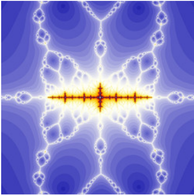
reb-IkenagaRoots-Julia-01.jpg
