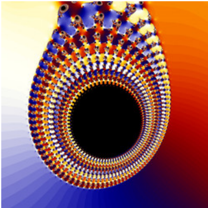
mt-newton-error-03c.jpg
