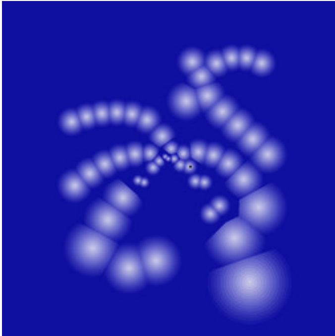
abs-Fortuitus_Mistakes_05.jpg
