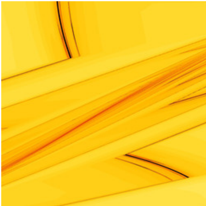
lkm3-MixexupJulia-01.jpg
