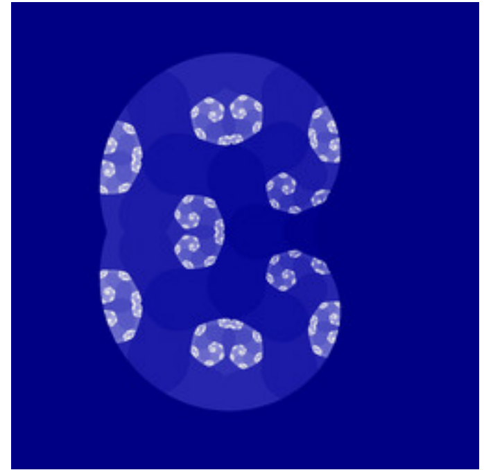
reb-ZeePi-03.jpg
