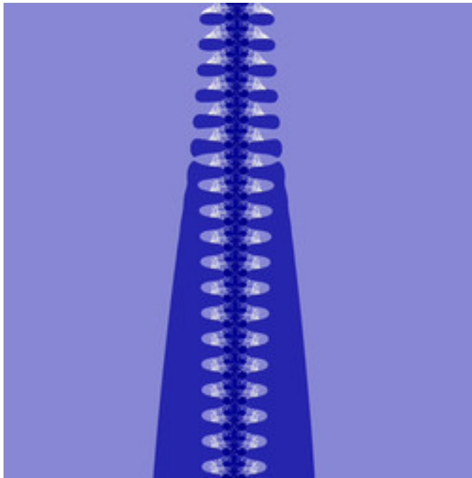
ldm-DM23-14.jpg
