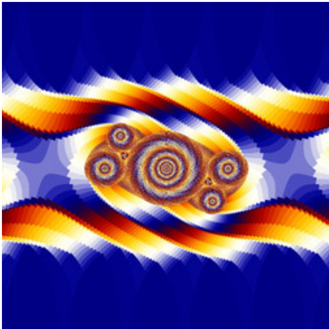
reb-JuliaTentMap-10.jpg
