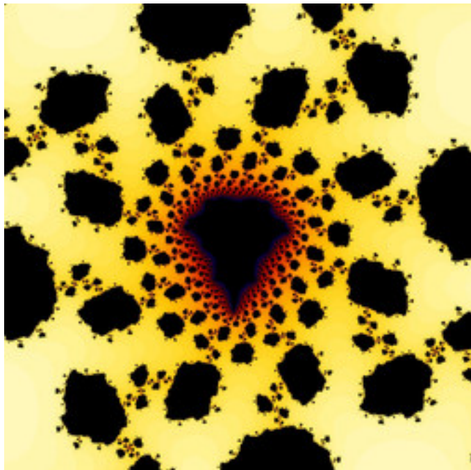
mt-990807aMset-01.jpg
