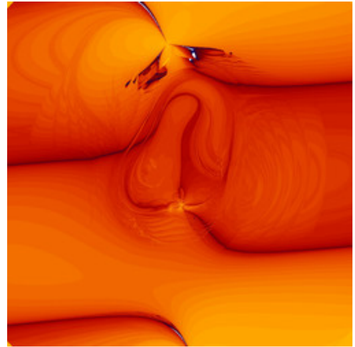
asz-andrextandom-1-16.jpg
