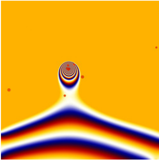
dmj-PhoenixDoubleNova-24.jpg
