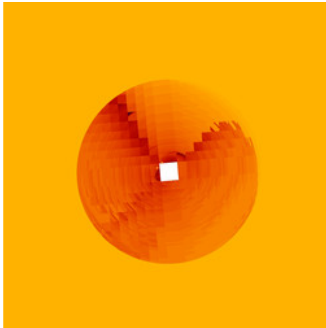
asz-andrexrandom-1-32.jpg
