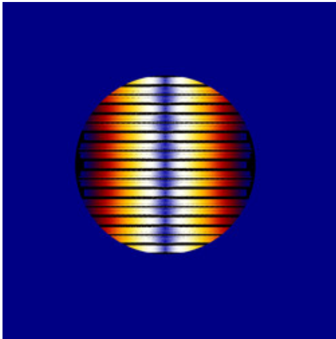
mt-zeepop-julia-03.jpg
