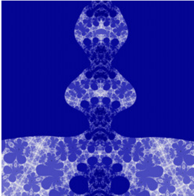
ldm-DM23-03.jpg
