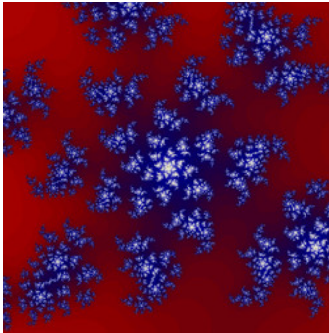
mt-990807bMset-03.jpg
