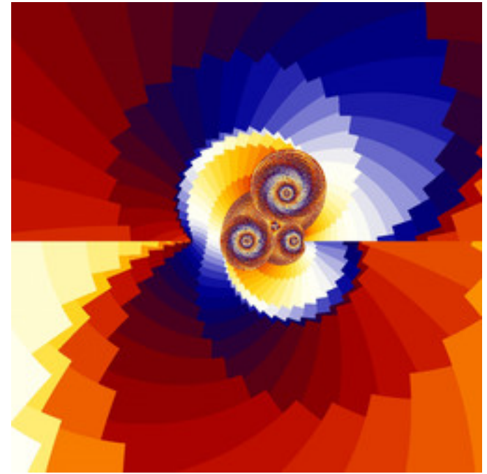
reb-JuliaTentMap-11.jpg
