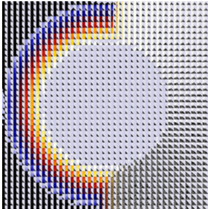
dmj-ManyNova-16.jpg
