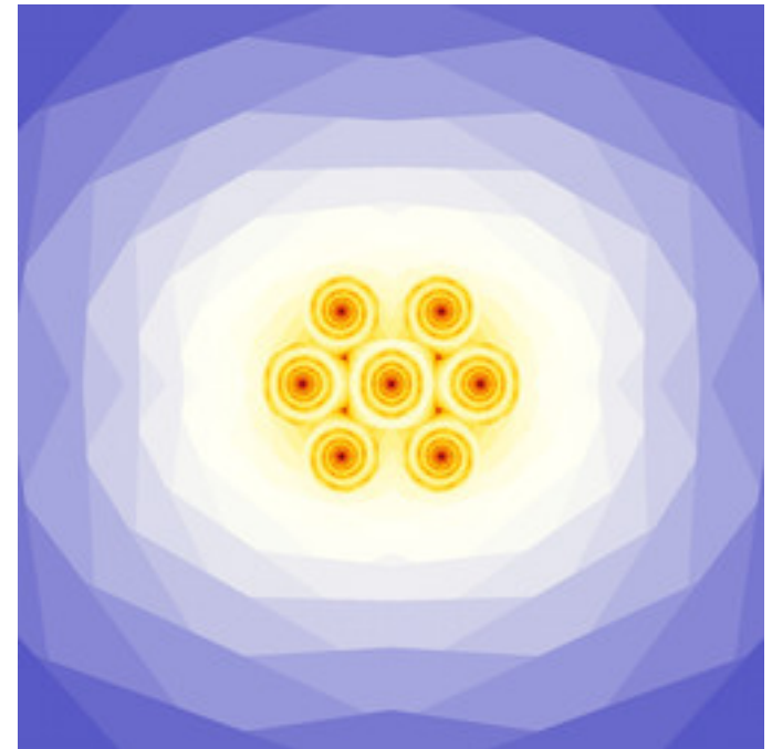
reb-JuliaTentMap-08.jpg
