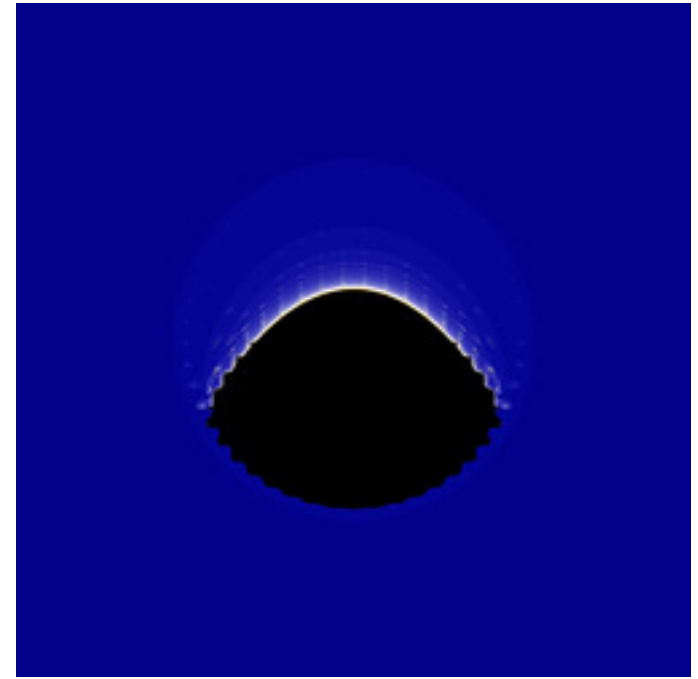
mt-ring-mset-01.jpg
