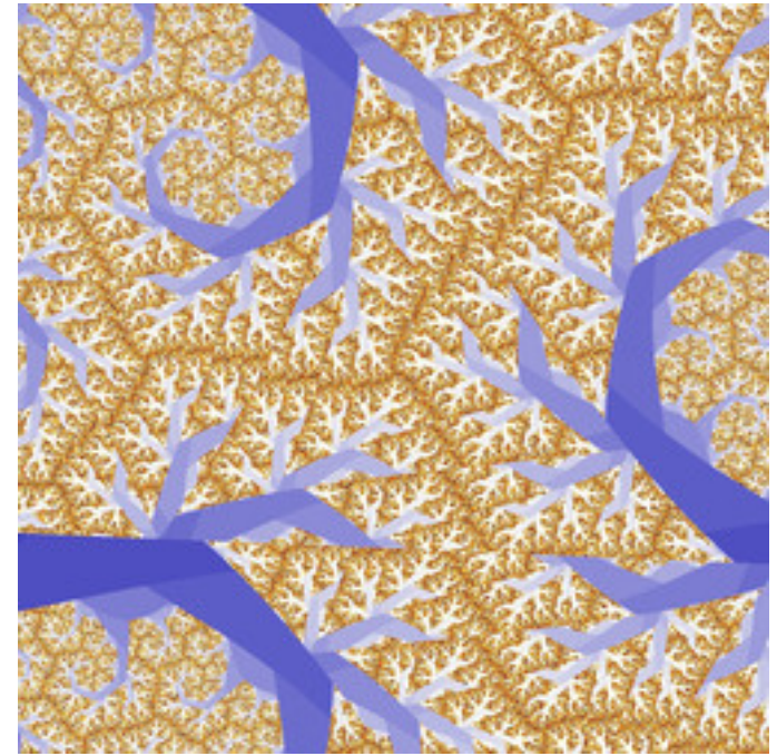
mt-barnsleyishJulia-10.jpg
