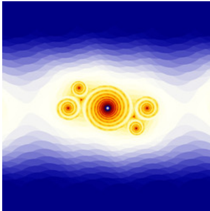
reb-JuliaTentMap-09.jpg
