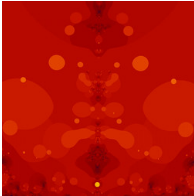
dmj-PhoenixDoubleNova-14.jpg
