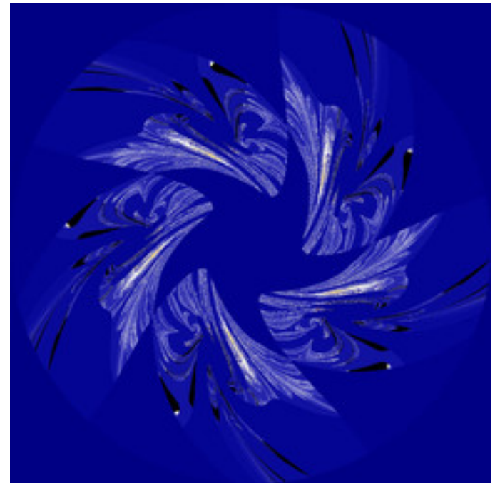
ahm-IndependantPower_06.jpg
