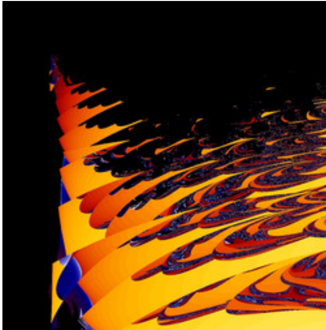
mt-990807aMset-25.jpg
