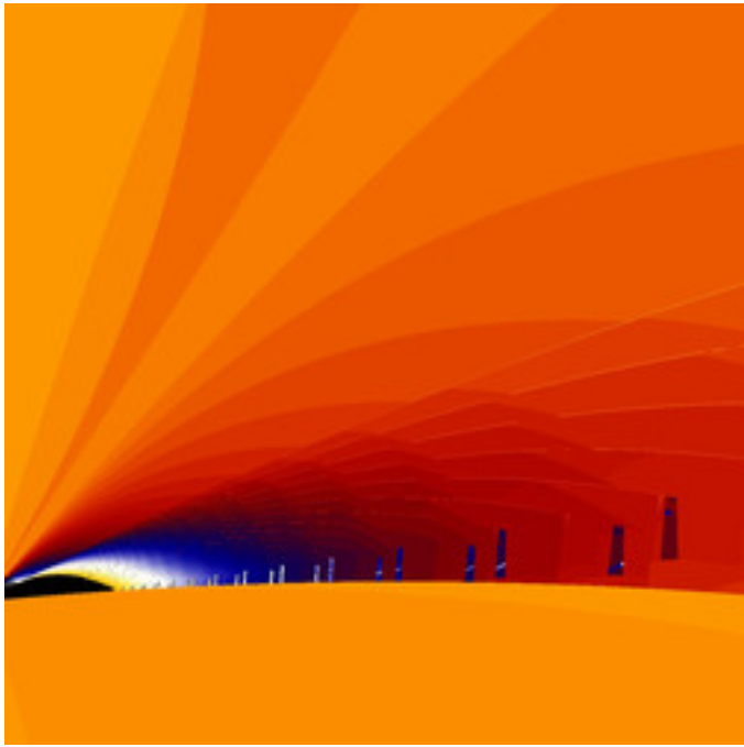
mt-990807bMset-25.jpg
