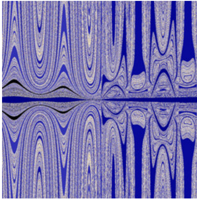
reb-GopalsamyFn-16.jpg
