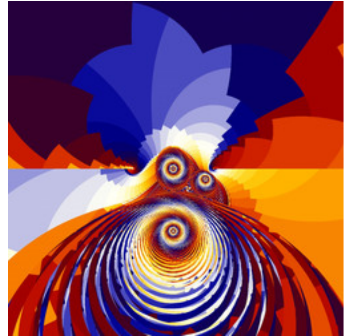
reb-JuliaTentMap-13B.jpg
