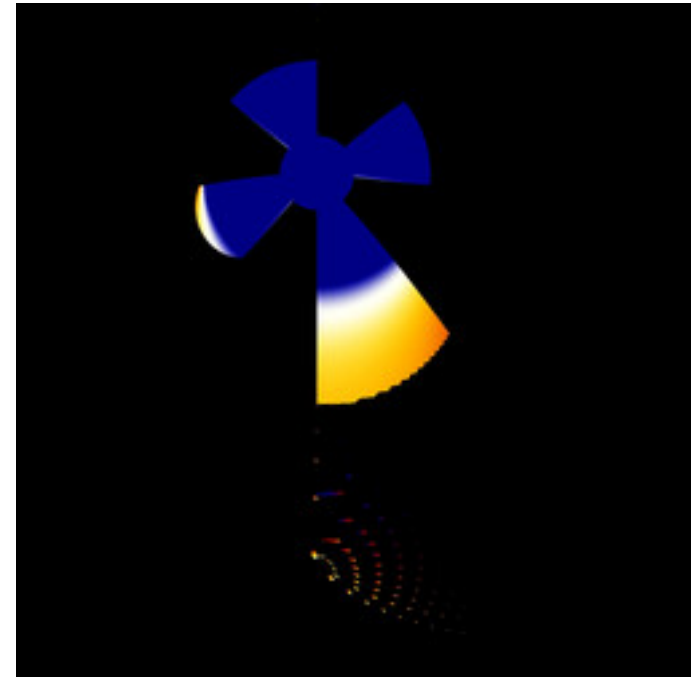
mt-zeepop-mset-46.jpg
