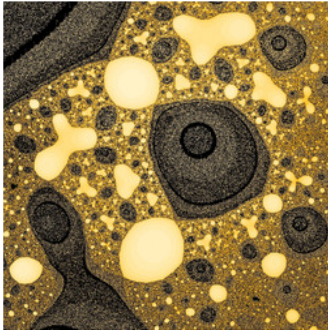
mt-magnetism-model-ii-08.jpg
