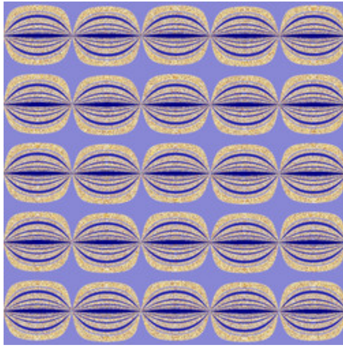
reb-GopalsamyFn-22.jpg
