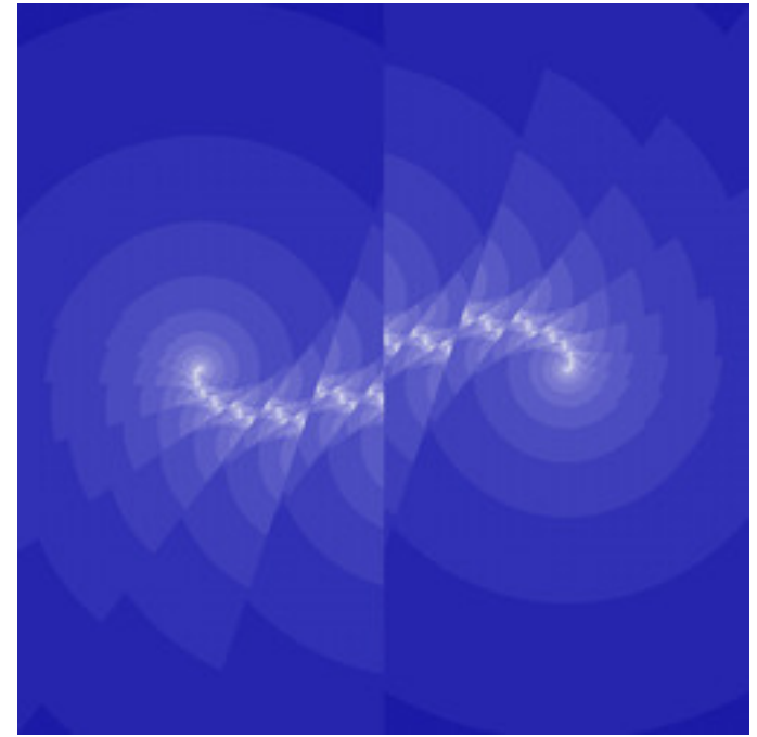
lkm-GeneralTentJulia-01.jpg
