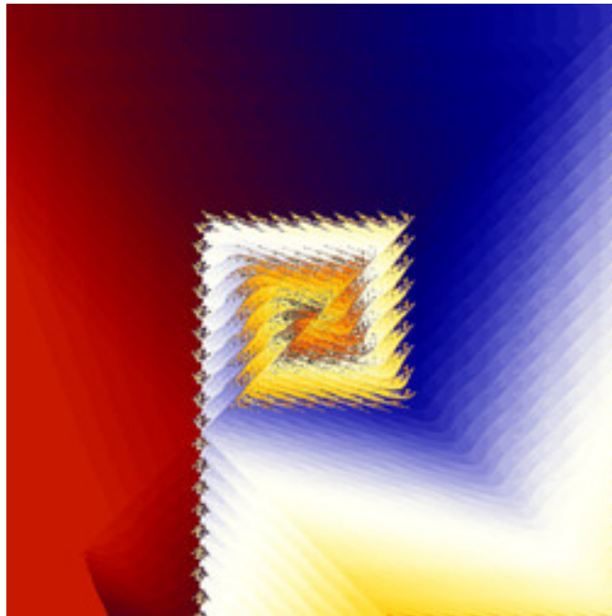
lkm3-FourierPopCorn-02.jpg
