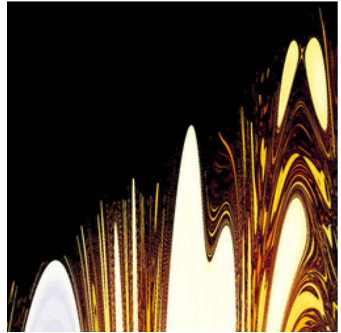
mt-990625bMset-07.jpg
