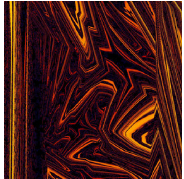
lkm3-MixexupMandelbrot-04.jpg
