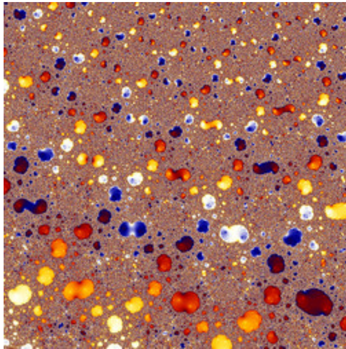
dmj-DoubleNova-08.jpg
