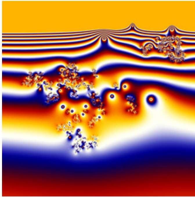
dmj-PhoenixDoubleNova-17.jpg
