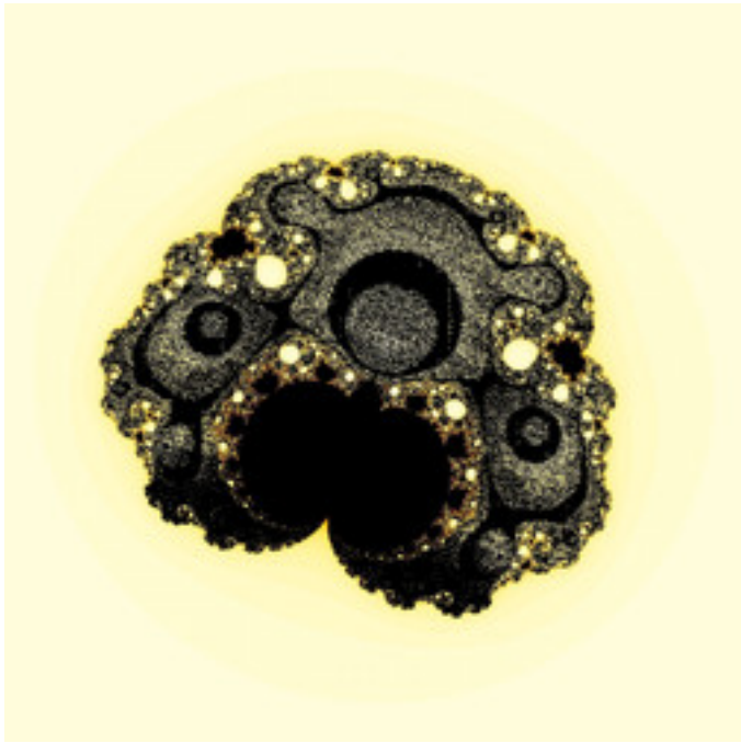
mt-magnetism-model-ii-03.jpg
