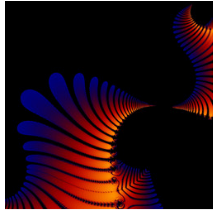
lkm-EmbossedNewton-03.jpg
