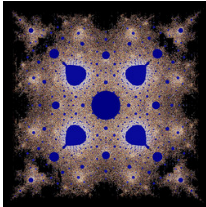
mt-rudys-cubic-mandelbrot-04b.jpg
