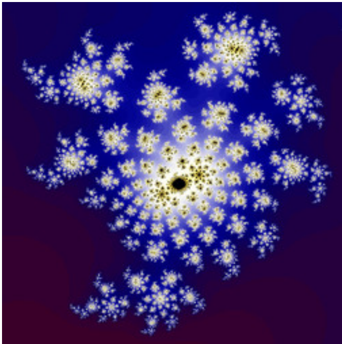
mt-990807bMset-04.jpg
