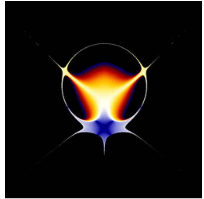
mt-zeepop-mset-05.jpg
