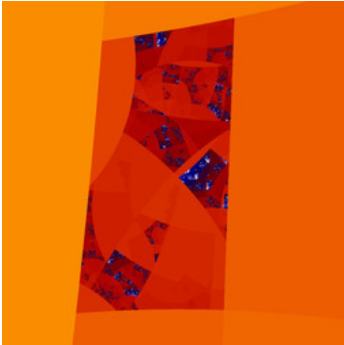
mt-990807bMset-10.jpg
