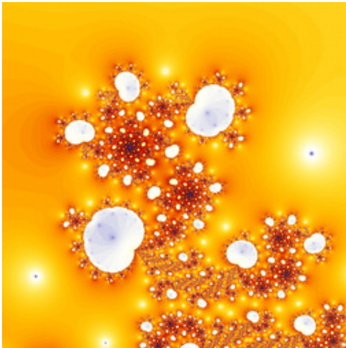
dmj-DoubleNova-03.jpg
