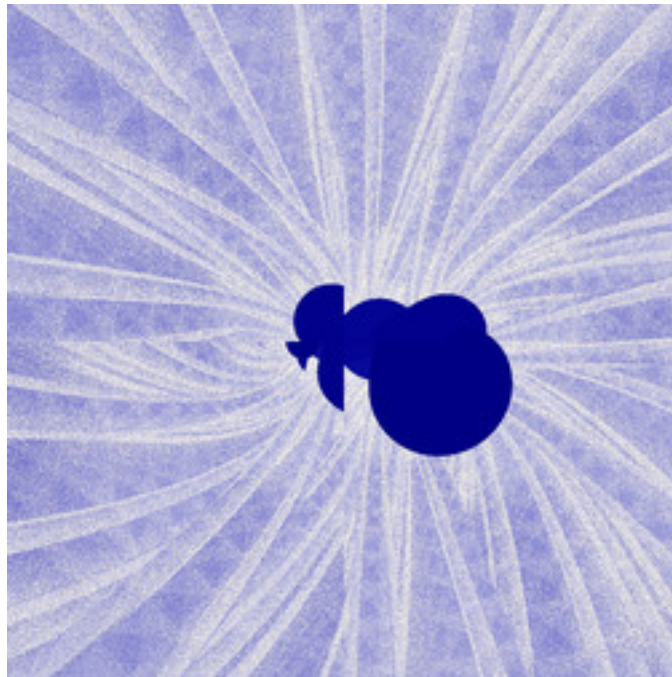
ahm-MonotonicGrowthJulia_04.jpg
