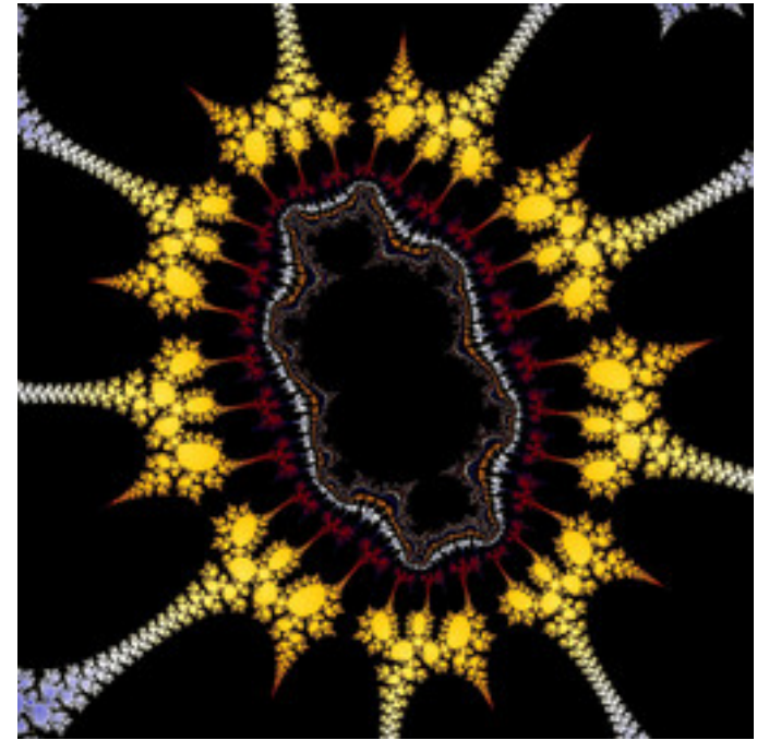
mt-magnetism-model-ii-01.jpg
