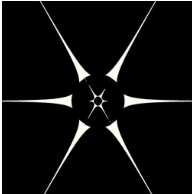
mt-rudys-cubic-mandelbrot-28.jpg
