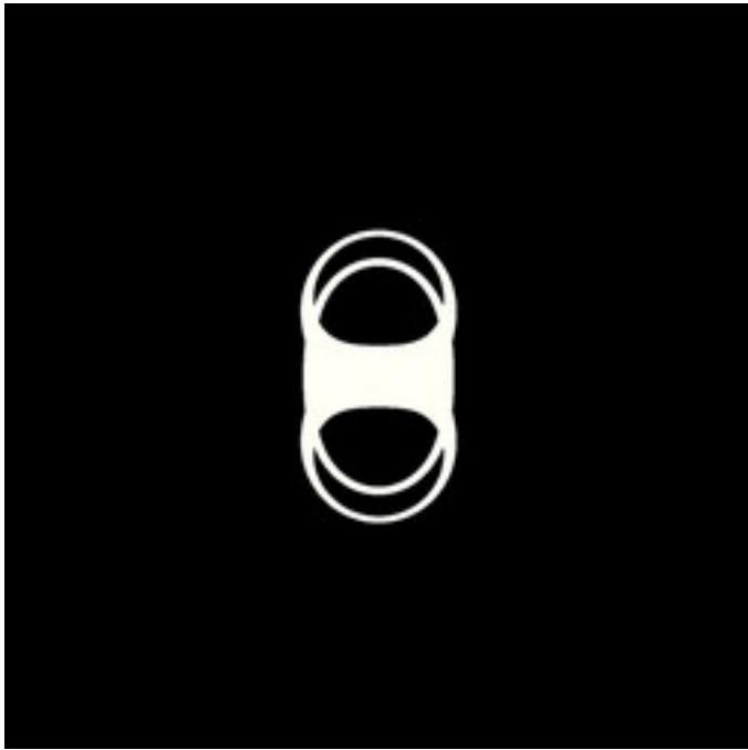
reb-FormulaTracer-17A.jpg
