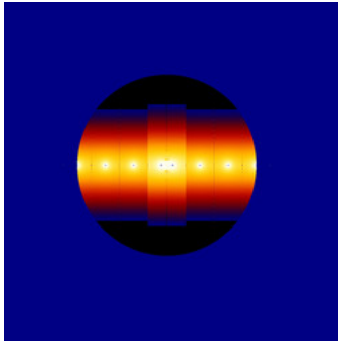
mt-zeepop-julia-09.jpg
