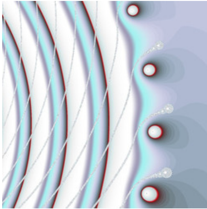
dmj-NovaMandel-09.jpg
