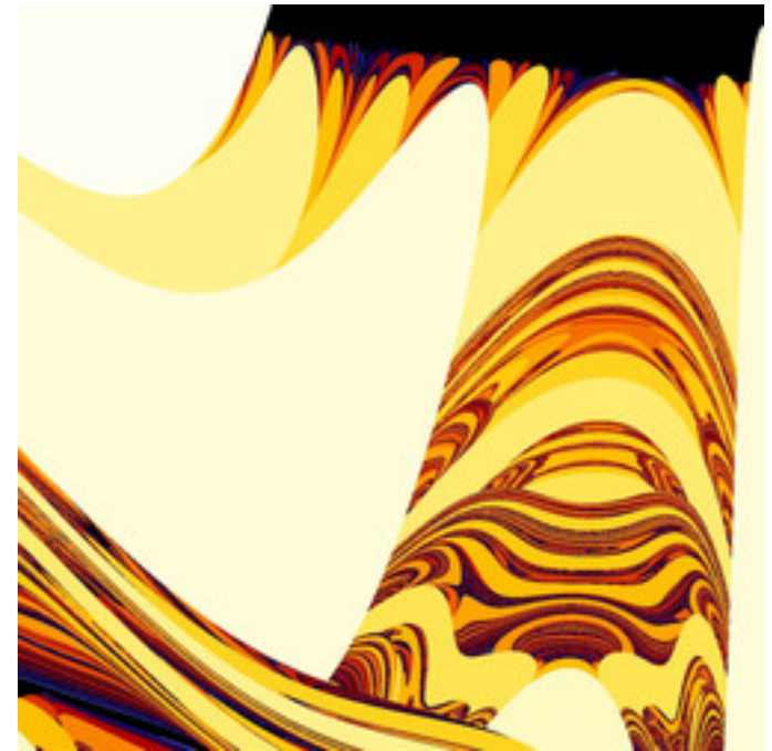
mt-990807aMset-30.jpg
