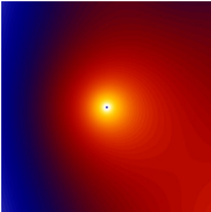
mt-newton-error-17d.jpg
