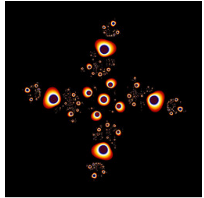
mt-rudys-cubic-mandelbrot-12.jpg
