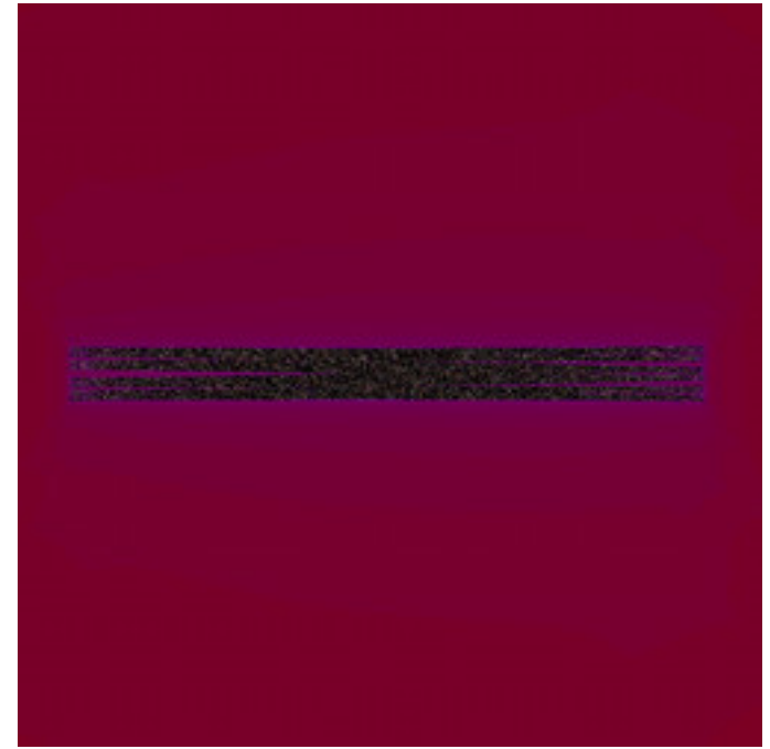
mt-GeneralizedCelticJulia_03.jpg
