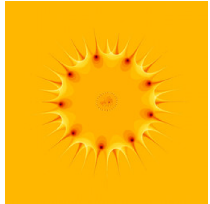
mt-rudys-cubic-julia-12.jpg
