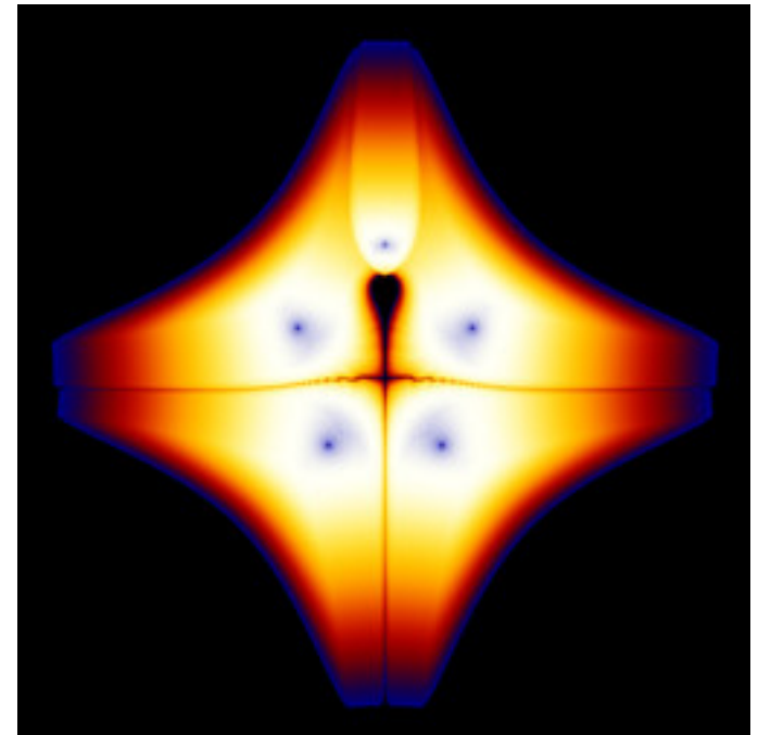
mt-zeepop-mset-38.jpg
