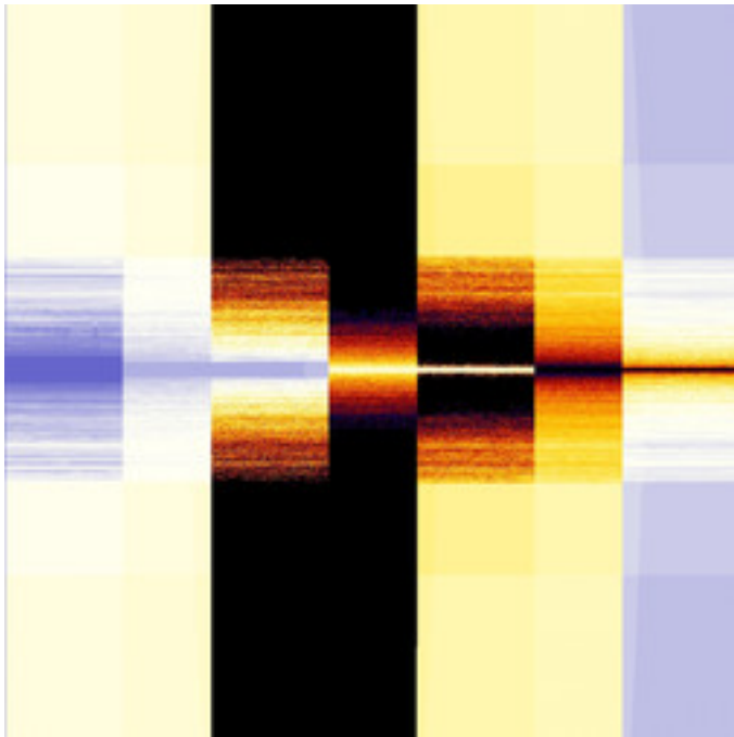
mt-bifunctionalMset-10.jpg
