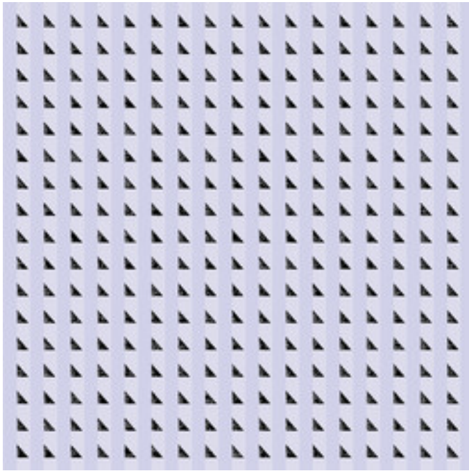
dmj-ManyNova-14.jpg
