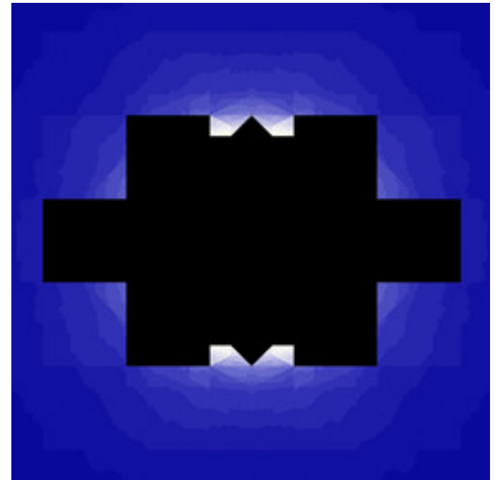
reb-SlopeExpFun_BarnsleyM1-01.jpg
