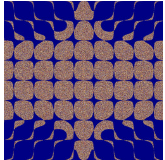
reb-GopalsamyFn-09.jpg
