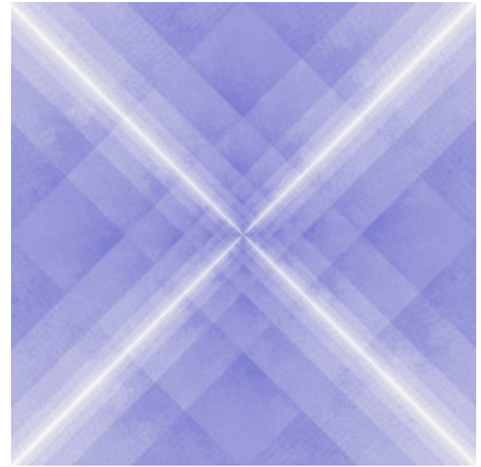
dmj-NovaMandel-102.jpg
