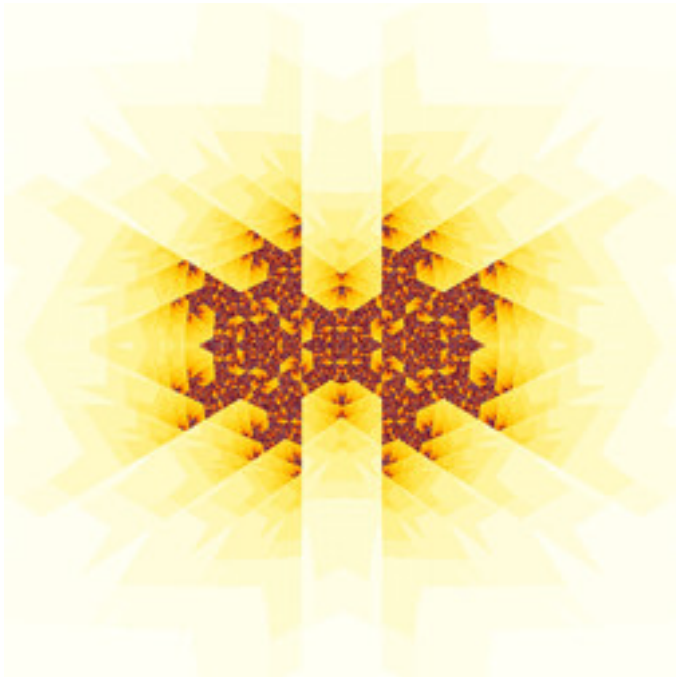
reb-JuliaTentMap-01.jpg
