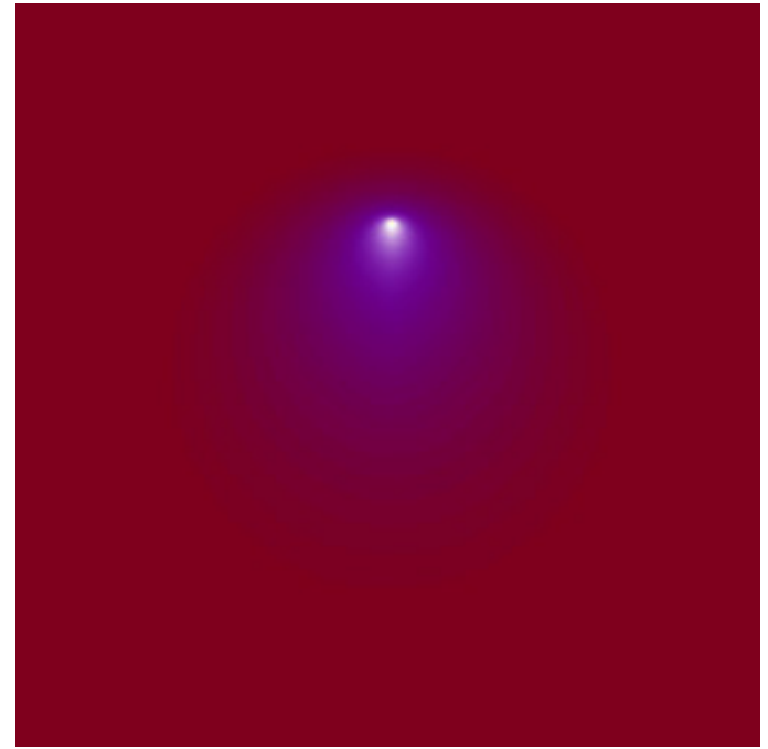
mt-GeneralizedCelticJulia-55.jpg
