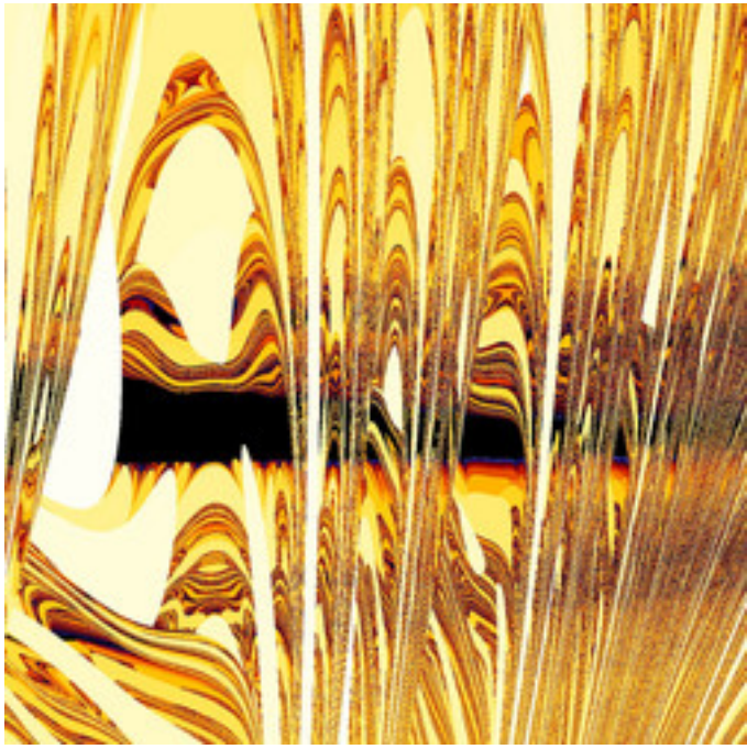
mt-990807aMset-29.jpg
