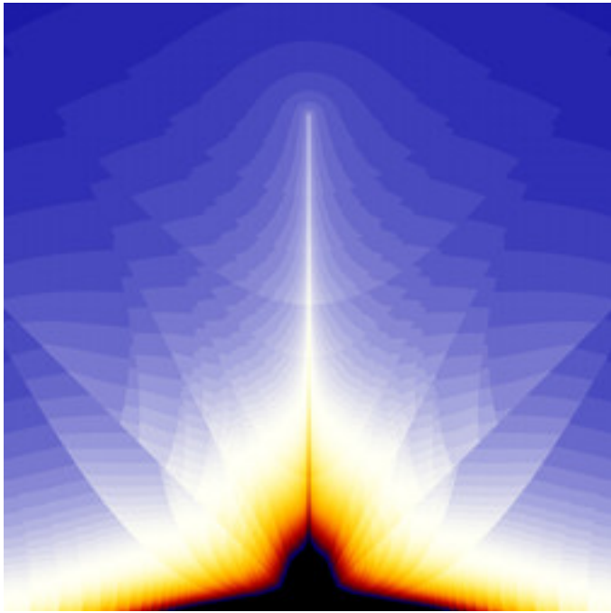
lkm-GeneralTentMandelbrot-01.jpg
