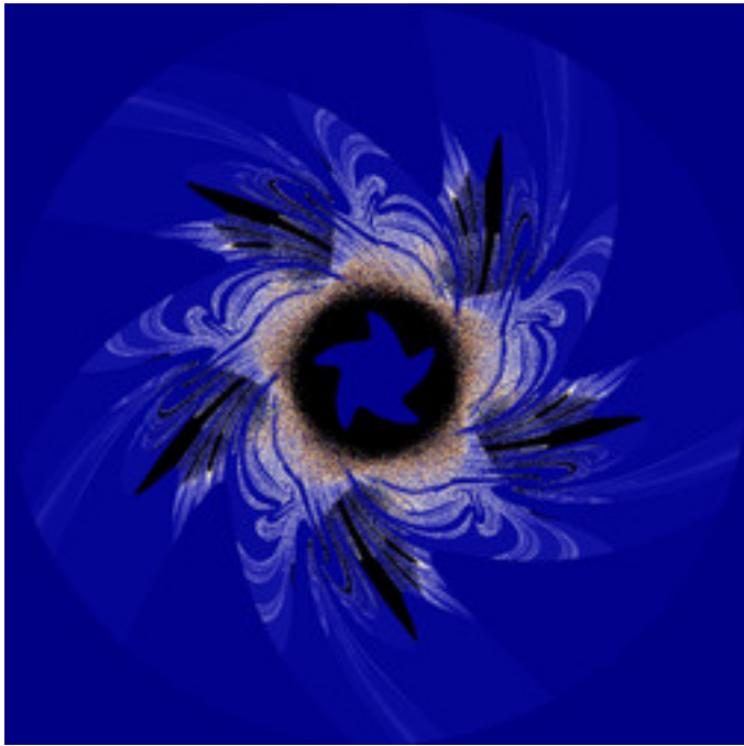
ahm-IndependantPower_05.jpg
