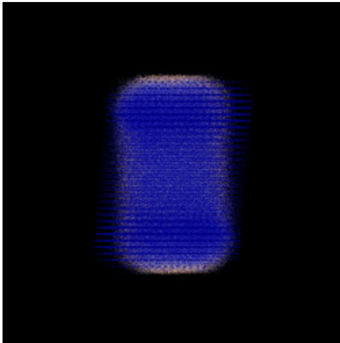
mt-latoocarfian-ii-36.jpg
