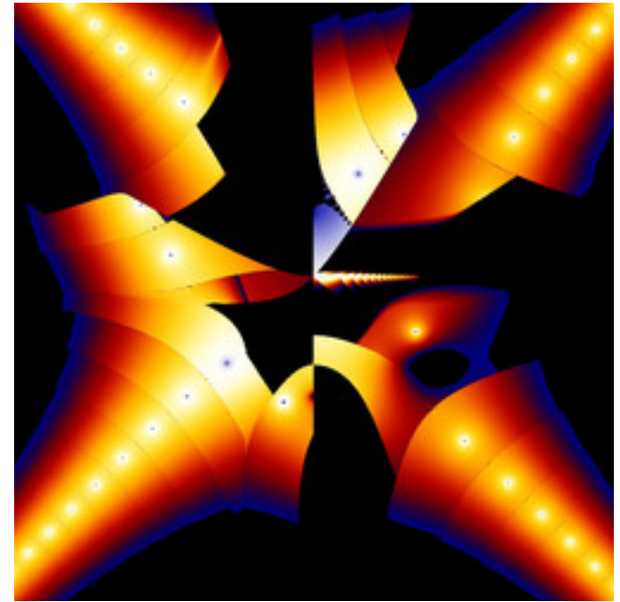
mt-zeepop-mset-29.jpg
