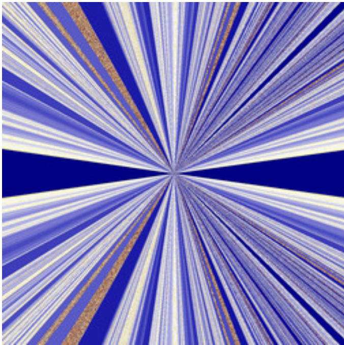
reb-GopalsamyFn-26.jpg
