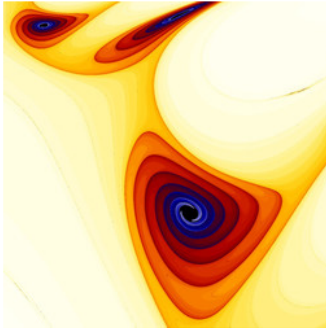
mt-990807aMset-40.jpg
