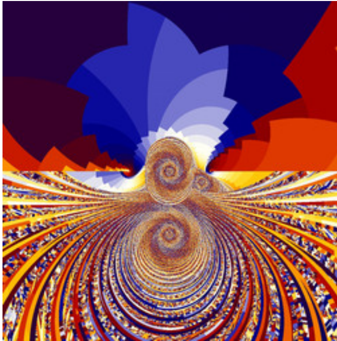
reb-JuliaTentMap-13C.jpg
