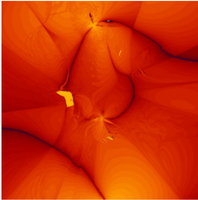
asz-andrextandom-1-17.jpg
