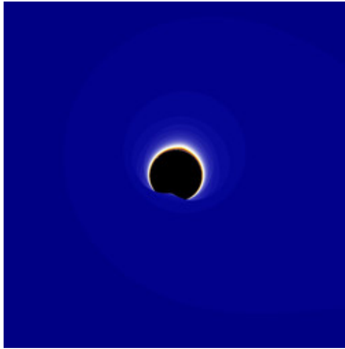
reb-Ikenagafn-04.jpg
