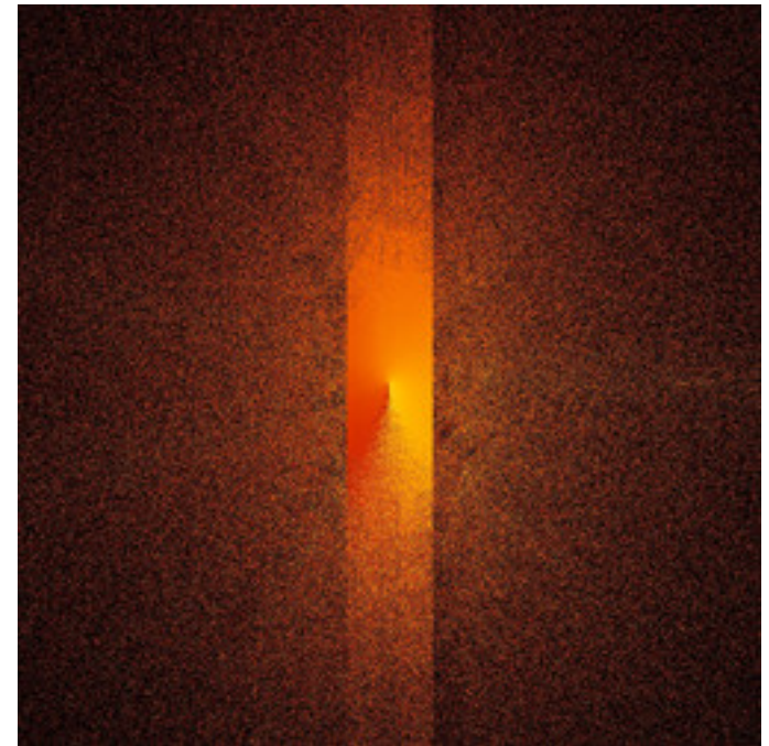
mt-newton-twist-12.jpg
