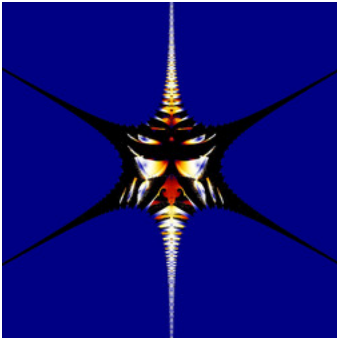
mt-zeepop-mset-45.jpg
