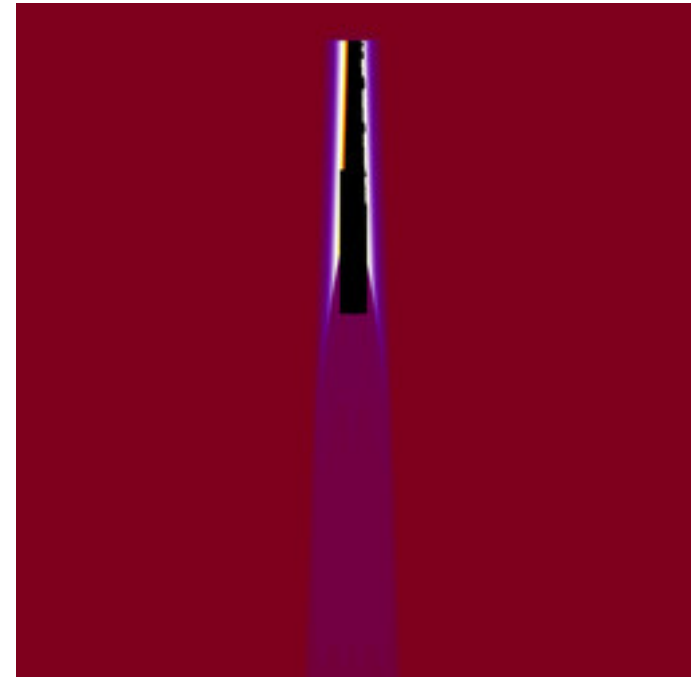
mt-GeneralizedCelticJulia-19.jpg
