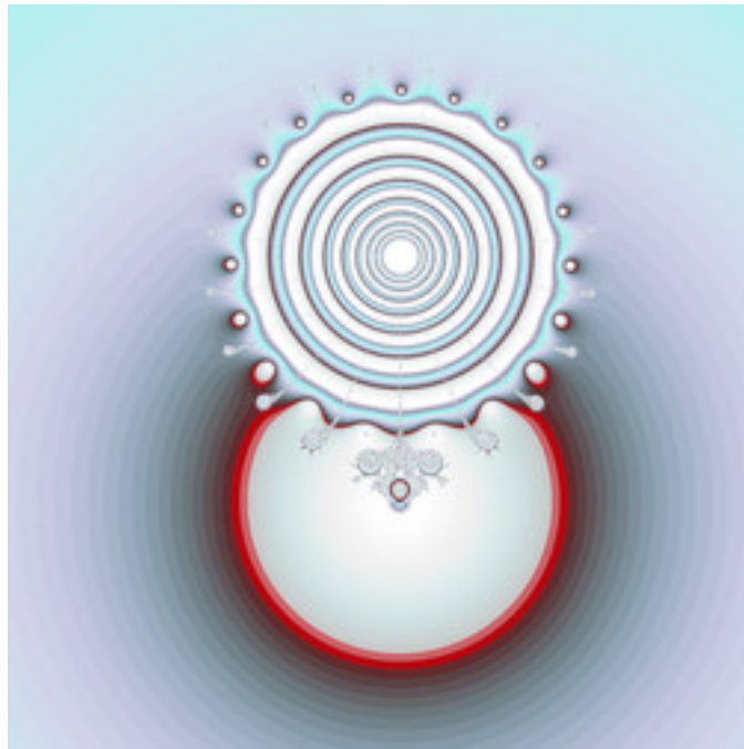
dmj-NovaMandel-06.jpg
