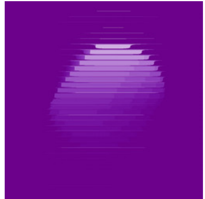
mt-GeneralizedCelticJulia-64.jpg
