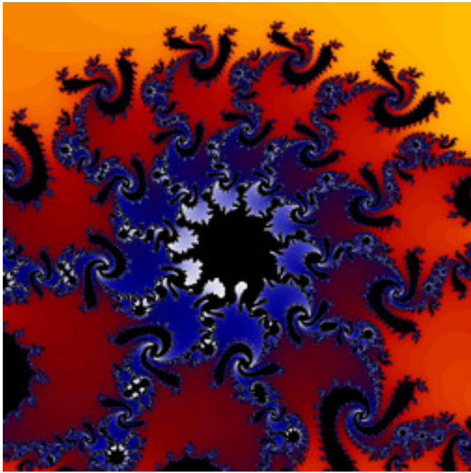
mt-990807aMset-07.jpg
