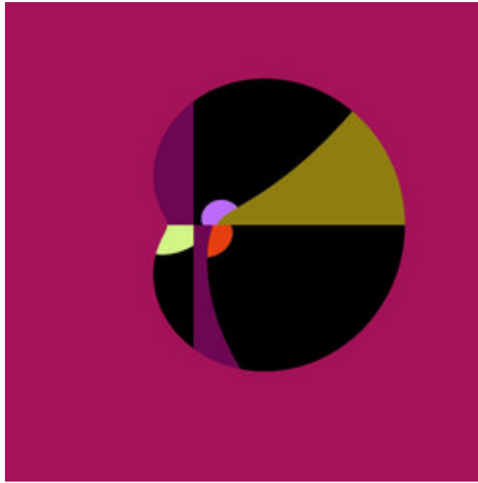
ads-Cantant_02.jpg
