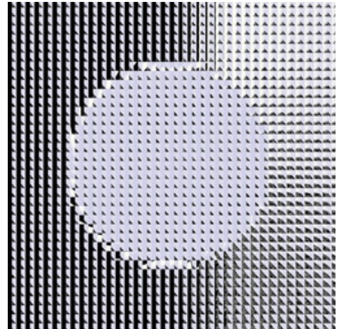
dmj-ManyNova-15.jpg
