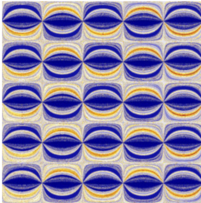
reb-GopalsamyFn-25.jpg
