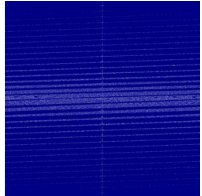
reb-GopalsamyFn-02.jpg
