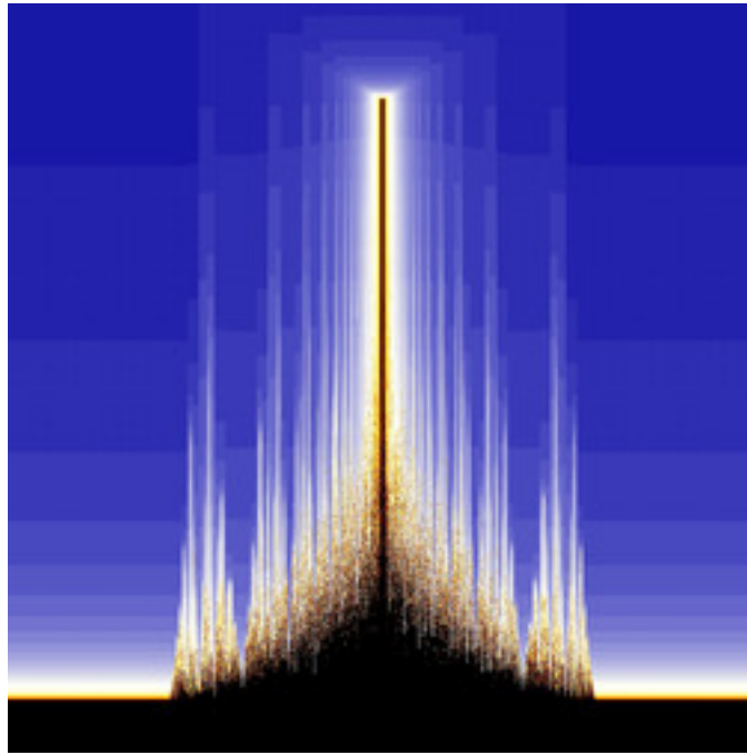
mt-bifunctionalMset-12.jpg
