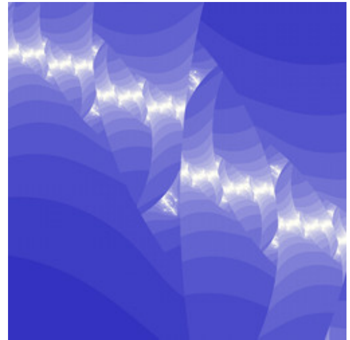
dmj-OrbitBoost-01.jpg
