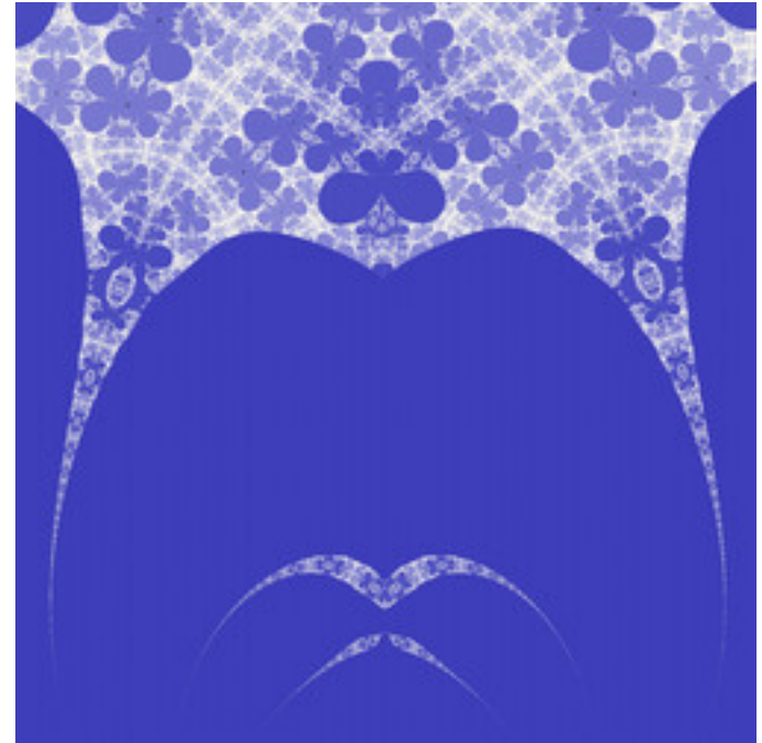
ldm-DM23-02.jpg
