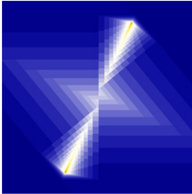
reb-FunBarnsley1Julia-06B.jpg
