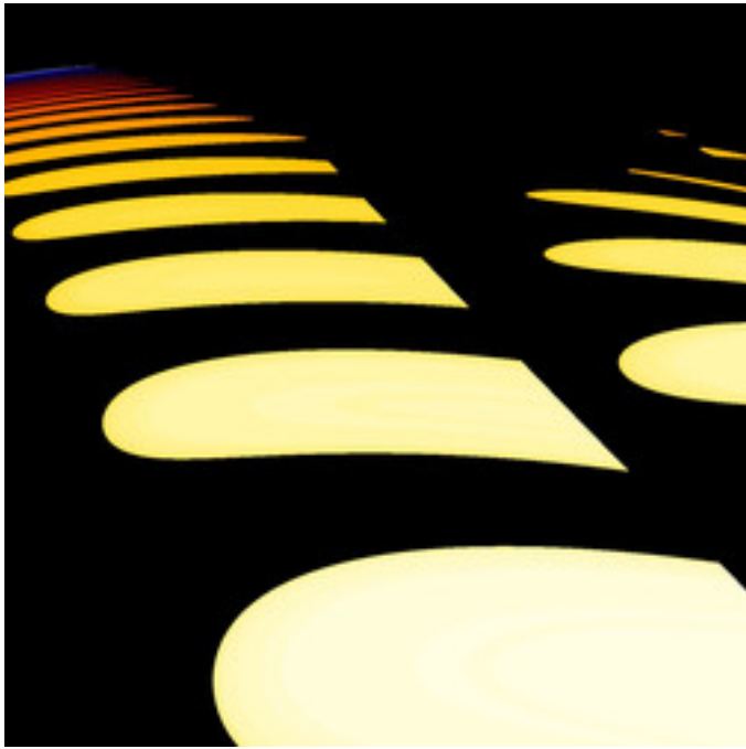
mt-990807aMset-41.jpg
