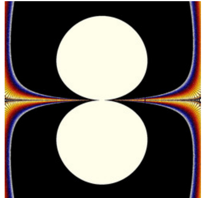
mt-newton-function-01.jpg
