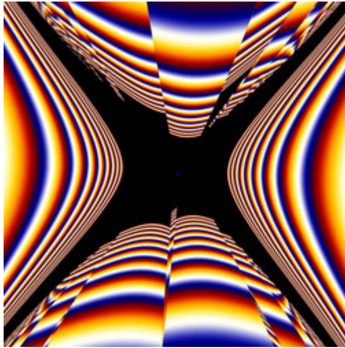
mt-newton-9904a-06.jpg
