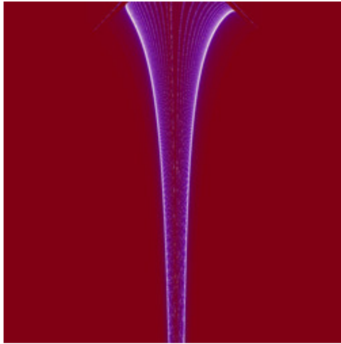
mt-GeneralizedCelticJulia-08.jpg
