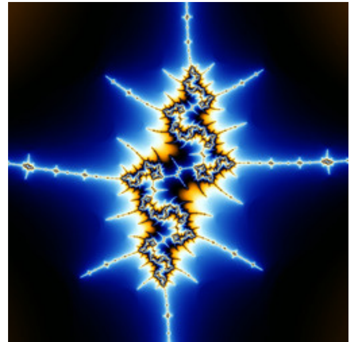
standard-FastMandel-05.jpg
