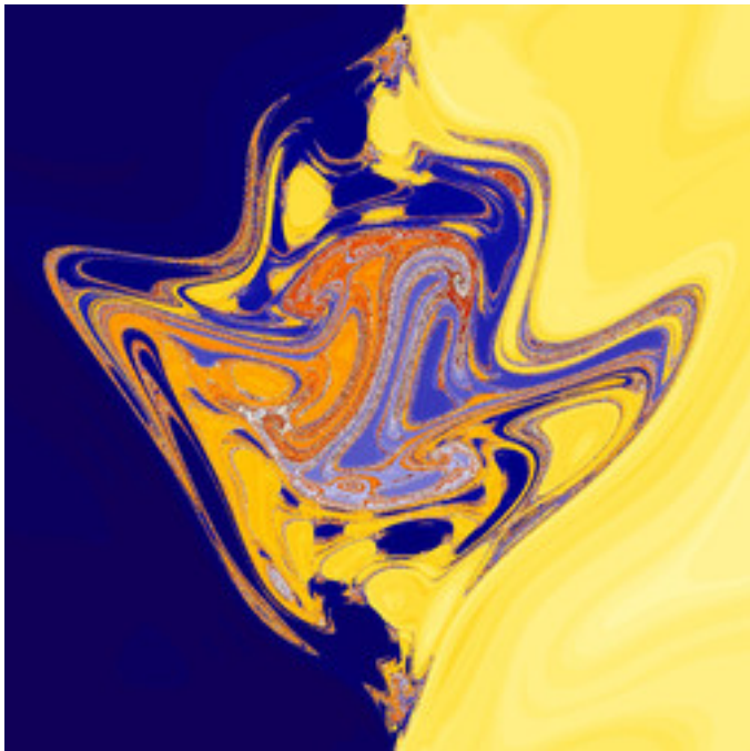
lkm3-FourierPopCorn-03.jpg
