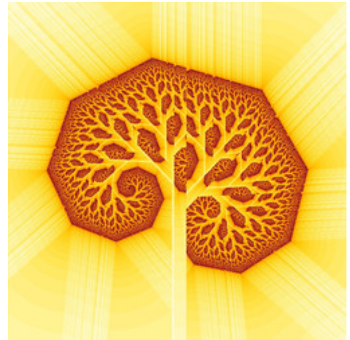
reb-IFSEscape1-06.jpg
