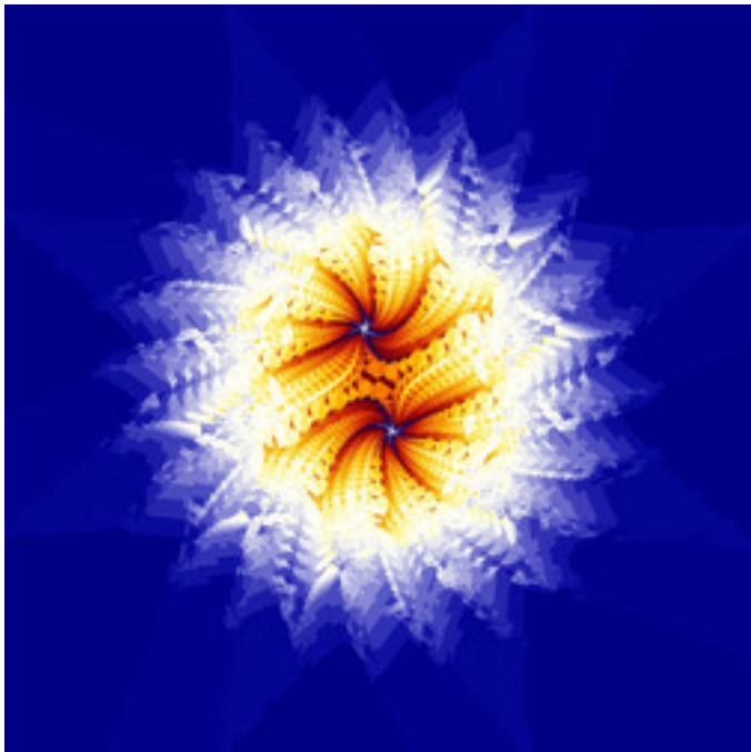
reb-JuliaTentMap-26.jpg
