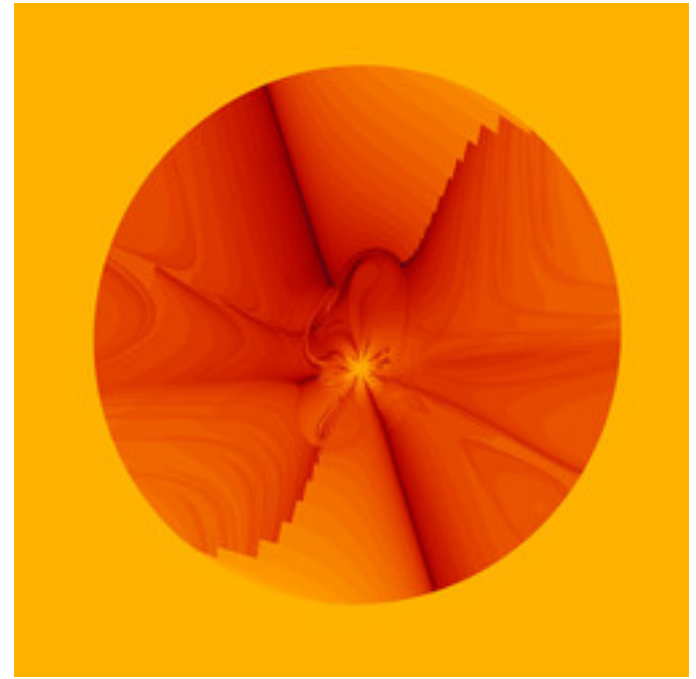
asz-andrexrandom-1-28.jpg
