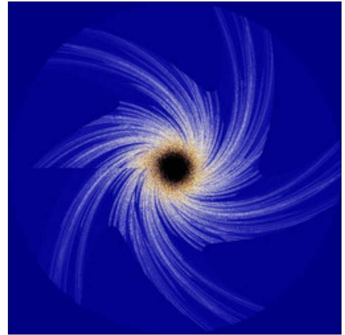
ahm-IndependantPower_03.jpg
