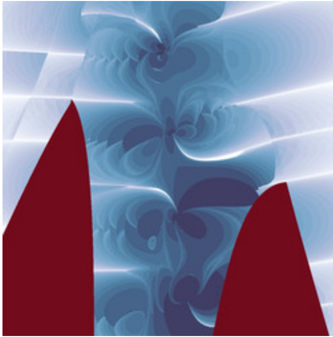
asz-andrextandom-1-11.jpg
