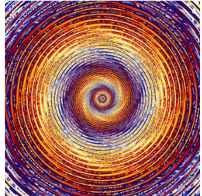
reb-JuliaTentMap-17.jpg
