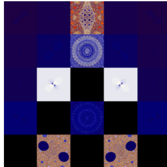
dmj-ManyNova-07.jpg
