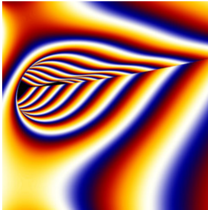
mt-newton-9904a-03.jpg
