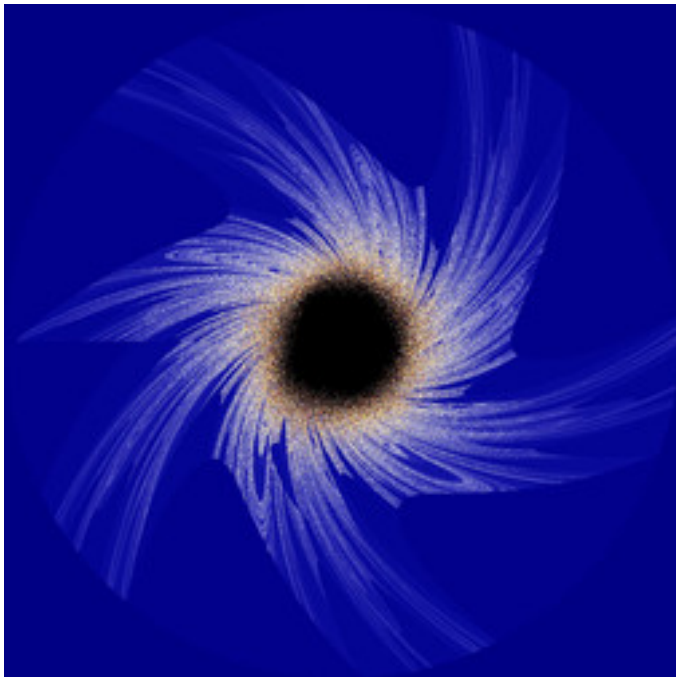
ahm-IndependantPower_02.jpg
