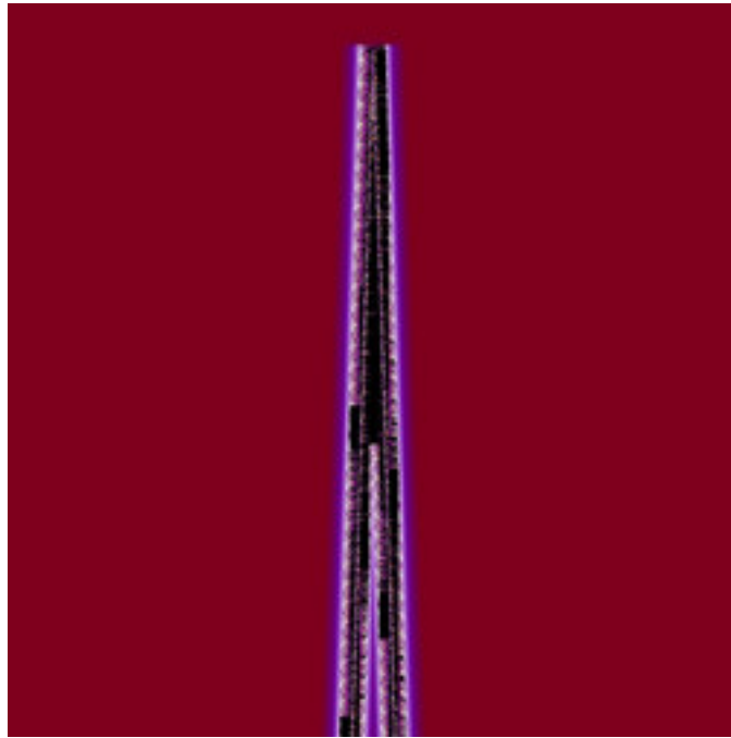
mt-GeneralizedCelticJulia-20.jpg
