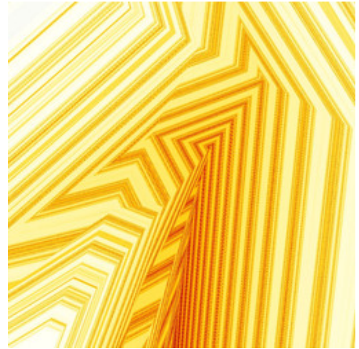
lkm3-MixexupMandelbrot-01.jpg
