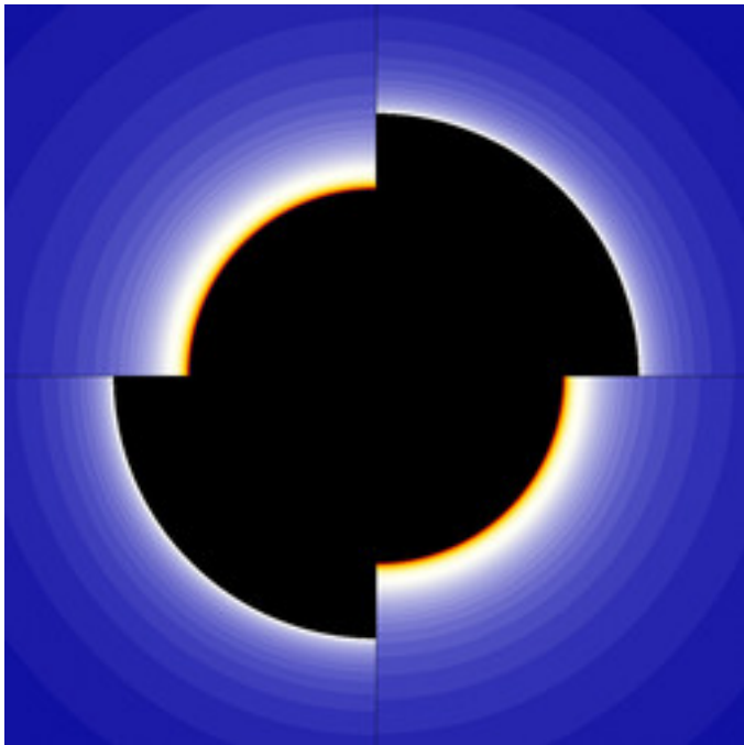
reb-SlopeExpFun_BarnsleyM2-01.jpg
