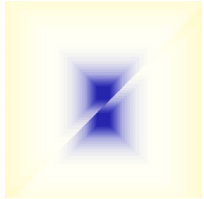
mt-zeepop-julia-23.jpg
