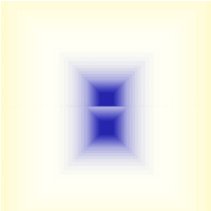
mt-zeepop-julia-22.jpg
