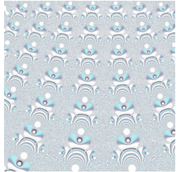
dmj-NovaMandel-08.jpg
