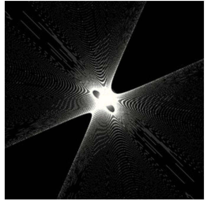
reb-FormulaTracer-06A.jpg
