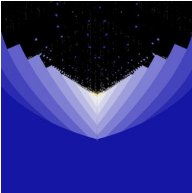
mt-rudys-cubic-mandelbrot-29.jpg
