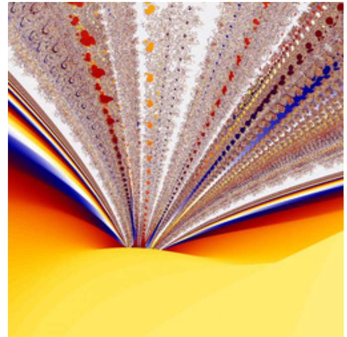
dmj-PhoenixDoubleNova-07.jpg
