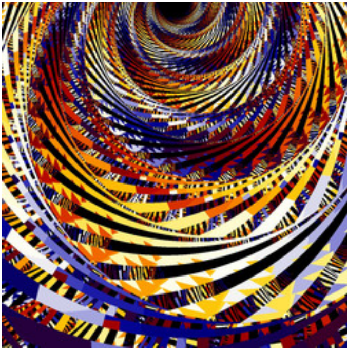
reb-JuliaTentMap-20B.jpg
