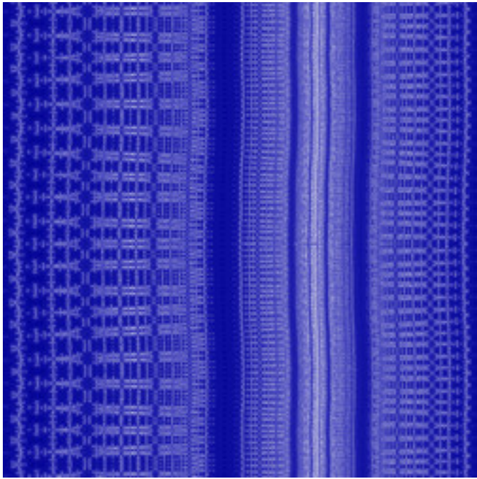
mt-GeneralizedCelticJulia-03.jpg
