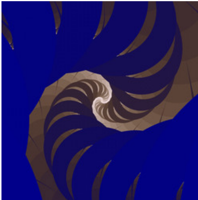
lkm-GapMandelbrot-12.jpg
