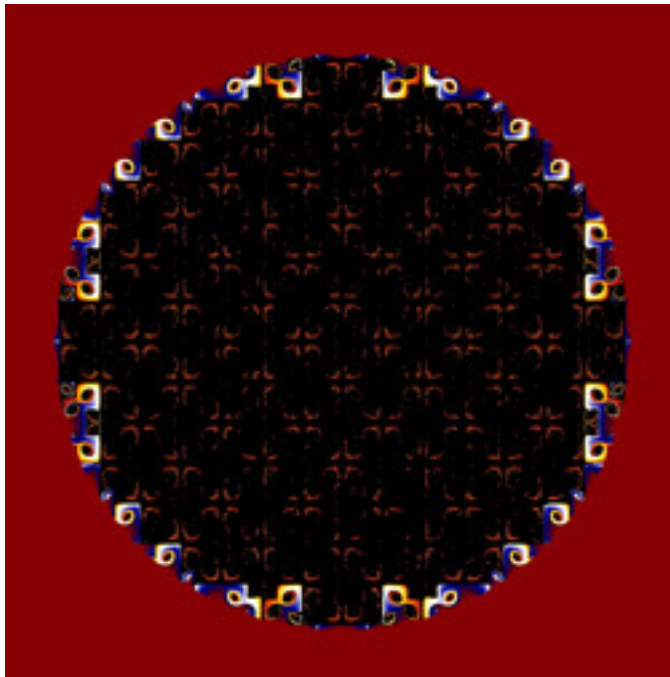
lkm3-FourierPopCorn-04E.jpg
