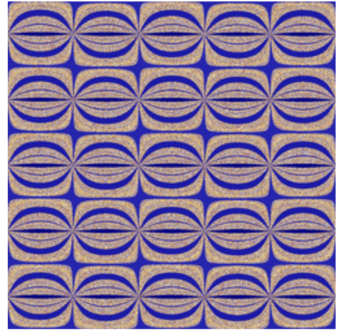
reb-GopalsamyFn-21.jpg
