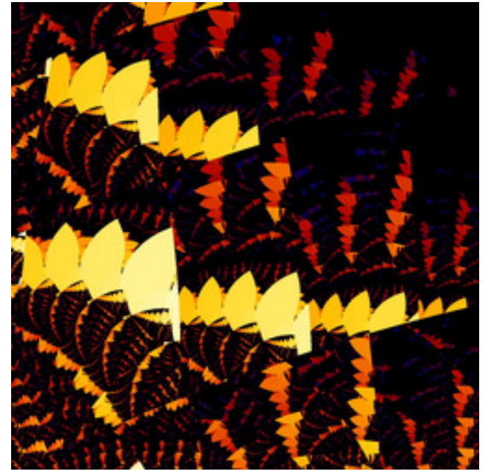
mt-barnsleyishMest-07.jpg
