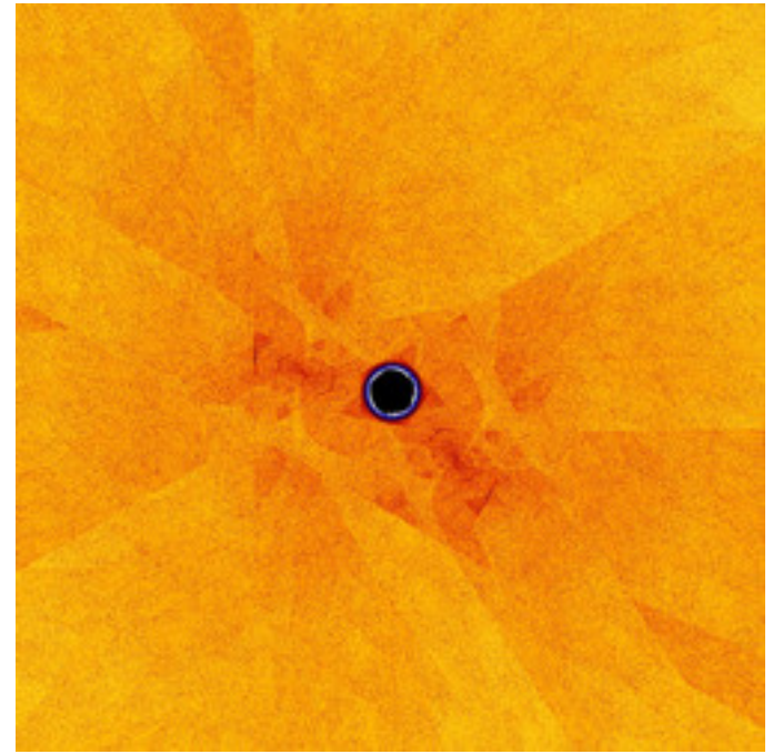
mt-rudys-cubic-julia-03.jpg
