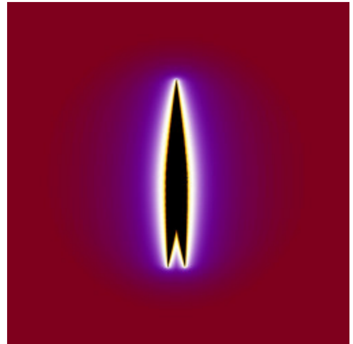
mt-GeneralizedCelticJulia-52.jpg
