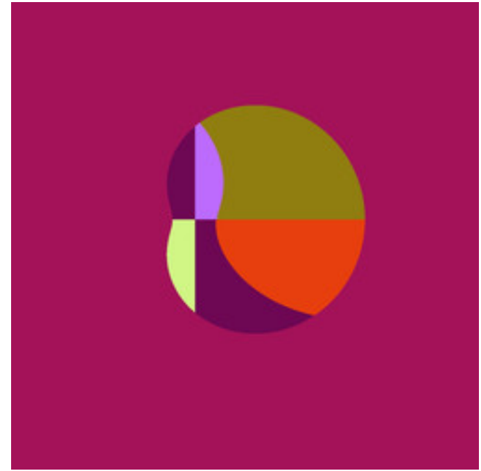
ads-Cantant_01.jpg
