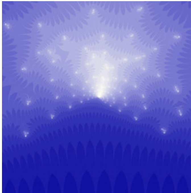
reb-JonHomerSpider-01.jpg
