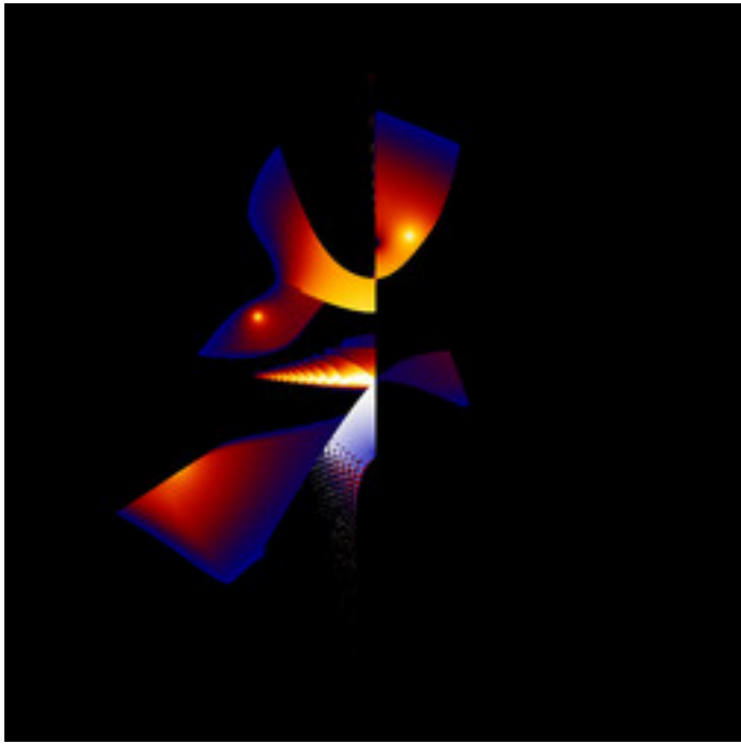
mt-zeepop-mset-42A.jpg
