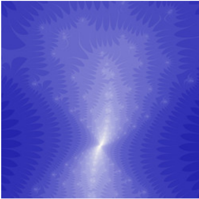
reb-JonHomerSpiderJulia-02.jpg
