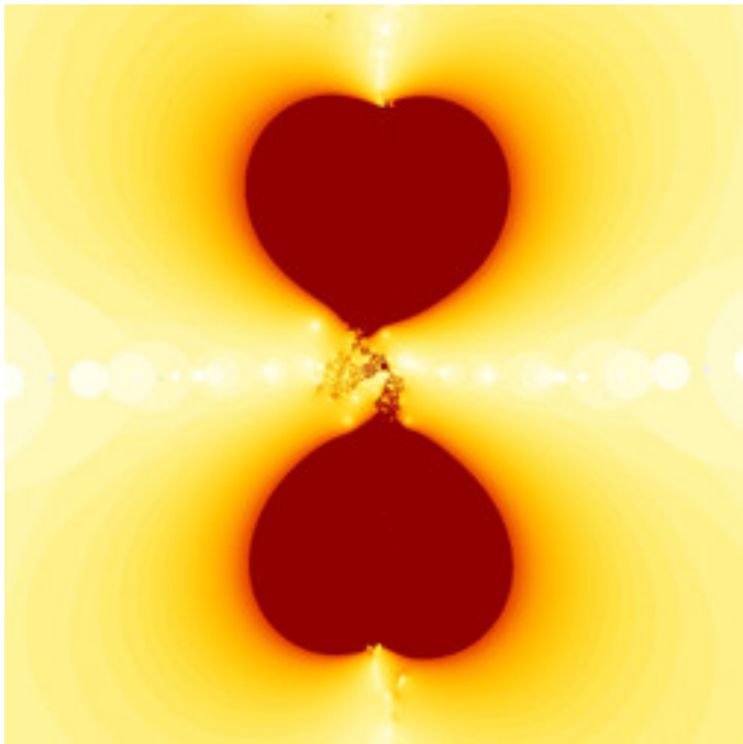
dmj-PhoenixDoubleNova-09a.jpg
