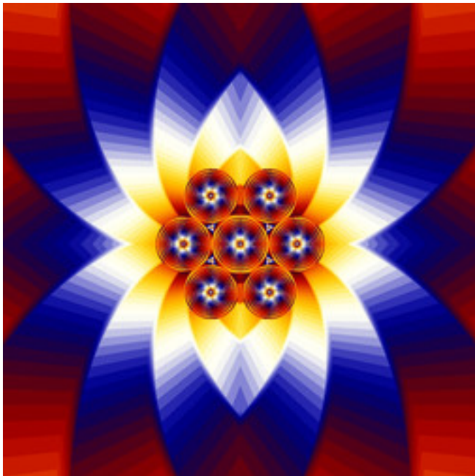
reb-JuliaTentMap-04.jpg
