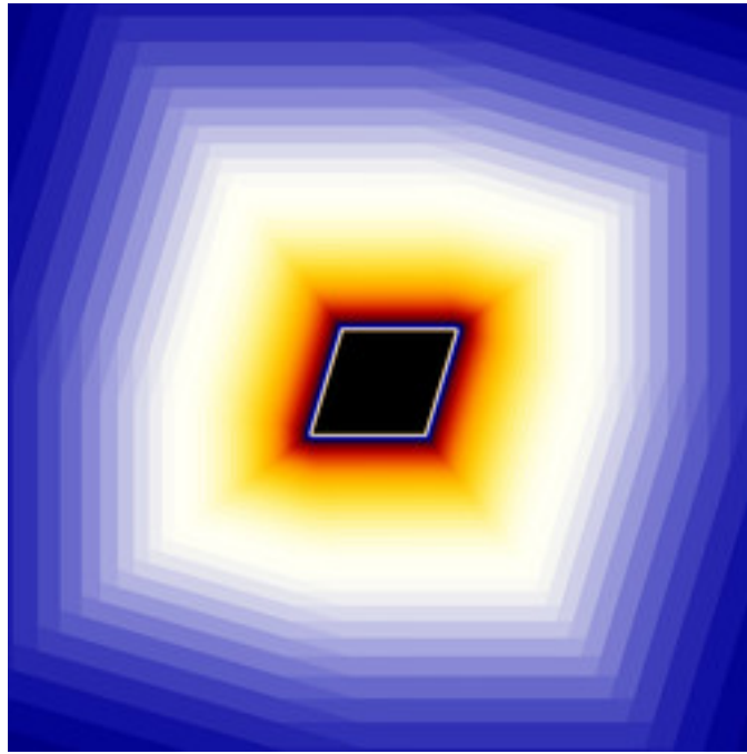
reb-FunBarnsley1Julia-11.jpg
