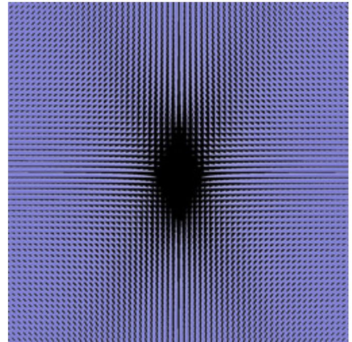
reb-GopalsamyFn-36.jpg
