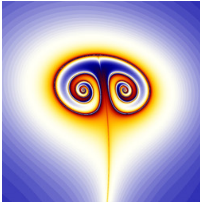
mt-Fractalia1-01.jpg
