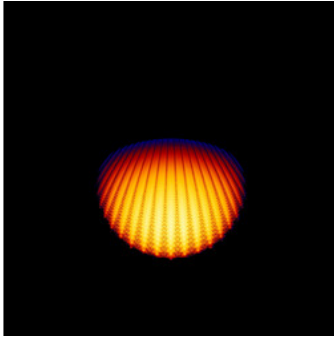
lkm3-BreakingNewton-01.jpg
