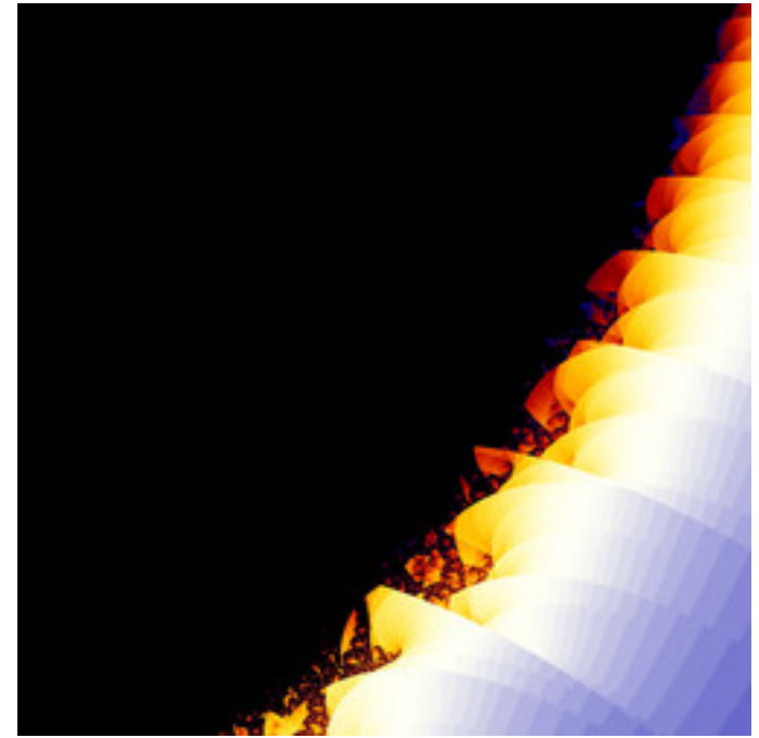
lkm-GeneralTentMandelbrot-10.jpg
