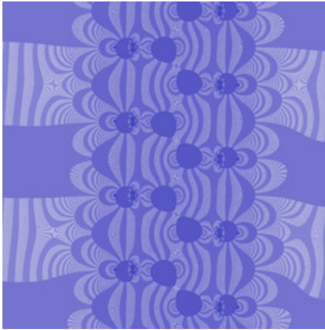
ldm-DM23-102.jpg
