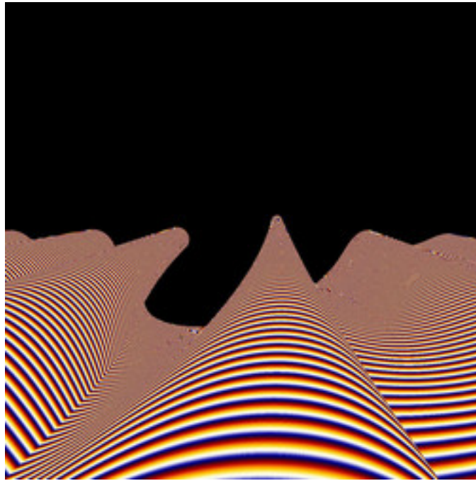
mt-rudys-cubic-mandelbrot-37.jpg
