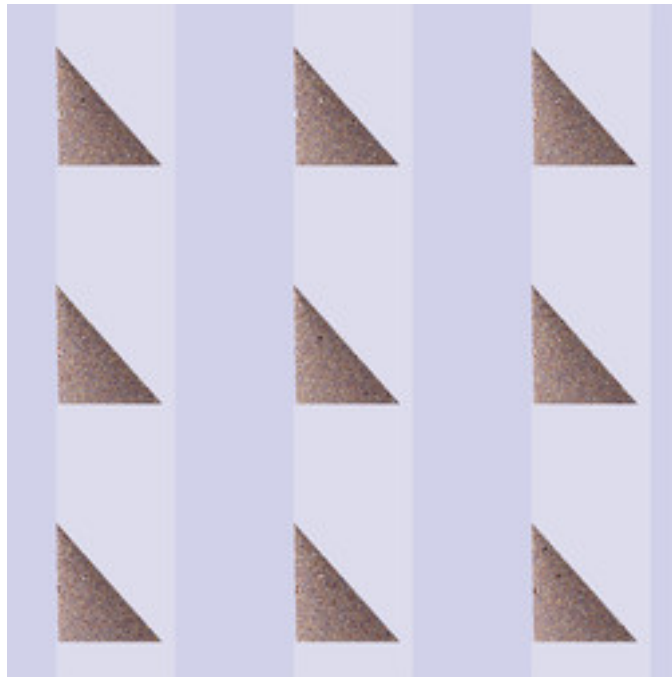
dmj-ManyNova-11.jpg
