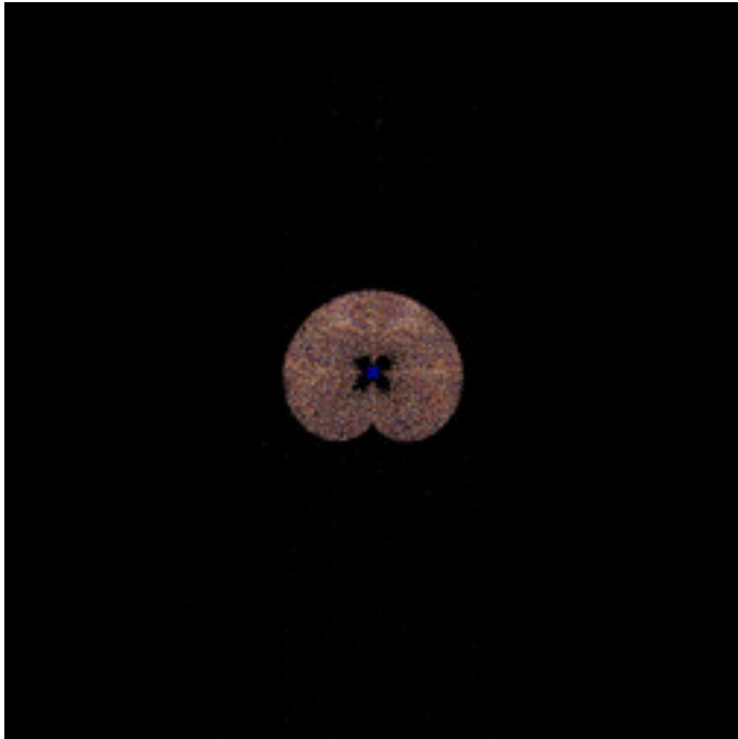
dmj-SimNova-01.jpg
