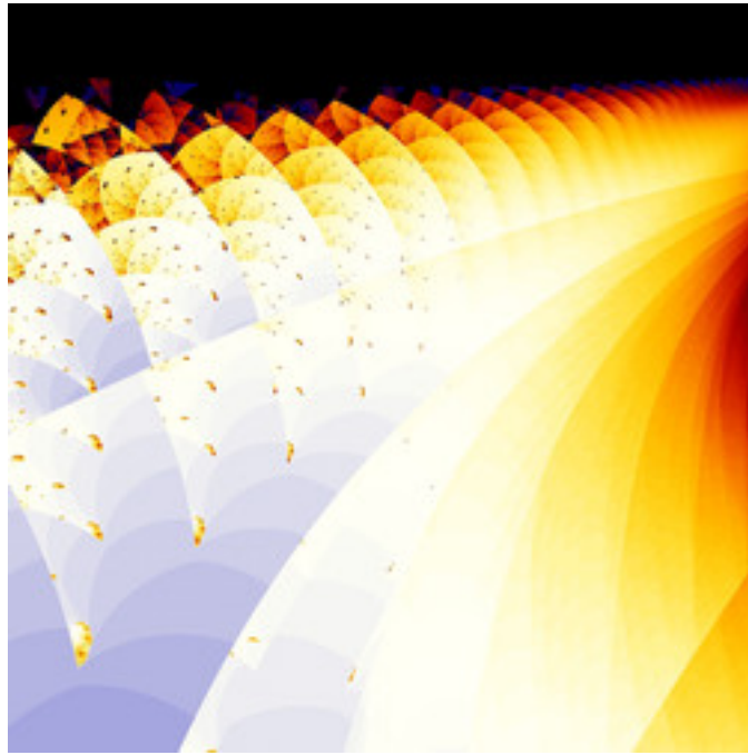
mt-barnsleyishMest-02.jpg
