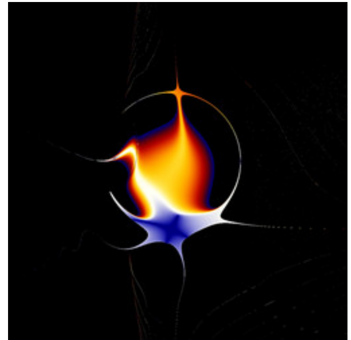
mt-zeepop-mset-20.jpg
