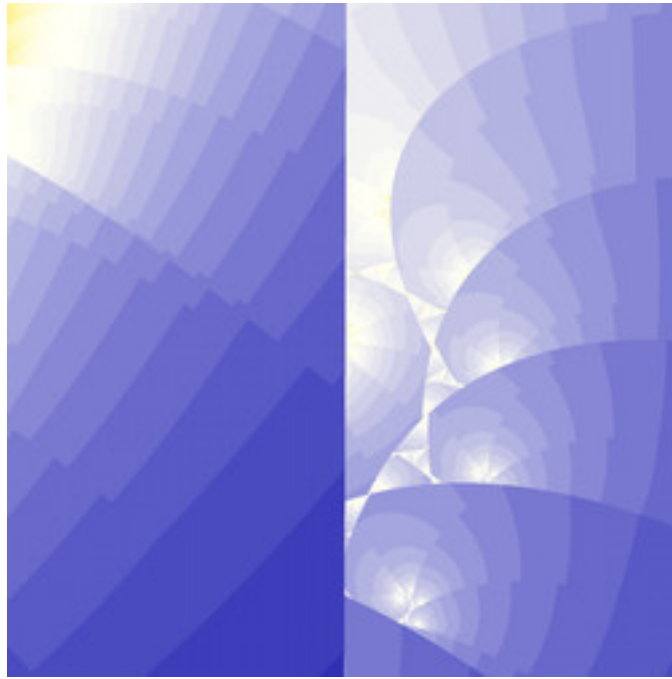
lkm-GeneralTentMandelbrot-11.jpg
