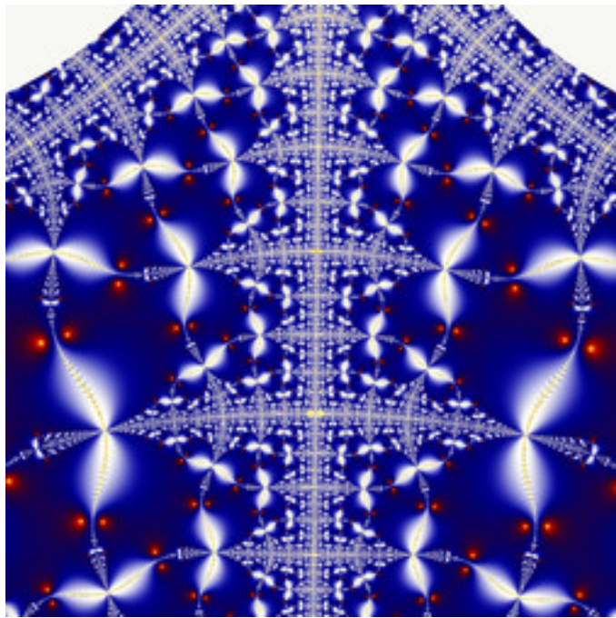
dmj-NovaMandel-04.jpg
