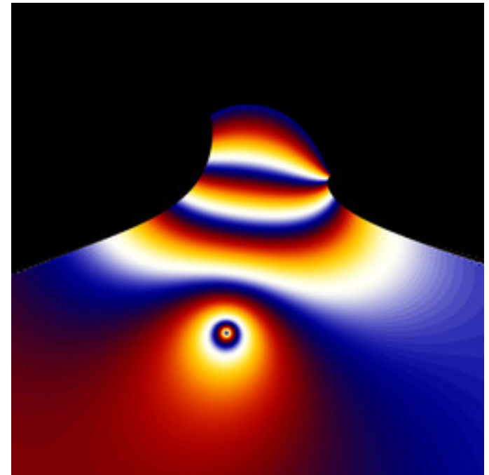
mt-newton-error-17b.jpg
