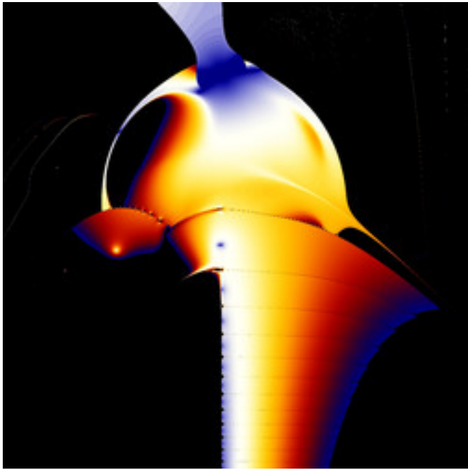
mt-zeepop-mset-13.jpg
