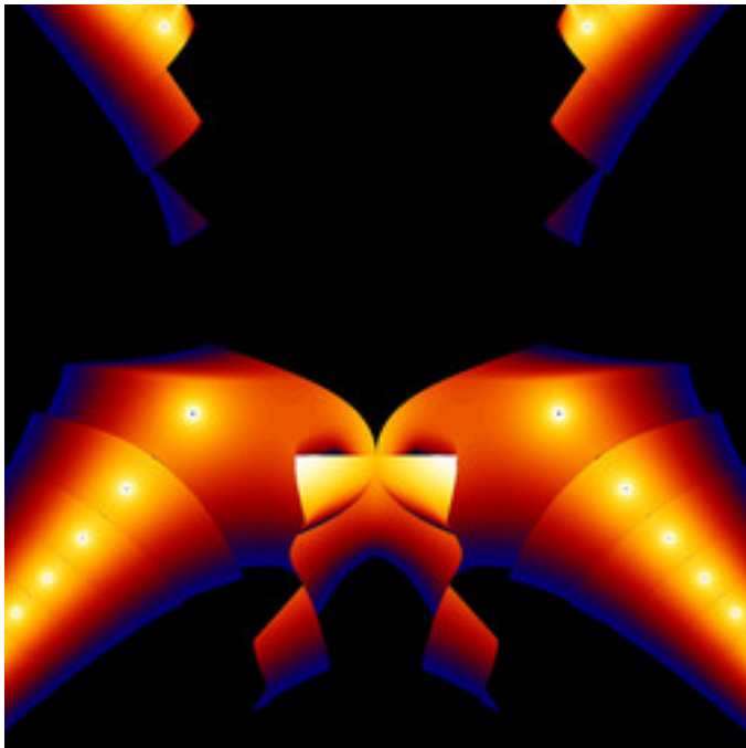
mt-zeepop-mset-28.jpg
