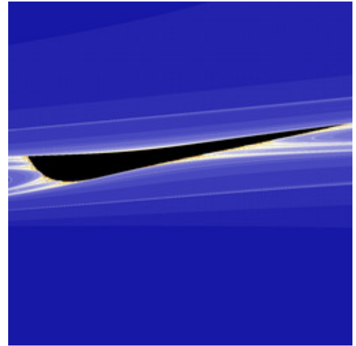
mt-bifunctionalMset-05.jpg
