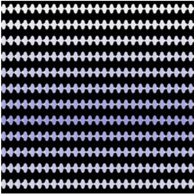
mt-zeepop-julia-25.jpg
