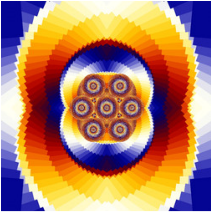
reb-JuliaTentMap-07.jpg
