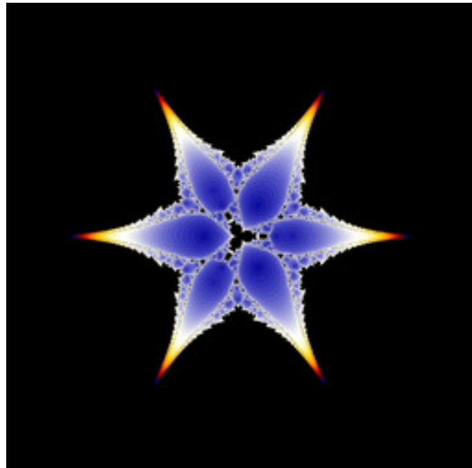
mt-secant-I-03.jpg
