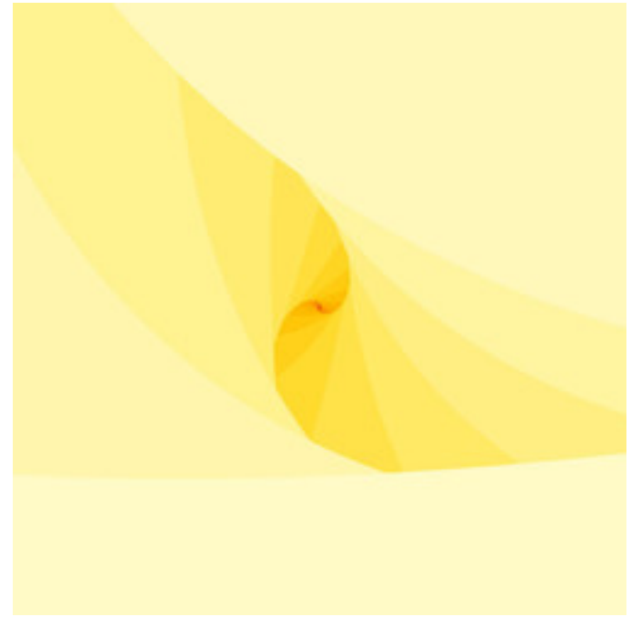
mt-990807bMset-23.jpg
