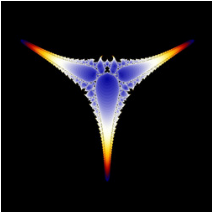
mt-secant-I-04.jpg
