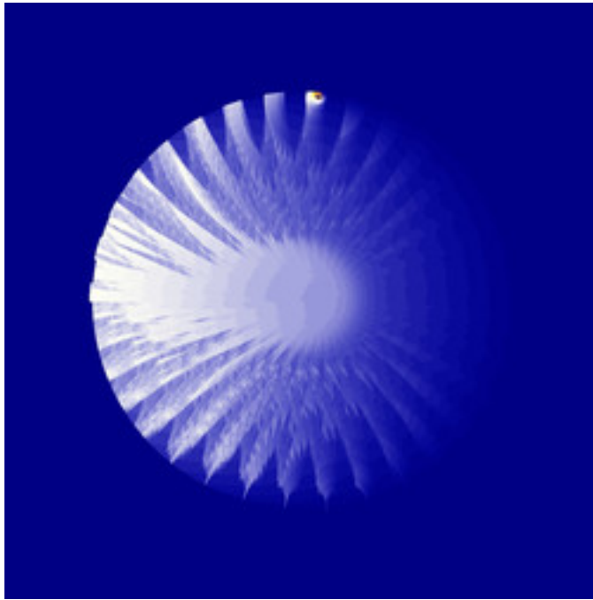
reb-PseudoZeePi-02.jpg
