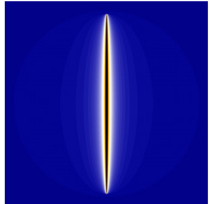
mt-bifunctionalMset-08.jpg
