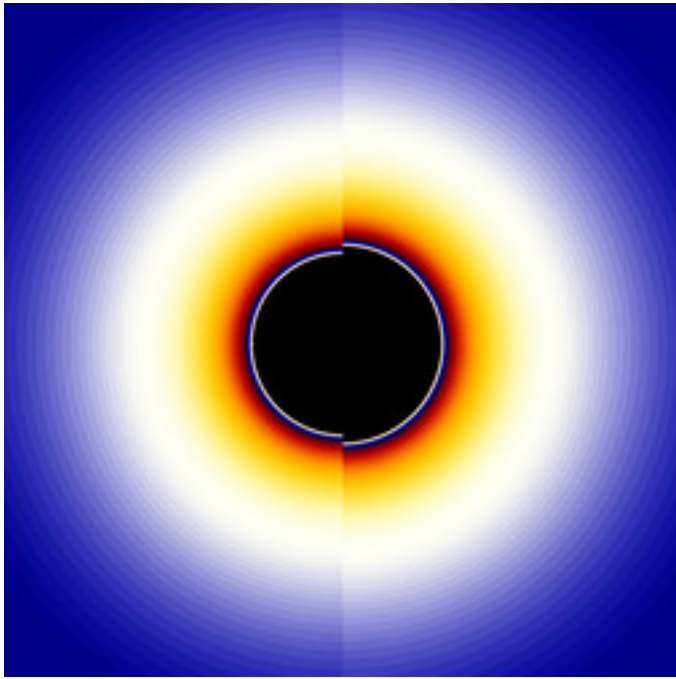
reb-FunBarnsley1Julia-12.jpg
