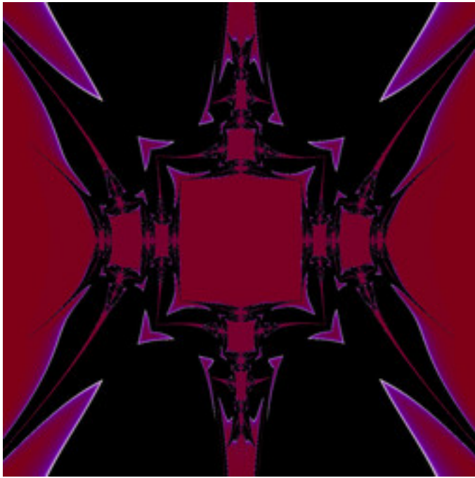
mt-GeneralizedCelticJulia-09.jpg
