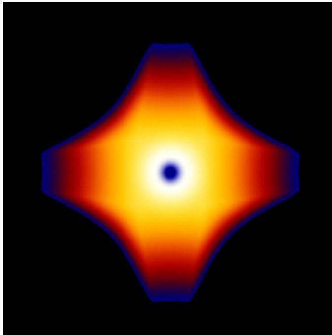
mt-zeepop-mset-39.jpg
