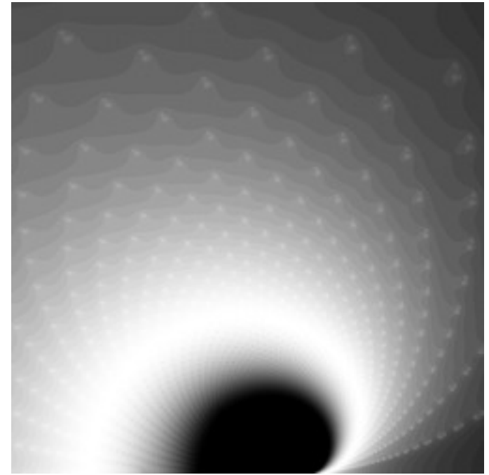
mt-modulate-mset-05.jpg
