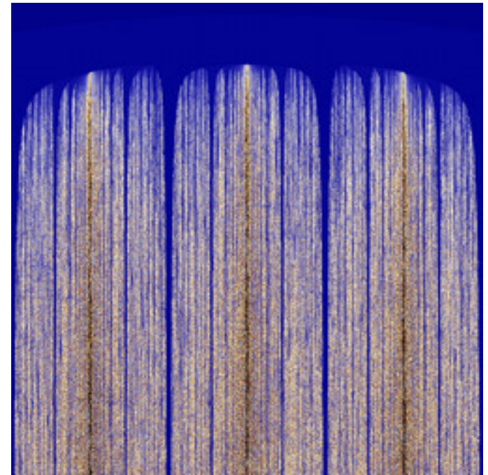
mt-bifunctionalMset-14.jpg
