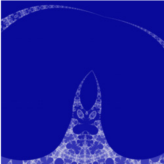
ldm-DM23-04.jpg
