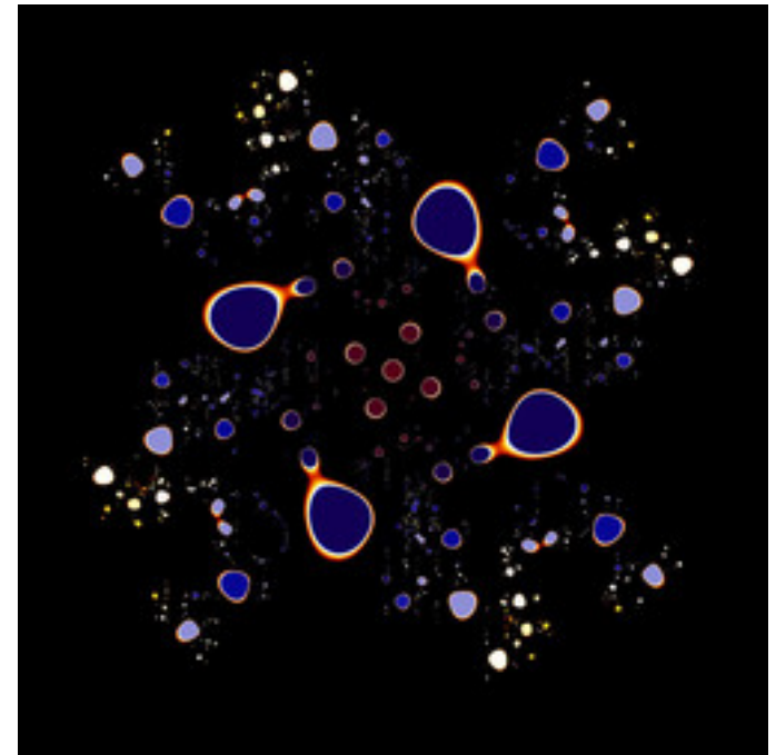
mt-rudys-cubic-mandelbrot-15.jpg
