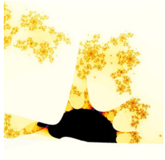
mt-990807aMset-15.jpg
