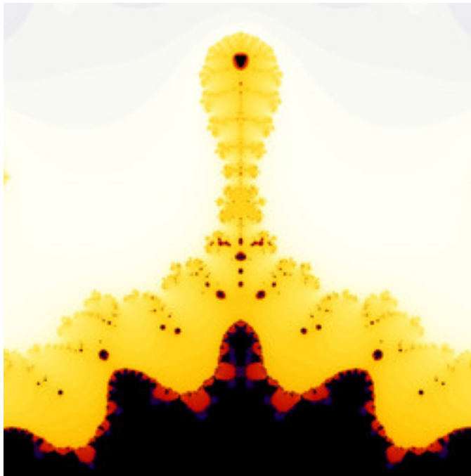
mt-modulate-mset-03.jpg
