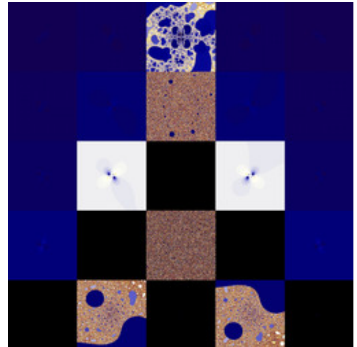
dmj-ManyNova-10.jpg
