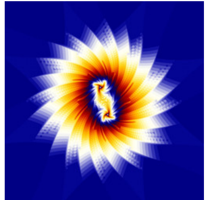
reb-JuliaTentMap-24.jpg
