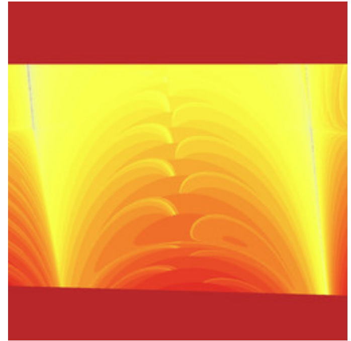
asz-andrextrandom-1-04.jpg
