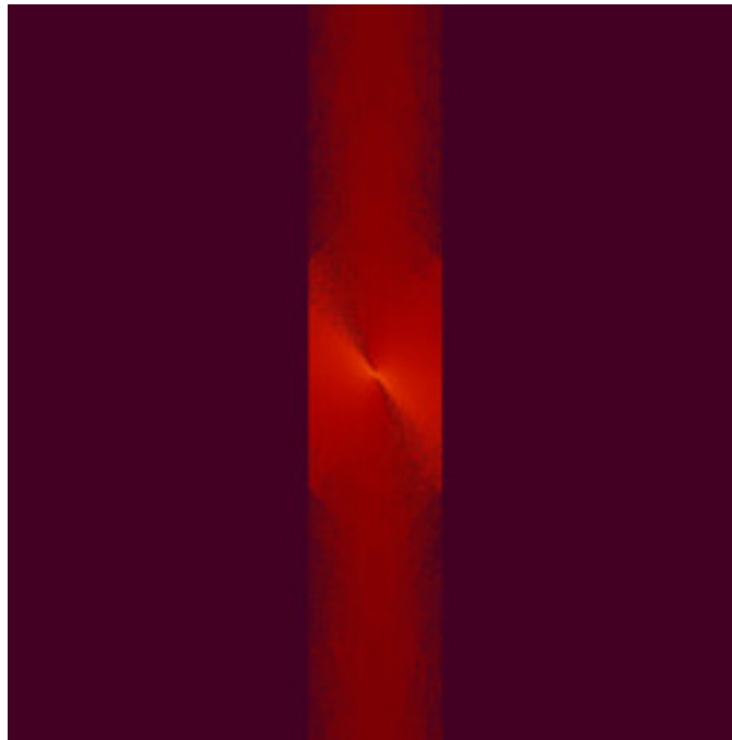
mt-newton-twist-07.jpg
