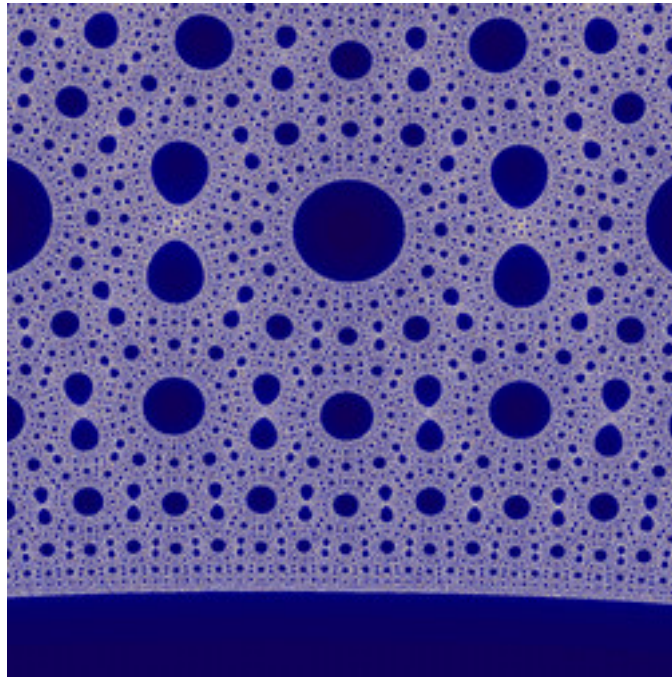
lkm-MitchsMandelbrot-02.jpg
