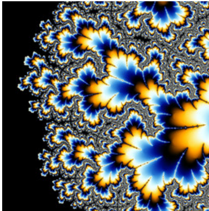
standard-FastMandel-06.jpg
