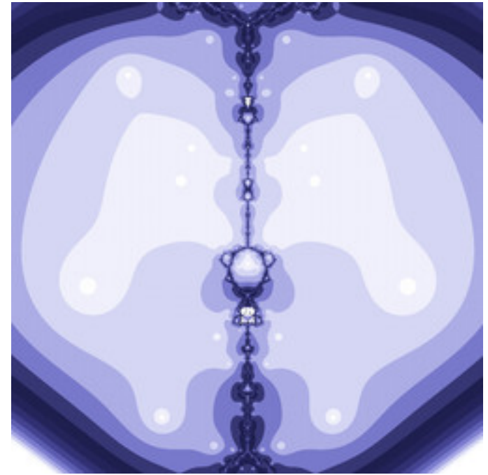
dmj-DoubleHalleyNova-02.jpg
