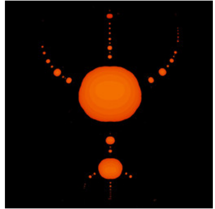
Ikm3-ExtraFoam-07.jpg
