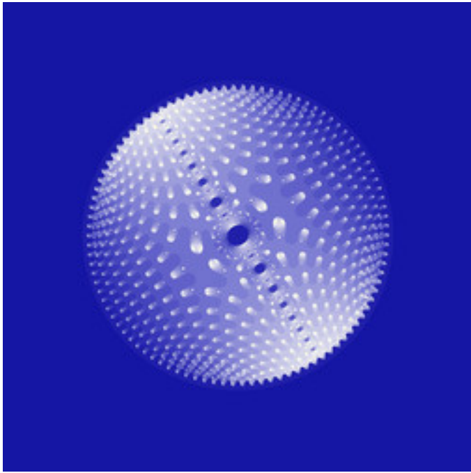
mt-pseudo-magnet-julia-04.jpg
