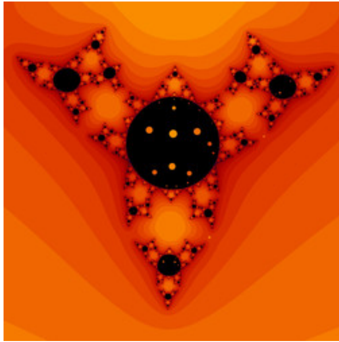
Ikm3-AlternativeFunctions-06.jpg
