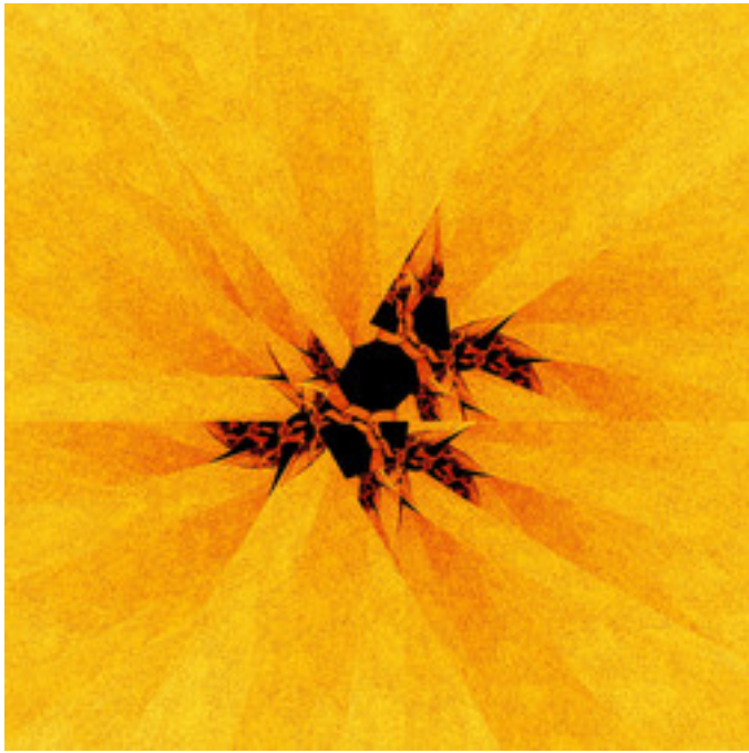
mt-rudys-cubic-julia-05.jpg
