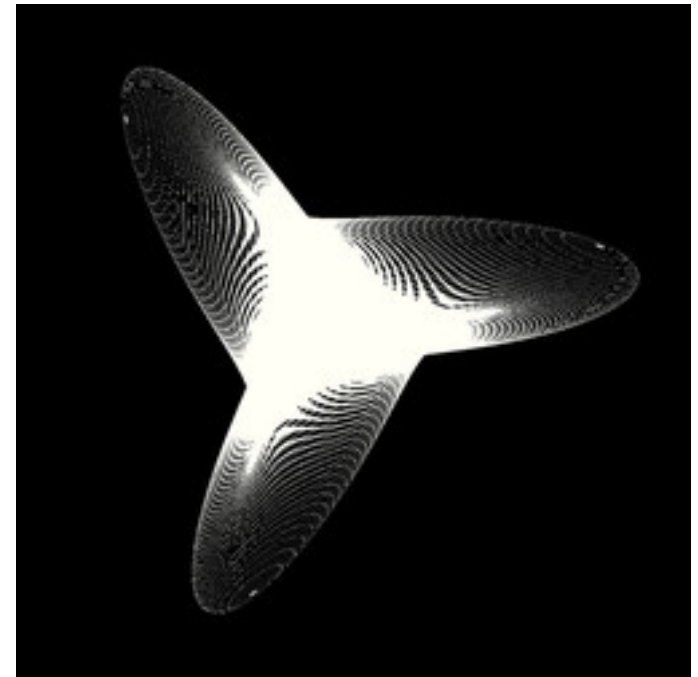
reb-FormulaTracer-03A.jpg
