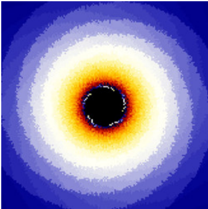
reb-FunBarnsley1Julia-09B.jpg
