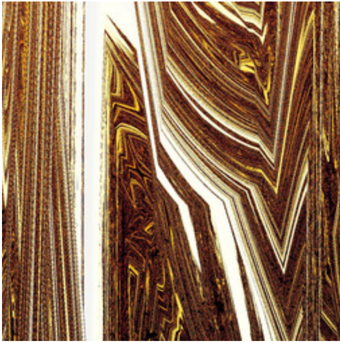
lkm3-MixexupMandelbrot-03.jpg
