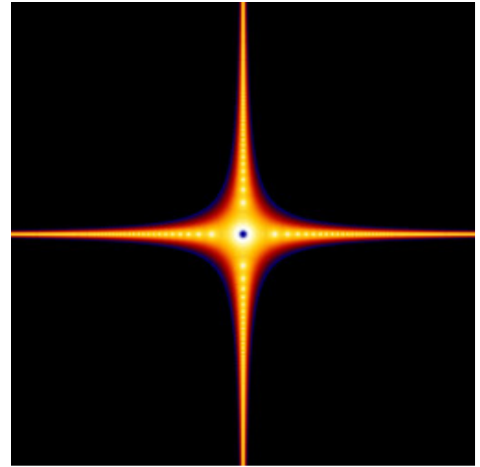
mt-zeepop-mset-17.jpg
