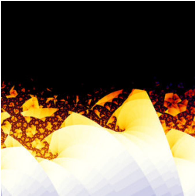
lkm-GeneralTentMandelbrot-04.jpg
