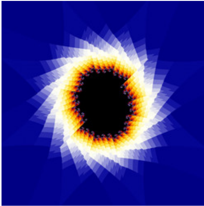
reb-JuliaTentMap-28.jpg
