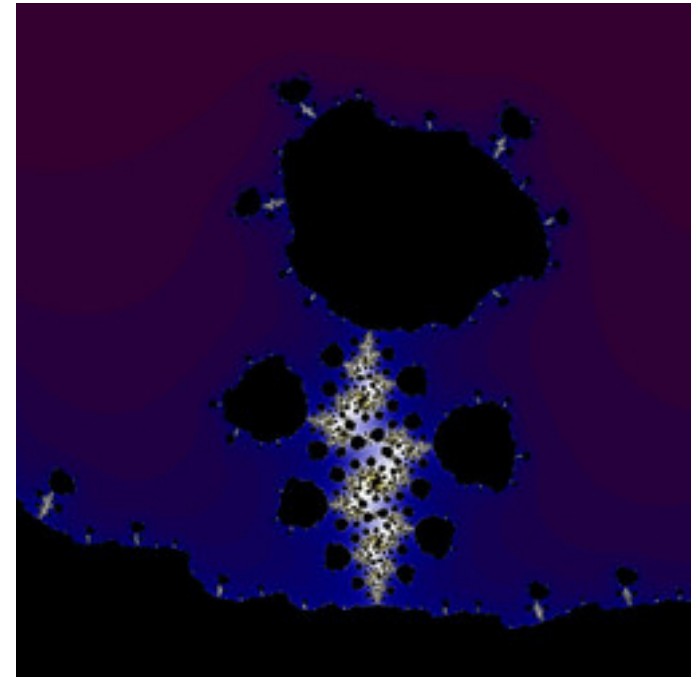
mt-990807aMset-05.jpg
