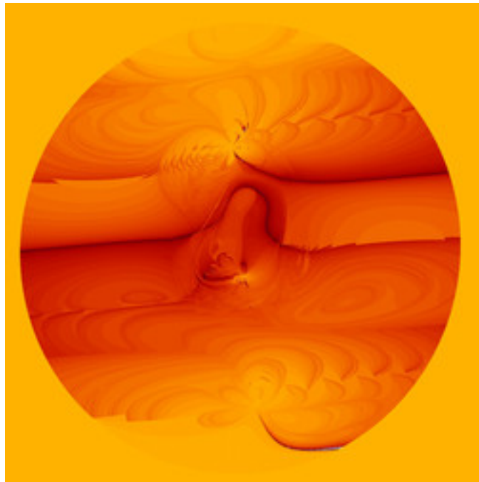
asz-andrextrandom-1-20.jpg
