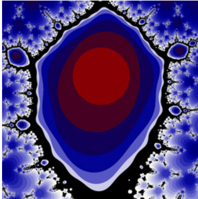
lkm3-AlternativeFunctions-09.jpg
