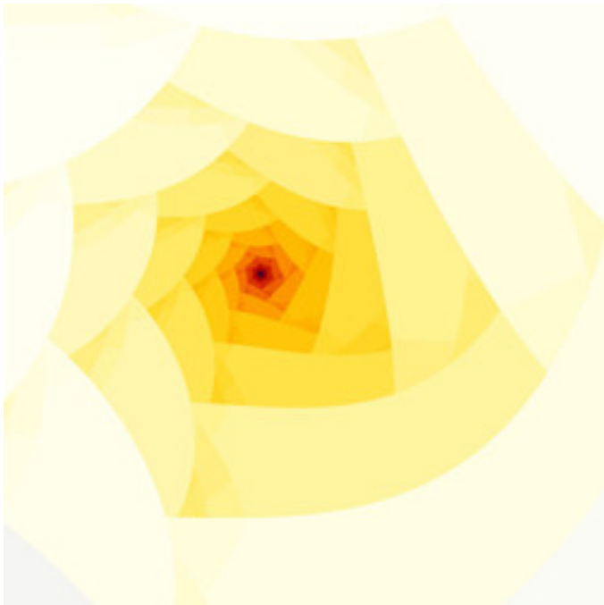
mt-rudys-cubic-mandelbrot-35.jpg
