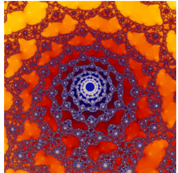
dmj-DoubleNova-01.jpg
