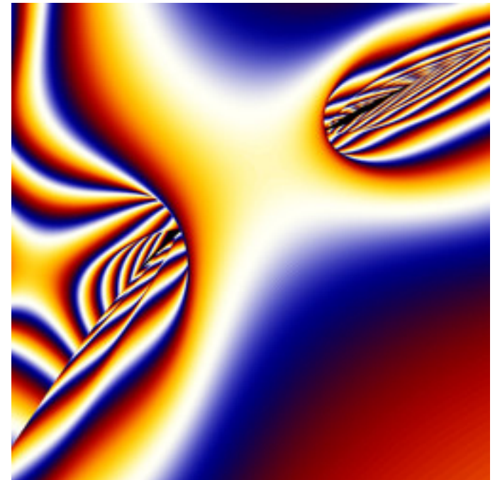
mt-BofNewton1-04.jpg
