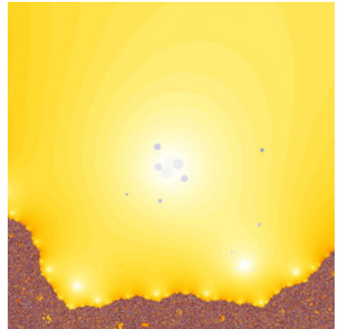
dmj-PhoenixDoubleNova-01.jpg
