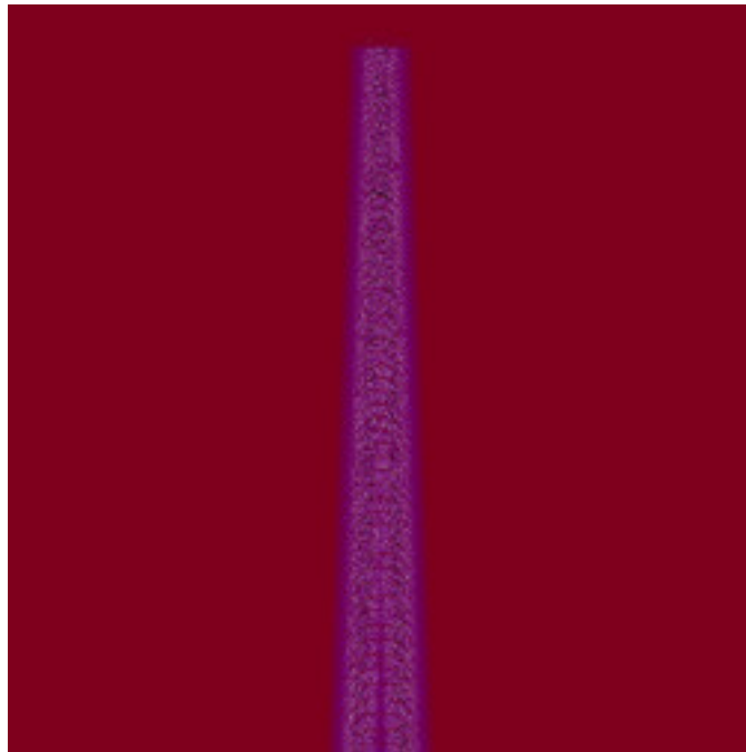
mt-GeneralizedCelticJulia-17.jpg
