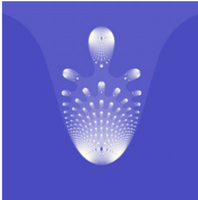
mt-pseudo-magnet-julia-06.jpg
