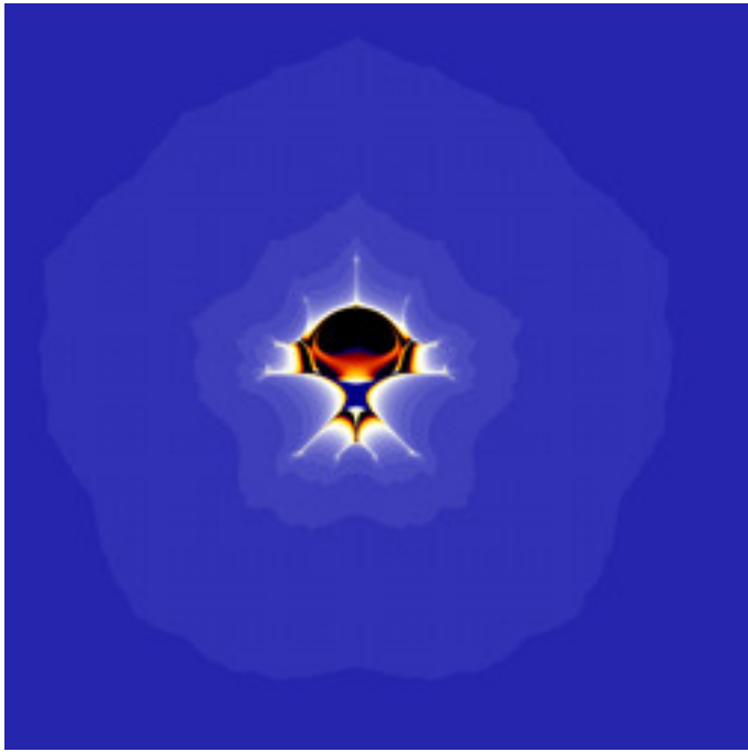
mt-zeepop-mset-54.jpg
