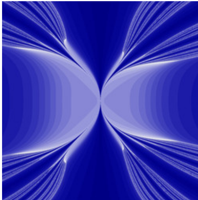
reb-GopalsamyFn-31.jpg
