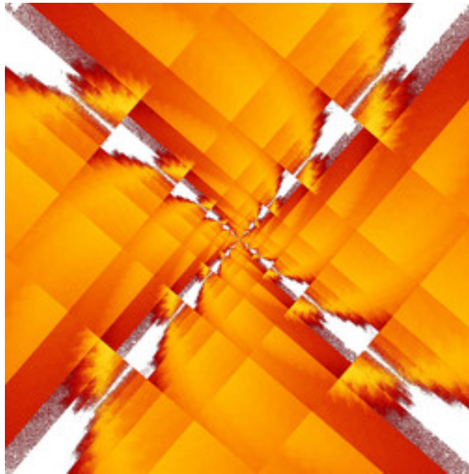
dmj-NovaMandel-100.jpg
