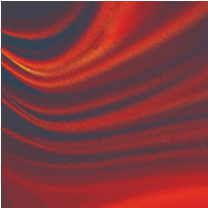
asz-andrextrandom-1-02.jpg
