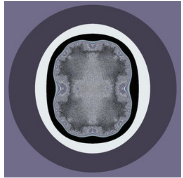
mt-magnetism-model-ii-julia-05.jpg
