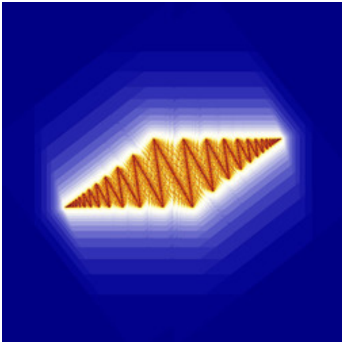
reb-FunBarnsley1Julia-05C.jpg
