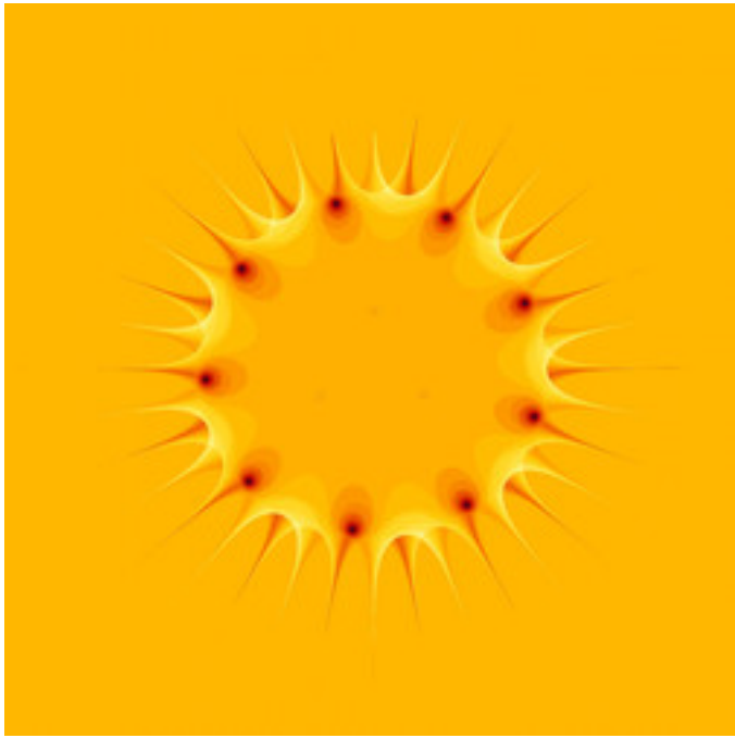
mt-rudys-cubic-julia-11.jpg
