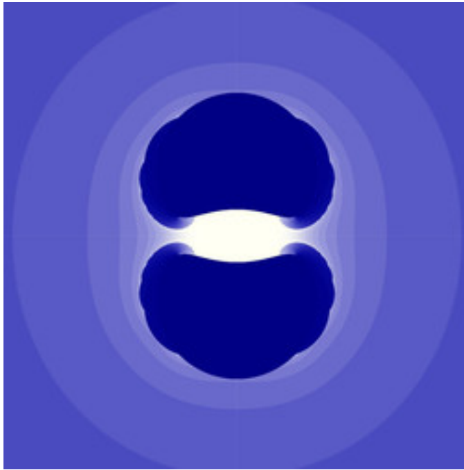
ahm-MonotonicGrowthJulia_01.jpg
