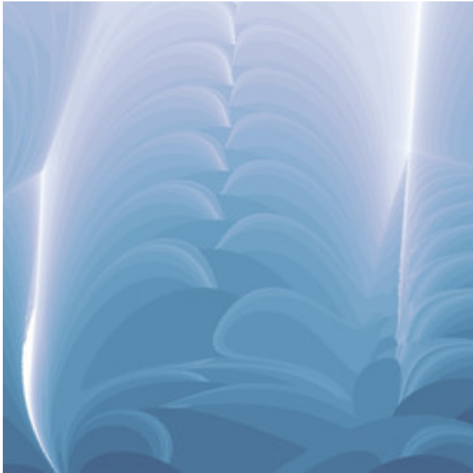
asz-andrextandom-1-09.jpg
