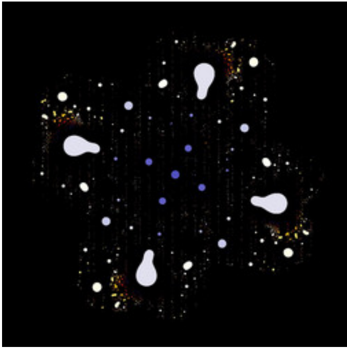
mt-rudys-cubic-mandelbrot-14.jpg
