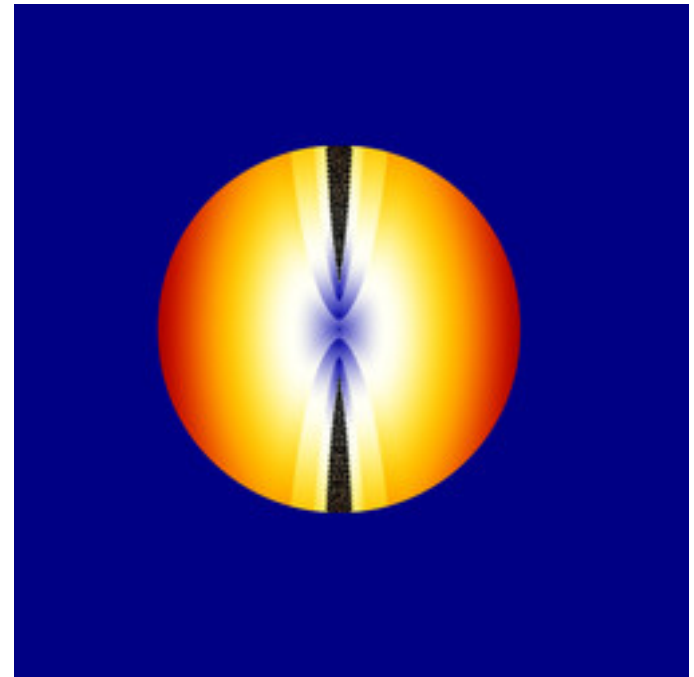
mt-zeepop-julia-02.jpg
