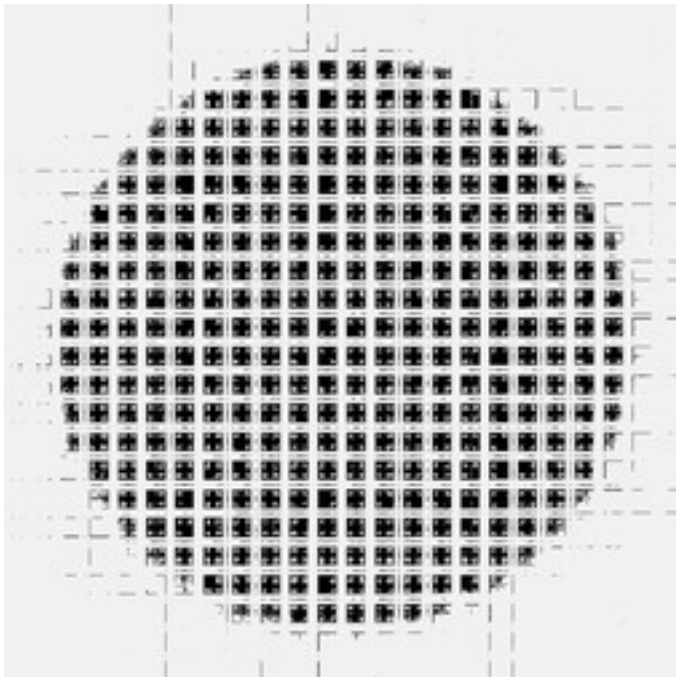
lkm3-FourierPopCorn-11.jpg
