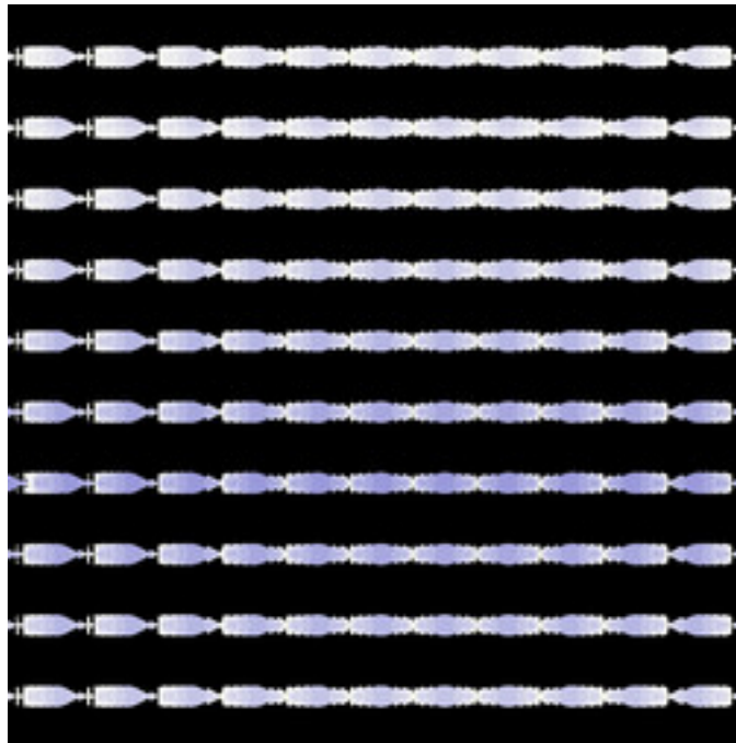
mt-zeepop-julia-27.jpg
