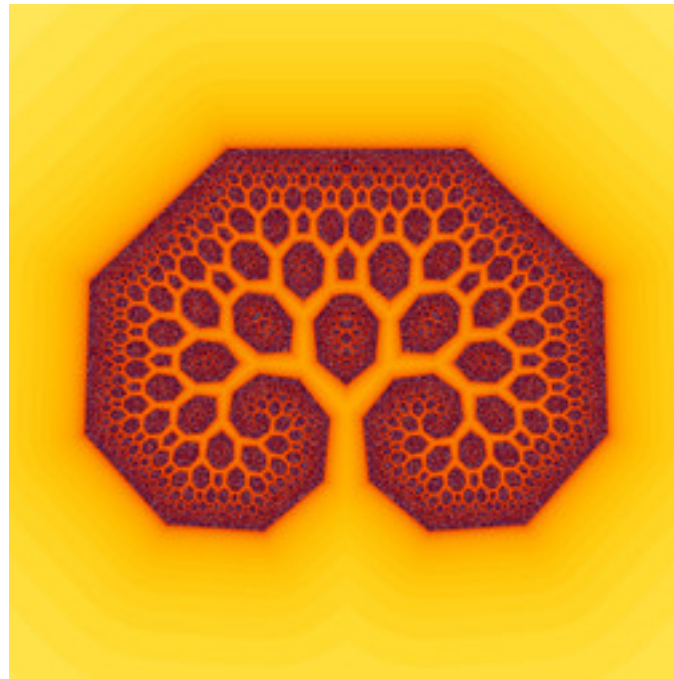
reb-IFSEscape1-01.jpg
