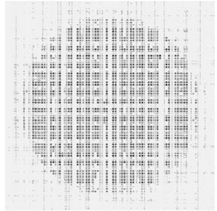
lkm3-FourierPopCorn-12.jpg
