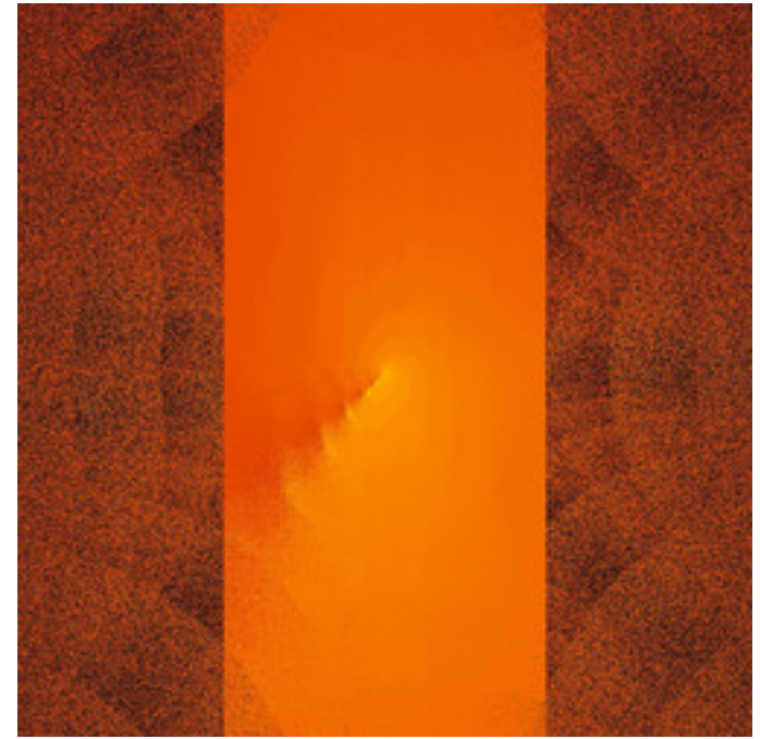
mt-newton-twist-03.jpg
