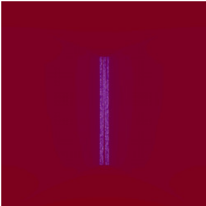
mt-GeneralizedCelticJulia-06.jpg
