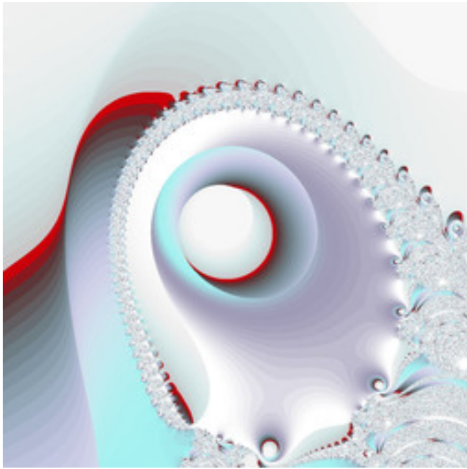
dmj-NovaMandel-10.jpg
