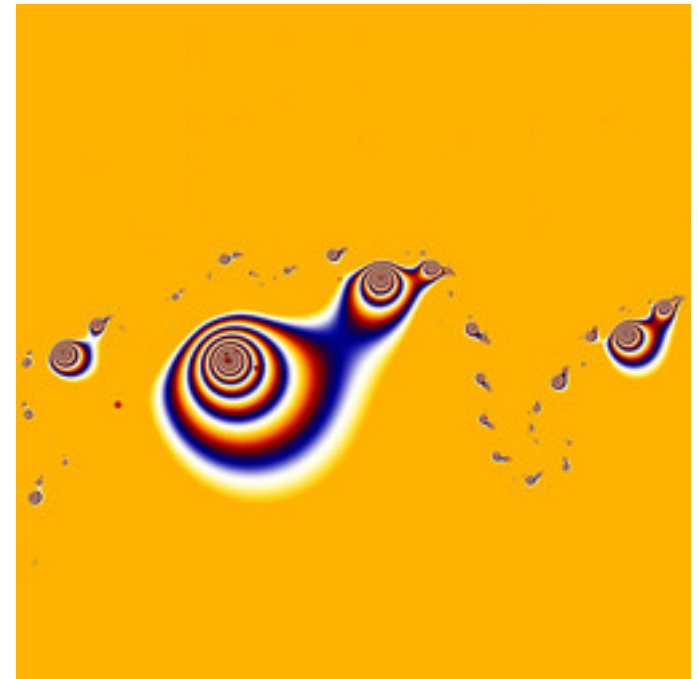
dmj-PhoenixDoubleNova-25.jpg
