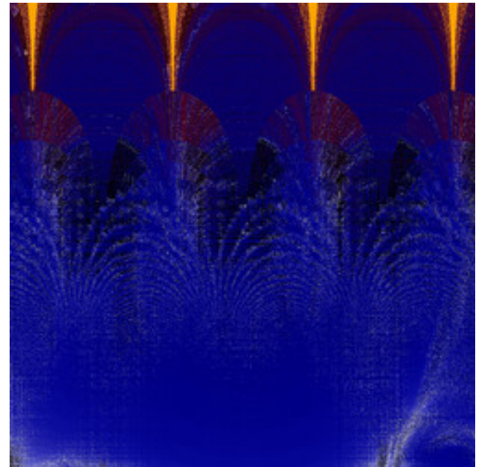
mt-secant-I-02.jpg
