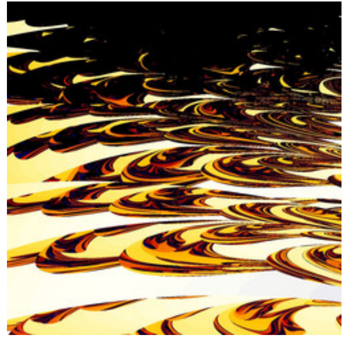
mt-990807aMset-27.jpg
