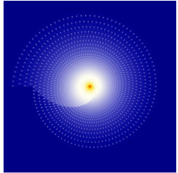
reb-LambdaPower-02.jpg
