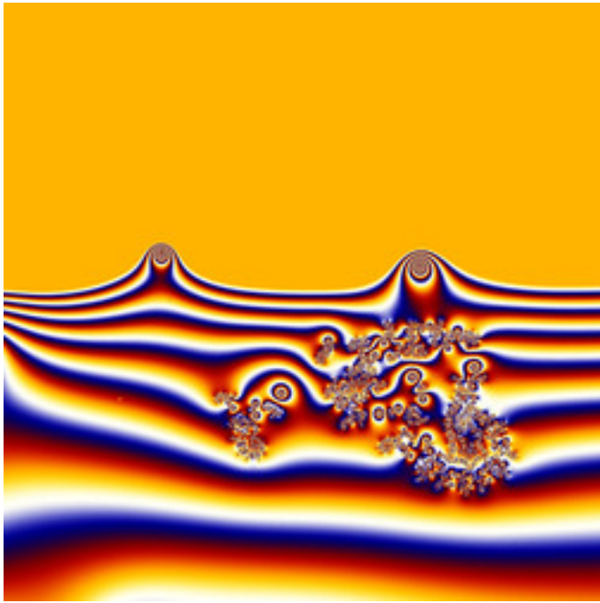
dmj-PhoenixDoubleNova-18.jpg
