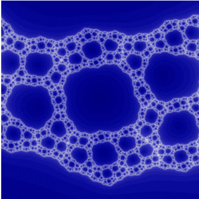
lkm-MitchsMandelbrot-06.jpg
