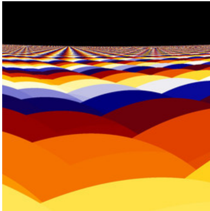
mt-rudys-cubic-mandelbrot-34.jpg
