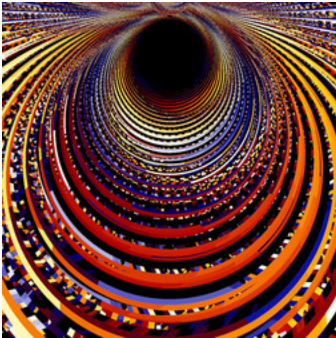
reb-JuliaTentMap-21A.jpg
