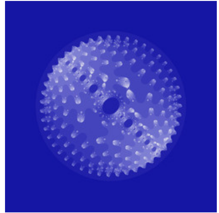
mt-pseudo-magnet-julia-02.jpg
