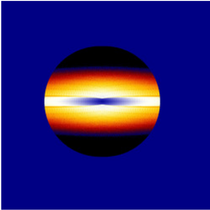
mt-zeepop-julia-07.jpg
