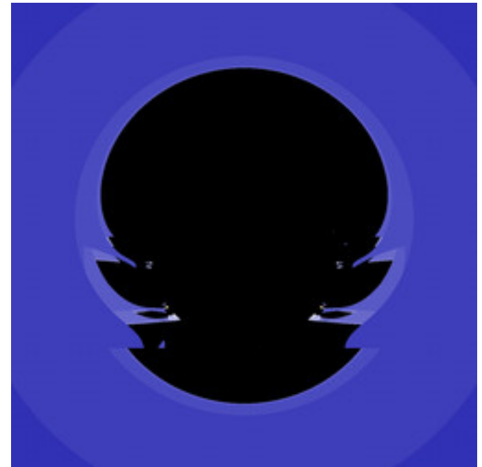
mt-barnsleyishMest-16.jpg
