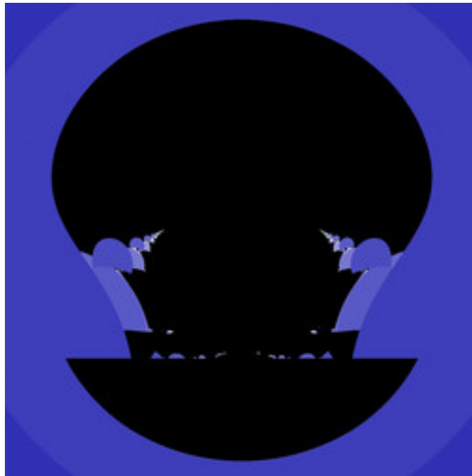
mt-barnsleyishMest-17.jpg
