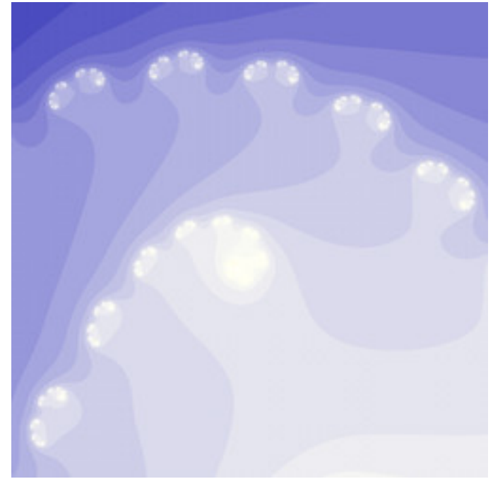
lkm-CompundingTM-09.jpg
