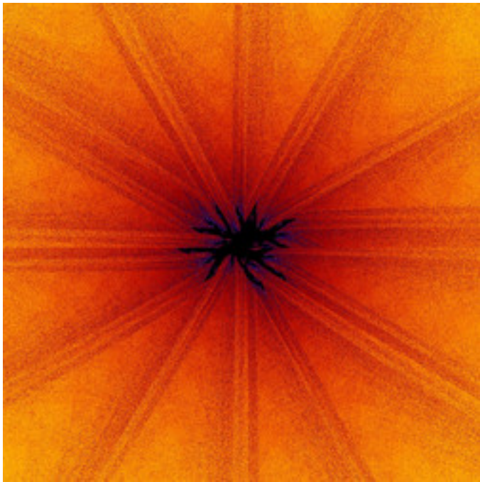
mt-rudys-cubic-julia-08.jpg
