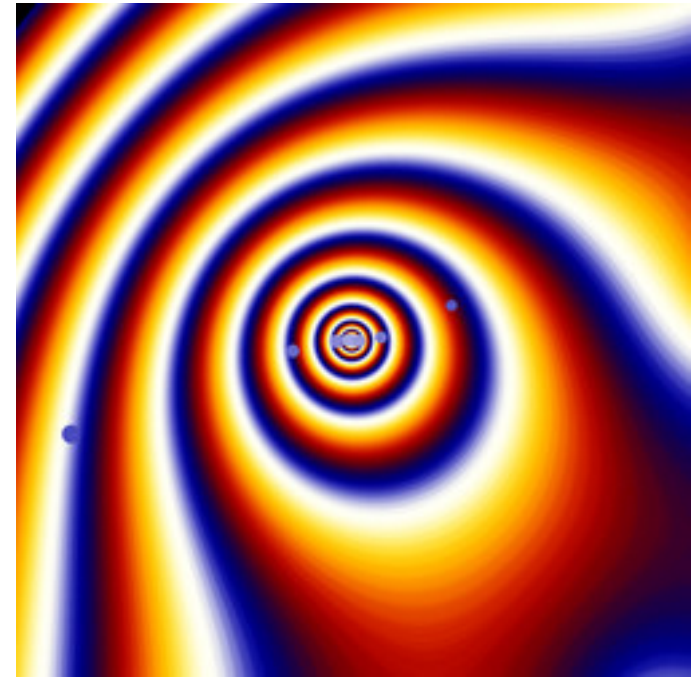
dmj-PhoenixDoubleNova-04.jpg
