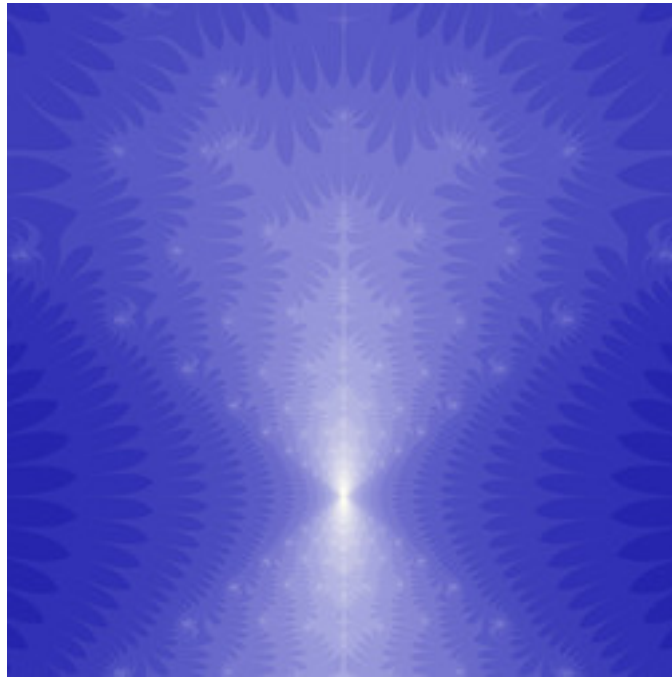
reb-JonHomerSpiderJulia-01.jpg
