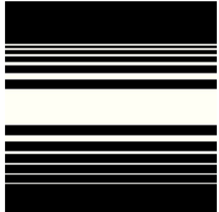
reb-FormulaTracer-12A.jpg
