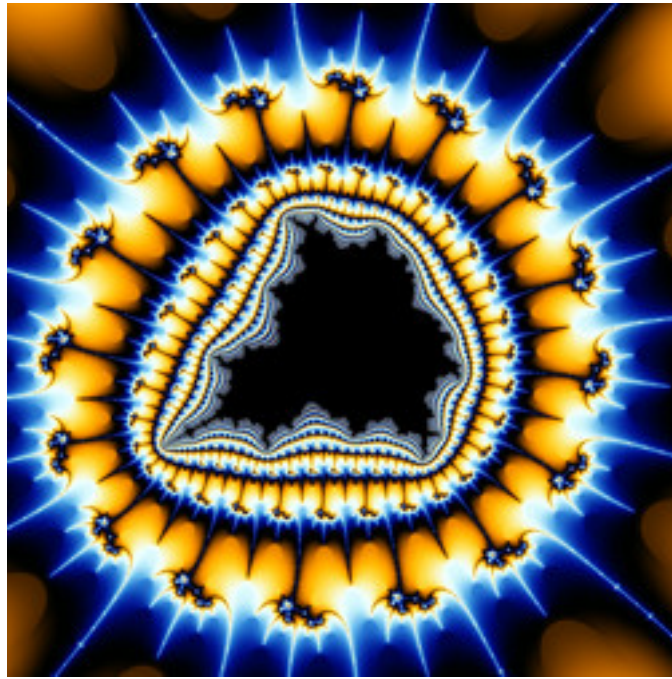
standard-FastMandel-03.jpg
