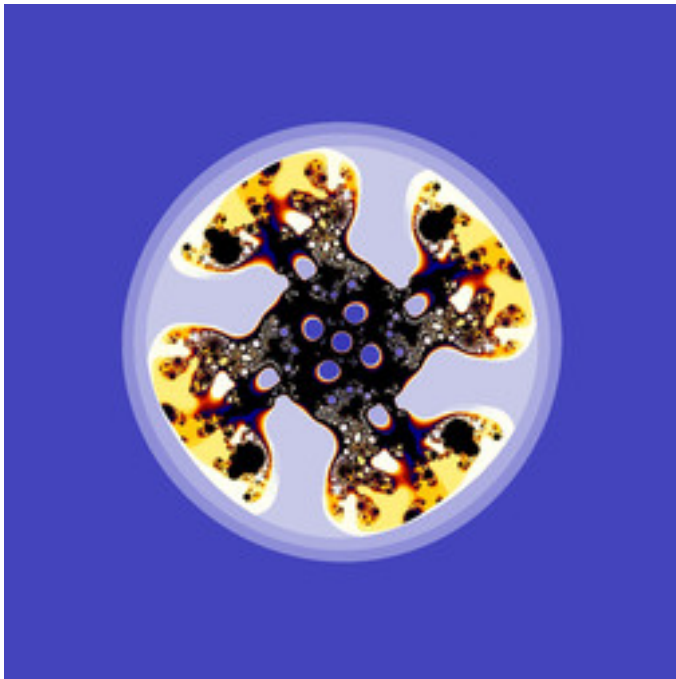
mt-rudys-cubic-mandelbrot-17.jpg
