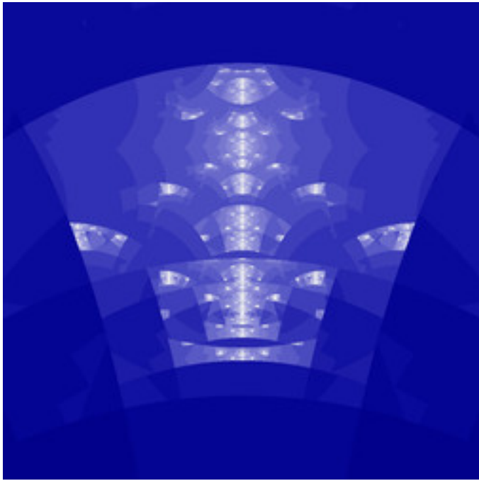
mt-rudys-cubic-mandelbrot-03.jpg
