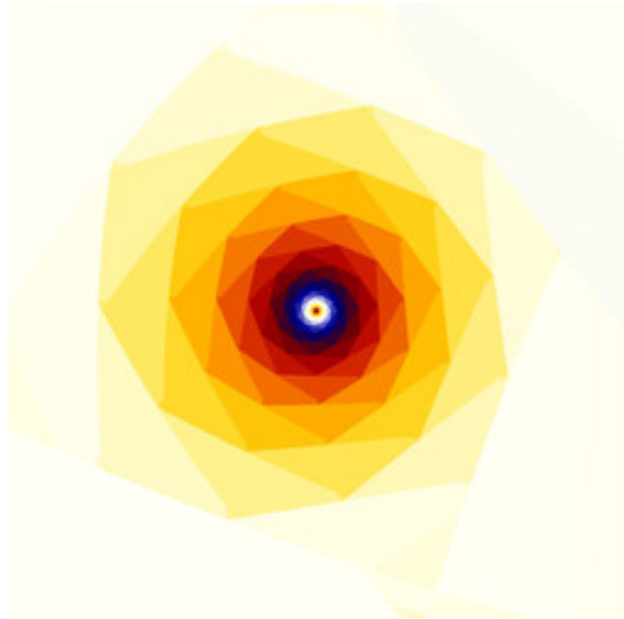
mt-Sign-I-Mset-02.jpg
