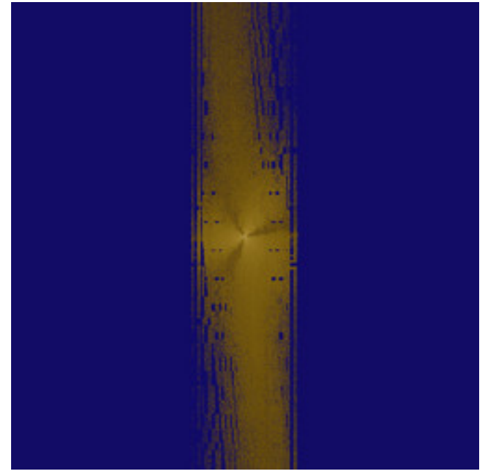
mt-newton-error-julia-03.jpg
