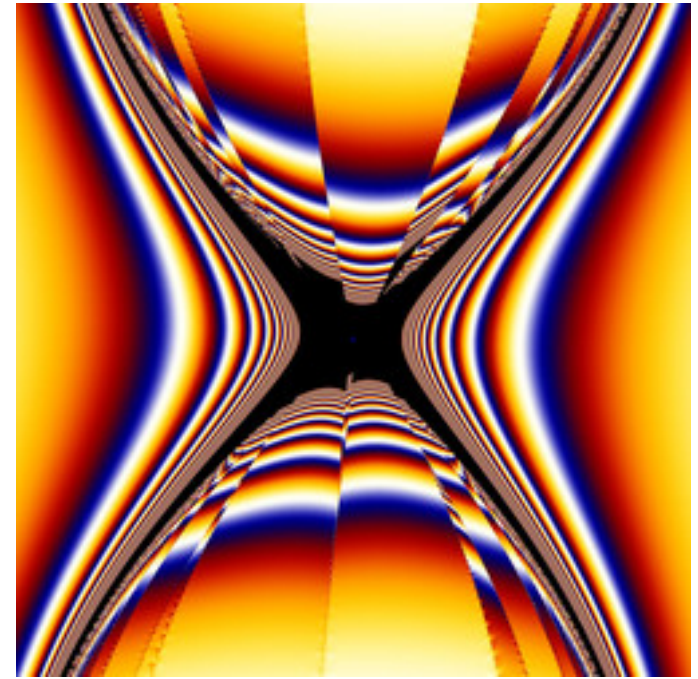
mt-newton-9904a-05.jpg
