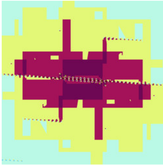
mt-zeepop-julia-30.jpg
