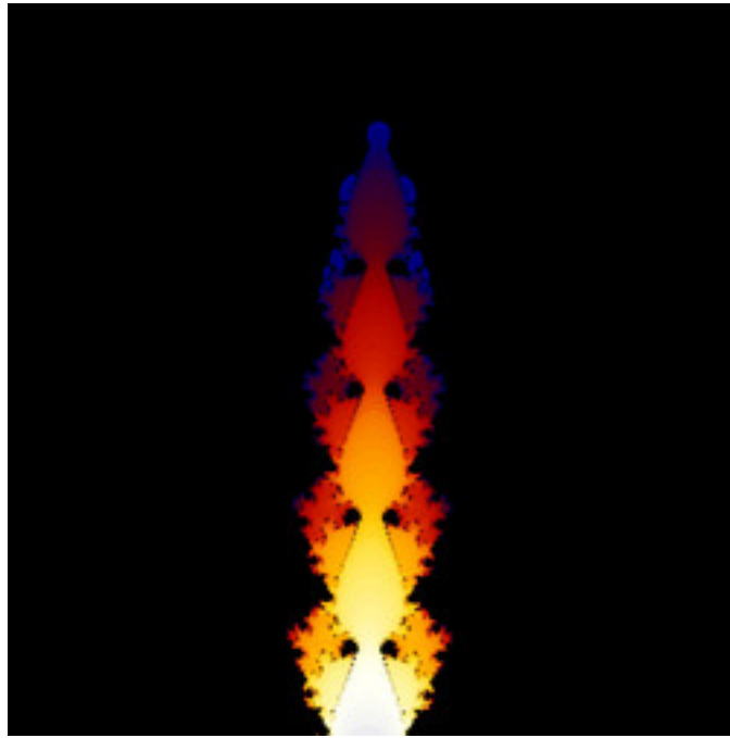
dmj-StutterMandel-02.jpg
