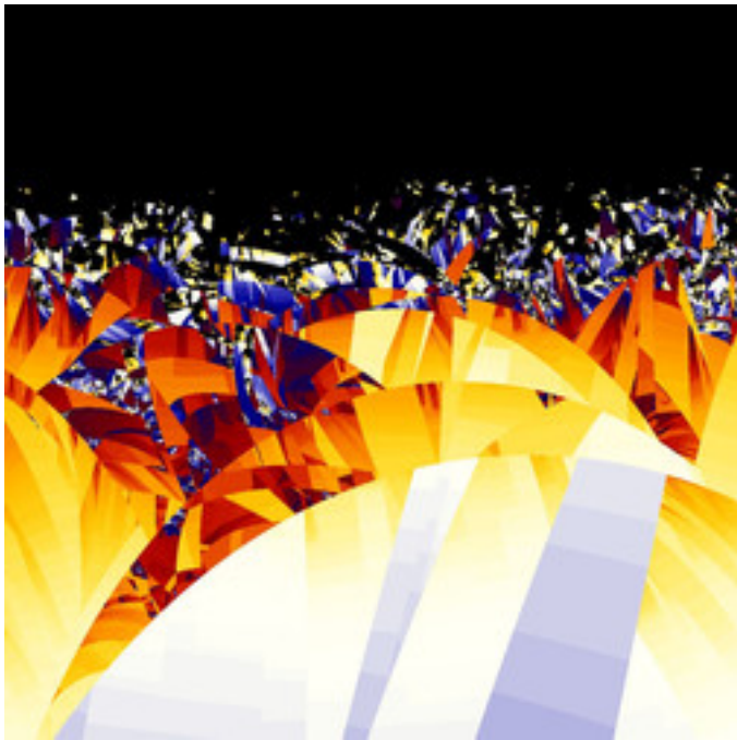
lkm-GeneralTentMandelbrot-NEW1-04.jpg
