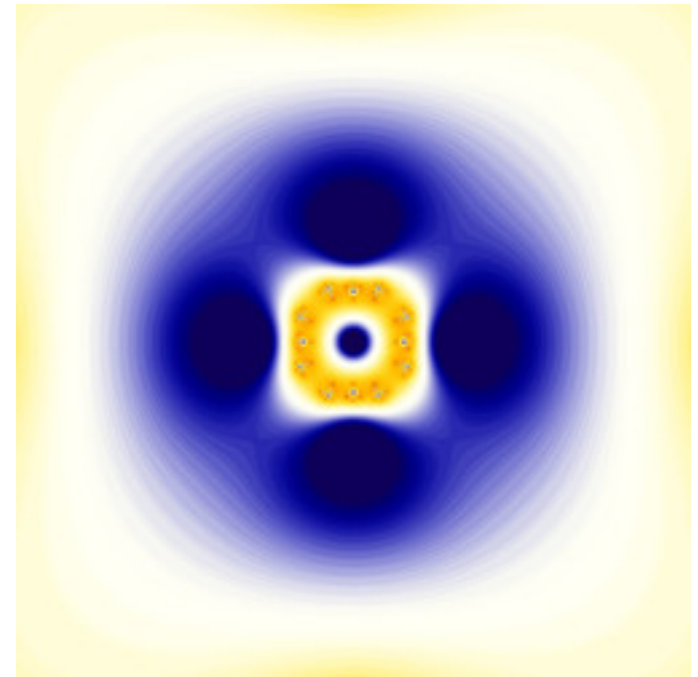
mt-rudys-cubic-mandelbrot-09.jpg
