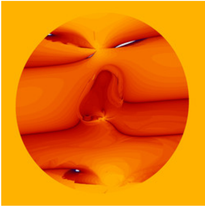
asz-andrextandom-1-18.jpg
