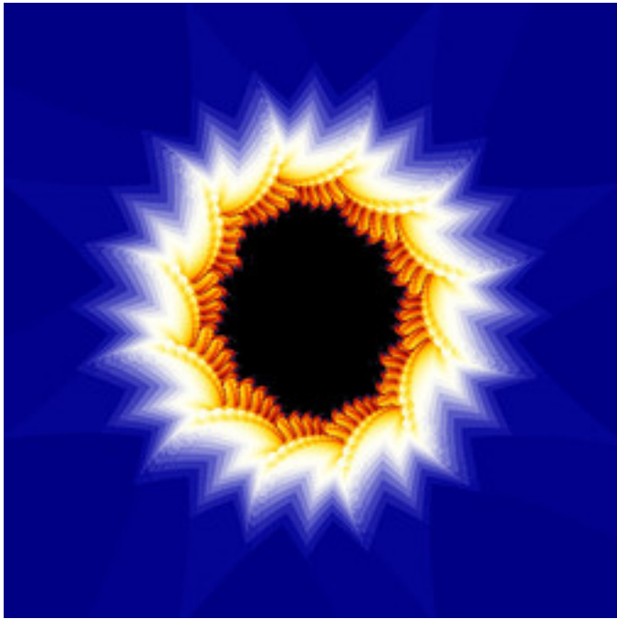
reb-JuliaTentMap-29.jpg
