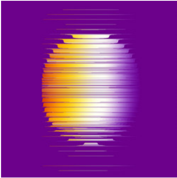
mt-GeneralizedCelticJulia-63.jpg
